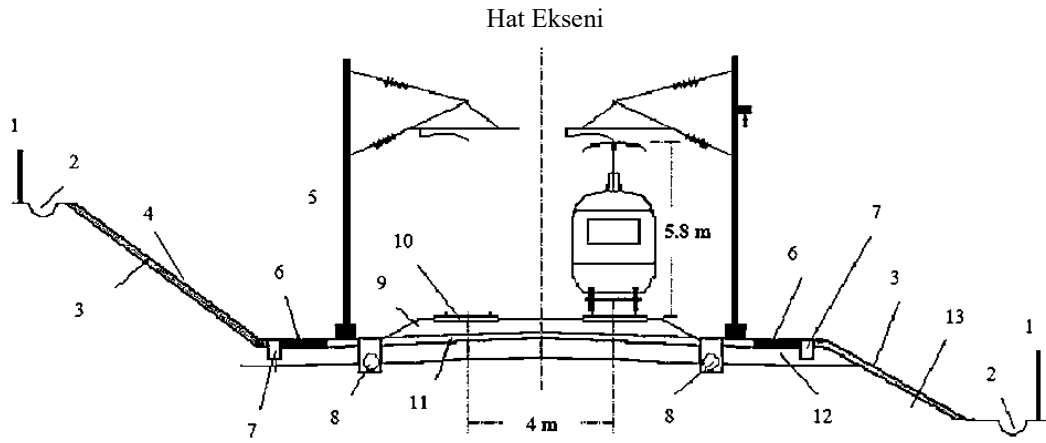
Şekil 2.1. Çift hatlı demiryolu enkesiti
