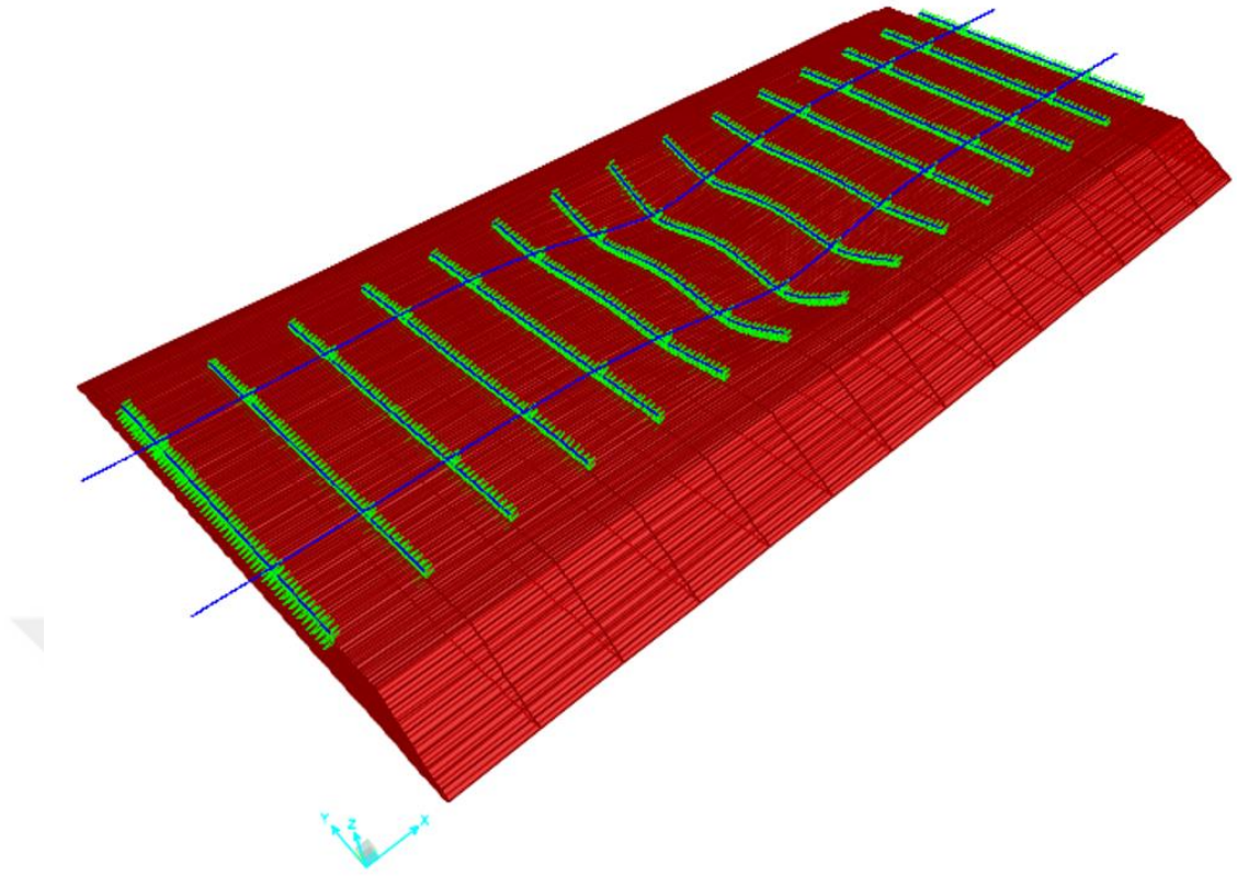
Şekil 7.10. Model-6'nın SAP2000'de analizi sonucu deforme olmuş hali
