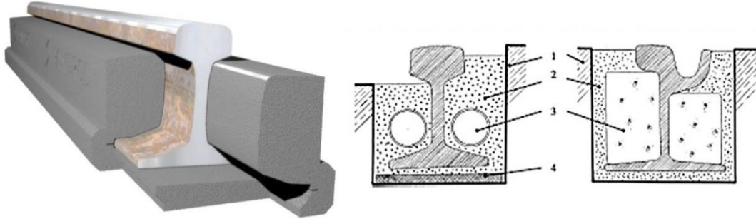
Şekil 3.10. Gömülü ve sıkılaştırılmış ray sistemi
