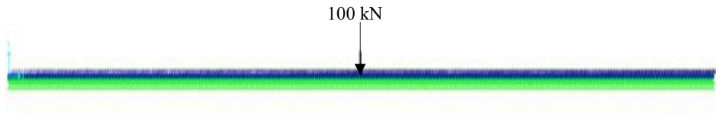
Şekil 7.1. Elastik yatağa oturan kiriş elemanın SAP2000 modeli
