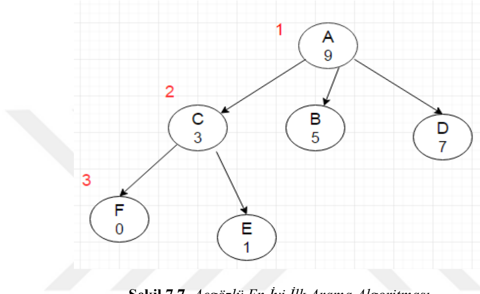
Şekil 7.7. Açgözlü En İyi İlk Arama Algoritması
