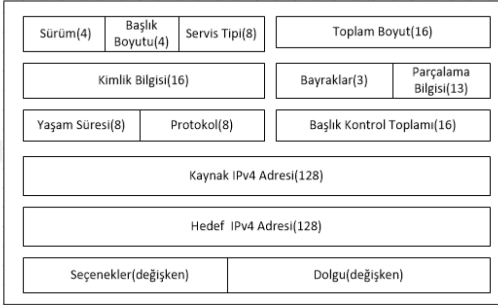
Şekil 2.1. Ipv4 Başlık Yapısı
