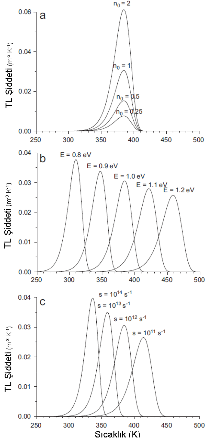
Şekil 3.4. Randall Wilkins birinci derece TL denkleminin özellikleri; (a) n_0 ışınlanmasından sonra, tuzaklanmış doz taşıyıcılarının yoğunlukla değişimi. (b) E , aktivasyon enerjisi ile değişimi (c) Parametre değerleri; n_0 = 1 \text{ m}^{-3} ; E = 1 \text{ eV} ; s = 1 \times 10^{12} \text{ s}^{-1} kaçış frekansı ile değişimi. Bütün eğriler için ısıtma hızı 1 \text{ K s}^{-1} 'dir. Belirlenen tepenin maksimum konumu n_0 'la değişmez [Boss, 2006].
