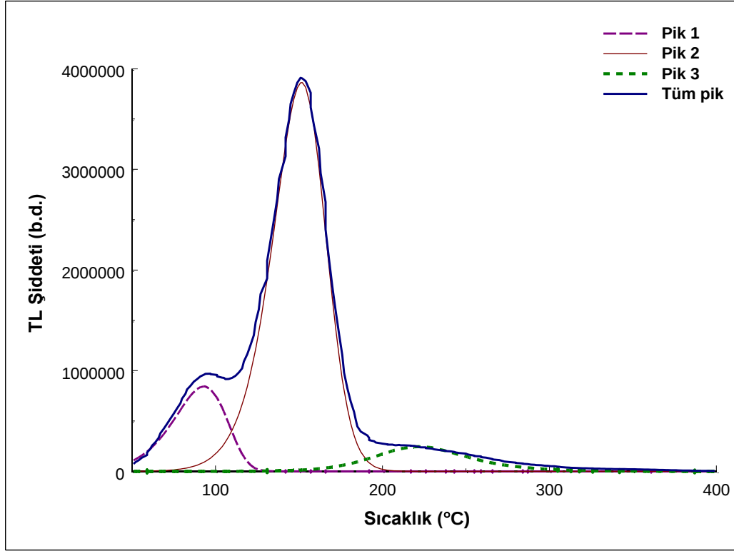
Şekil 6.7. YNbO 4 dozimetresinin 5dk UVB ışınlamasının ardından elde edilen TL ışıma eğrisi.
