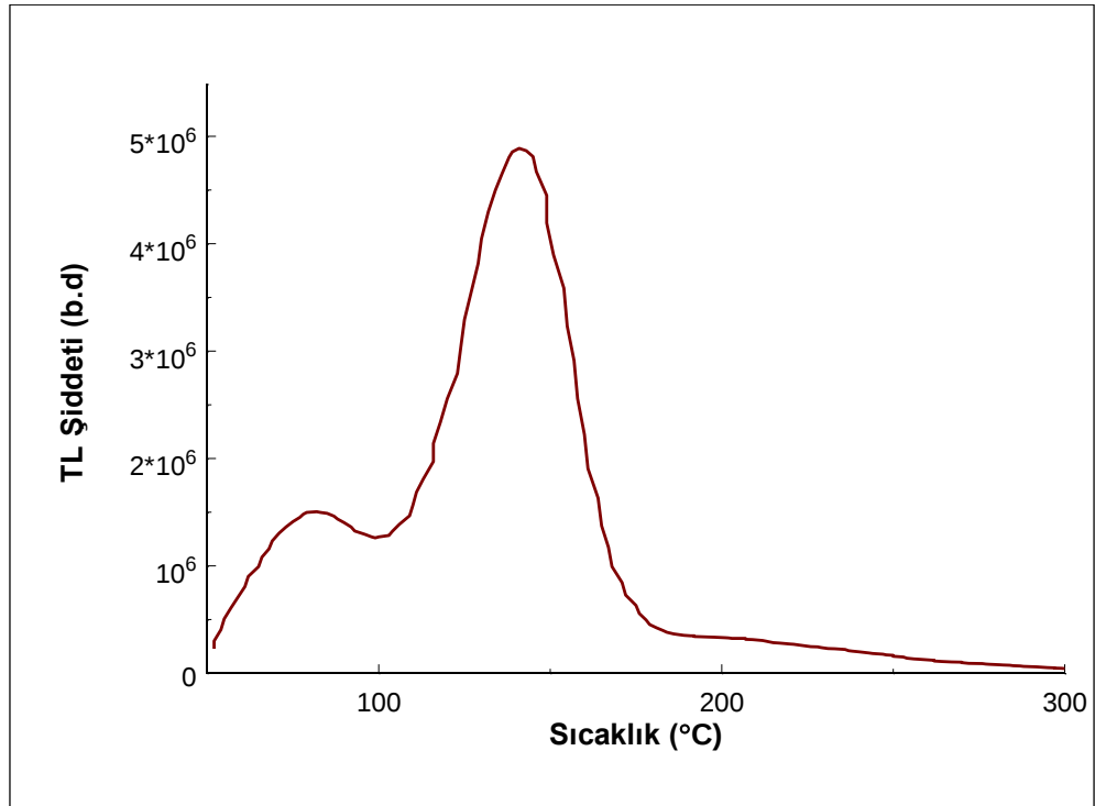
Şekil 2.4. ısıma eğrisi örneği. Her bir pik iyi tanımlanmış bir tuzaka karşılık gelmektedir.
