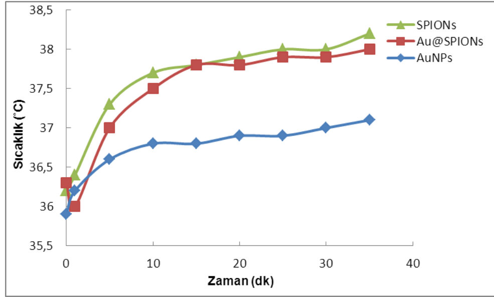
Şekil 40 5µg/ml derişimdeki nanopartikül çözeltilerinin 120w gücünde RF uygulaması ve zamana bağı sıcaklık artışı
