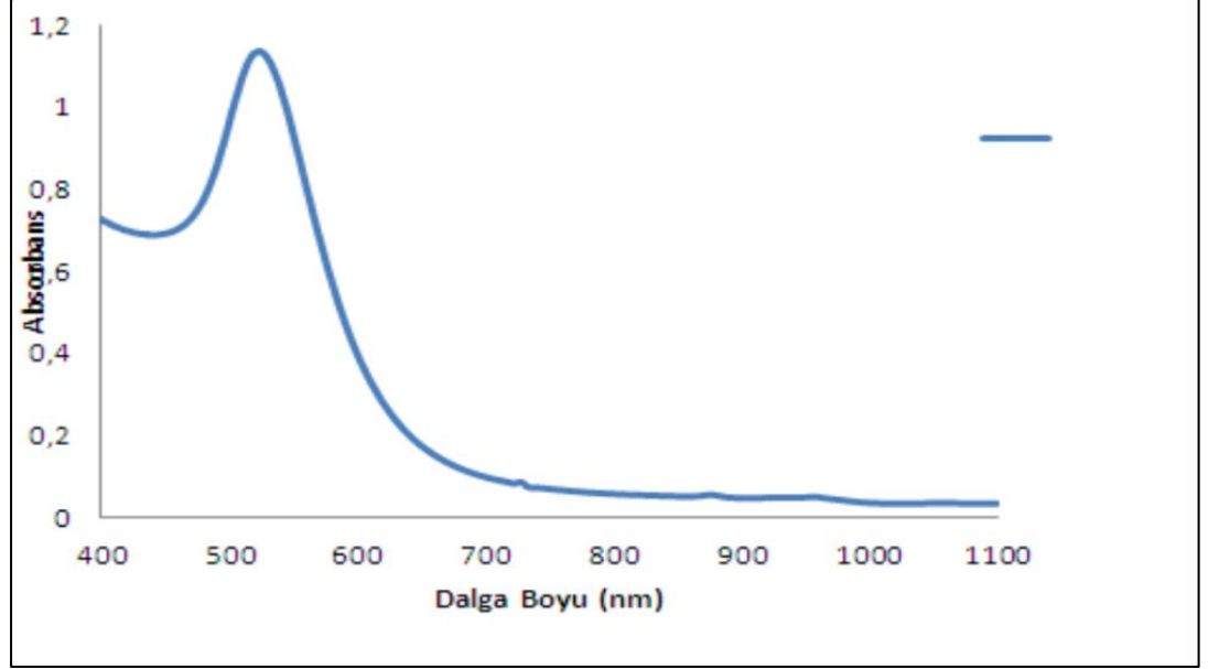
Şekil 20 Altın kaplı manyetit nanopartiküllerin UV/VIS absorbands verilerinin grafiği
