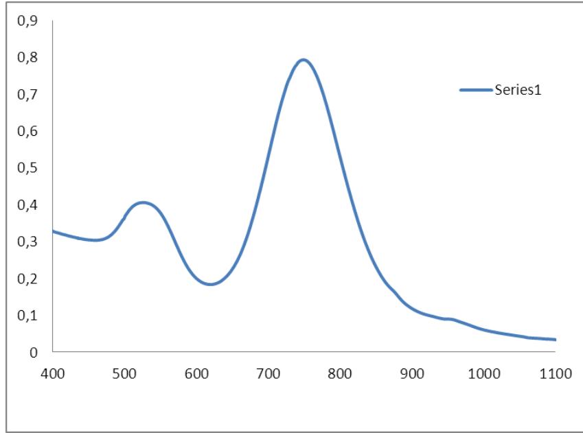
Şekil 26 Altın nanorodların UV/VIS absorbands spektrısı
