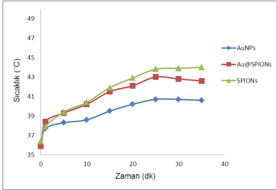
Şekil 33 30µg/ml yoğunlukta olan farklı nanopartiküllerin 180W RF uygulaması ve sıcaklık artışının değerlendirilmesi
