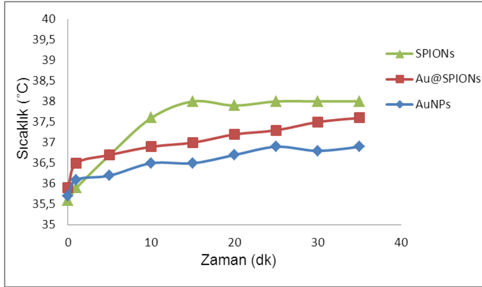
Şekil 38 15 µg/ml derişimdeki nanopartikül çözeltilerinin 80W gücünde RF uygulaması ve zamana bağı sıcaklık artışı
