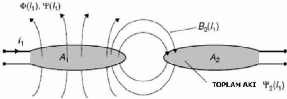
Şekil 2.18. İki Bobinin Oluşturduğu Karşılıklı Endüktans
