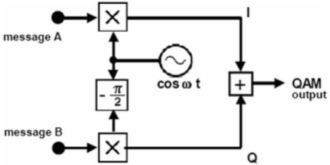
Şekil 2.28. QAM(QPSK) Modülatörü
