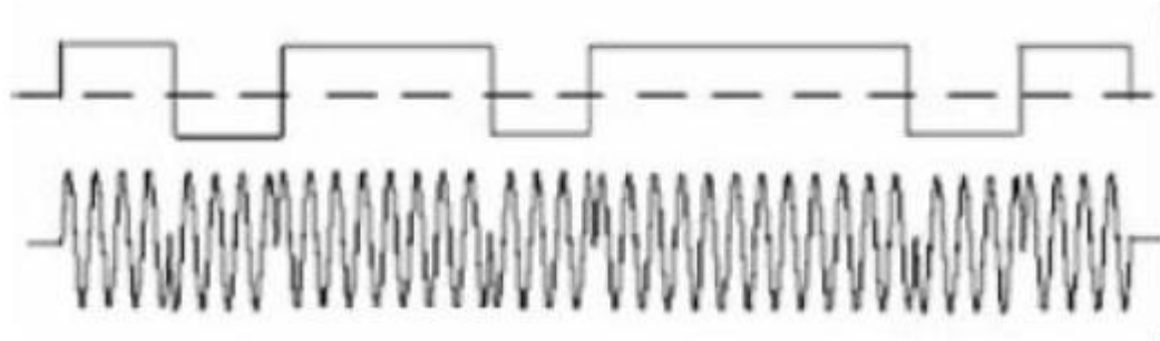
Şekil 2.27. BPSK İşareti
