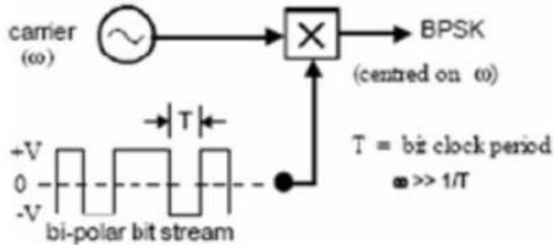
Şekil 2.26. BPSK İşaretinin Üretilmesi
