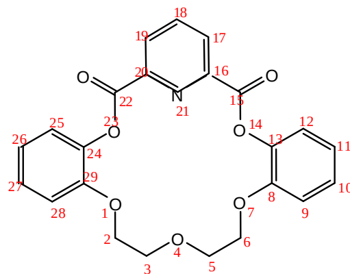
15,22-diokso-1,4,7,14,23-pentaoksa-(7)(1,2)benzeno(2)(2,6)pridino(2)(1,2)benzenofan
