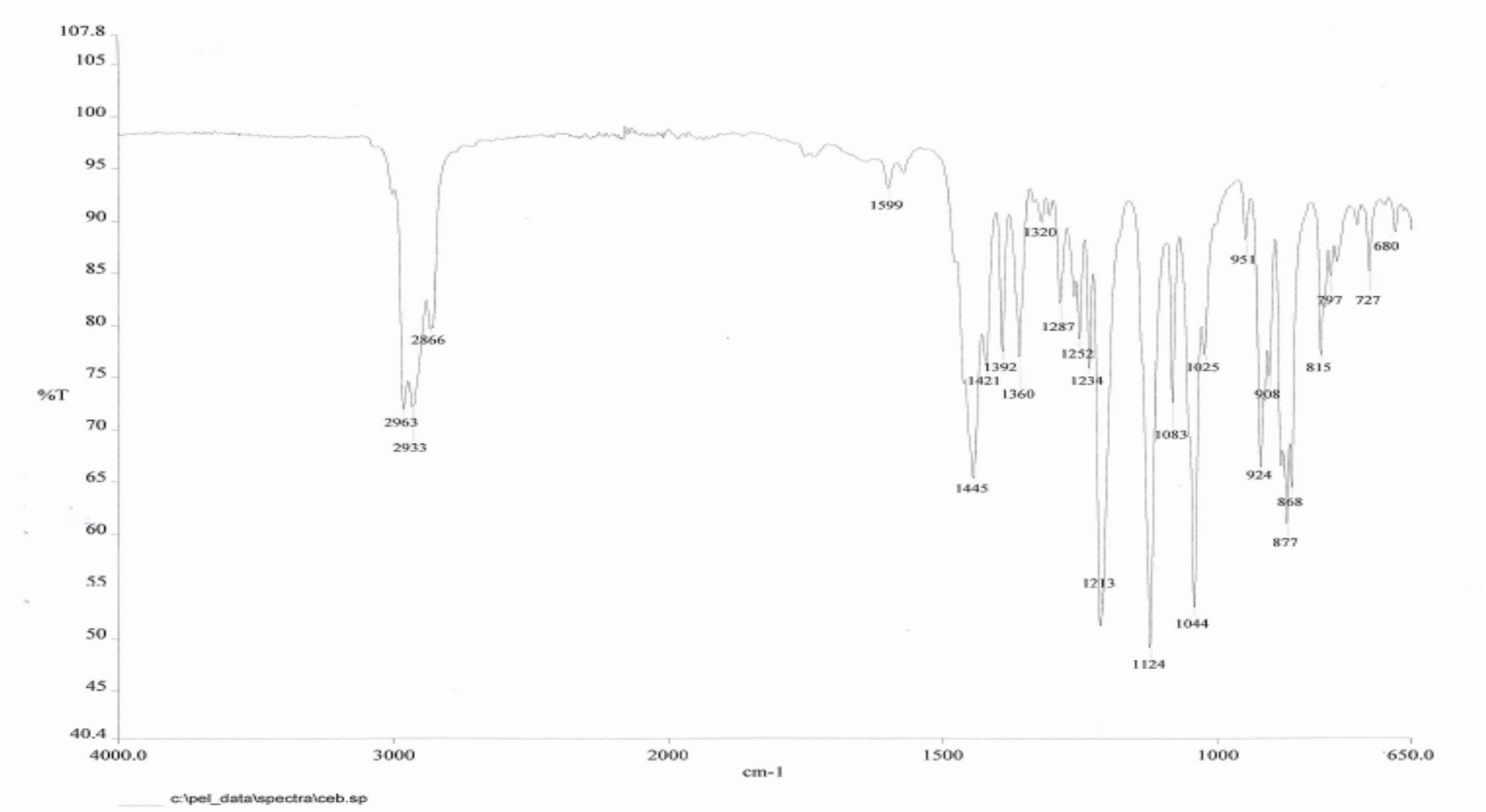
5 nolu bileşik
