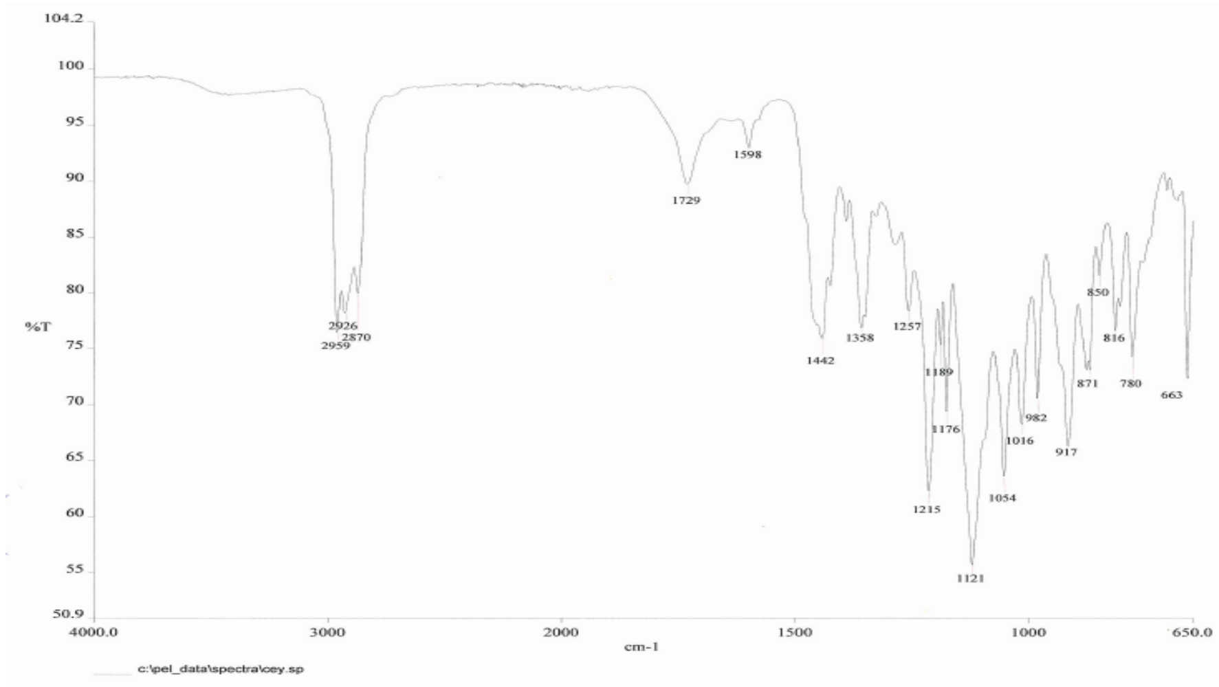
6 nolu bileşik
