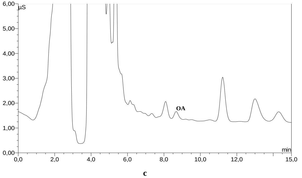
Şekil 6.2 (devam) : 1:250 seyreltilmiş patolojik idrar numunesinin a) 80 mM isoc b) 70 mM isoc c) 60 mM isoc alınan kromatogramlar (tR sırasıyla; 6,2, 6,4, 8,5 dk).
