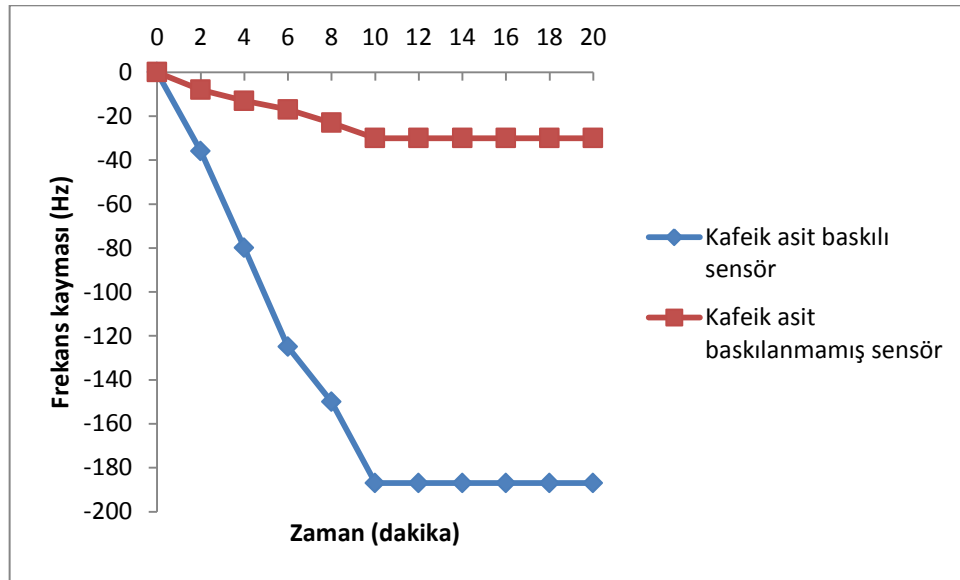
Şekil 4.9. Kafeik asit baskılanmış ve baskılanmamış nanosensörün frekans değerleri
