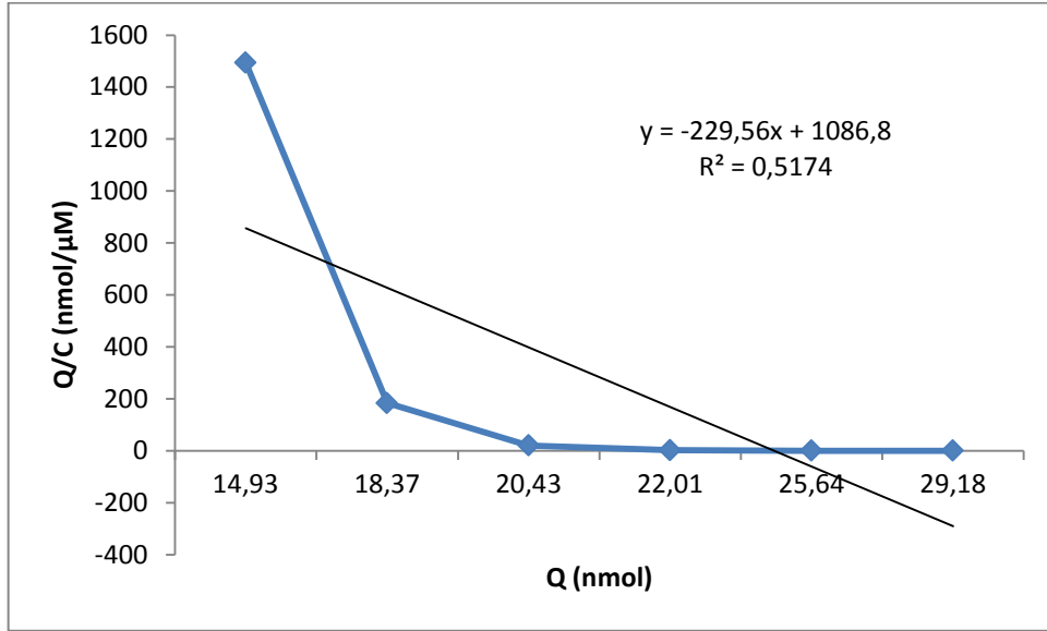
Şekil 4.10. Kafeik asit baskılı polimerin Scatchard eğrisi
