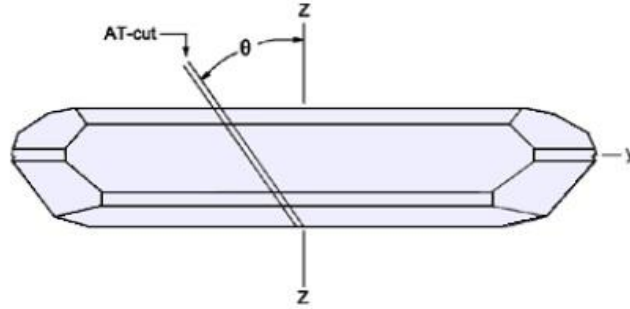
Şekil 1.3. AT kesim kuvars kristal (Kanazawa et al., 2009)
