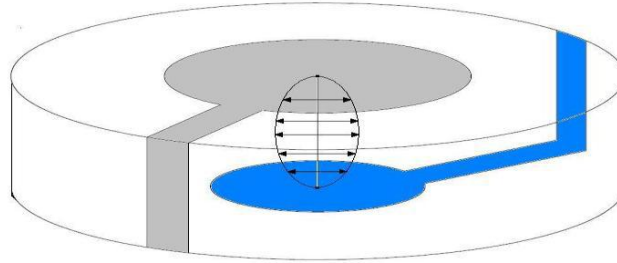
Şekil 1.4. Disk biçimindeki kuvars kristalin ve elektrotları arasında oluşan kararlı dalganın n=1 için gösterimi
