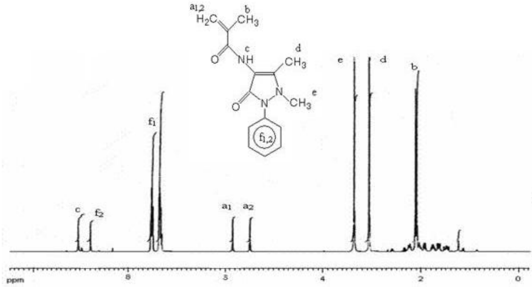
Sekil 4.2. MAAP monomerinin ^1\text{H} -NMR spektrumu
