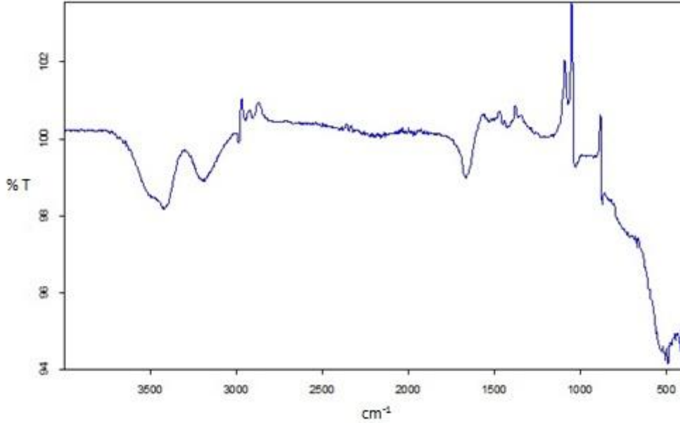
Sekil 4.4. MAAP-Fe-kafeik asit kompleksinin FTIR spektrumu
