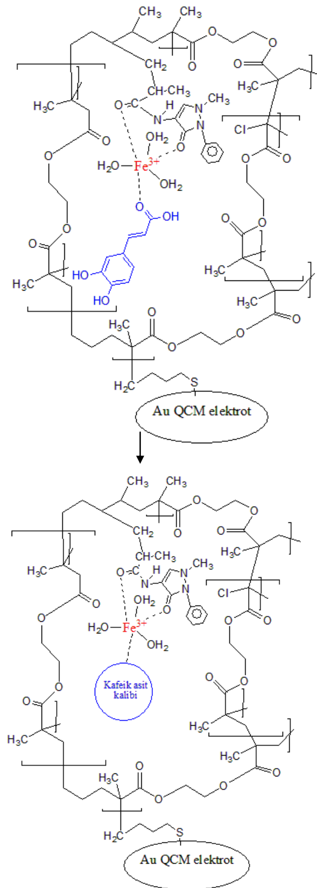
Sekil 3.2. QCM nanosensör yüzeyindeki kafeik asit bellek oluşumu
