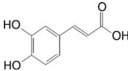
Şekil 1.1. Kafeik asidin kimyasal yapısı
