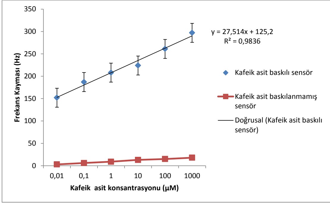
Şekil 4.14. Kafeik asit baskılı sensör için kalibrasyon grafiği
