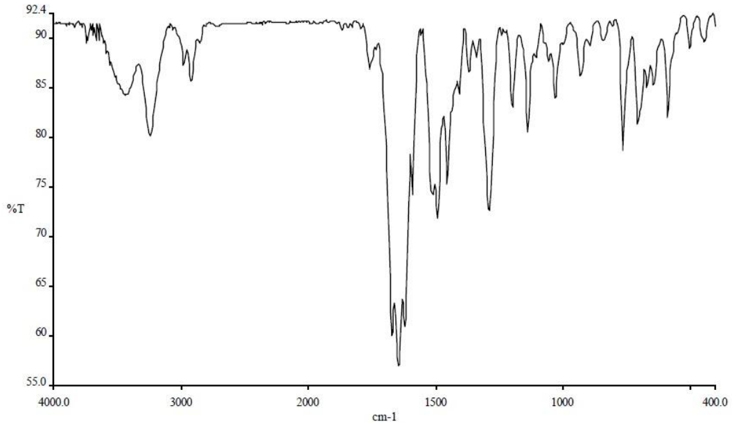
Sekil 4.3. MAAP-Fe kompleksinin FTIR spektrumu
