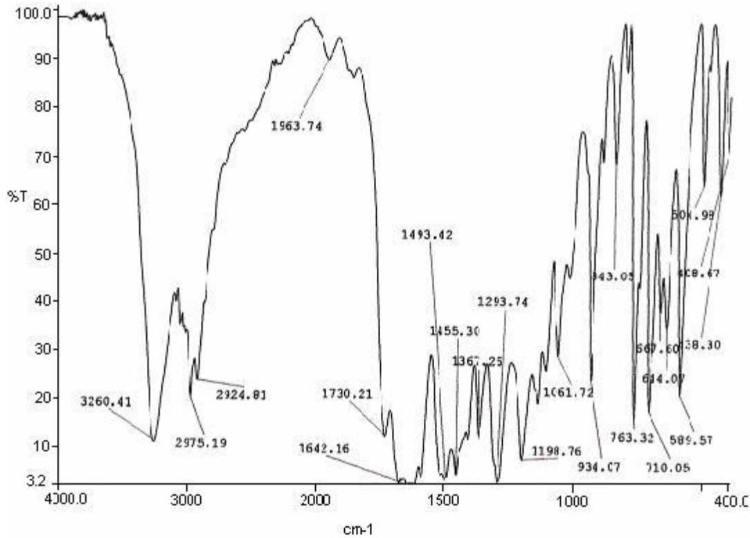
Sekil 4.1. MAAP monomerinin FTIR spektrumu
