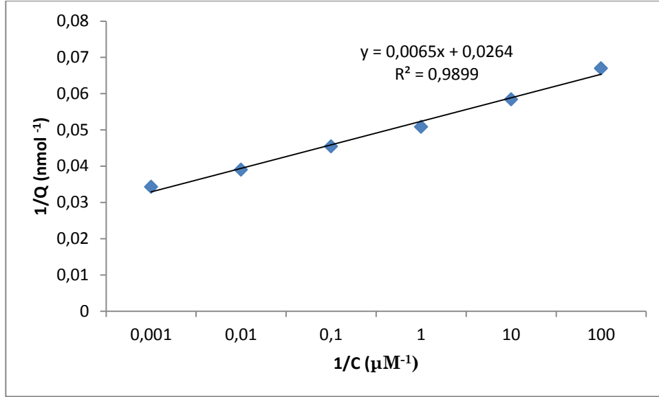
Şekil 4.11. Kafeik asit baskılı polimerin Langmuir eğrisi
