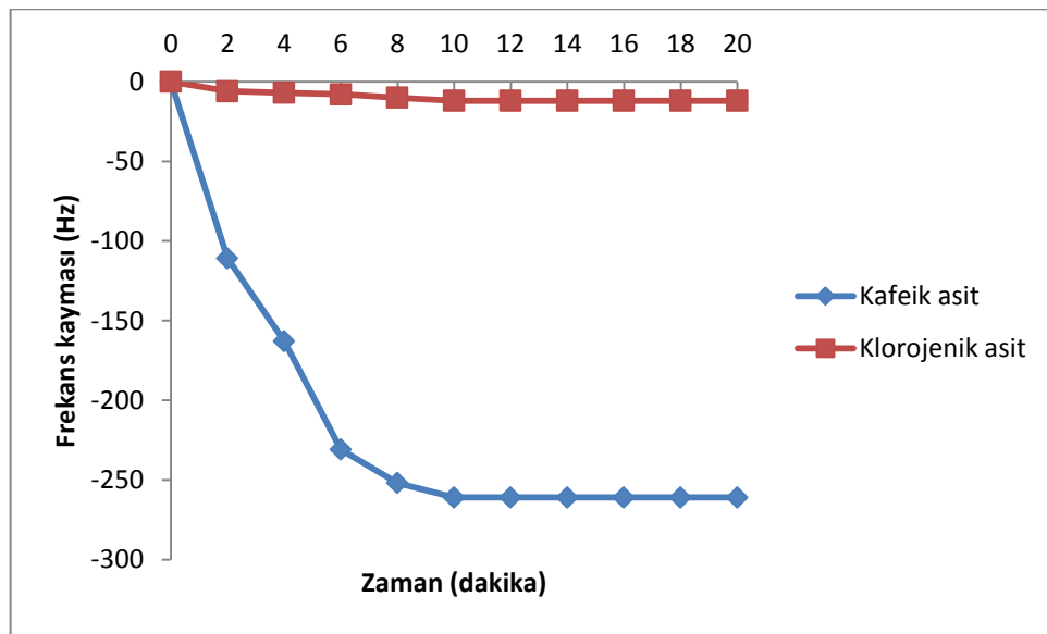
Şekil 4.13. Kafeik asit baskılı sensörün kafeik asit ve klorojenik asit için frekans değerleri (100 \mu M için)
