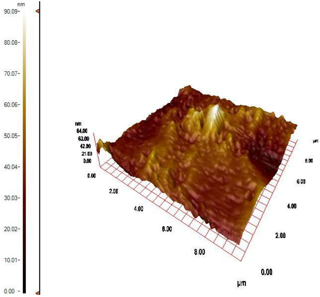
Şekil 4.7. Allil mercaptan ile modifiye edilmiş QCM elektrotun altın yüzeyinin AFM görüntüsü
