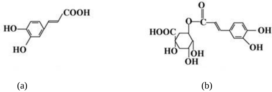
Şekil 4.12. (a) Kafeik asit (b) Klorojenik asidin kimyasal yapısı
