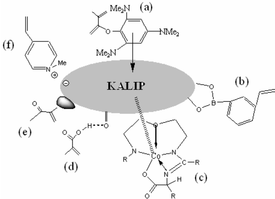
Şekil 1.7. Moleküler baskılanmış polimerlerde kalıp-fonksiyonel monomer etkileşimleri: (a) p-p etkileşimi, (b) kovalent etkileşim, (c) metal-ligand etkileşimi, (d) hidrojen bağı ile etkileşim, (e) hidrofobik ya da van der Waals etkileşimi, (f) iyonik etkileşim
