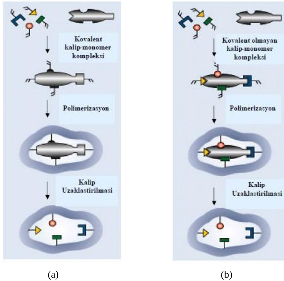
Sekil 1.6. (a) Kovalent ve (b) kovalent olmayan moleküler baskılama yönteminin şematik görünümü
