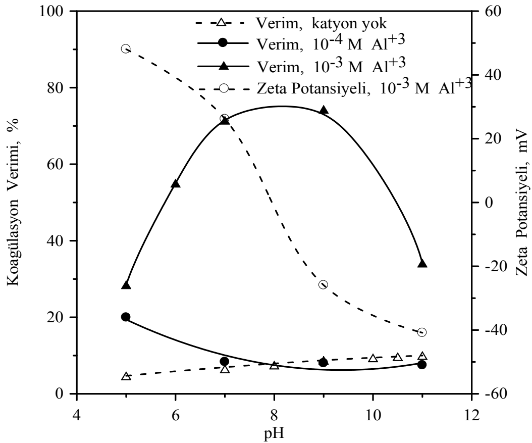
Şekil 4.9. Al^{+3} iyonu varlığında zeolit koagülasyonunu üzerine pH'ın etkisi.
