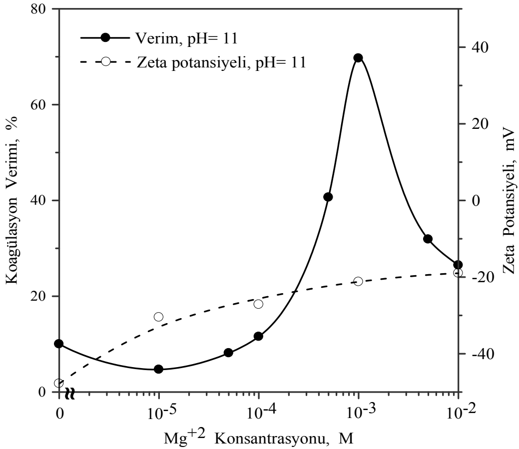
Şekil 4.5. pH 11’de Mg 2+ iyonu konsantrasyonunun zeolitin koagülasyonuna etkisi
