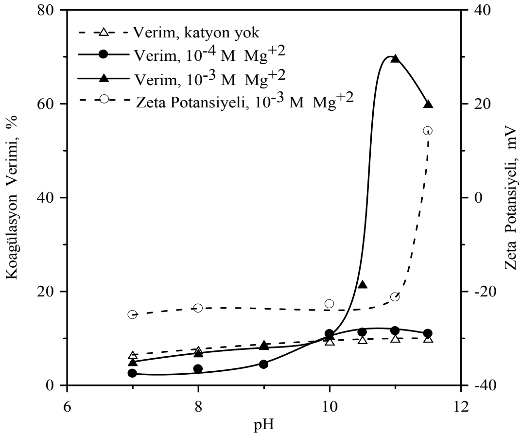
Şekil 4.3. \text{Mg}^{+2} iyonu varlığında zeolit koagülasyonu üzerine pH'ın etkisi.
