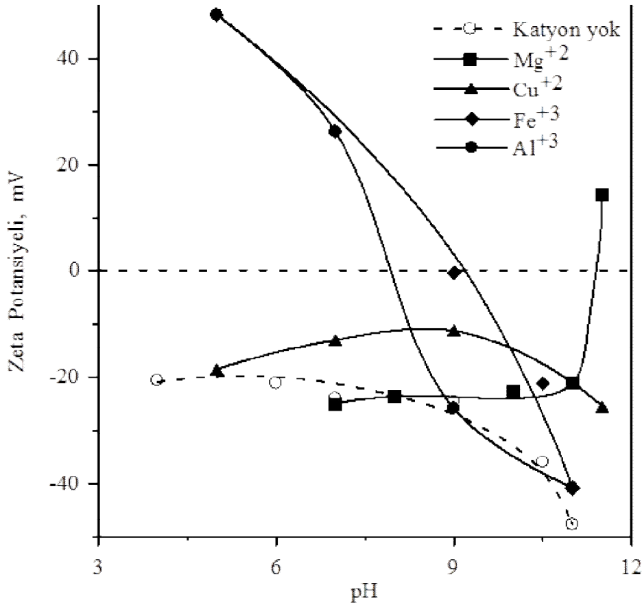
Şekil 4.2. 10^{-3} M Mg^{+2} , Cu^{+2} , Al^{+3} ve Fe^{+3} iyonu konsantrasyonunda zeolit pH'a bağlı olarak zeta potansiyelinin değişimi.
