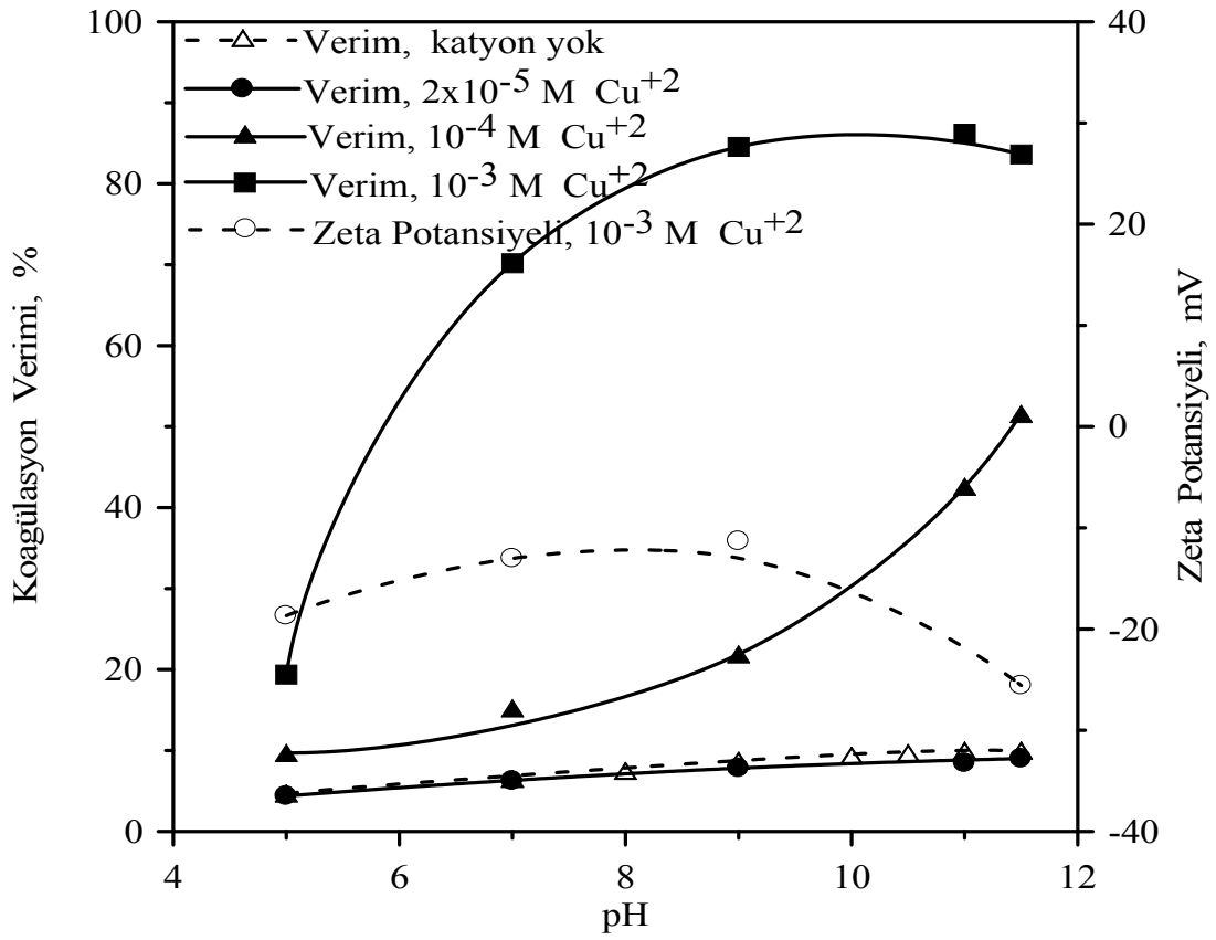
Şekil 4.6. \text{Cu}^{+2} iyonu varlığında zeolit koagülasyonu üzerine pH'nin etkisi.
