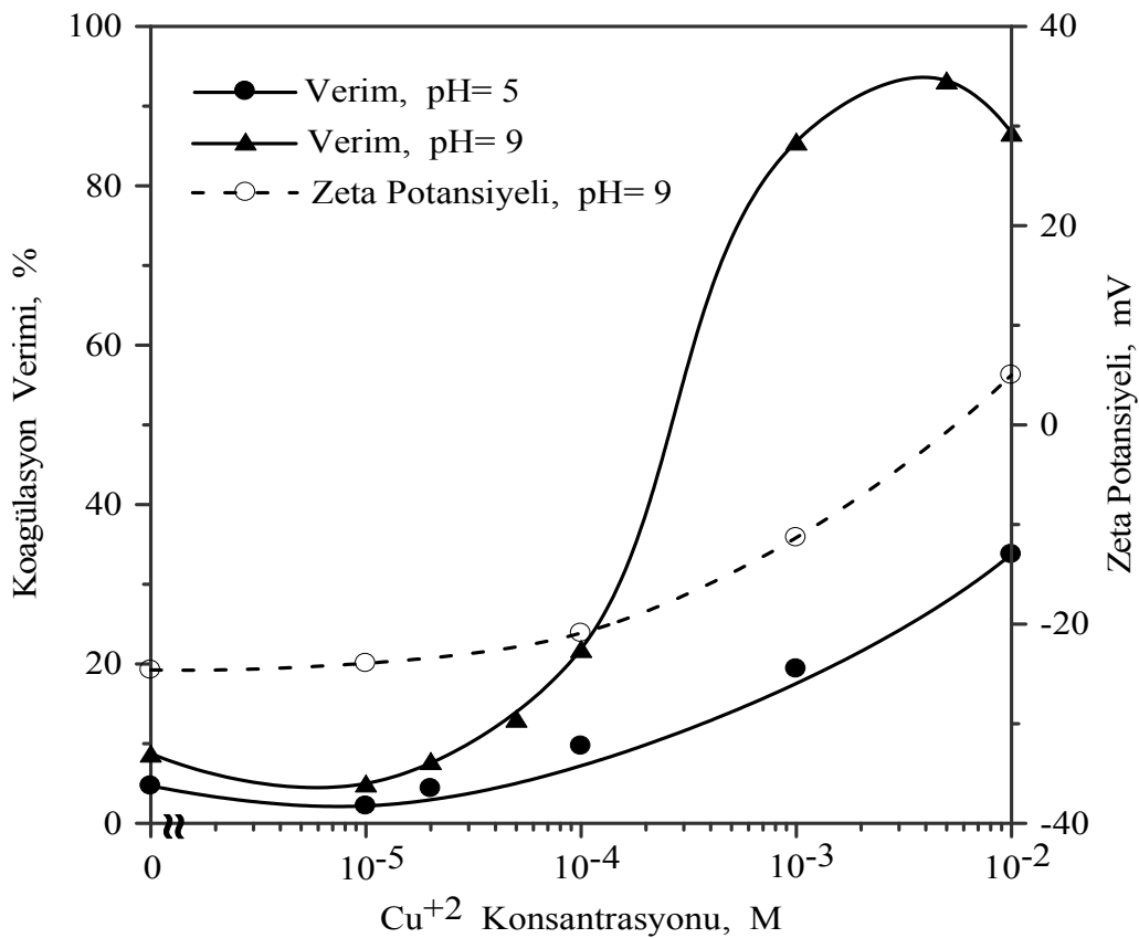
Şekil 4.8. Farklı pH'larda \text{Cu}^{+2} iyonu konsantrasyonunun zeolitin koagülasyonuna etkisi.
