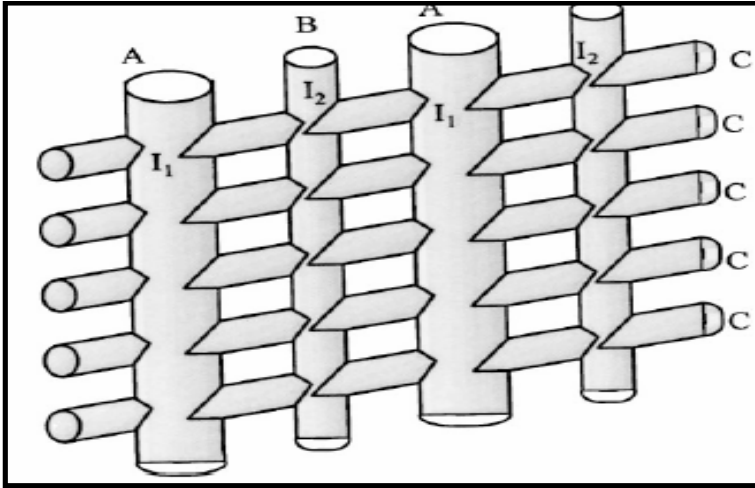
Şekil 2.4. Klinoptilolitin temsili kanal yapısı (Hernandez ve Corona, 2000).
