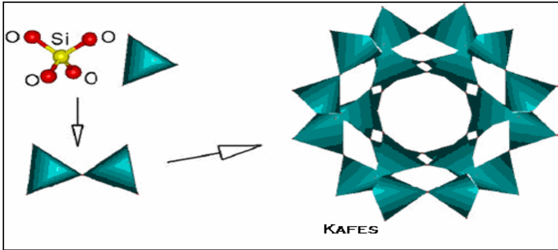
Şekil 2.2. SiO 2 tetrahedralarından oluşan zeolit kafesi
