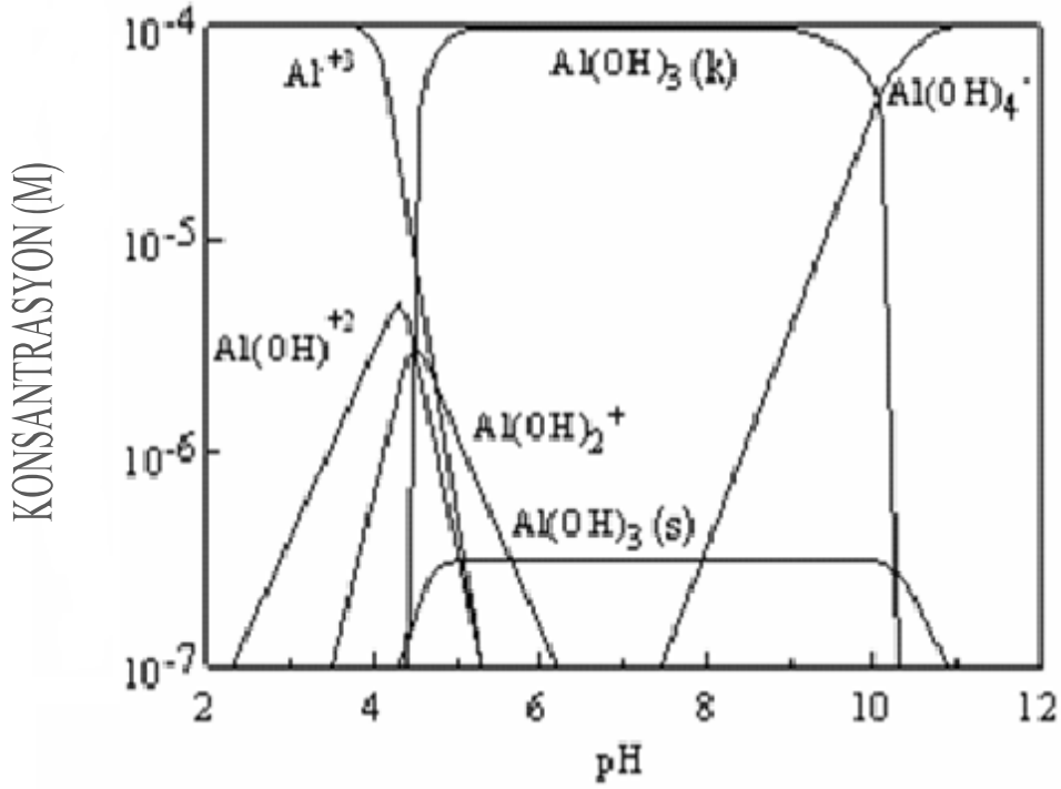
Şekil 4.10. 10^{-4} M \text{Al}^{+3} iyonu için pH'a bağlı tür diyagramı (Kragten, 1978).
