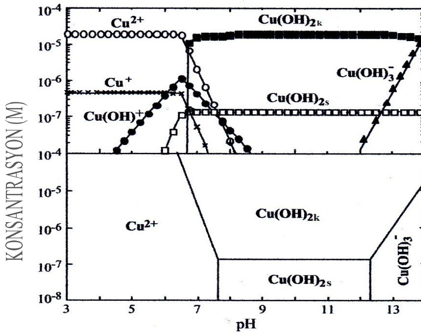
Şekil 4.7. 2 \times 10^{-5} M \text{Cu}^{+2} iyonu için pH'a bağlı tür diyagramı (Pugh ve Tjus, 1987).
