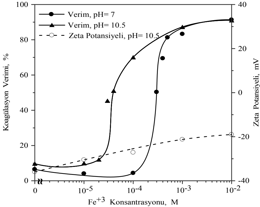
Şekil 4.14. Farklı pH'larda \text{Fe}^{+3} iyonu konsantrasyonunun zeolit koagülasyonuna etkisi.
