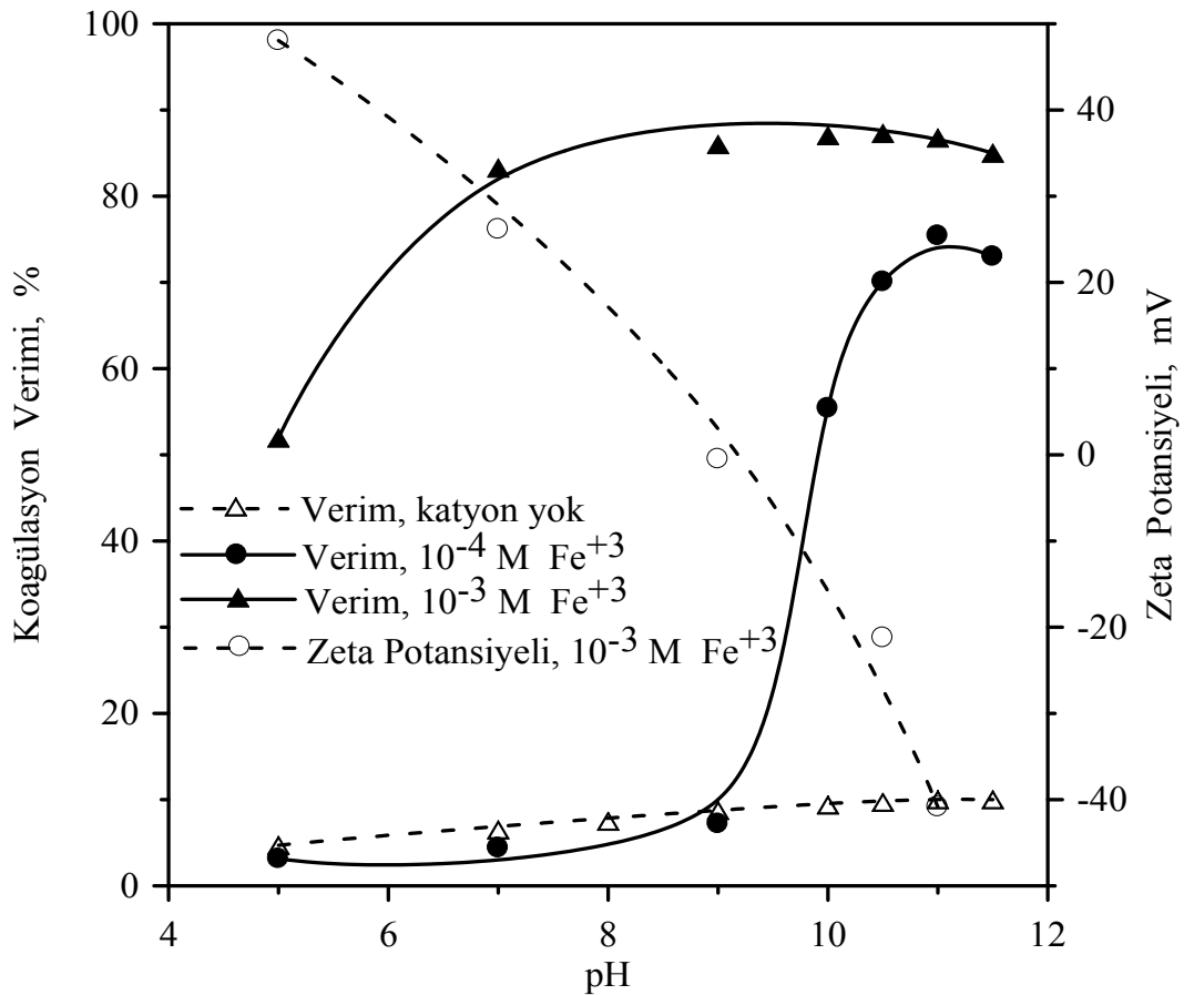
Şekil 4.12. \text{Fe}^{+3} iyonu varlığında zeolitin koagülasyonunu üzerine pH'nın etkisi.
