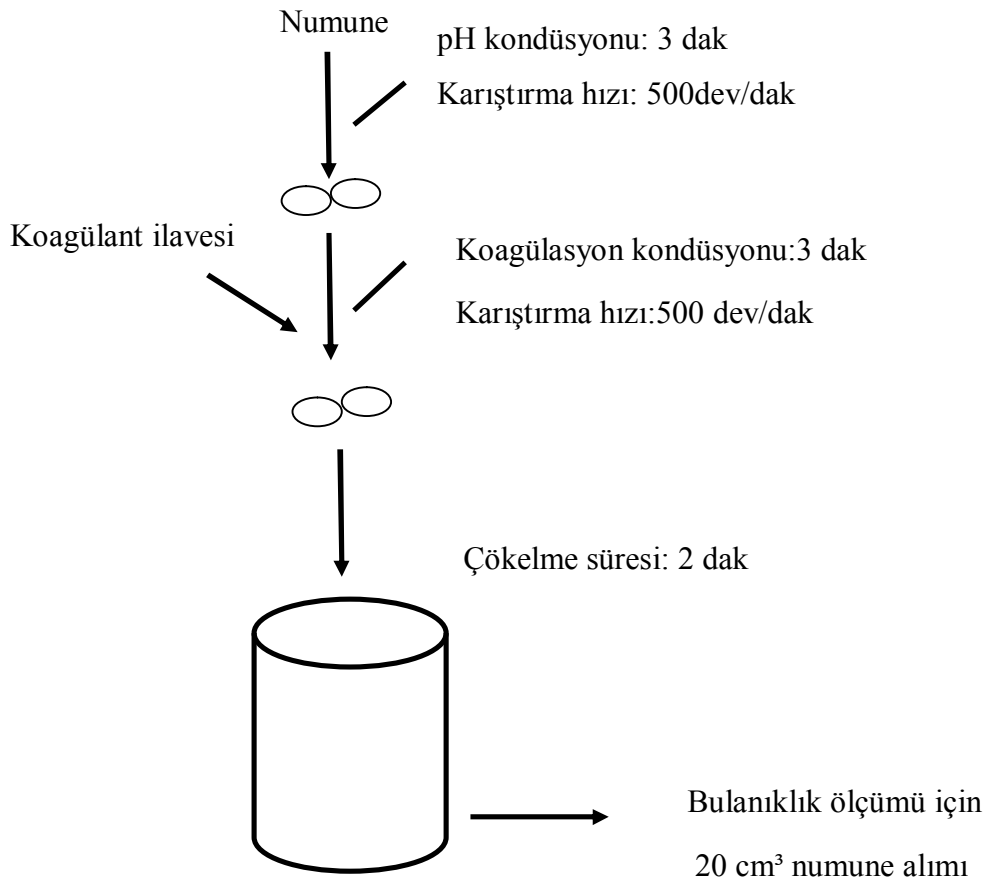
Şekil 3.1. Koagülasyon deneylerinde izlenen akım şeması
