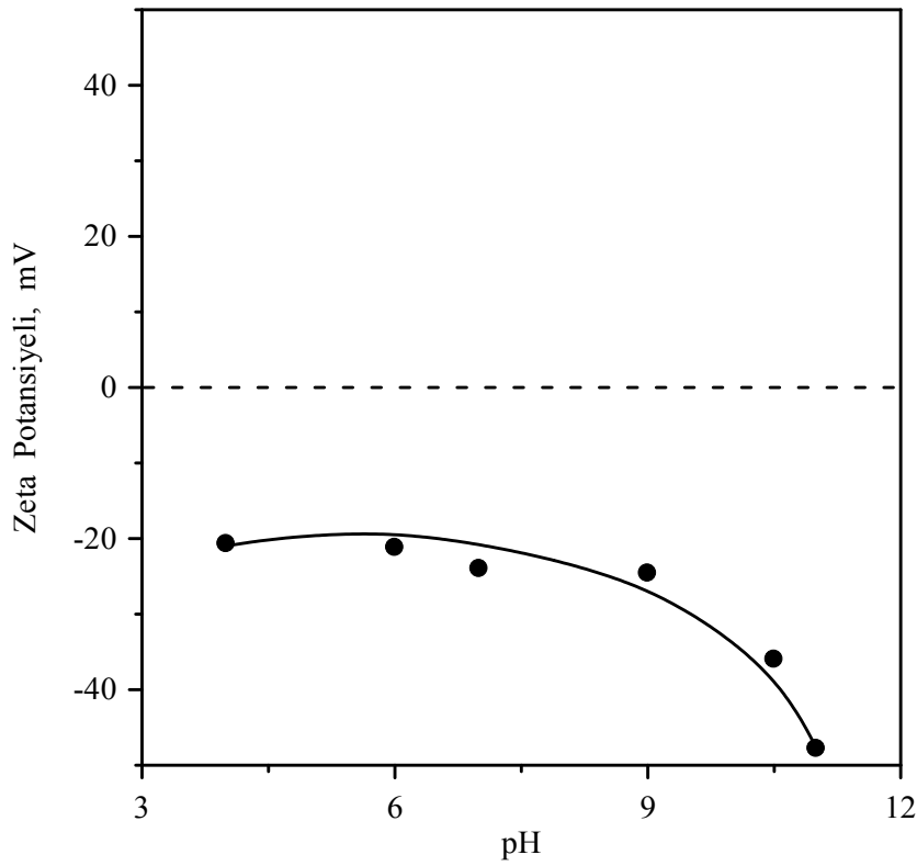
Şekil 4.1. Zeolitin pH'a bağlı olarak zeta potansiyelinin değişimi.
