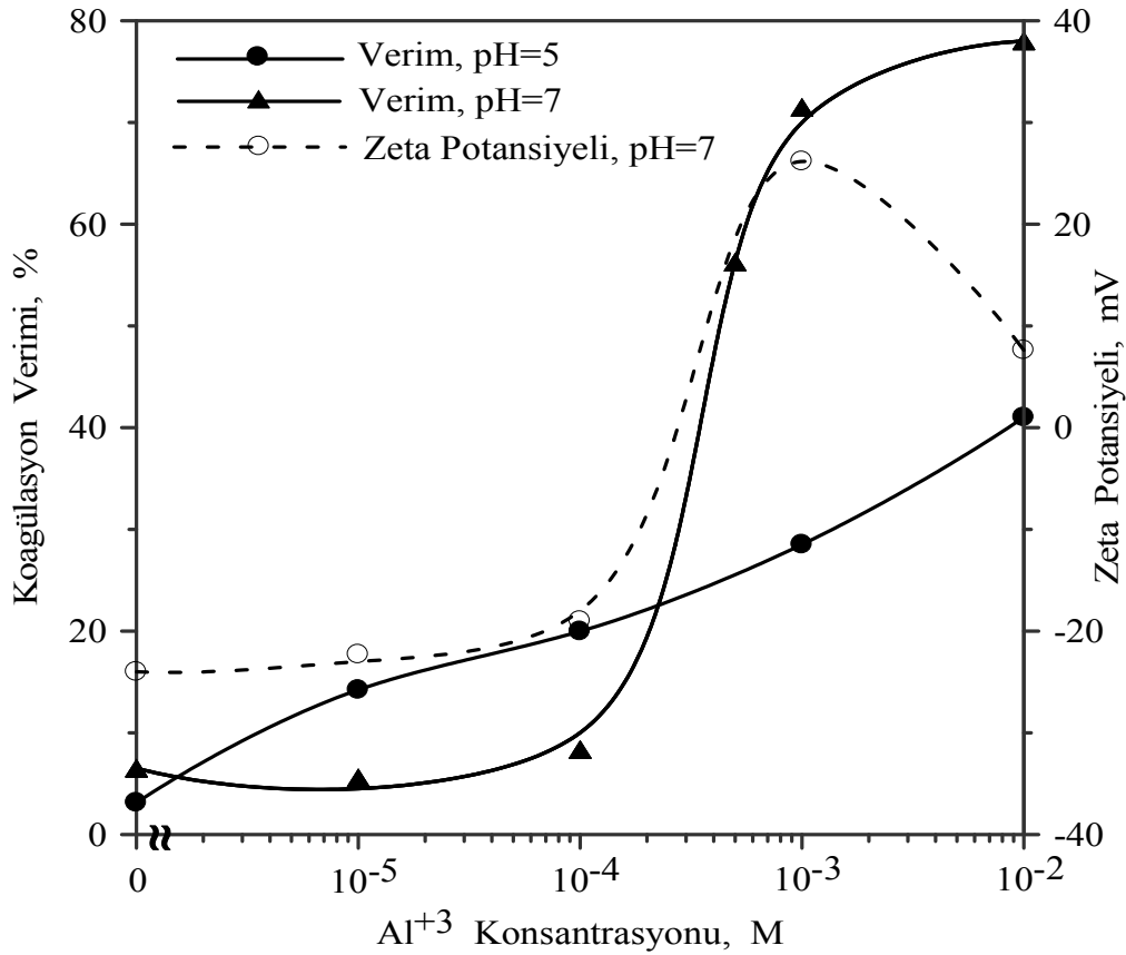
Şekil 4.11. Farklı pH'larda Al 3+ iyonu konsantrasyonunun zeolitin koagülasyonuna etkisi.
