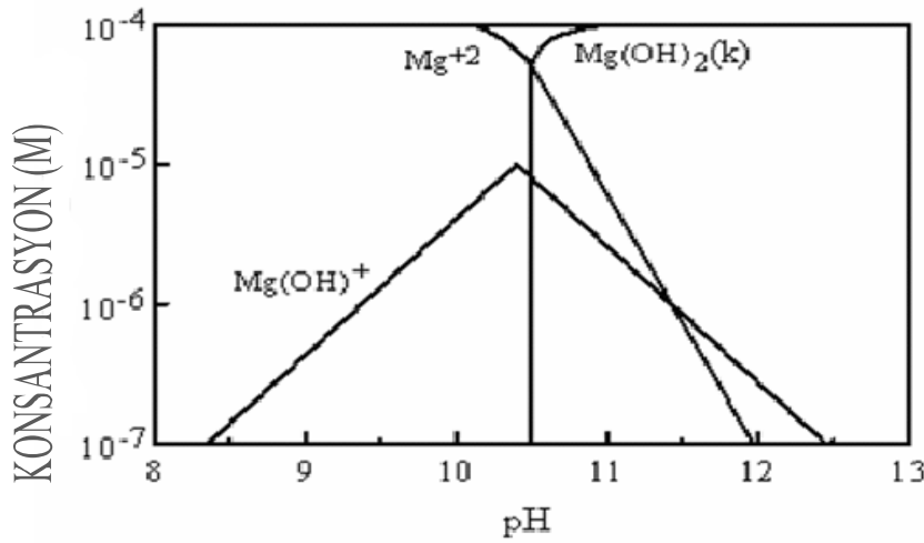
Şekil 4.4. 10^{-4} M Mg^{+2} iyonu için pH'a bağlı tür diyagramı (Butler, 1964).
