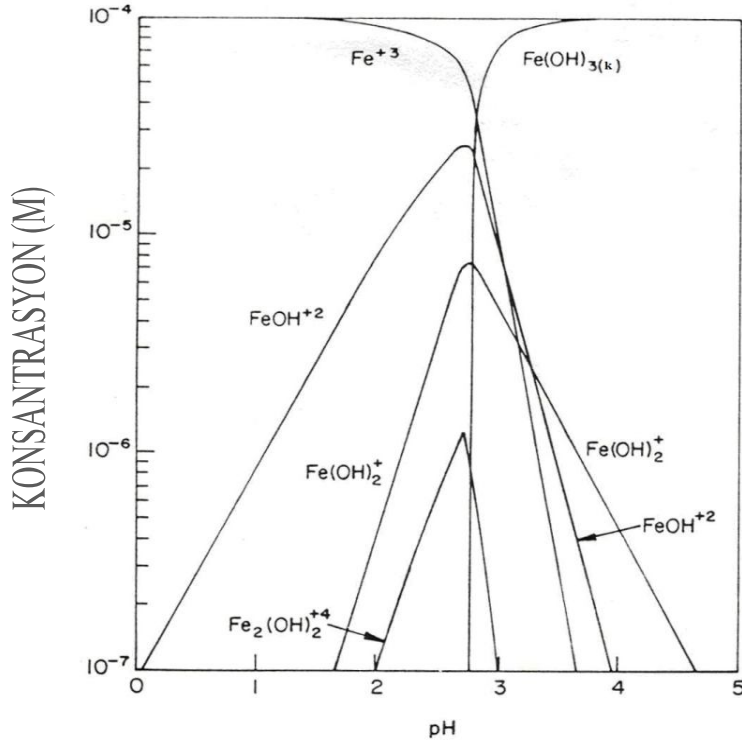
Şekil 4.13. 10^{-4} M \text{Fe}^{+3} iyonu için pH'a bağlı tür diyagramı (Butler, 1964).
