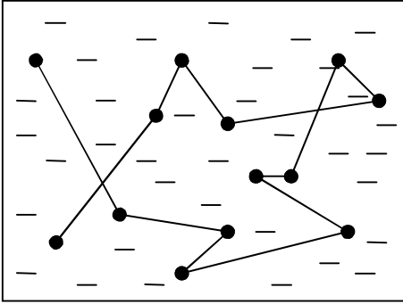
Şekil 2.6. Kolloidal patikülün Brown hareketi ile yer değiştirmesi
