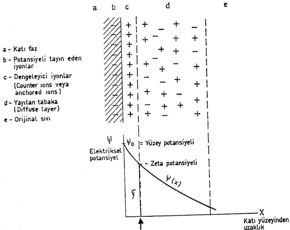
Şekil 2.8. Elektriksel çift tabaka ve zeta potansiyeli (İpekoğlu, 1985)
