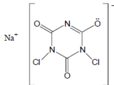
Şekil 2.8. Sodyum dikloroizosiyanürat molekül yapısı.
