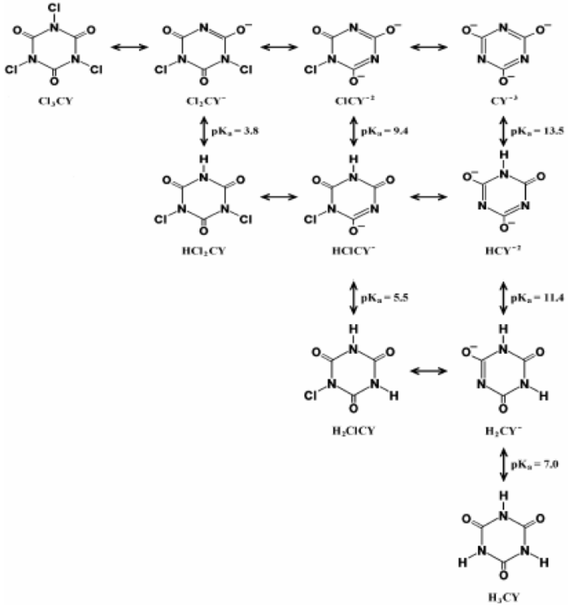
Şekil 2.10. İzosiyanürat ve kloroizosiyanüratların denge reaksiyonları (Kuznesof, 2004).
