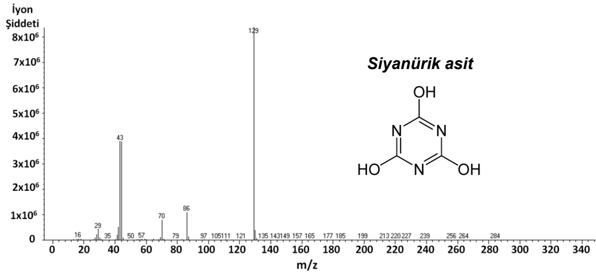
Şekil 4.17. Gübre içerisindeki ürenin yakılması ile elde edilen ham siyanürik asidin toplam iyon kromatogramındaki 1 no'lu pike (siyanürik asit'i tanımlamaktadır) ait kütle spektrumu.
