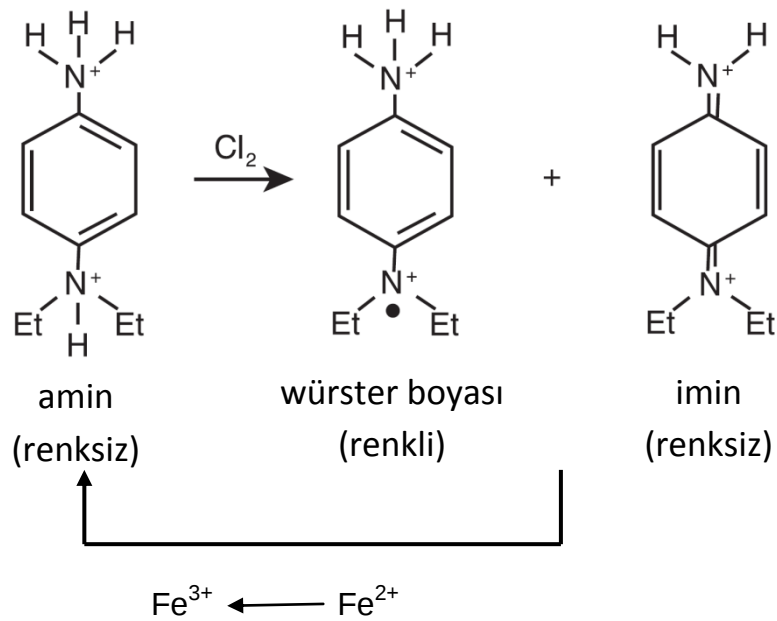
řekil 2.4. DPD titrasyonu (Harp, 2002).
