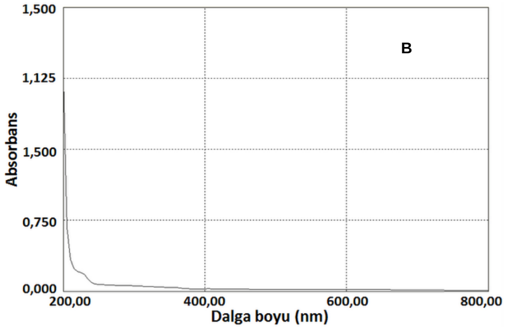
Şekil 4.4. UV – Görünür bölge spektrumları. (A) Siyanürük asit ve (B) üre.
