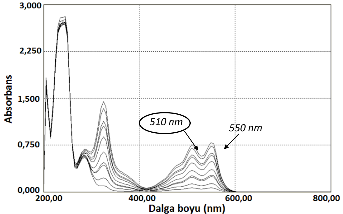
Şekil 4.1. Serbest klor – DPD komplekslerinin farklı \text{Ca}(\text{OCl})_2 derişimlerindeki absorpsiyon spektrumlarındaki değişim.
