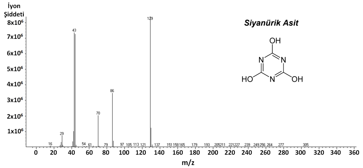
Şekil 4.8. Saf siyanürik asidin Katı Prop-MS kütle spektrumu.
