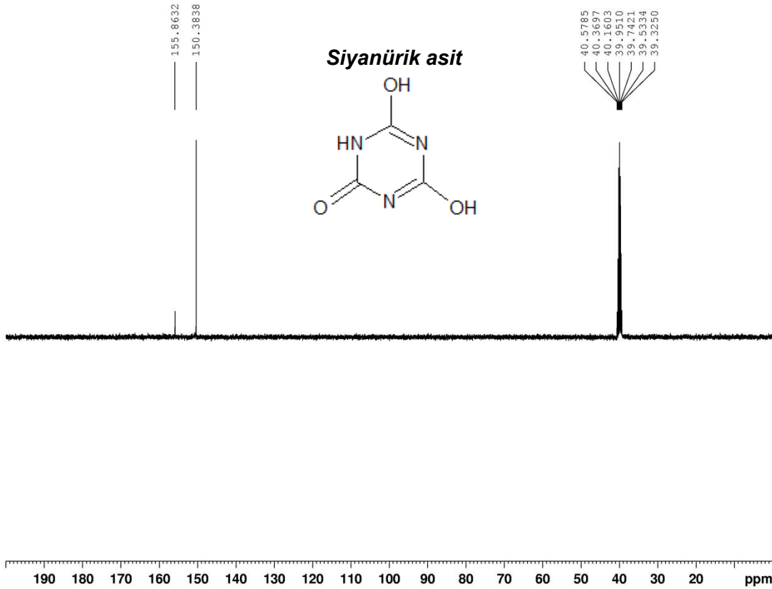
Şekil 4.30. Kerosen içerisinde gerçekleştirilen sıvı faz siyanürük asit sentezi sonucunda oluşan ham siyanürük asidin 0,5 M HCl ile hidroliz işlemi gerçekleştirildikten sonra elde edilen ürüne ait APT ^{13}\text{C} NMR spektrumu (Çözücü: dötero dimetil sülfoksit).
