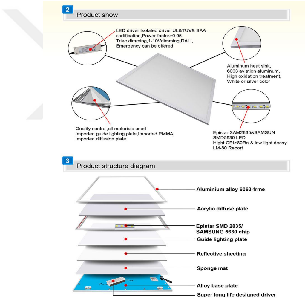
Şekil 8.5 60x60 LedPanel aydınlatmalı armatür şematik şekli
