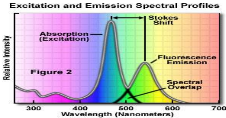
Şekil 3.14: Uyarma ve emisyon eğrileri
