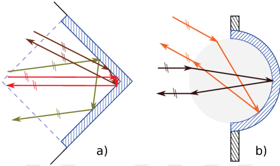
Şekil 4.9: Retroreflektör: a) Köşe küp geri yansıtıcı, b) Küresel retroreflektör (kedi gözü).
