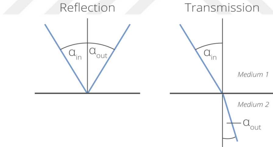
Şekil 4.15: Doğrudan yansıtıldığında veya doğrudan iletilildiğinde, tek yönlü bir ışın geometrik optik yasalarına uyar: doğrudan yansıma (sol): \alpha_{in} = \alpha_{out} , doğrudan iletim (sağ): n_1 \times \sin(\alpha_{in}) = n_2 \times \sin(\alpha_{out}) ilgili ortamın kırılma indisini gösteren n_1 ve n_2 ile \sin(\alpha_{out})
