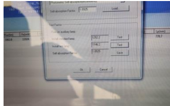
11. Öz soğurma katsayı (self-absorption factor) sonucu
