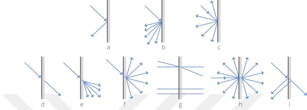
Şekil 4.14: Doğrudan, karışık ve dağınık yansıma alt: doğrudan, karışık ve dağınık iletim
