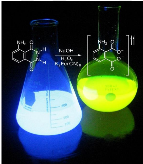
Şekil 3.15: Luminol testi. Büyük miktarda ışık üreten bir erlenmeyer şişesinde gerçekleştirilen kemo-ışıldayan bir reaksiyon.
