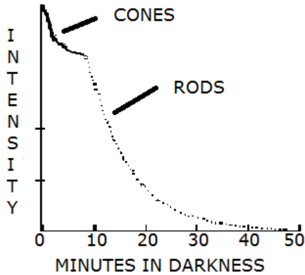
Şekil 6.8: Karanlık Adaptasyon grafiği
