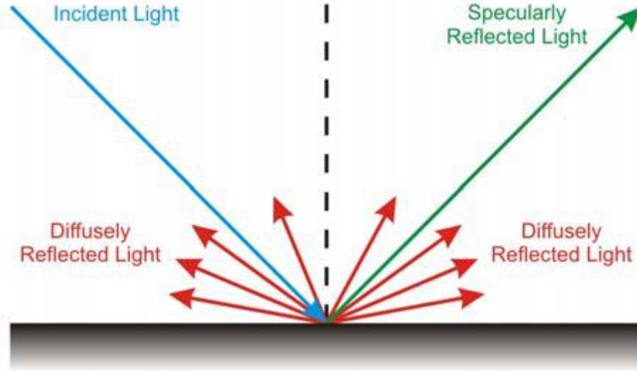
Şekil 4.12: Karışık yansıma, aynasal ve yaygın yansımanın bir kombinasyonudur.
