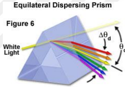
Şekil 4.21: Beyaz ışığın prizmada kırılması ile ayrılan renklerin açılarını gösterir şekil
