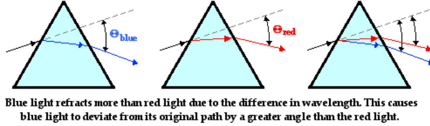
Şekil 4.20: Bir ışığın bir prizmada sapması Mavi ışık, dalga boyundaki farklılık nedeniyle kırmızı ışıktan daha fazla kırılır. Bu, mavi ışığın orijinal yoldan kırmızı ışıktan daha büyük bir açıyla sapmasına neden olur.
