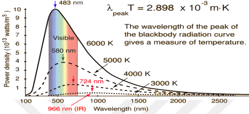
Şekil 3.8: Wien Yasasına uygun siyah cisim radyasyonu grafiği
