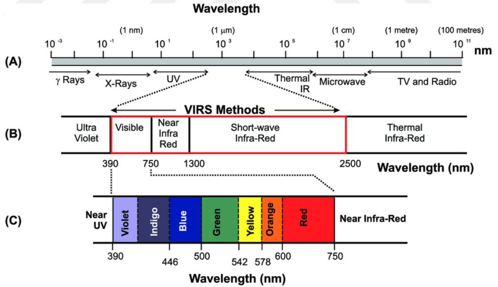
Şekil 5.3: Dalga Boyları ve Renkler
