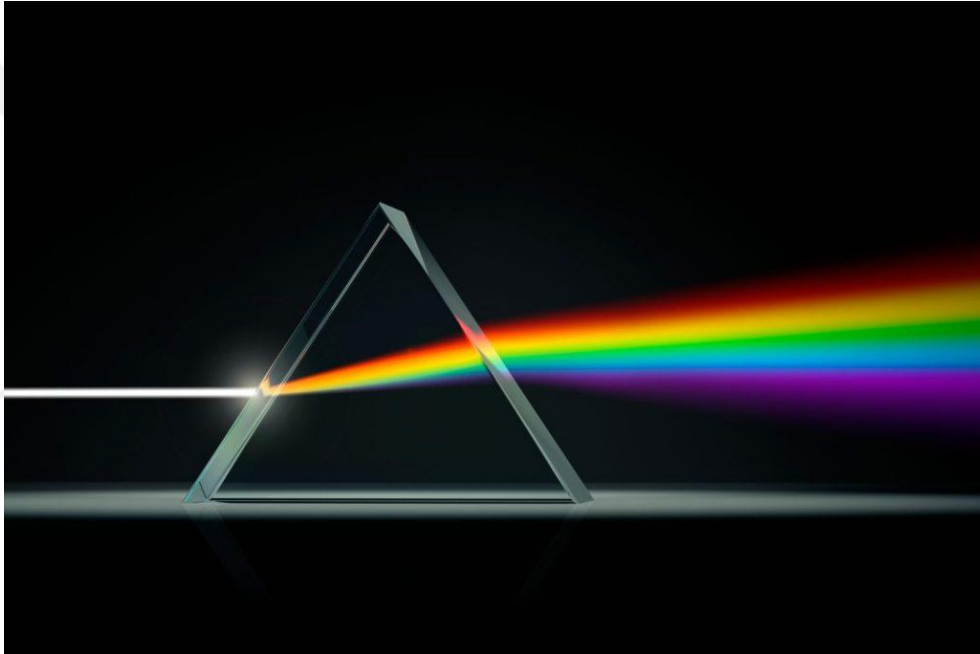
Şekil 2.7: Işık spektrumun Prizmada üretimi. Işık saçan üçgen prizma; farklı ışık dalga boylarını göstermek için gösterilen dalgalar.
