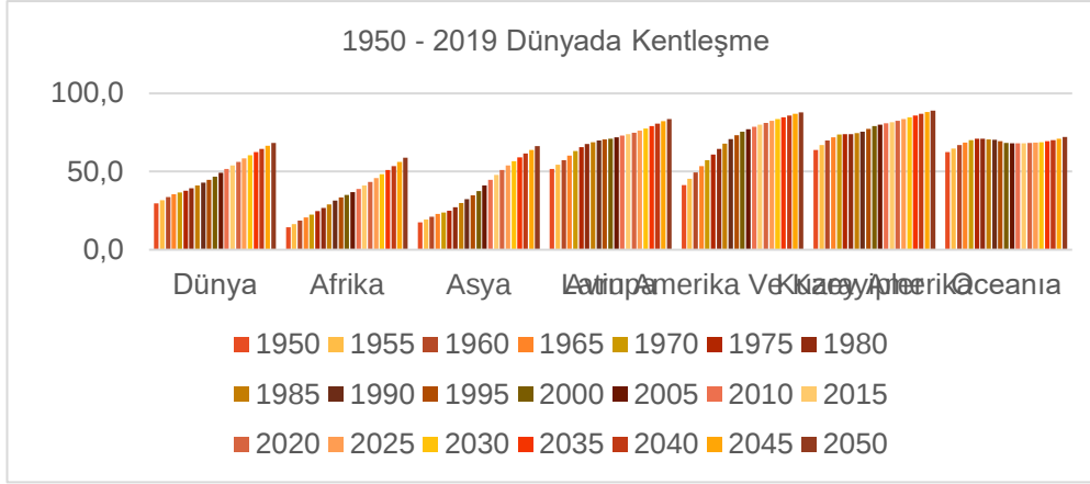
Şekil 2 : 1950 - 2019 Dünyada Kentleşme
