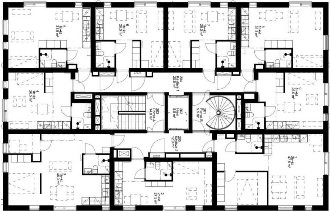
Şekil 4-15: Lighthouse Yapısı Kat Planı (Url-43)
