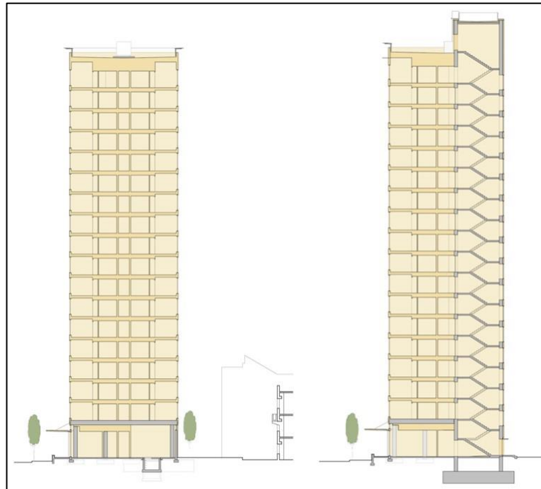
Şekil 4-14: Brock Commons Yapı Kesiti (Url- 50).
