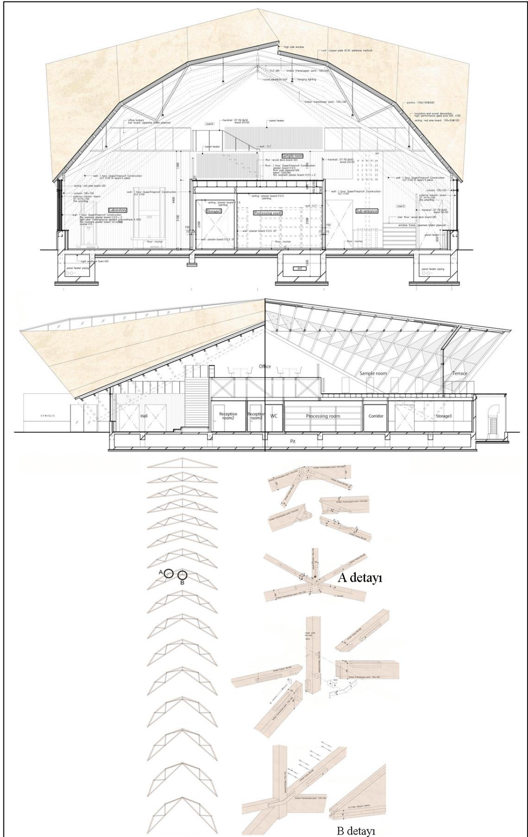
Şekil 3-12: Syneçic Office Kesitler ve Nokta Detayı (Url-16).
