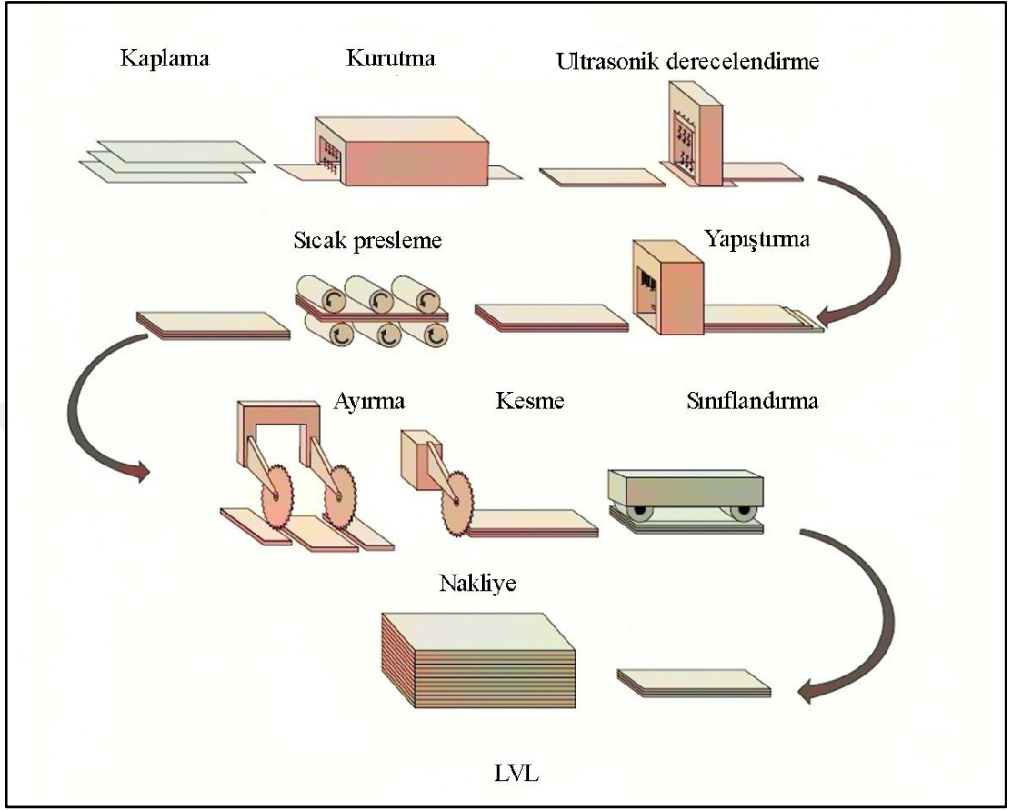
Şekil 3-13: LVL Üretim Aşaması (APA Engineered Wood Handbook, 2001).
