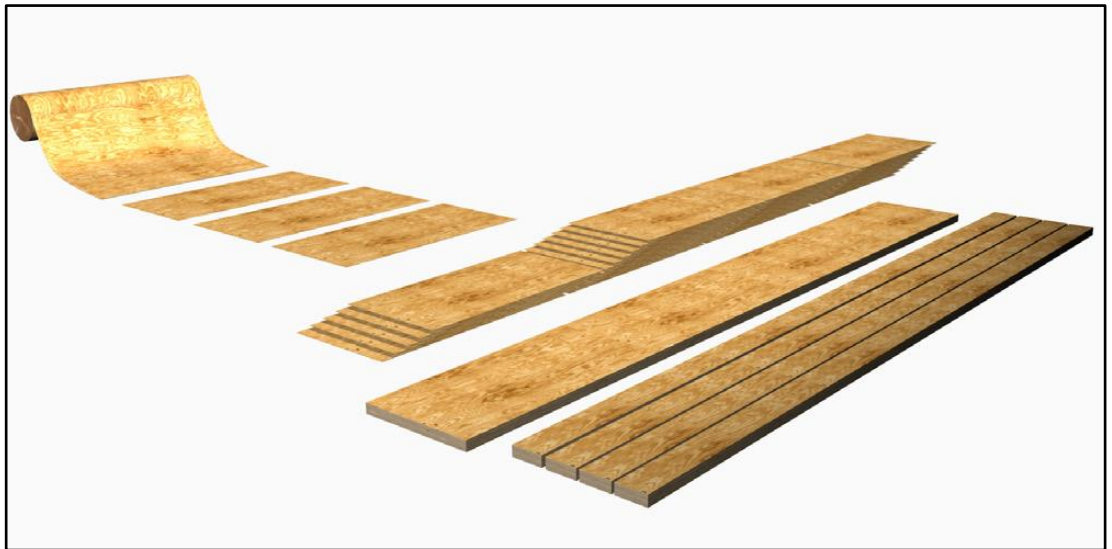
Resim 3-10: LVL Üretim Aşaması (LVL Handbook Europe, 2020).
