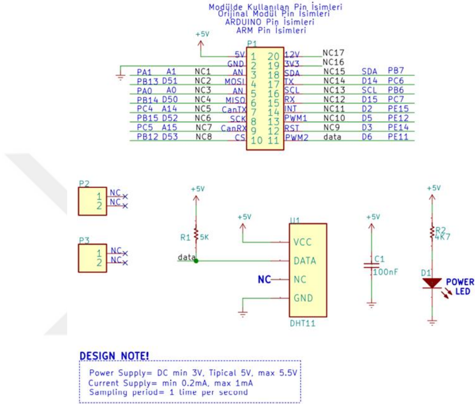
Şekil 7.1: Nem Sensör Modülü şematik çizimi ve pin bağlantıları.
