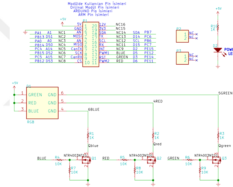
Şekil 7.4: RGB Modül şematik çizimi ve pin bağlantıları.
