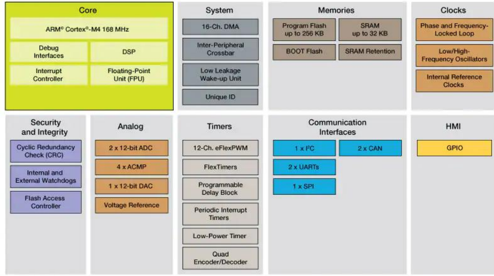
Şekil 4.8: ARM Cortex®-M4 STM32F407VGT6 mikrodnetleyicisi (NXP 2021).
