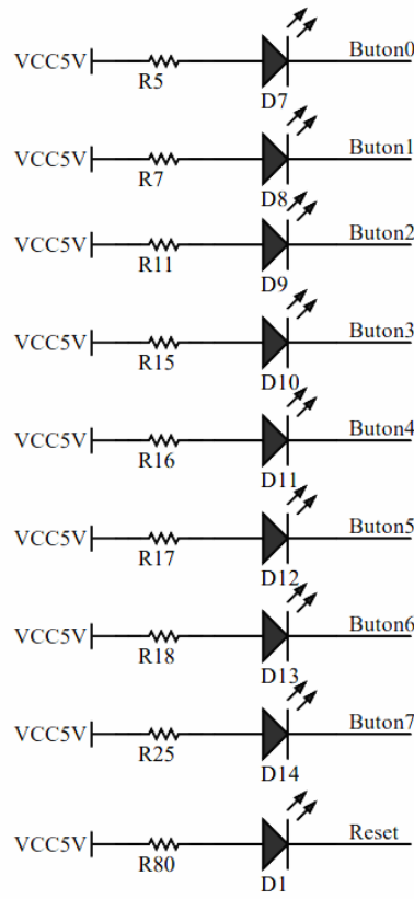
Şekil 5.9: Arduino-Arm Uyumlu Esnek Yapılı Mikrodenetleyici Eğitim Seti buton takımına ait LED şematik çizimleri.
