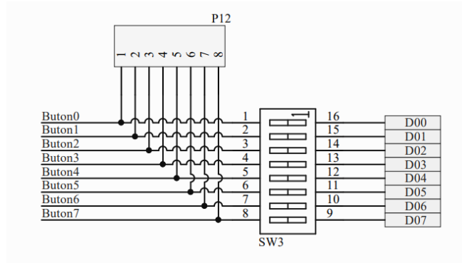
Şekil 5.11: Buton takımına ait 8’li DIP-Switch şematik çizimi.
