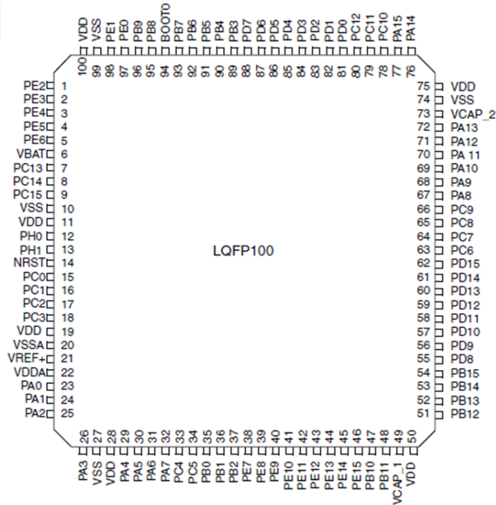
Şekil 4.9: STM32F407VGT6 mikrodnetleyicisi pin konfigürasyonu (Datasheetgo 2021).
