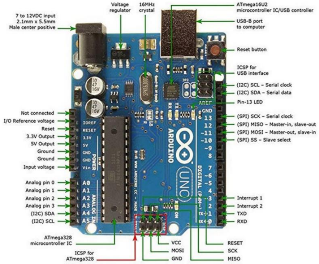
Şekil 4.4: Arduino UNO R3 mikrodnetleyici kartı
