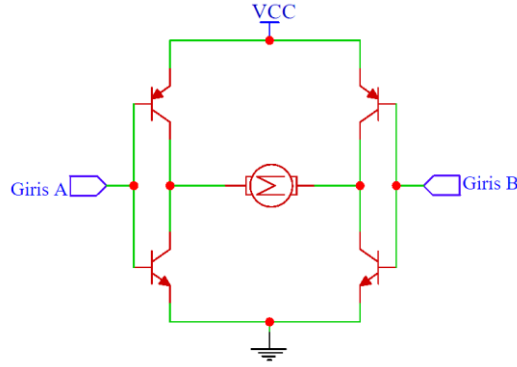
Şekil 7.11: 4 adet transistörden oluşan H-köprüsü devresi.
