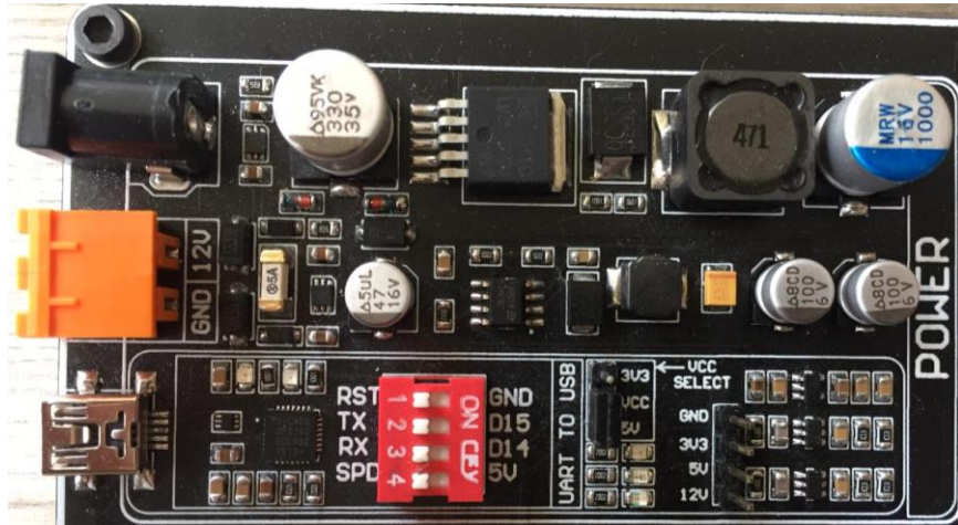
Şekil 5.7: Arduino-Arm Uyumlu Esnek Yapılı Mikrodenetleyici Eğitim Seti besleme katı.
