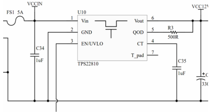
Şekil 5.4: TPS22810 entegresi şematik çizimi.
