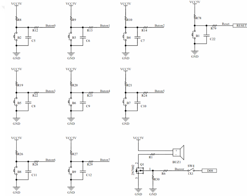
Şekil 5.8: Arduino-Arm Uyumlu Esnek Yapılı Mikrodenetleyici Eğitim Seti üzerindeki butonların şematik çizimi.
