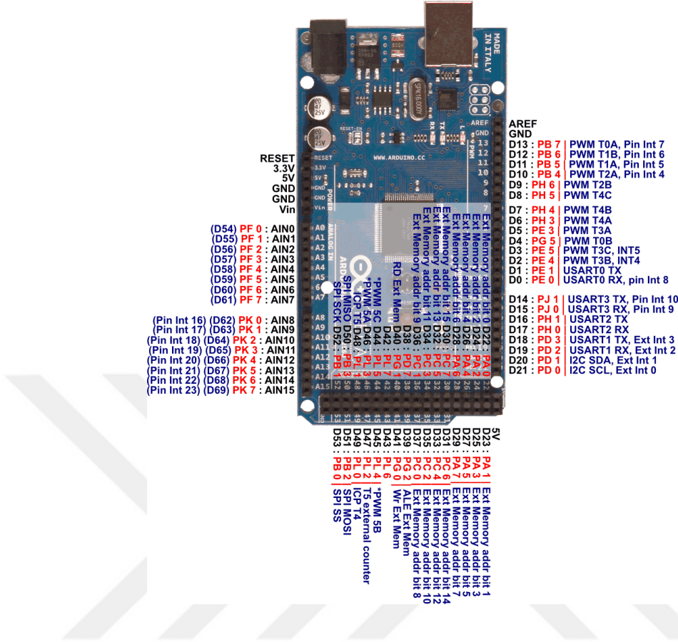
Şekil 4.7: Arduino Mega 2560 R3 mikrodnetleyici kartı (Arduonik 2021).
