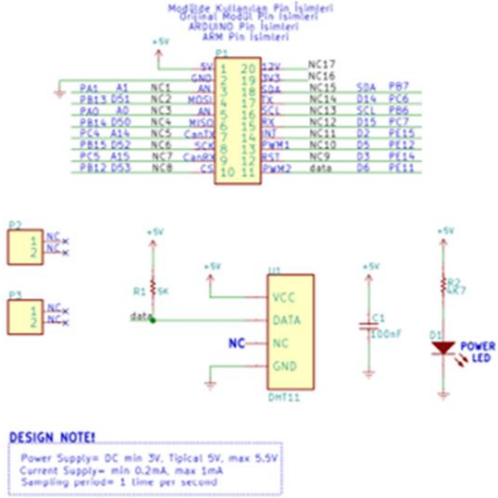
Şekil 2. Humid Module açık devre şeması ve pin bağlantıları
