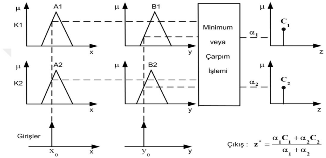
Şekil 14: Sıfırıncı dereceden Sugeno BÇS genel işleyişi (Karasakal 2012).
