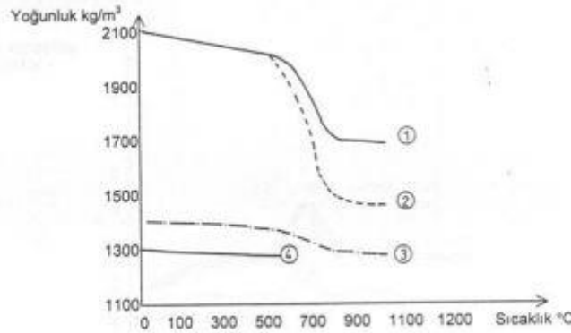
Şekil 4. 17: Betonda yoğunluk ile sıcaklık kapasitesinin değişimi (Aydın, 1998).
