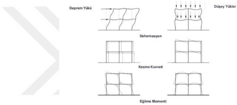
Şekil 4. 22: Deprem yüklerinin yapıya etkisi ve sonucunda yapıda oluşan farklı bozulmalar (URL 48).
