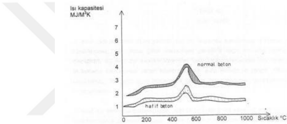
Şekil 4. 18: Farklı betonlarda ısı kapasitesinin değişimi (Aydın, 1998).
