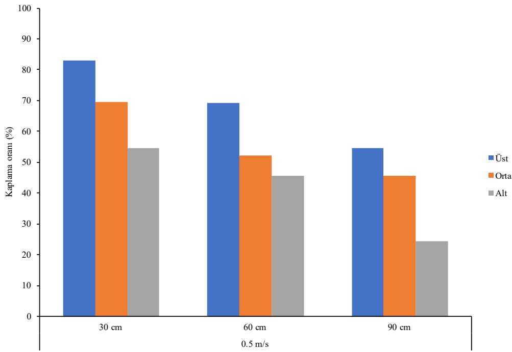
Şekil 4.4. 0.5 m/s hızda ve farklı yüksekliklerde (30 cm, 60 cm, 90 cm) asma bitkisi içindeki üst, orta ve alt bölgelerde ölçülen kaplama oranı değerleri
