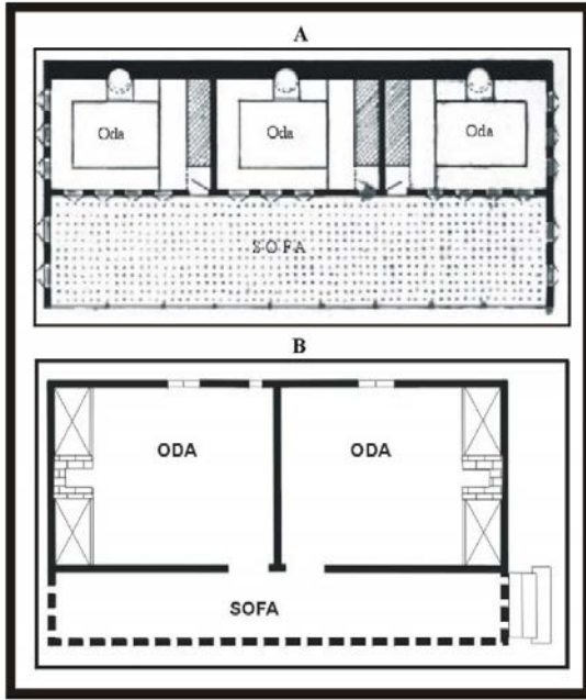
Drawing 4.4: Dış Sofalı plan tipleri/Sedad Hakkı Eldem
