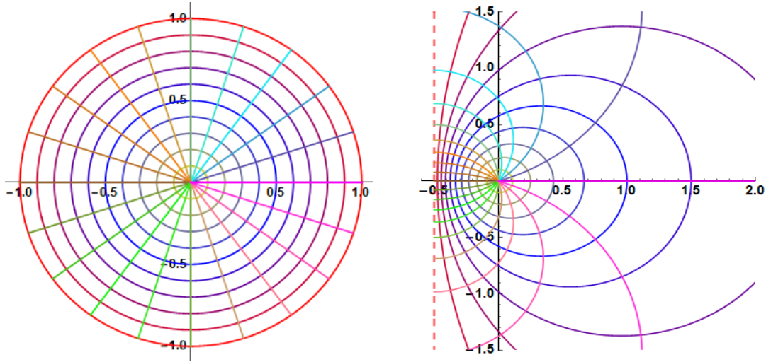
Şekil 3.6. U birim diskinin f(z) = \frac{z}{1-z} fonksiyonu altındaki resmi
