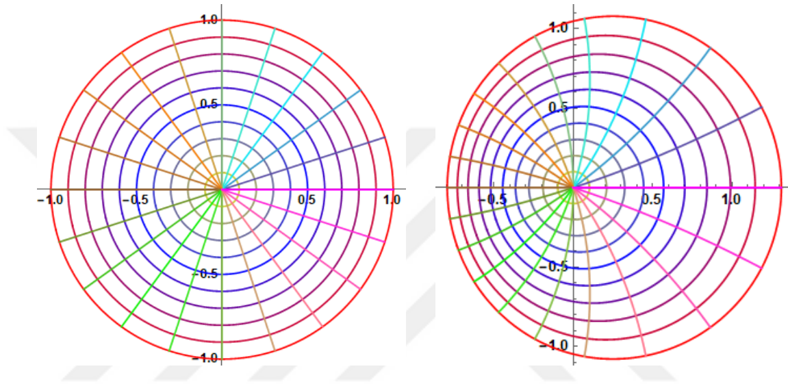
Şekil 4.7. \mathcal{U} diskinin \mathbb{E}_{3,1}(z) = z + \sum_{k=2}^{\infty} \frac{\Gamma(4)}{\Gamma(3+k)} z^k fonksiyonu altındaki resmi
