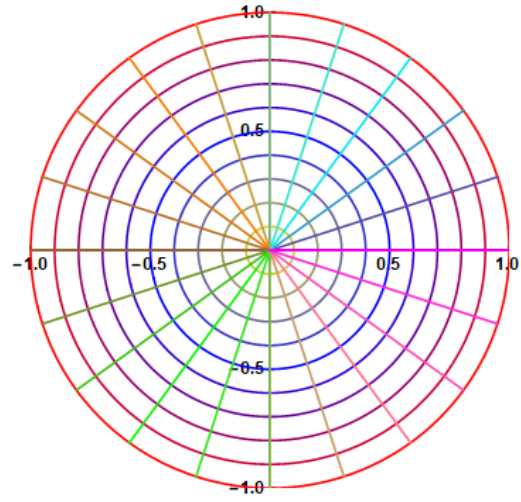
Şekil 3.5. Konveks Küme
