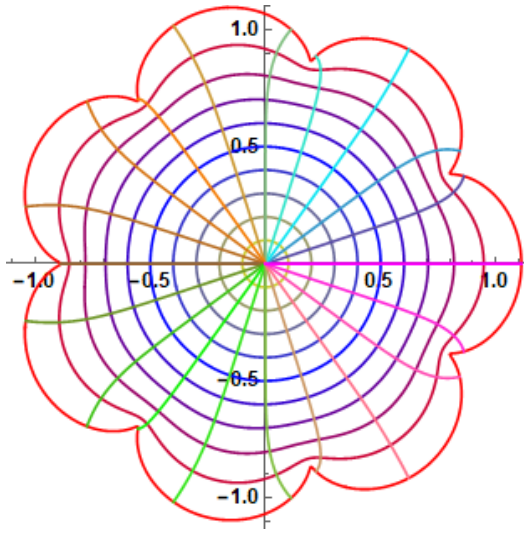
Şekil 3.4. Yıldızlı Küme
