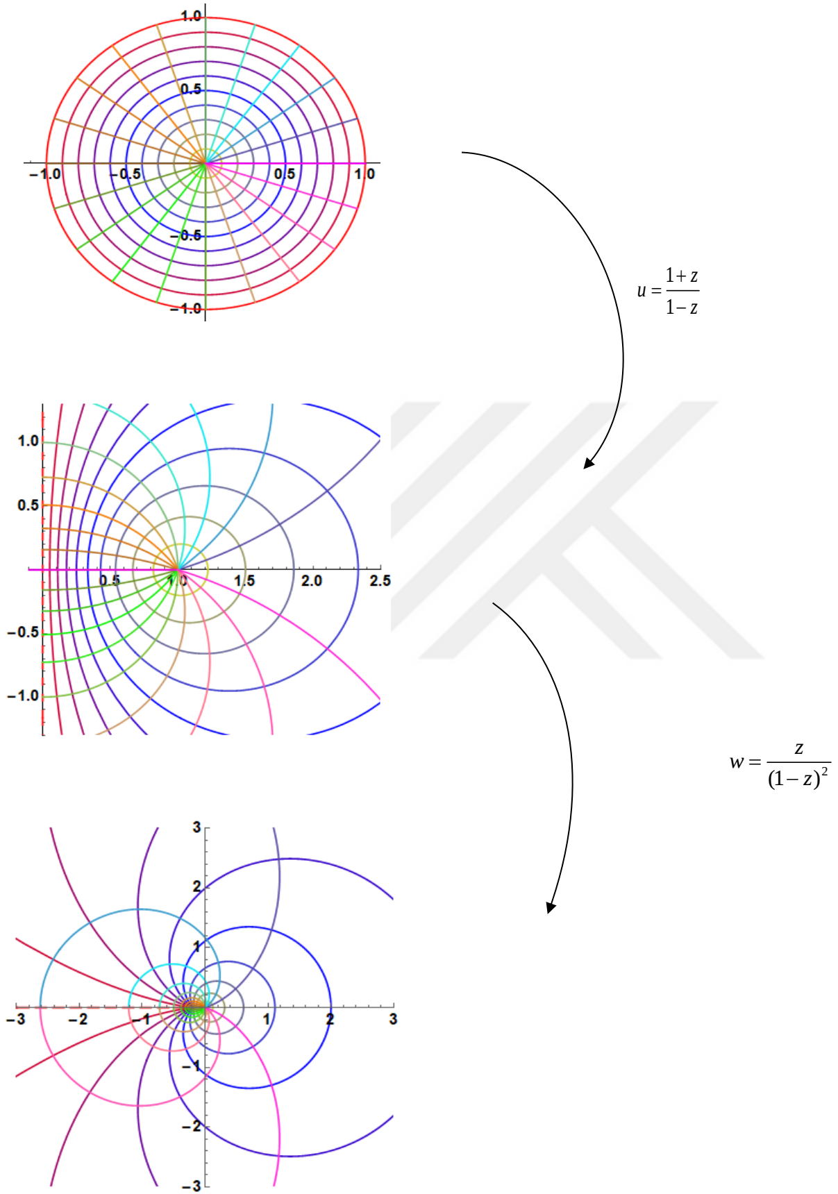
Şekil 3.3. Koebe fonksiyonu
