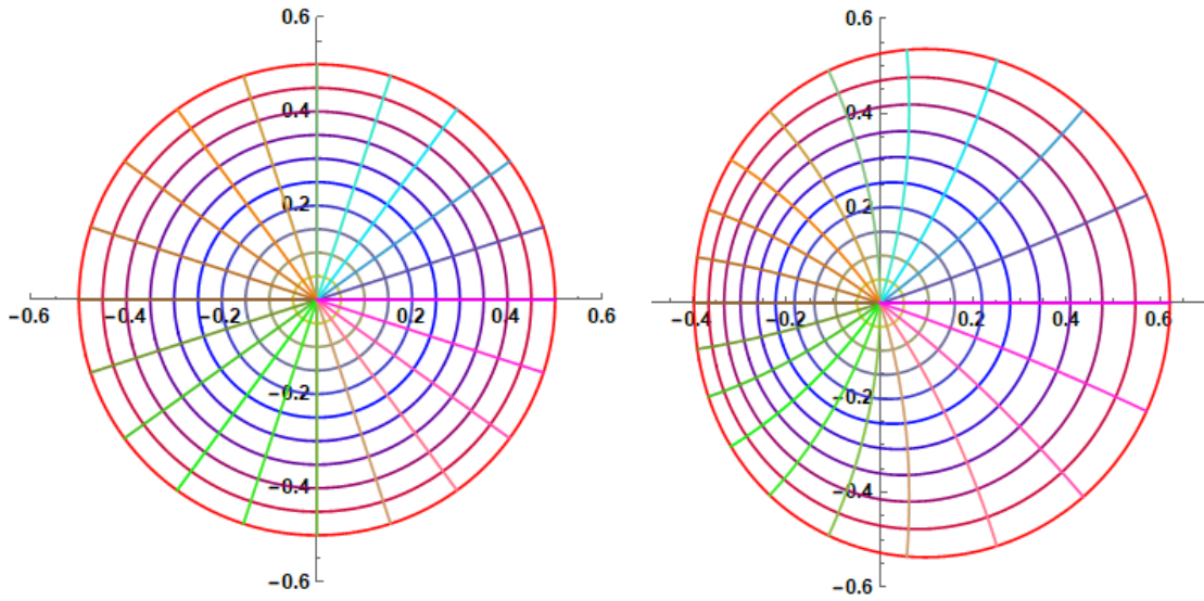
Şekil 4.16. \mathcal{U}_{1/2} diskinin \mathbb{R}_{1/2}(z) = z + \sum_{k=2}^{\infty} \frac{\Gamma(3/2)}{\Gamma(3k/2)} z^k fonksiyonu altındaki resmi
