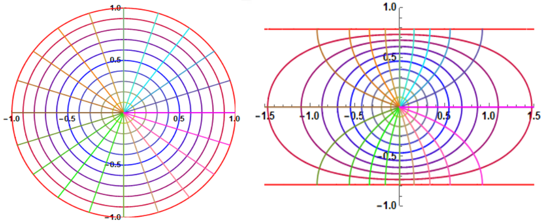
Şekil 3.7. U birim diskinin f(z) = \frac{1}{2} \log\left(\frac{1+z}{1-z}\right) fonksiyonu altındaki resmi
