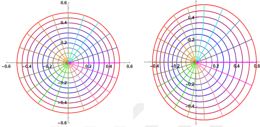
Şekil 4.17. \mathcal{U}_{1/2} diskinin \Re_{0, \frac{1}{3}}(z) = z + \sum_{k=2}^{\infty} \frac{1}{3^{k-1} \Gamma(k)} z^k fonksiyonu altındaki resmi
