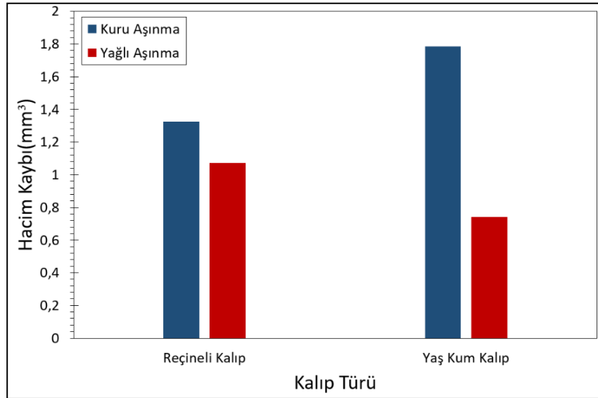
Şekil 4.16 : Hacim kayıpları.
