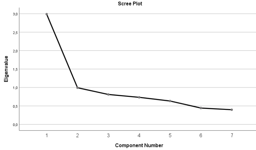
Şekil 3.1: Yamaç-Eğim (Scree Plot) Grafiği
