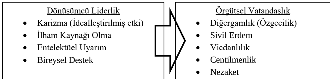
Şekil 1. Araştırma Modeli
