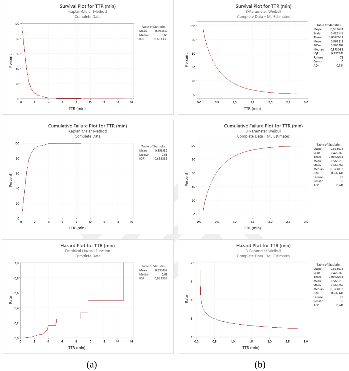
Şekil 4.8. M1 ve M2'nin tamir süreleri için sağ kalım, kümülatif arıza ve arıza oranı grafikleri: a) M1'e ait grafikler, b) M2'ye ait grafikler
