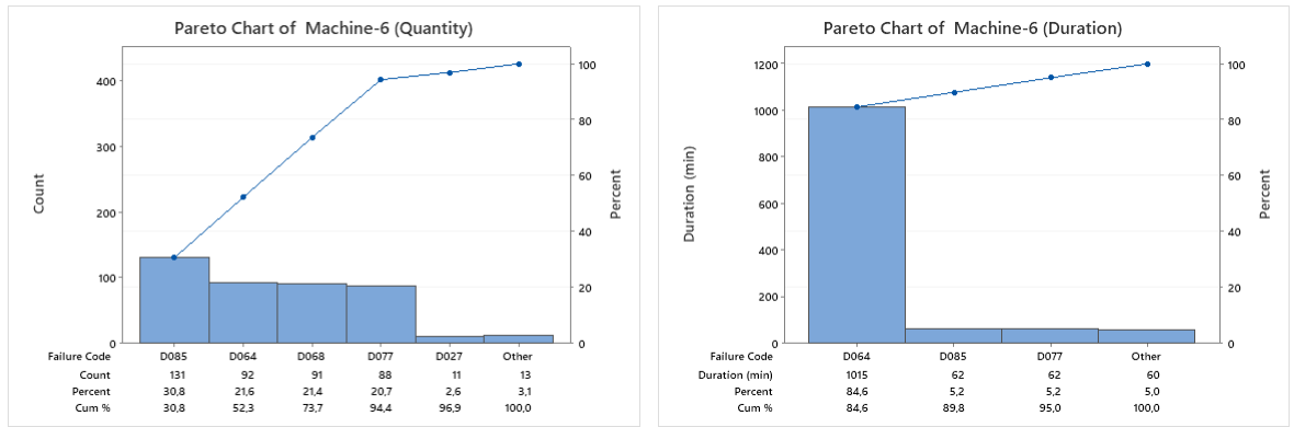
Şekil 4.2. M4, M5 ve M6 pareto grafikleri: a) M4 için duruş sıklığına ve süresine göre pareto grafikleri, b) M5 için duruş sıklığına ve süresine göre pareto grafikleri, c) M6 için duruş sıklığına ve süresine göre pareto grafikleri
