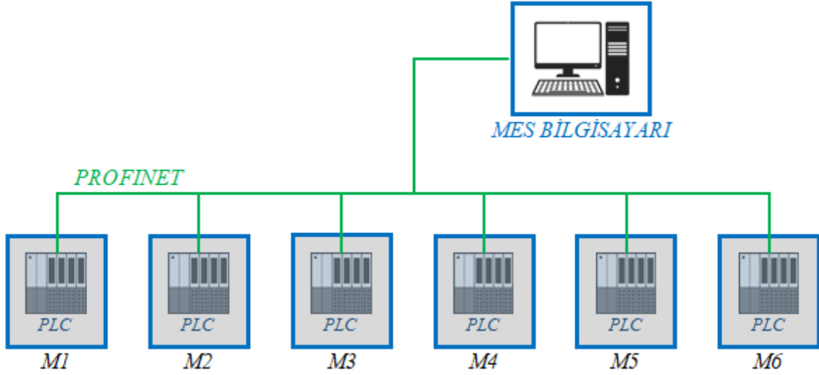
Şekil 3.3. MES haberleşme yapısı
