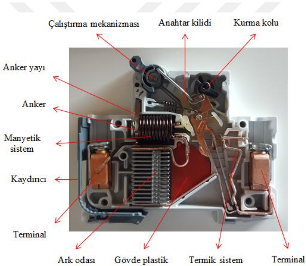
Şekil 3.1. Siemens minyatür devre kesicinin iç yapısı
