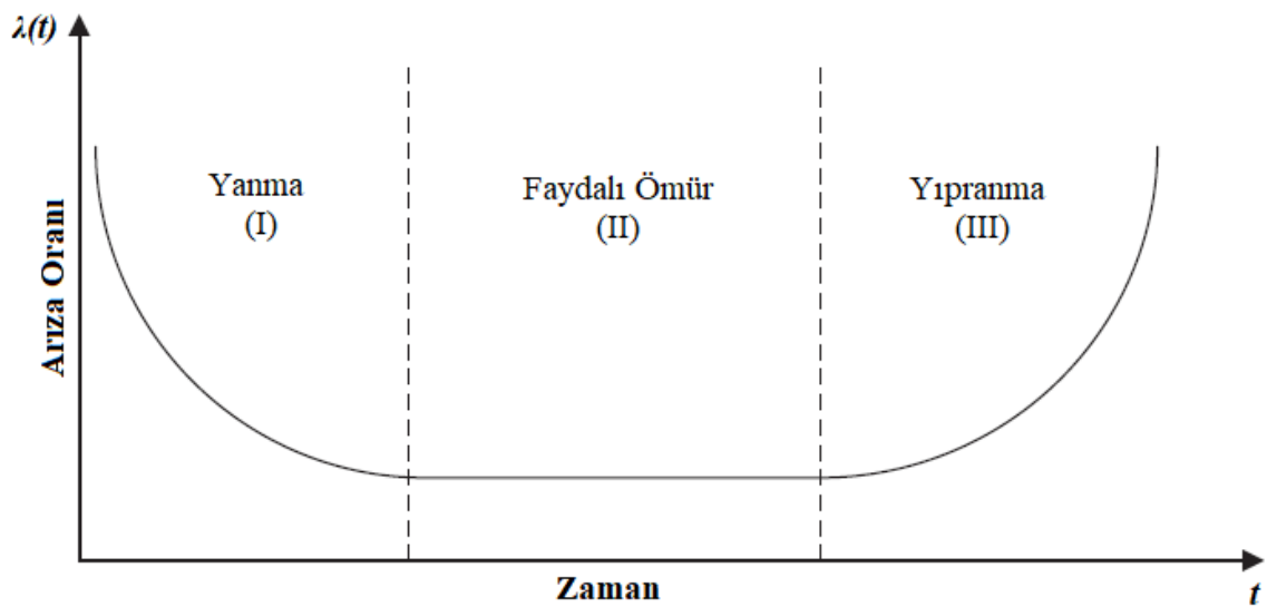
Şekil 2.3. Küvet eğrisi
