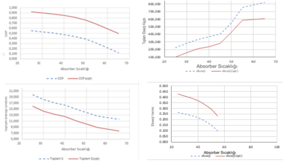
Şekil 4.35 Amonyak-Lityum Nitrat Çifti Absorber Giriş Sıcaklığının Etkisi
