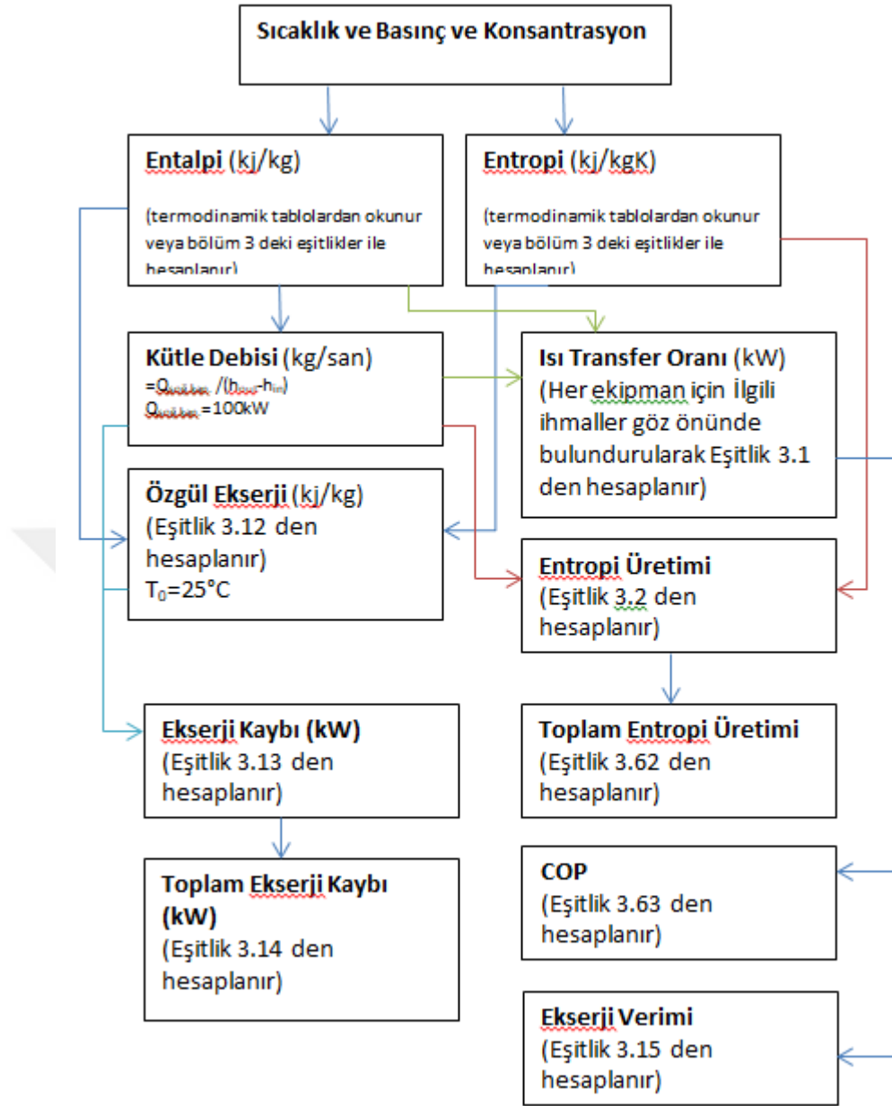
Şekil 4.4 Yapılan Hesaplamalar İçin Akış Diyagramı
