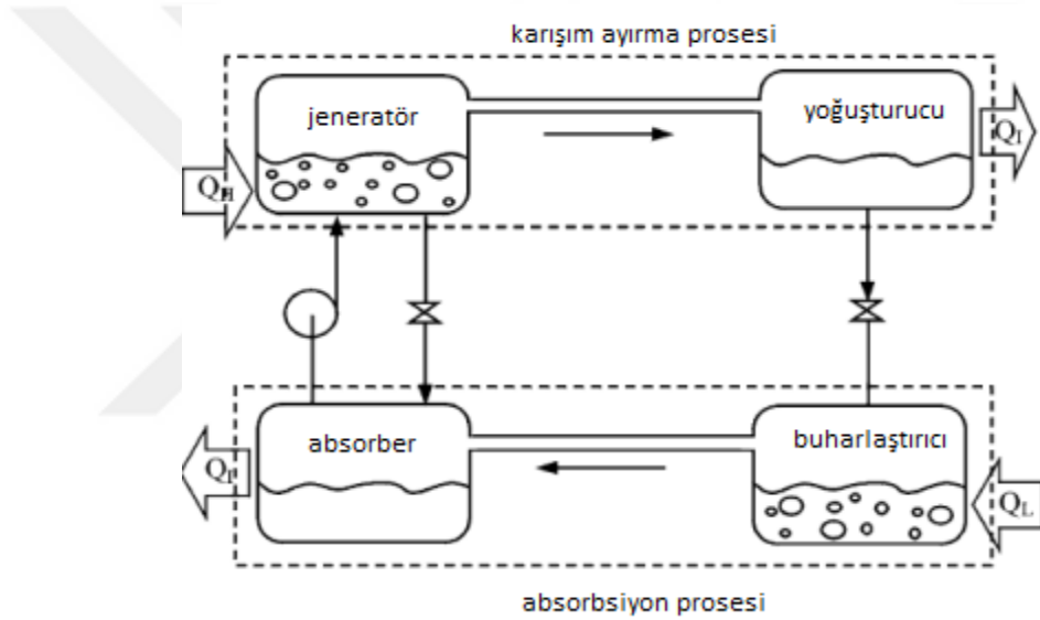
Şekil 2.1 Sürekli soğurmalı bir soğutma çevriminin iki aşaması [3]
