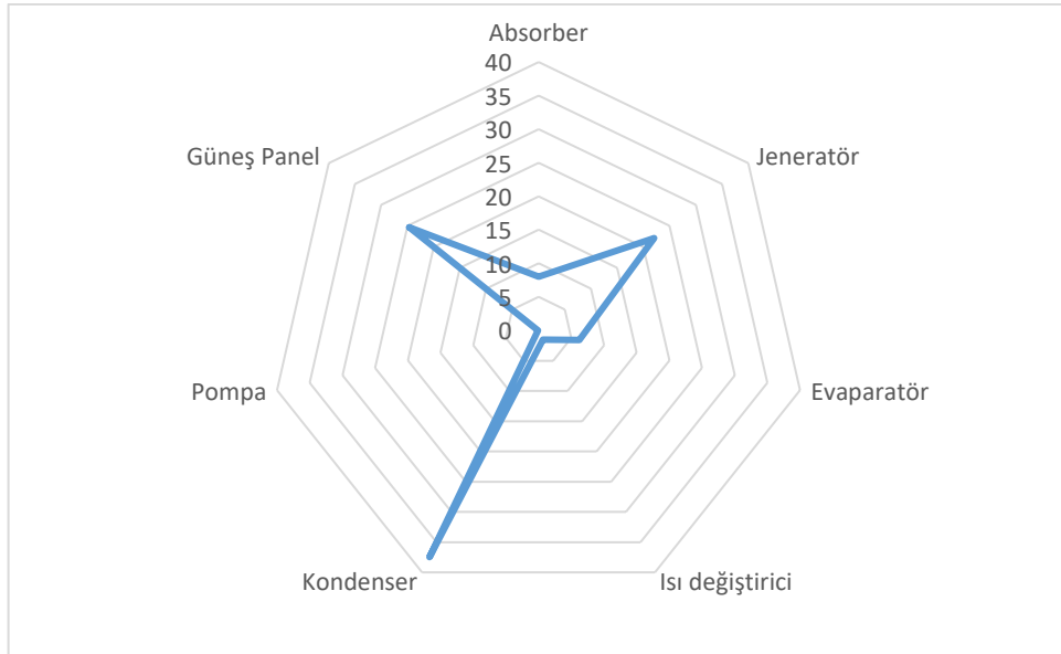
Şekil 4.8 Amonyak-Sodyum Tiyosiyanat çifti yüzde olarak yıkım oranları
