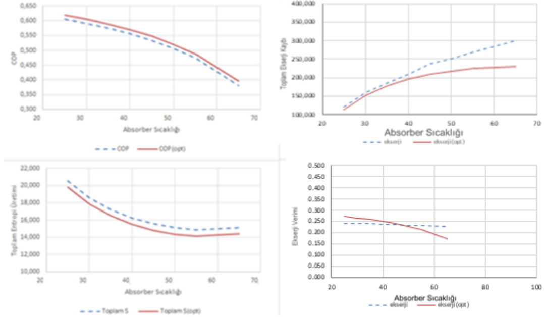
Şekil 4.31 Amonyak-Su Çifti Absorber Giriş Sıcaklığının Etkisi
