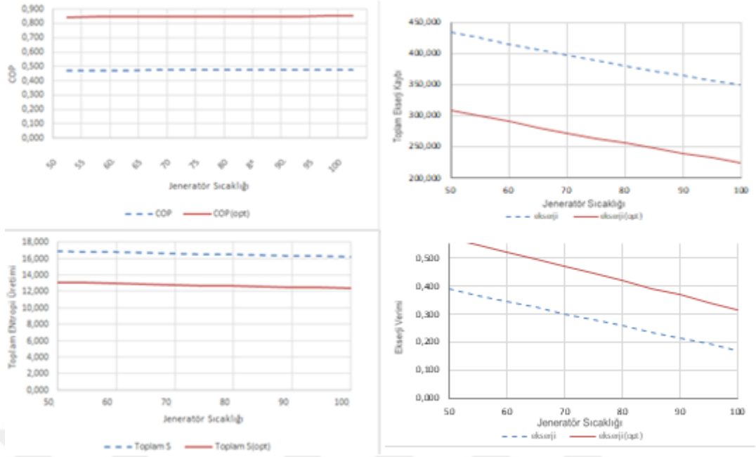
Şekil 4.33 Amonyak-Lityum Nitrat Çifti jeneratör Giriş Sıcaklığının Etkisi
