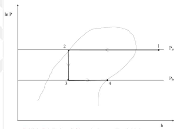
Şekil 2.6 Tek kademeli sistemin \ln P ve h diyagramı [2]
