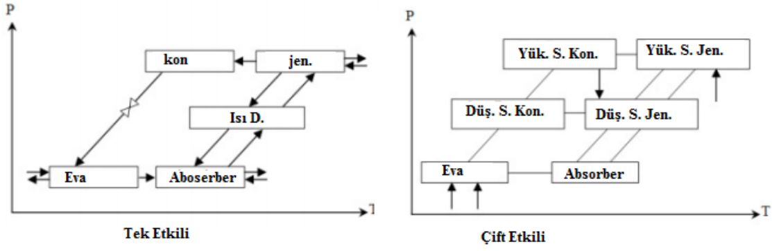
Şekil 2.4. Çift Etkili ve Tek Etkili Absorbsiyon Döngüsü P-T Diyagramalar [1,5]
