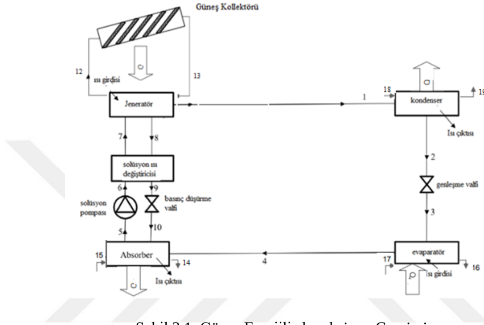
Şekil 3.1. Güneş Enerjili absorpsiyon Çevrimi
