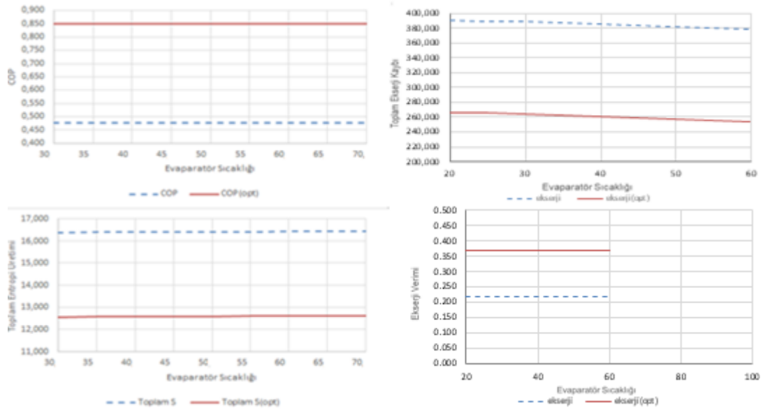
Şekil 4.34 Amonyak-Lityum Nitrat Çifti Evaporatör Giriş Sıcaklığının Etkisi
