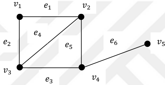
Şekil 2.2. Beş köşeli çizge.
