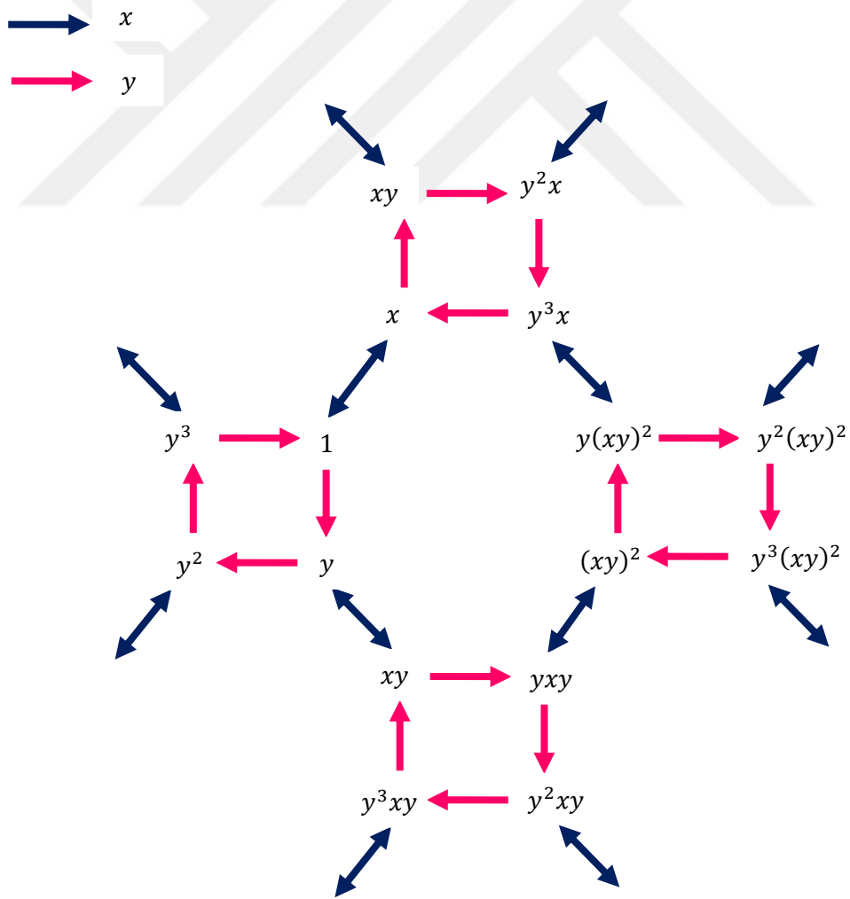
Şekil 3.14. p_4 grubunun Cayley çizgesi.
