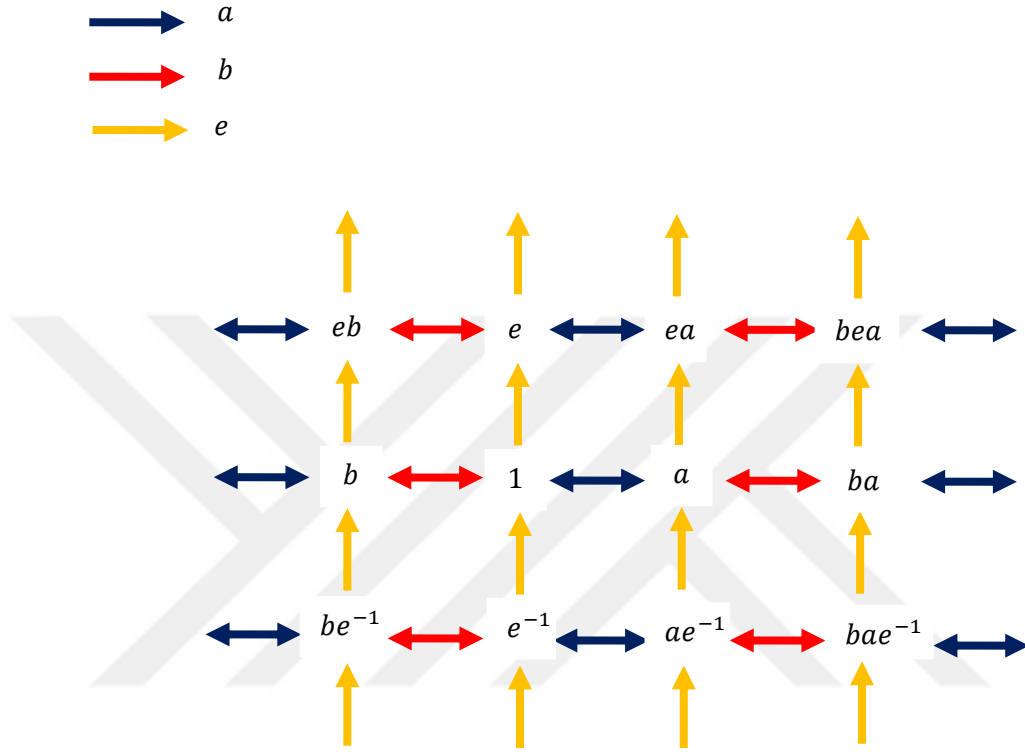
Şekil 3.24. pm grubunun Cayley çizgesi
