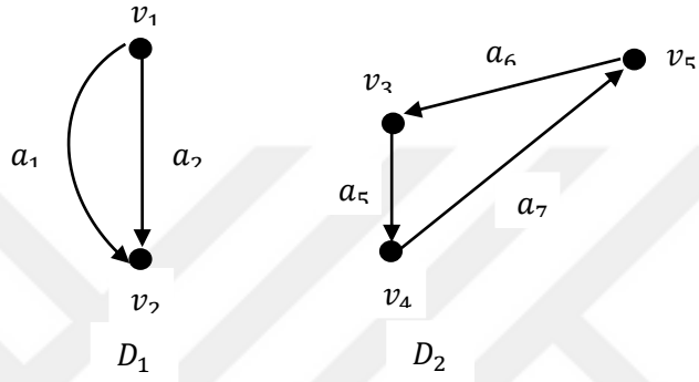
Şekil 2.11. Bir yönlü çizge ve alt çizgeleri.
