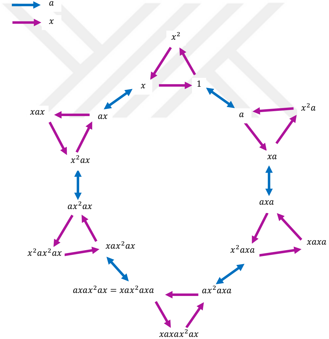
Şekil 3.21. p3m1 grubunun Cayley çizgesi.
