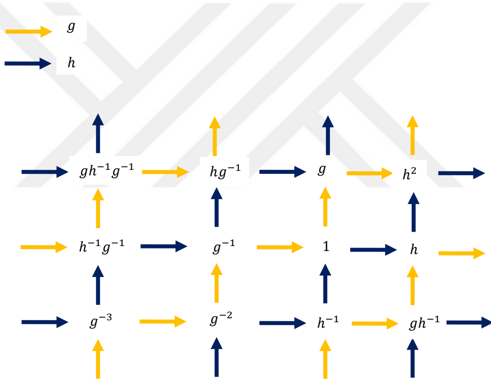
Şekil 3.22. pg grubunun Cayley çizgesi
