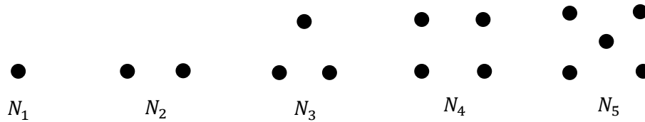
Şekil 2.5. Boş çizgeler.
