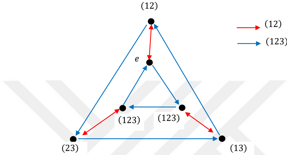
Şekil 3.5. S_3 grubunun Cayley çizgesi.
