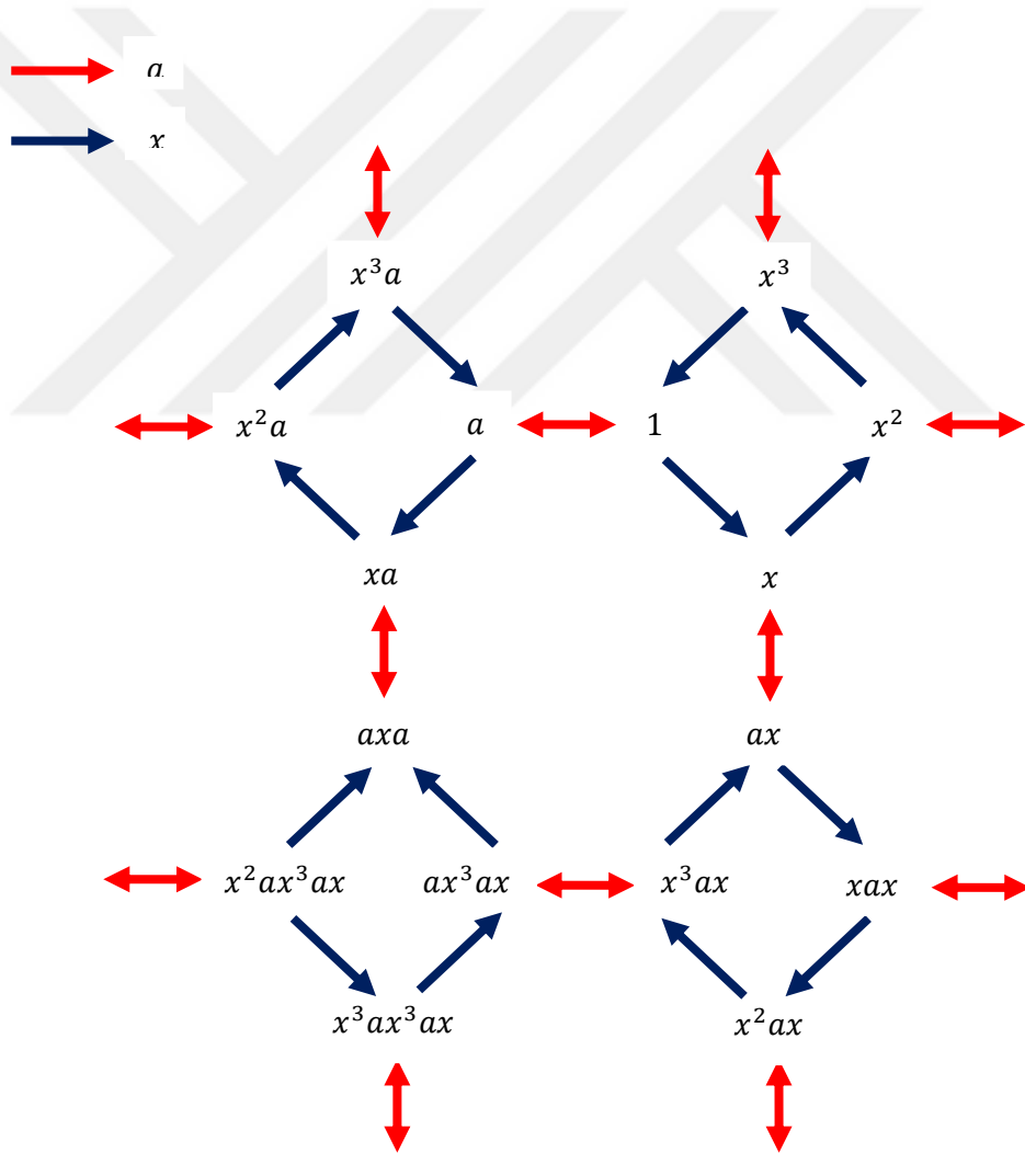
Şekil 3.20. p4g grubunun Cayley çizgesi.
