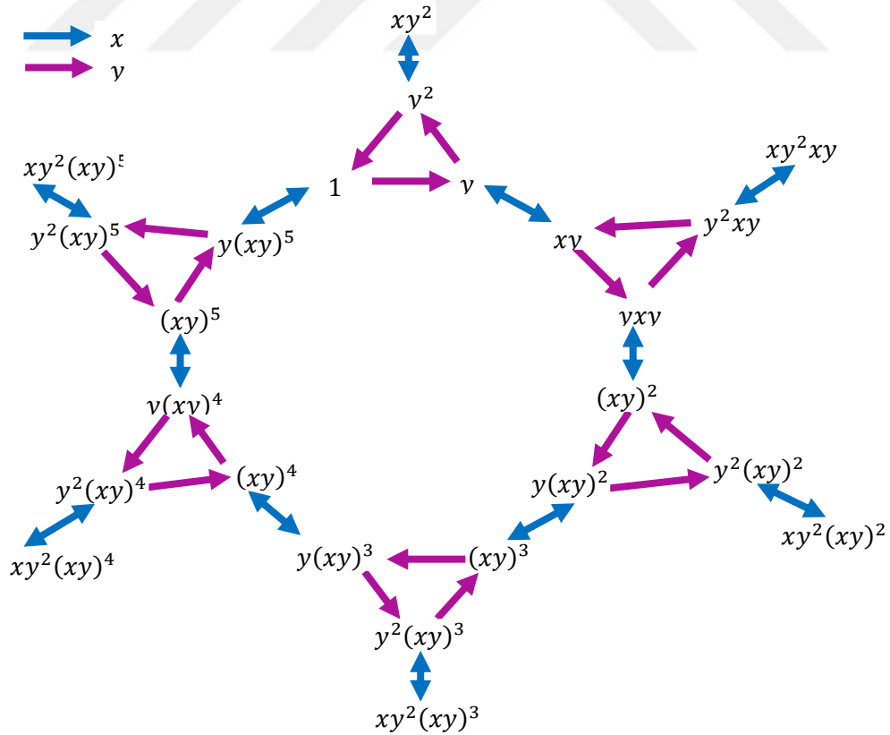
Şekil 3.15. p_6 grubunun Cayley çizgesi.
