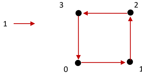
Şekil 3.2. \mathbb{Z}_4 grubunun Cayley çizgesi.
