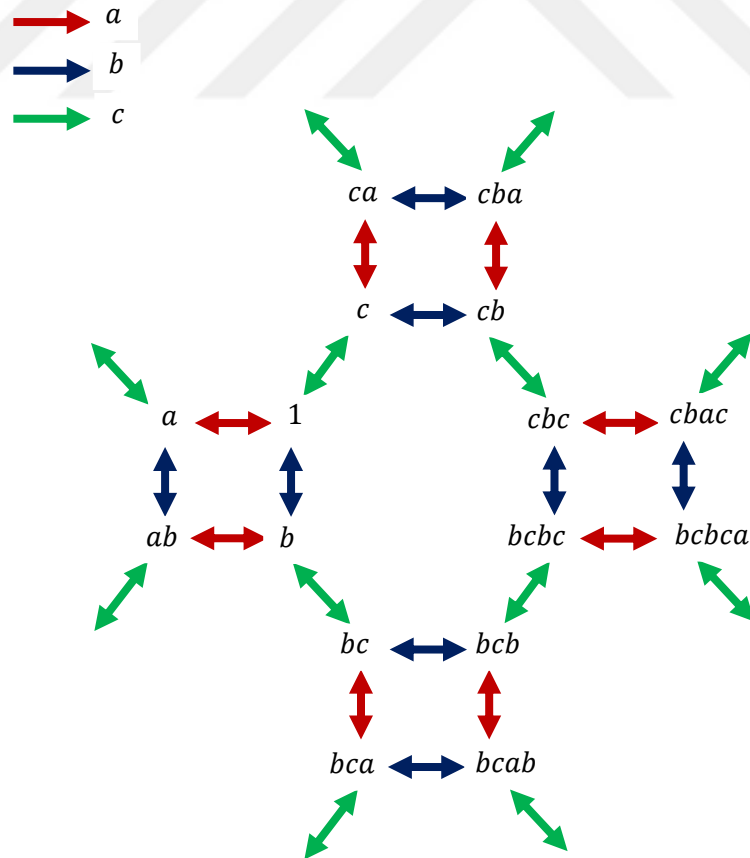
Şekil 3.17. p4m grubunun Cayley çizgesi.
