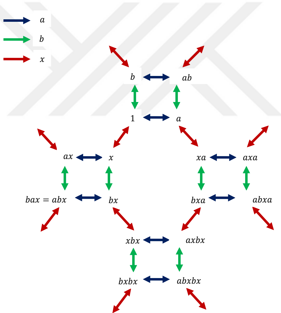
Şekil 3.19. cmm grubunun Cayley çizgesi.
