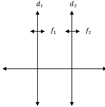
Şekil 1.1. Paralel iki doğru üzerindeki yansımaların bileşkesi.
