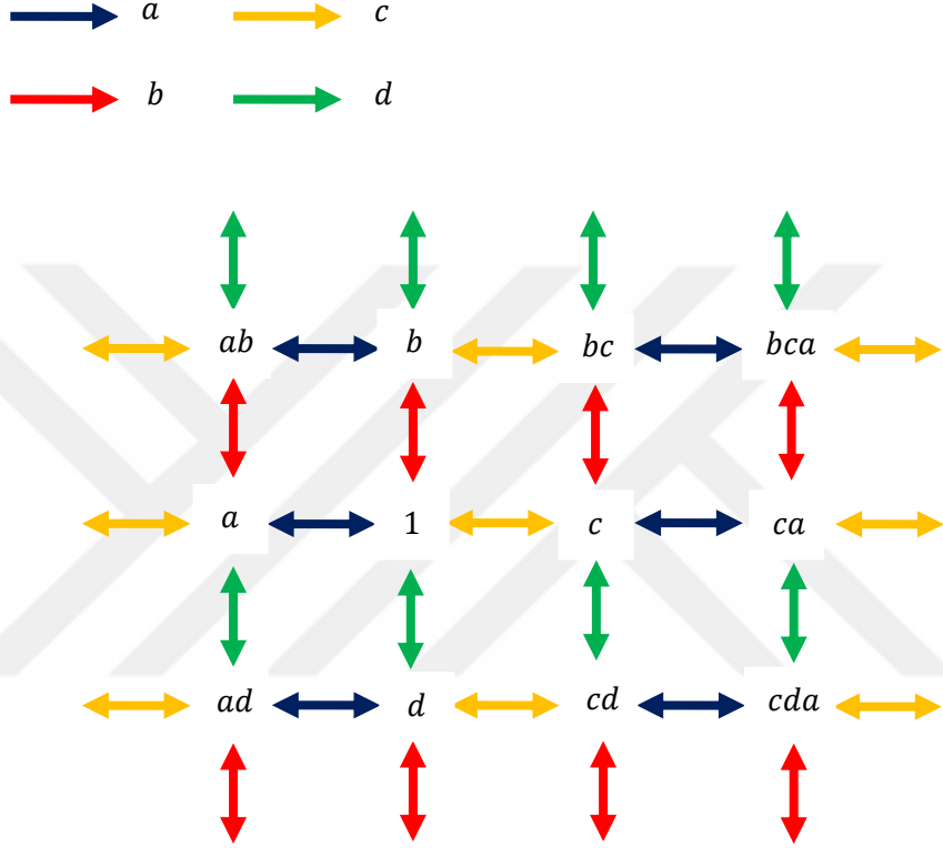
Şekil 3.12. pmm grubunun Cayley çizgesi.
