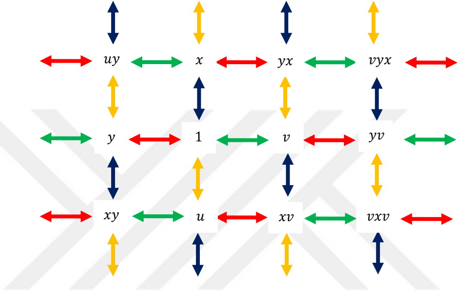
Şekil 3.11. p_2 grubunun Cayley çizgesi.
