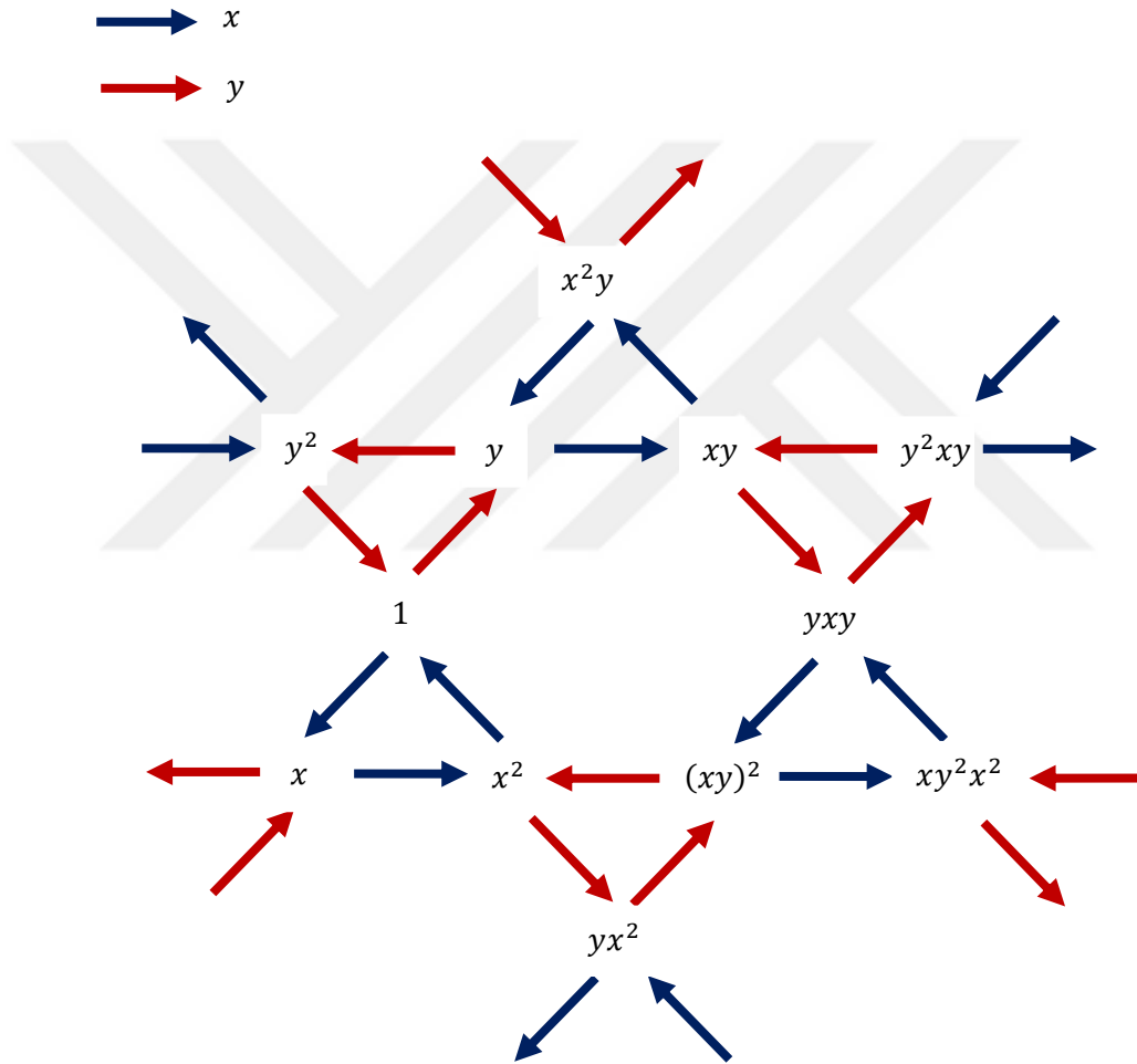
Şekil 3.13. p3 grubunun Cayley çizgesi.
