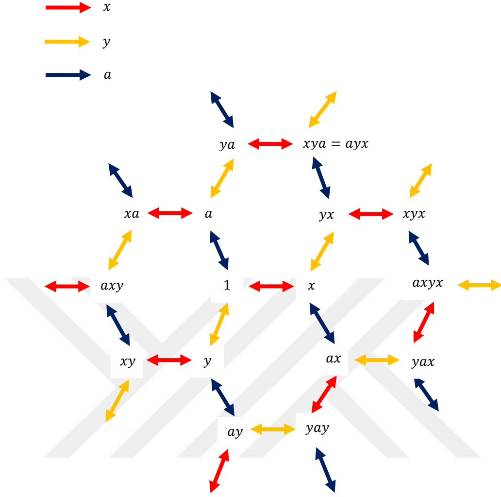
Şekil 3.26. pmg grubunun Cayley çizgesi
