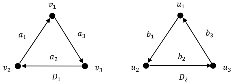
Şekil 2.12. D_1 ve D_2 çizgeleri.
