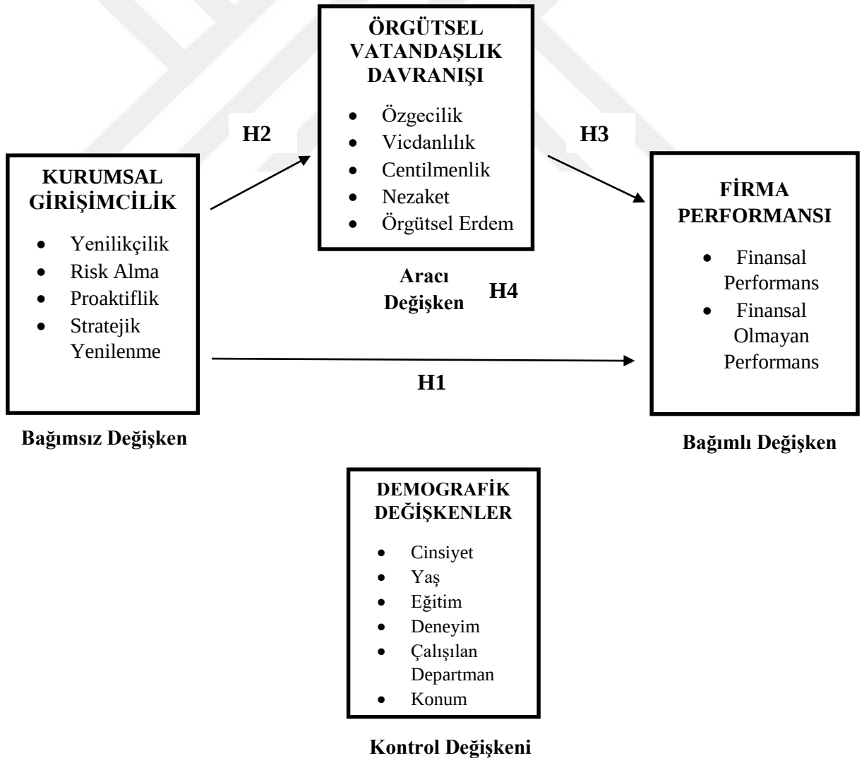
Şekil 6. Araştırma modeli
