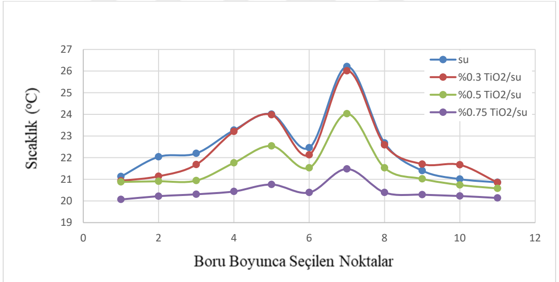
Şekil 4.28. 150°C de motoryağı ve 20°C de saf su, %0.3, %0.5 ve %0.75 oranlarında TiO 2 /su nanoakışkanlarının sıcaklık değişimi
