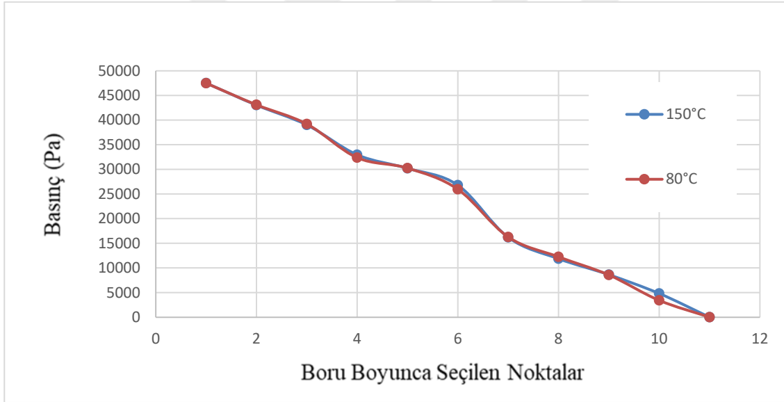
Şekil 4.16. 150° - 80°C de motoryağı ve 20°C de %0.75 TiO 2 /su nanoakışkanı için basınç değişimi
