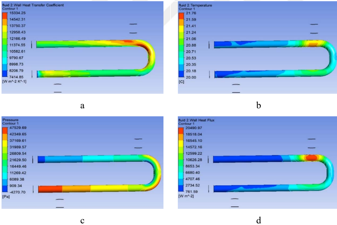
Şekil 4.24. 150°C de motoryağı ve 20°C de %0.75 \text{TiO}_2/\text{su} nanoakışkanı için değişimler (a- ısı transfer katsayısı değişimi, b- sıcaklık değişimi, c- basınç değişimi, d- ısı akısı değişimi)
