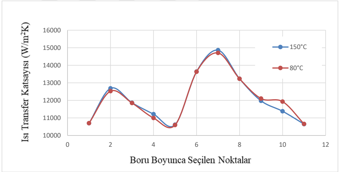
Şekil 4.10. 150° - 80°C de motoryağı ve 20°C de %0.75 TiO 2 /su nanoakışkanı için ısı transfer katsayısı değişimi
