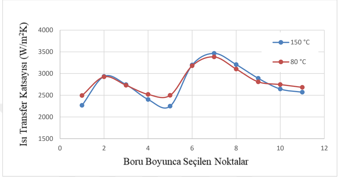
Şekil 4.2. 150°C - 80°C de motoryağı ve 20°C de saf su için ısı transfer katsayısı değişimi
