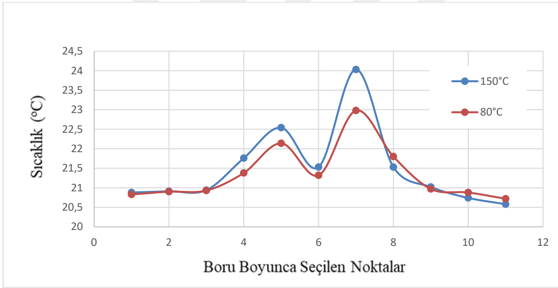
Şekil 4.12. 150° - 80°C de motoryağı ve 20°C de %0.5 TiO 2 /su nanoakışkanı için sıcaklık değişimi
