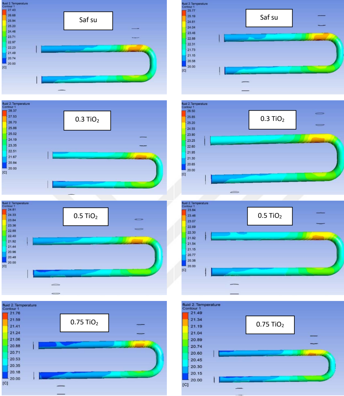
Şekil 4.35. 20°C de yukarıdan aşağıya sırasıyla saf su, %0.3, %0.5, %0.75 oranlarında \text{TiO}_2 /su nanoakışkanları için sıcaklık değişimleri (Sıcak akışkan olarak sol sütunda 150°C de motoryağı, sağ sütunda 80°C de motoryağı kullanılmıştır.)
