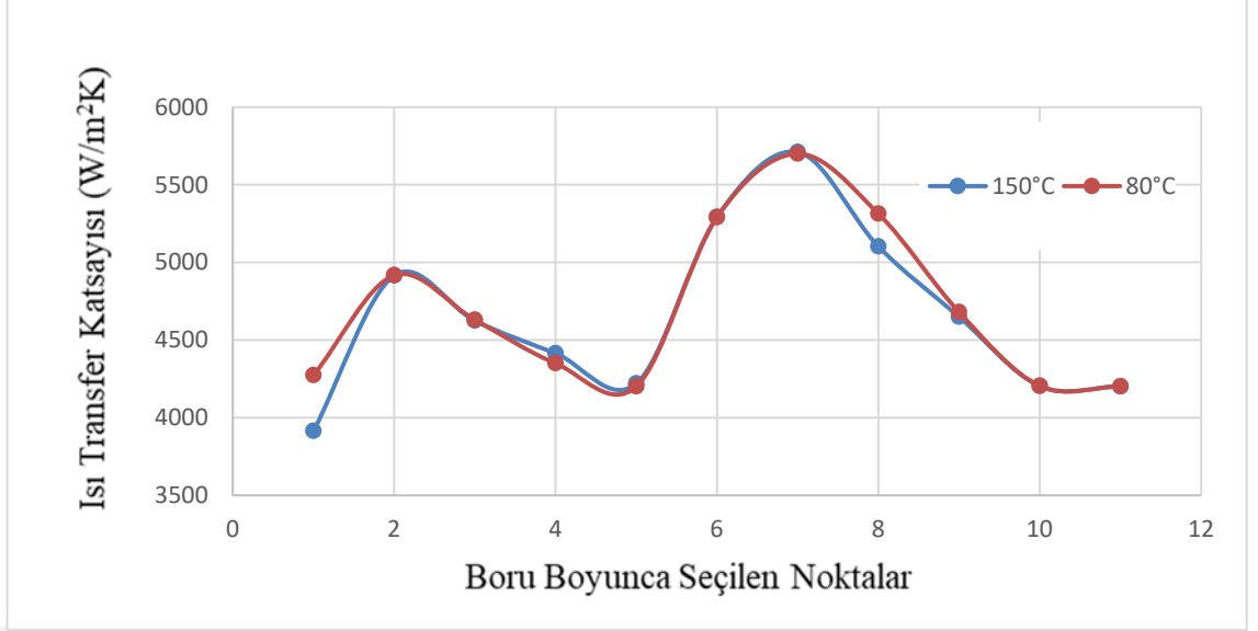
Şekil 4.9. 150° - 80°C de motoryağı ve 20°C de %0.5 TiO 2 /su nanoakışkanı için ısı transfer katsayısı değişimi
