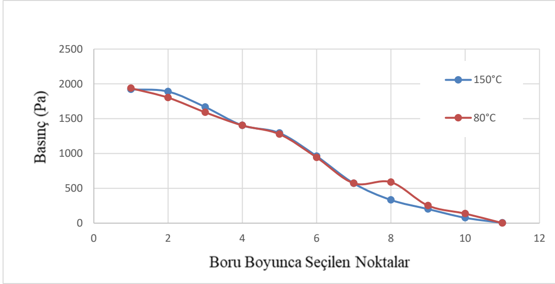
Şekil 4.15. 150° - 80°C de motoryağı ve 20°C de %0.5 TiO 2 /su nanoakışkanı için basınç değişimi
