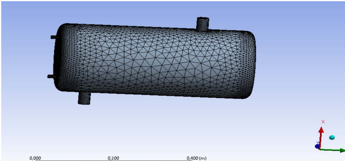
Şekil 3.4. Gövde boru tipi eşanjörün ağ yapısı
