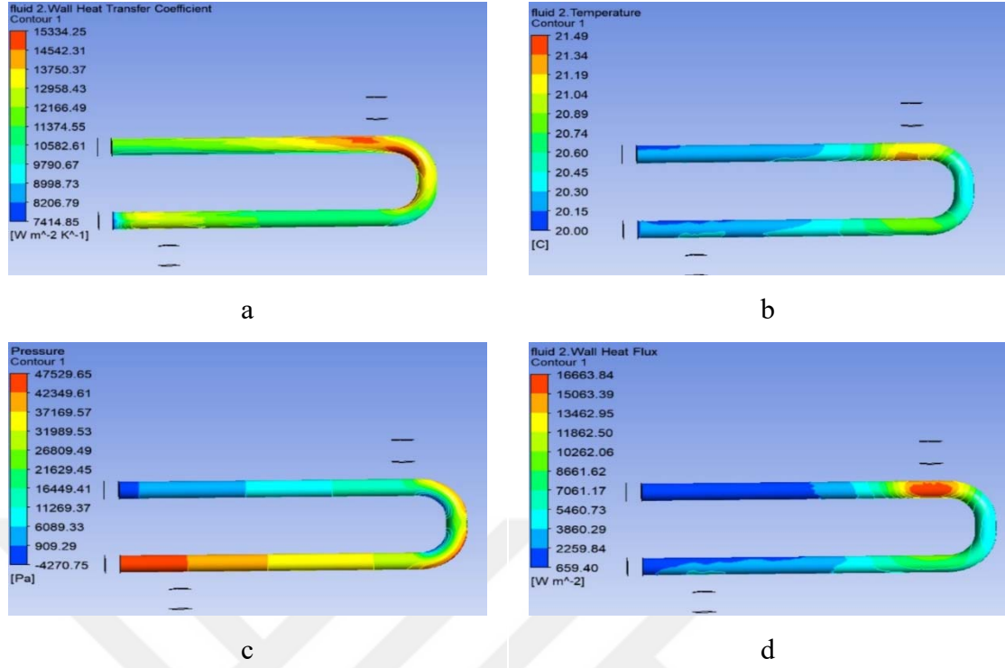
Şekil 4.25. 80°C de motoryağı ve 20°C de %0.75 TiO 2 /su nanoakışkanı için değişimler (a- ısı transfer katsayısı değişimi, b- sıcaklık değişimi, c- basınç değişimi, d- ısı akısı değişimi)
