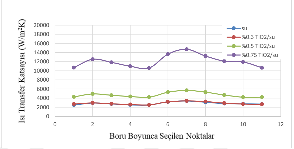
Şekil 4.27. 80°C de motoryağı ve 20°C de saf su, %0.3, %0.5 ve %0.75 oranlarında TiO 2 /su nanoakışkanlarının ısı transfer katsayısı değişimi
