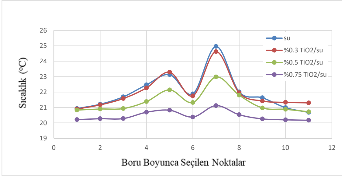
Şekil 4.29. 80°C de motoryağı ve 20°C de saf su, %0.3, %0.5 ve %0.75 oranlarında TiO 2 /su nanoakışkanlarının sıcaklık değişimi
