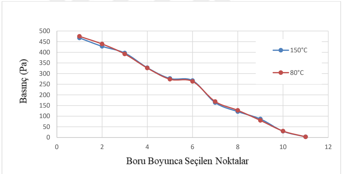
Şekil 4.14. 150° - 80°C de motoryağı ve 20°C de %0.3 TiO 2 /su nanoakışkanı için basınç değişimi
