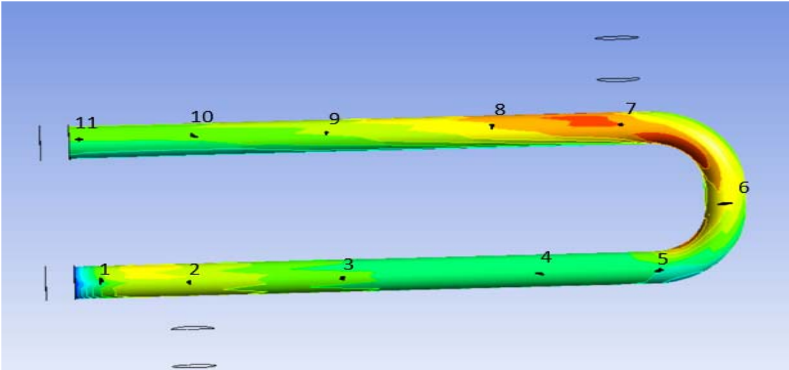
Şekil 4.1. Eşanjör borusu üzerinde seçilen noktaların konumu
