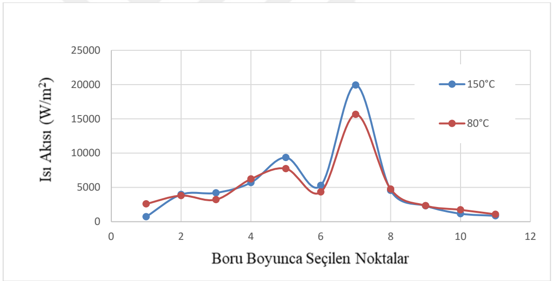
Şekil 4.18. 150° - 80°C de motoryağı ve 20°C de %0.5 TiO 2 /su nanoakışkanı için ısı akısı değişimi
