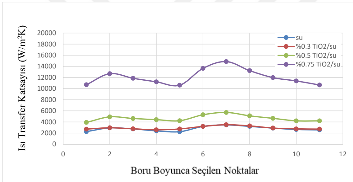
Şekil 4.26. 150°C de motoryağı ve 20°C de saf su, %0.3, %0.5 ve %0.75 oranlarında \text{TiO}_2 /su nanoakışkanlarının ısı transfer katsayısı değişimi
