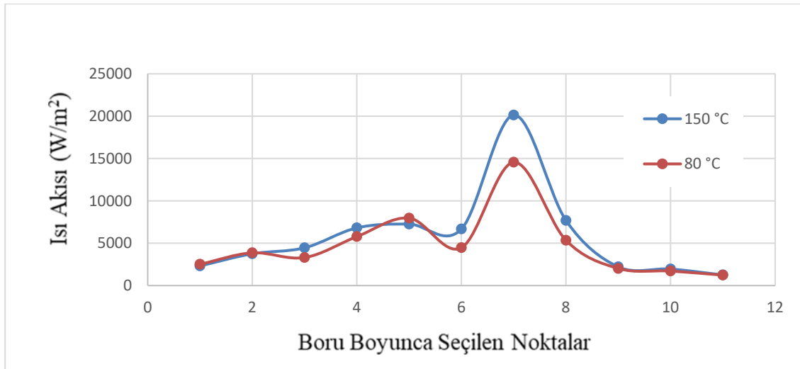
Şekil 4.5. 150°C - 80°C de motoryağı ve 20°C de saf su için ısı akısı değişimi
