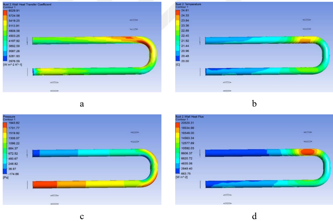
Şekil 4.22. 150°C de motoryağı ve 20°C de %0.5 TiO 2 /su nanoakışkanı için değişimler (a- ısı transfer katsayısı değişimi, b- sıcaklık değişimi, c- basınç değişimi, d- ısı akısı değişimi)
