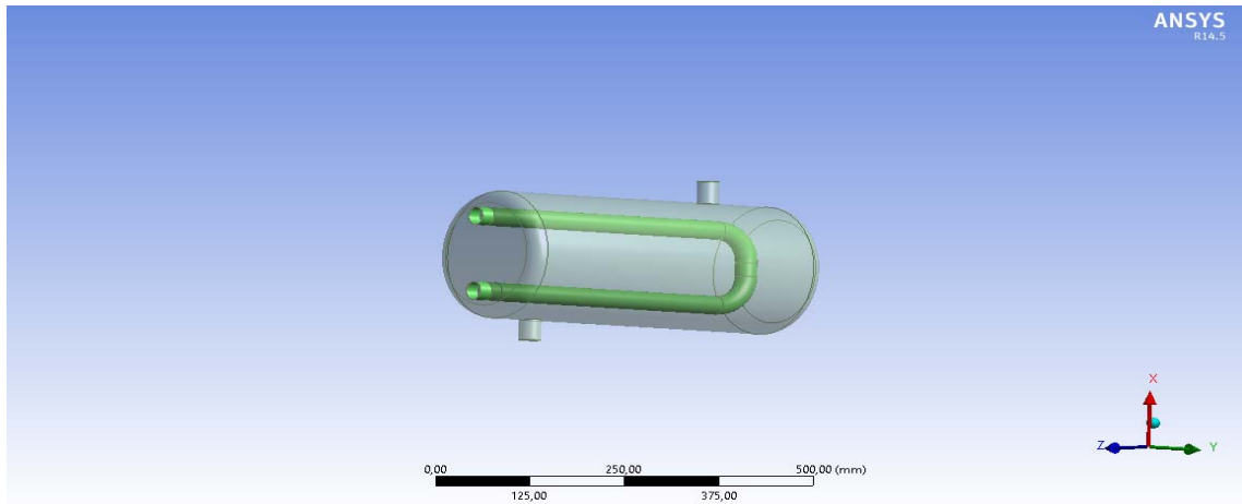
Şekil 3.2. Gövde boru tipi eşanjörün iç kısmının gösterilmesi
