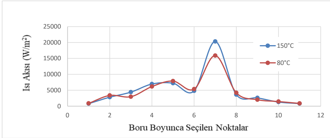
Şekil 4.19. 150° - 80°C de motoryağı ve 20°C de %0.75 TiO 2 /su nanoakışkanı için ısı akısı değişimi
