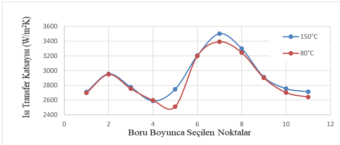
Şekil 4.8. 150° - 80°C de motoryağı ve 20°C de %0.3 TiO 2 /su nanoakışkanı için ısı transfer katsayısı değişimi
