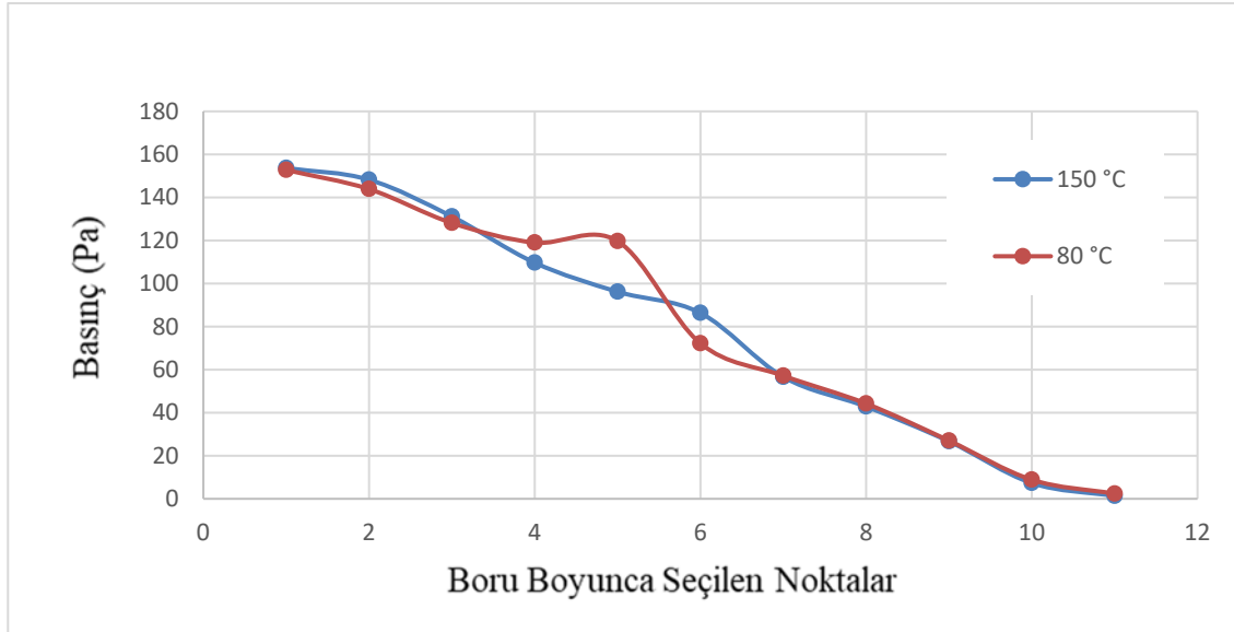
Şekil 4.4. 150°C - 80°C de motoryağı ve 20°C de saf su için basınç değişimi
