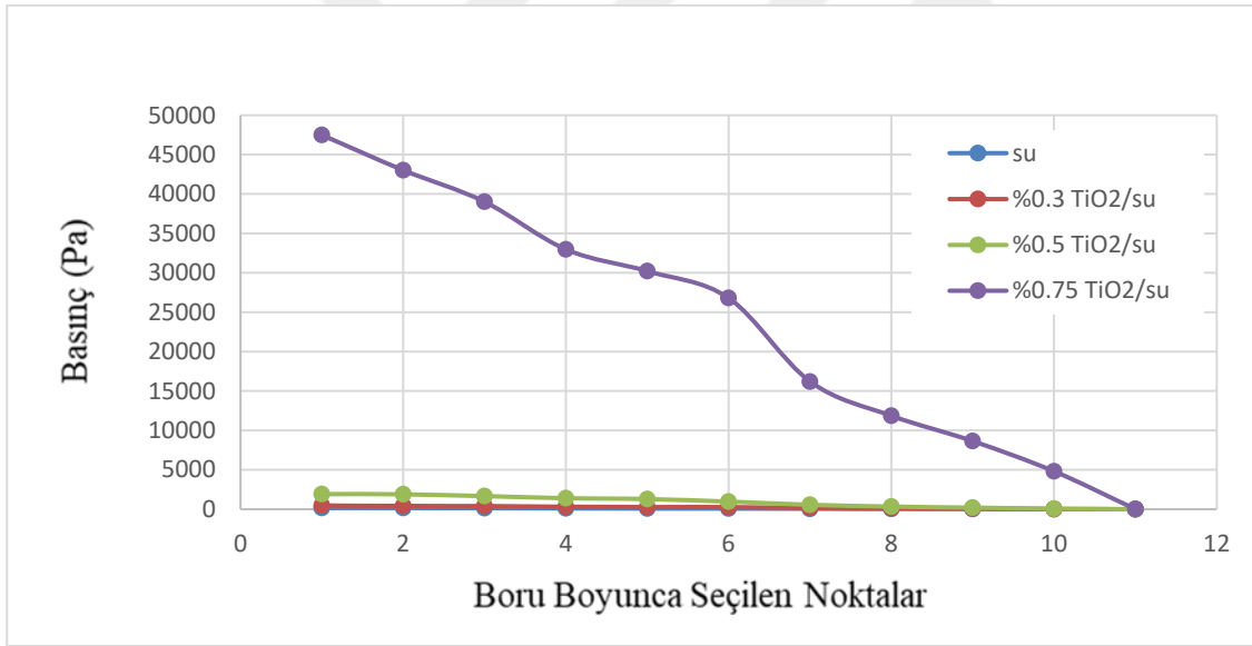
Şekil 4.30. 150°C de motoryağı ve 20°C de saf su, %0.3, %0.5 ve %0.75 oranlarında TiO 2 /su nanoakışkanlarının basınç değişimi
