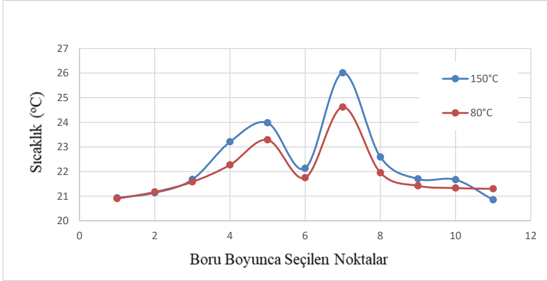
Şekil 4.11. 150° - 80°C de motoryağı ve 20°C de %0.3 TiO 2 /su nanoakışkanı için sıcaklık değişimi
