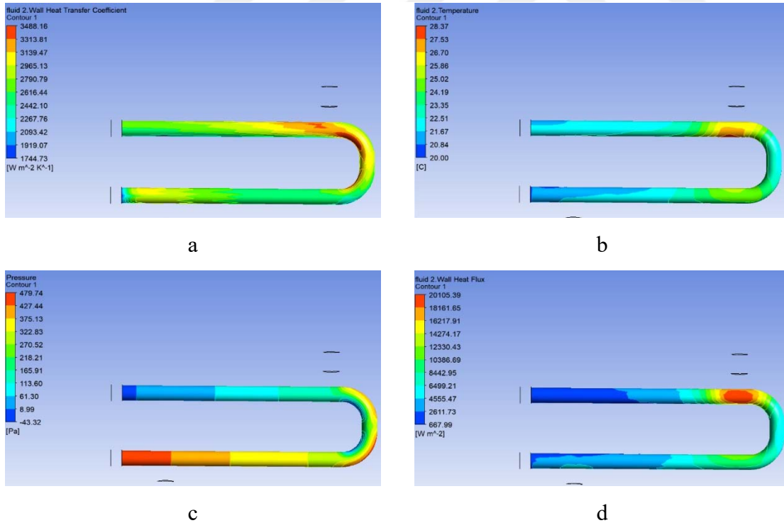
Şekil 4.20. 150°C de motoryağı ve 20°C de %0.3 TiO 2 /su nanoakışkanı için değişimler (a- ısı transfer katsayısı değişimi, b- sıcaklık değişimi, c- basınç değişimi, d- ısı akısı değişimi)
