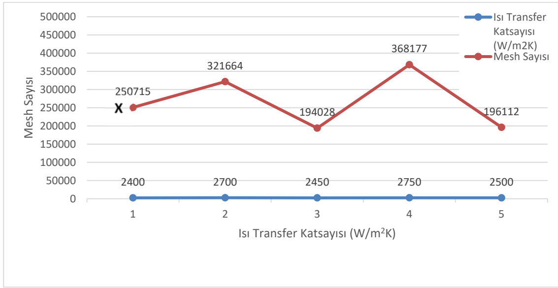
Şekil 3.7. Ağ yapısının eleman sayısına bağlı, sayısal analizden elde edilen ısı transferi
