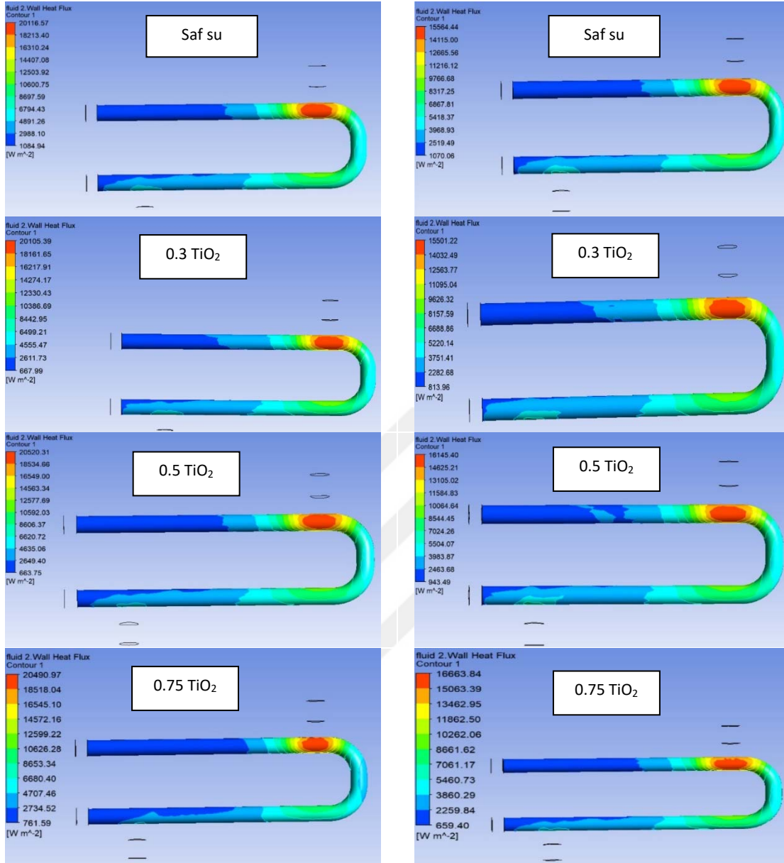
Şekil 4.37. 20°C de yukarıdan aşağıya sırasıyla saf su, %0.3, %0.5, %0.75 oranlarında \text{TiO}_2 /su nanoakışkanları için ısı akısı değişimleri (Sıcak akışkan olarak sol sütunda 150°C de motoryağı, sağ sütunda 80°C de motoryağı kullanılmıştır.)
