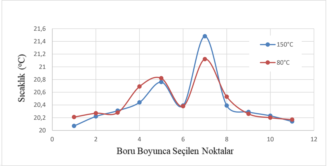
Şekil 4.13. 150° - 80°C de motoryağı ve 20°C de %0.75 TiO 2 /su nanoakışkanı için sıcaklık değişimi
