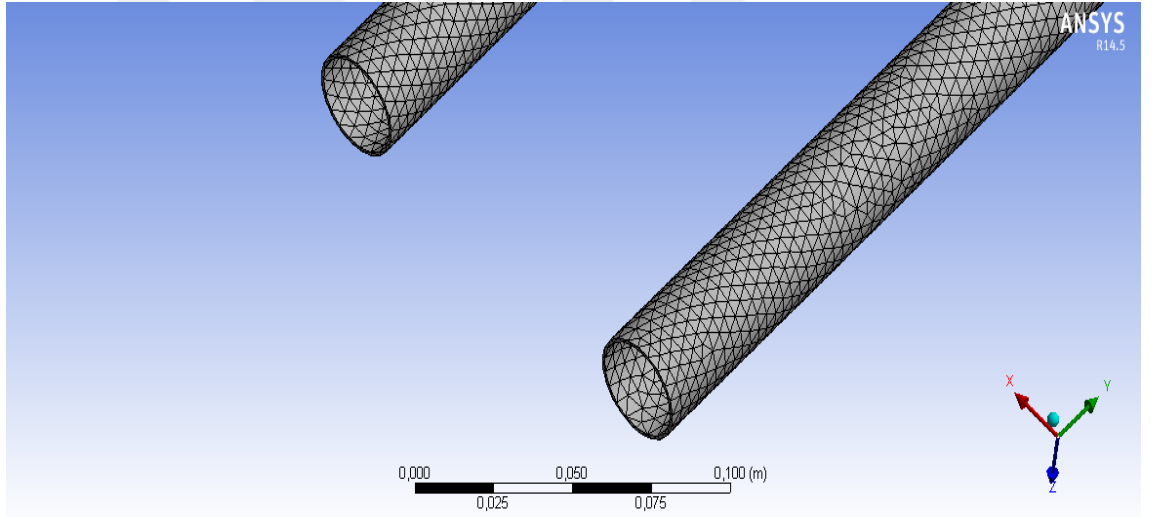
Şekil 3.6. Soğuk akışkanın geçtiği borunun ağ yapısı
