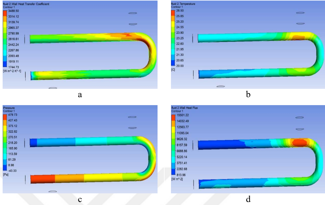
Şekil 4.21. 80°C de motoryağı ve 20°C de %0.3 TiO 2 /su nanoakışkanı için değişimler (a- ısı transfer katsayısı değişimi, b- sıcaklık değişimi, c- basınç değişimi, d- ısı akısı değişimi)
