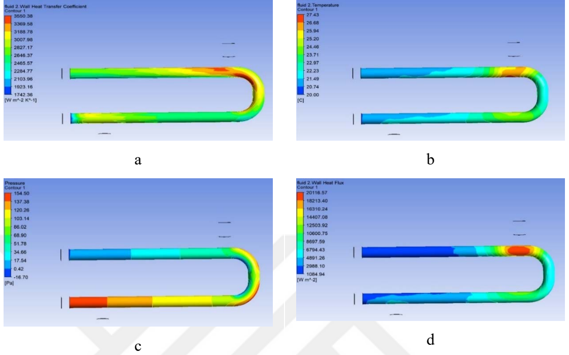
Şekil 4.6. 150°C de motoryağı ve 20°C de saf su için değişimler (a- ısı transfer katsayısı değişimi, b- sıcaklık değişimi, c- basınç değişimi, d- ısı akısı değişimi)
