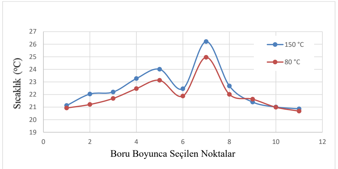
Şekil 4.3. 150°C - 80°C de motoryağı ve 20°C de saf su için sıcaklık değişimi
