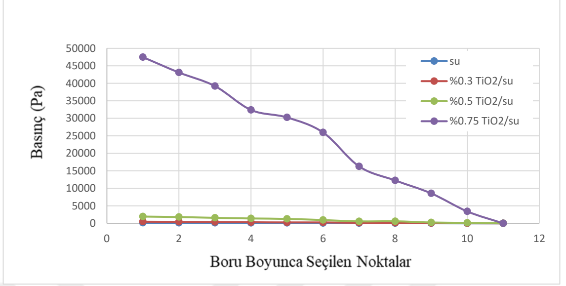
Şekil 4.31. 80°C de motoryağı ve 20°C de saf su, %0.3, %0.5 ve %0.75 oranlarında TiO 2 /su nanoakışkanlarının basınç değişimi
