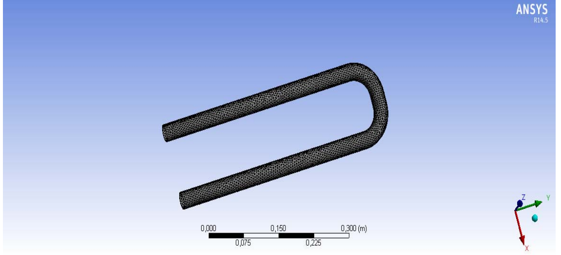
Şekil 3.5. Soğuk akışkanın geçtiği borunun ağ yapısı
