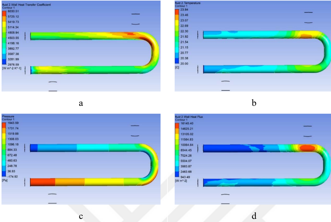
Şekil 4.23. 80°C de motoryağı ve 20°C de %0.5 \text{TiO}_2/\text{su} nanoakışkanı için değişimler (a- ısı transfer katsayısı değişimi, b- sıcaklık değişimi, c- basınç değişimi, d- ısı akısı değişimi)
