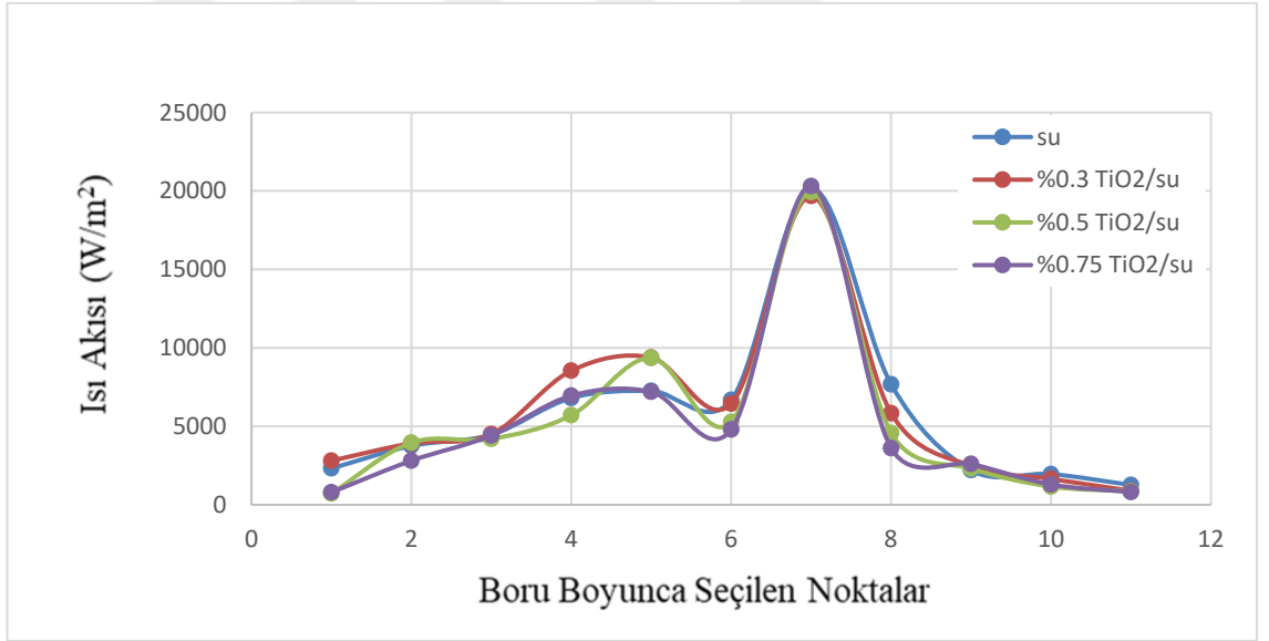
Şekil 4.32. 150°C de motoryağı ve 20°C de saf su, %0.3, %0.5 ve %0.75 oranlarında TiO 2 /su nanoakışkanlarının ısı akısı değişimi
