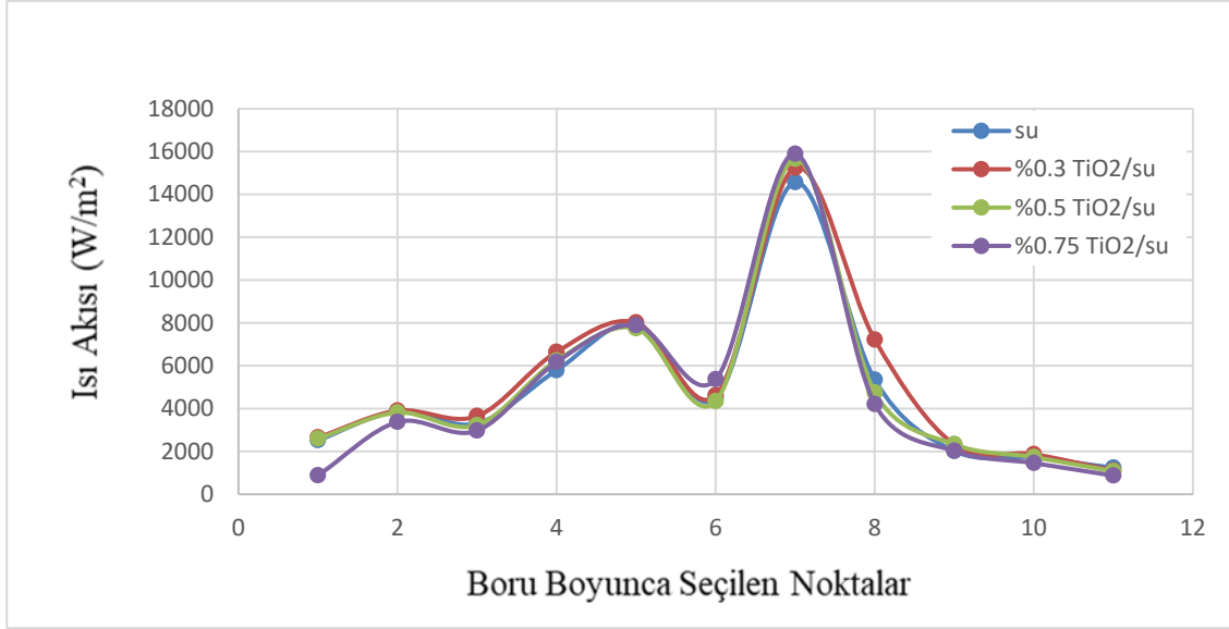
Şekil 4.33. 80°C de motoryağı ve 20°C de saf su, %0.3, %0.5 ve %0.75 oranlarında TiO 2 /su nanoakışkanlarının ısı akısı değişimi.
