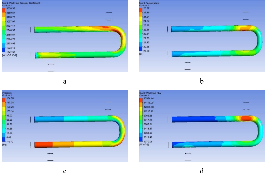
Şekil 4.7. 80°C de motoryağı ve 20°C de saf su için değişimler (a- ısı transfer katsayısı değişimi, b- sıcaklık değişimi, c- basınç değişimi, d- ısı akısı değişimi)
