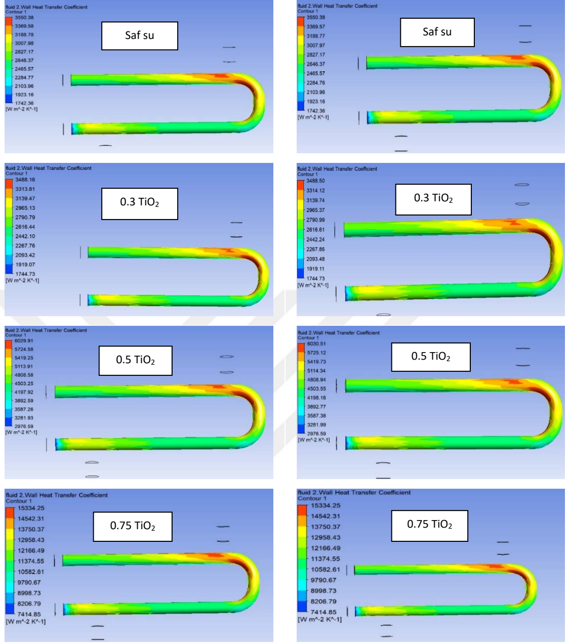
Şekil 4.34. 20°C de yukarıdan aşağıya sırasıyla saf su, %0.3, %0.5, %0.75 oranlarında TiO 2 /su nanoakışkanları için ısı transfer katsayısı değişimleri (Sıcak akışkan olarak sol sütunda 150°C de motoryağı, sağ sütunda 80°C de motoryağı kullanılmıştır.)
