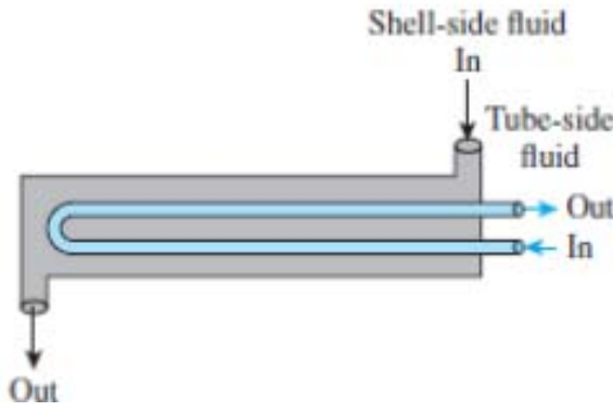
Şekil 2.3. Tek gövde ve iki boru geçişli gövde boru tipi eşanjör (Zohuri 2017)
