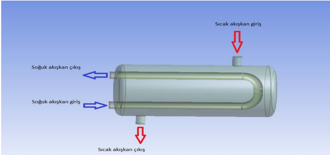
Şekil 3.3. Gövde boru tipi eşanjörde sıcak ve soğuk akışkanın giriş ve çıkışları
