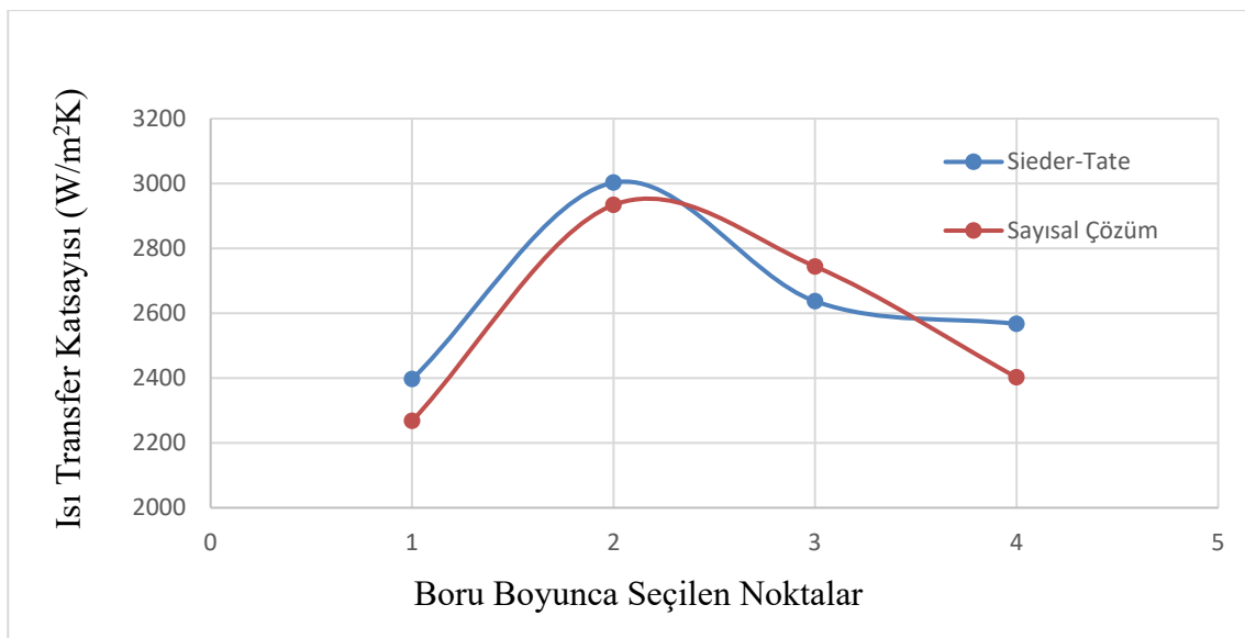
Şekil 3.8. Sayısal çözümün literatür ile karşılaştırılması
