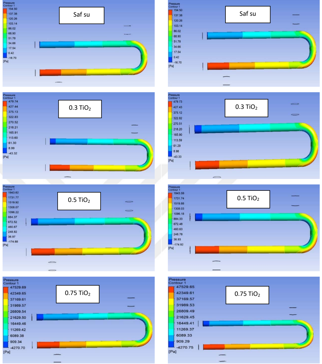
Şekil 4.36. 20°C de yukarıdan aşağıya sırasıyla saf su, %0.3, %0.5, %0.75 oranlarında \text{TiO}_2 /su nanoakışkanları için basınç değişimleri (Sıcak akışkan olarak sol sütunda 150°C de motoryağı, sağ sütunda 80°C de motoryağı kullanılmıştır.)
