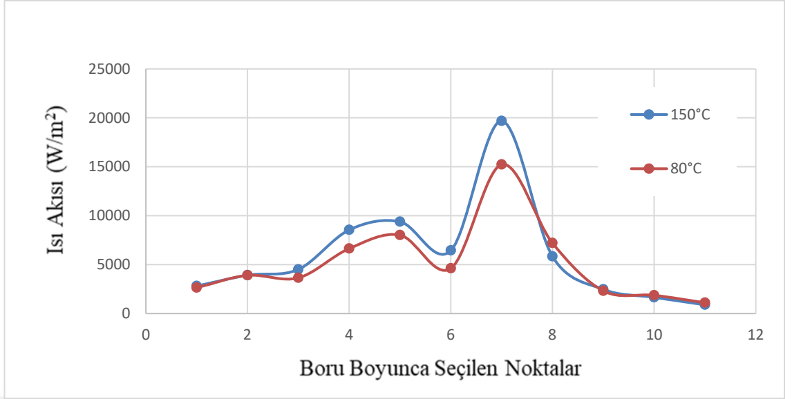
Şekil 4.17. 150° - 80°C de motoryağı ve 20°C de %0.3 TiO 2 /su nanoakışkanı için ısı akısı değişimi
