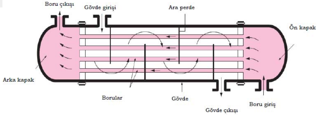
Şekil 2.2. Gövde boru tipi eşanjör (Zohuri 2017)
