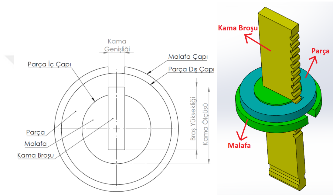
Şekil 3.8 Delik içi kama broş takımlarında parça, malafa ve broş takımının gösterimleri
