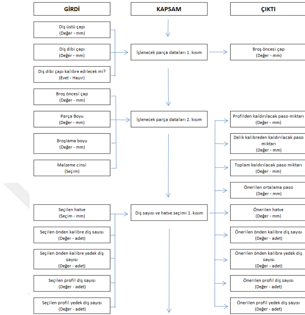
Şekil 3.6 Yuvarlak broş takımı tasarımında girdi, çıktı ve kapsam ilişkileri 1. kısım
