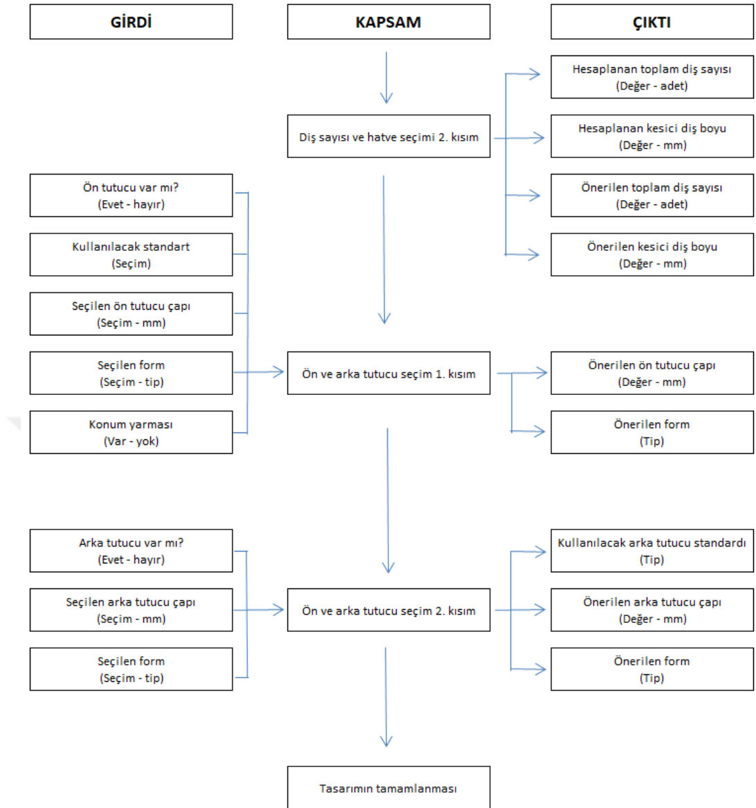
Şekil 3.7 Yuvarlak broş takımı tasarımında girdi, çıktı ve kapsam ilişkileri 2. kısım
