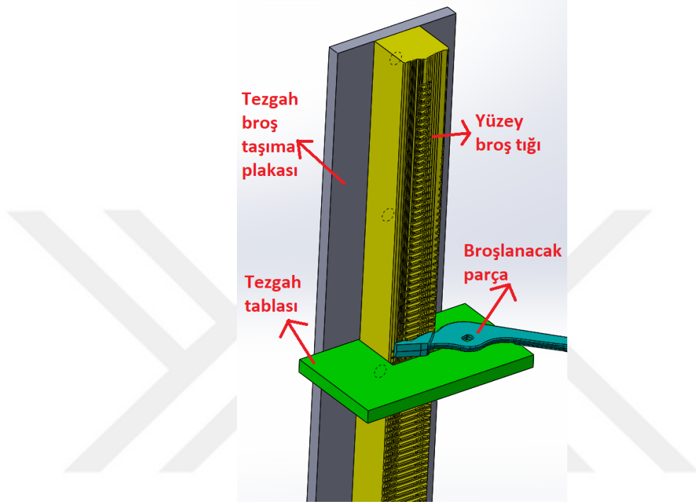
Şekil 3.15 Yüzey broş takımlarında parça, takım ve tezgâh yerleşimi
