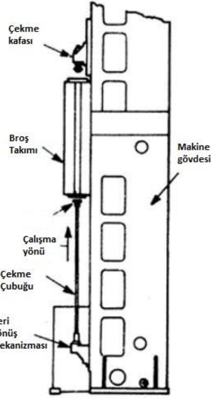
Şekil 2.6 Dikey bir broş çekme tezgâhı [24]
