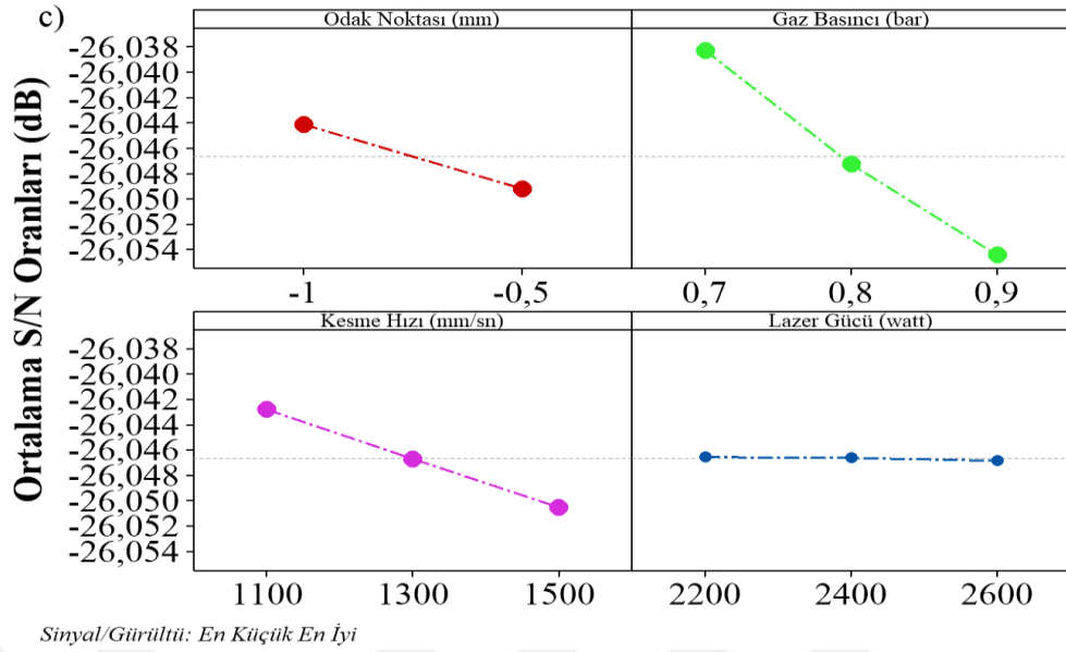
Şekil 7.9. Alt delik çapları için lazer delme deneylerinde S/N oranı grafiği.
