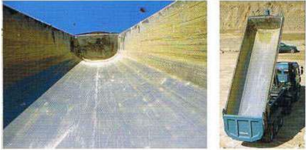
Şekil 5.1. Hardox aşınma levhasından imal edilmiş bir damper kasası [8].
