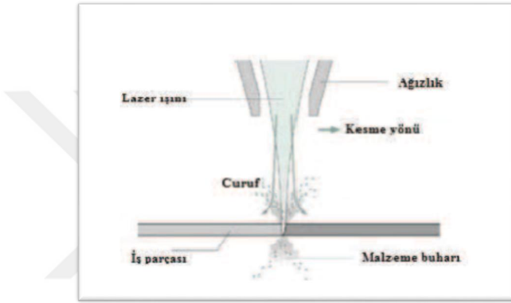
Şekil 4.1. Lazer-süblimleştirme kesme sistemi [49].
