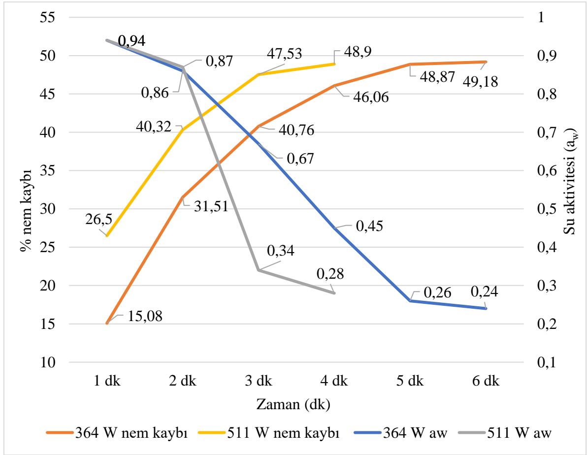
Şekil 4. 3 Mikrodalga fırın ile 364W ve 511W güçte yapılan kurutma ön denemesinde zeytin hamurlarının nem kaybı ve su aktivitesi değerlerinin zamanla değişimi
