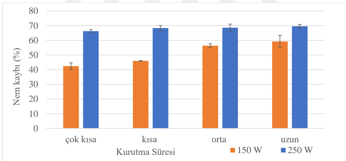
Şekil 4.6 Kızılötesi lamba ile kurutulmuş zeytin hamurlarına ait nem kaybının zamanla değişimi
