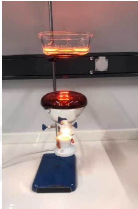
Şekil 3. 4 Kızılötesi lamba ile kurutma düzeneği
