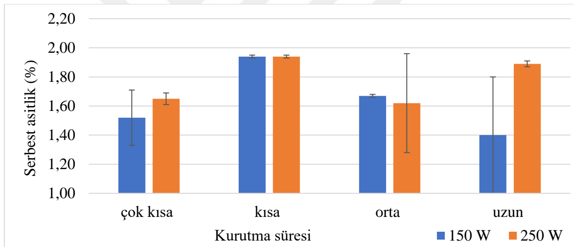
Şekil 4. 12 Kızılötesi lamba ile kurutulmuş zeytin hamurlarına serbest asitlik değerlerinin zamanla değişimi
