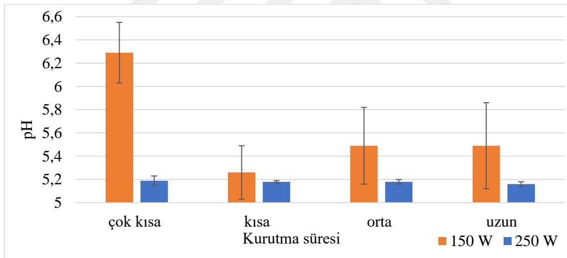
Şekil 4. 10 Kızılötesi lamba ile kurutulmuş zeytin hamurlarına ait pH değerlerinin zamanla değişimi
