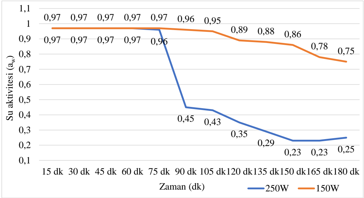
Şekil 4. 1 Kızılötesi lamba ile 150W ve 250W güçte yapılan kurutma ön denemesinde zeytin hamurlarının su aktivitesi değerlerinin zaman ile değişimi
