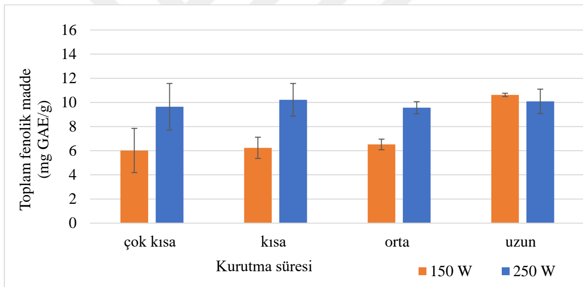
Şekil 4. 26 Kızılötesi lamba ile kurutulmuş zeytin hamurlarının toplam fenolik madde miktarlarının zamanla değişimi
