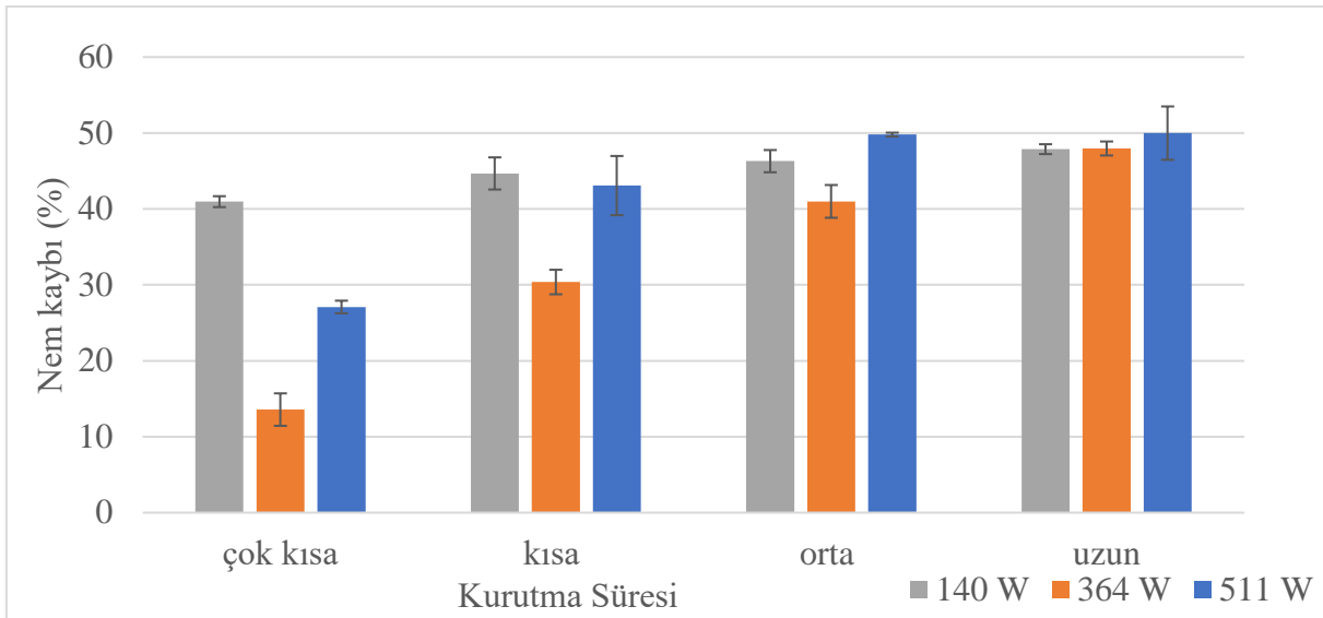
Şekil 4. 7 Mikrodalga fırında kurutulmuş zeytin hamurlarına ait nem kaybının zamanla değişimi
