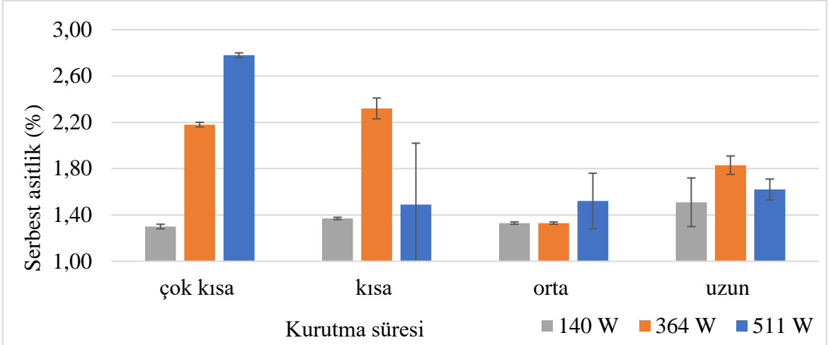
Şekil 4. 13 Mikrodalga fırın ile kurutulmuş zeytin hamurlarına serbest asitlik değerlerinin zamanla değişimi
