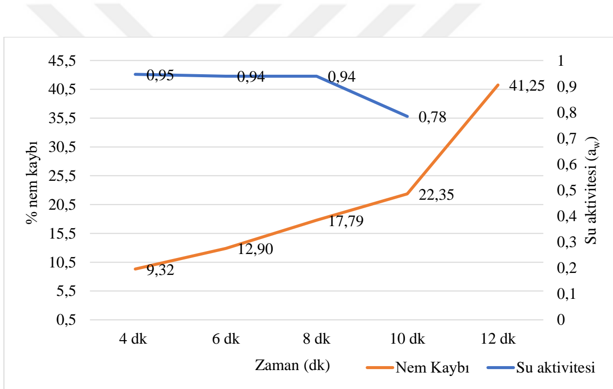
Şekil 4. 4 Mikrodalga fırın ile 140W güçte yapılan kurutma ön denemesinde zeytin hamurlarının nem kaybı ve su aktivitesi değerlerinin zamanla değişimi
