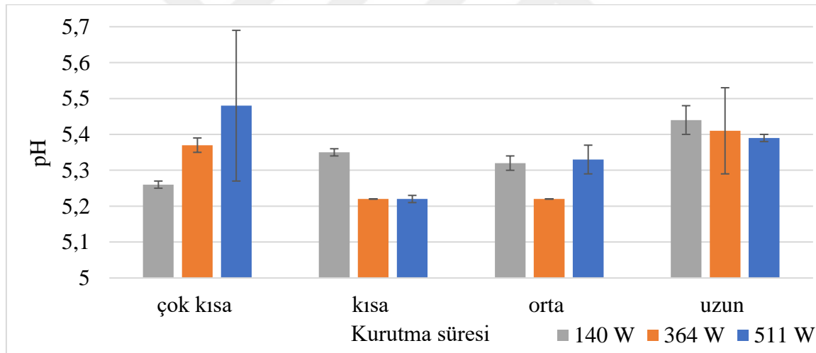
Şekil 4. 11 Mikrodalga fırın ile kurutulmuş zeytin hamurlarına ait pH değerlerinin zamanla değişimi
