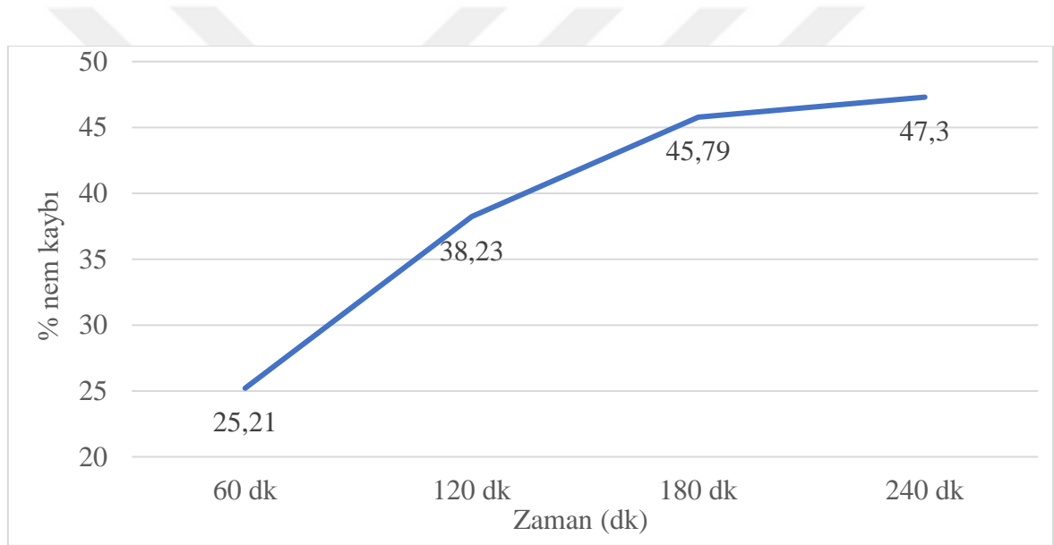
Şekil 4. 5 Etüv ile kurutulan zeytin hamurlarının nem kaybı değerlerinin zamanla değişimi
