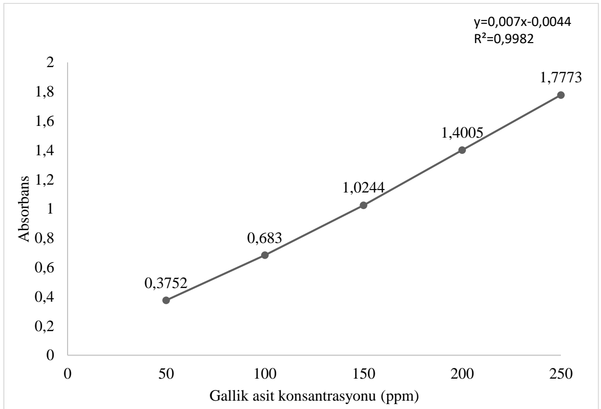
Şekil 4. 24 Gallik asit kalibrasyon eğrisi
