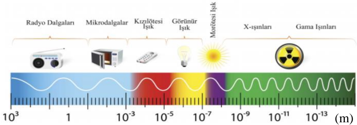
Şekil 2. 3 Elektromanyetik Spektrum [(TÜBİTAK, 2023) alınarak revize edilmiştir.]
