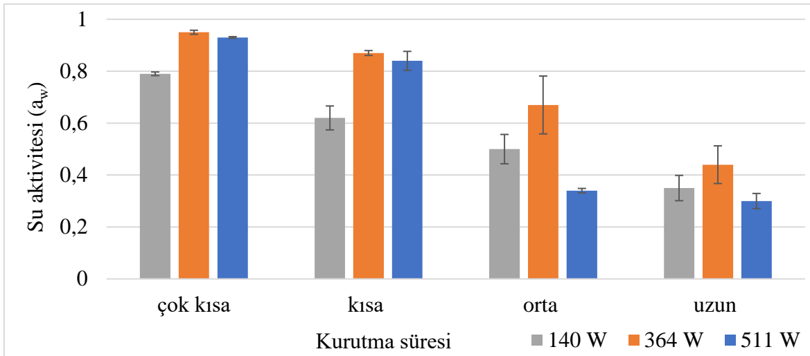
Şekil 4. 9 Mikrodalga fırın ile kurutulmuş zeytin hamurlarına ait su aktivitesi değerlerinin zamanla değişimi
