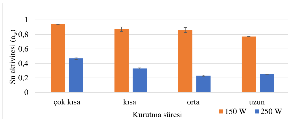
Şekil 4. 8 Kızılötesi lamba ile kurutulmuş zeytin hamurlarına ait su aktivitesi değerlerinin zamanla değişimi
