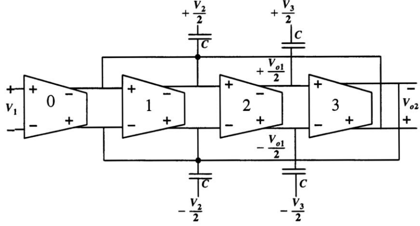
Şekil 4.23. FinFET OTA-C kullanılarak gerçekleştirilen biquad'ın diferansiyel versiyonu
