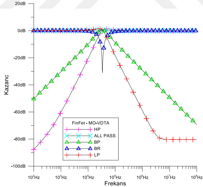
Şekil 5.17. Şekil 5.16'da önerilen filtre için simüle edilmiş LP, BP, HP ve BS yanıtları
