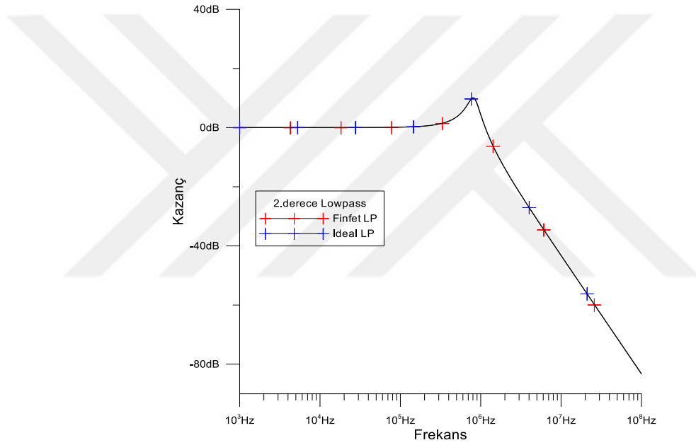
Şekil 4.27. Aktif ve pasif alçak geçiren filtresi
