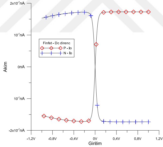
Şekil 4.18. Gelişmiş FinFET OTA Dc. çıkış direnci karakteristiği
