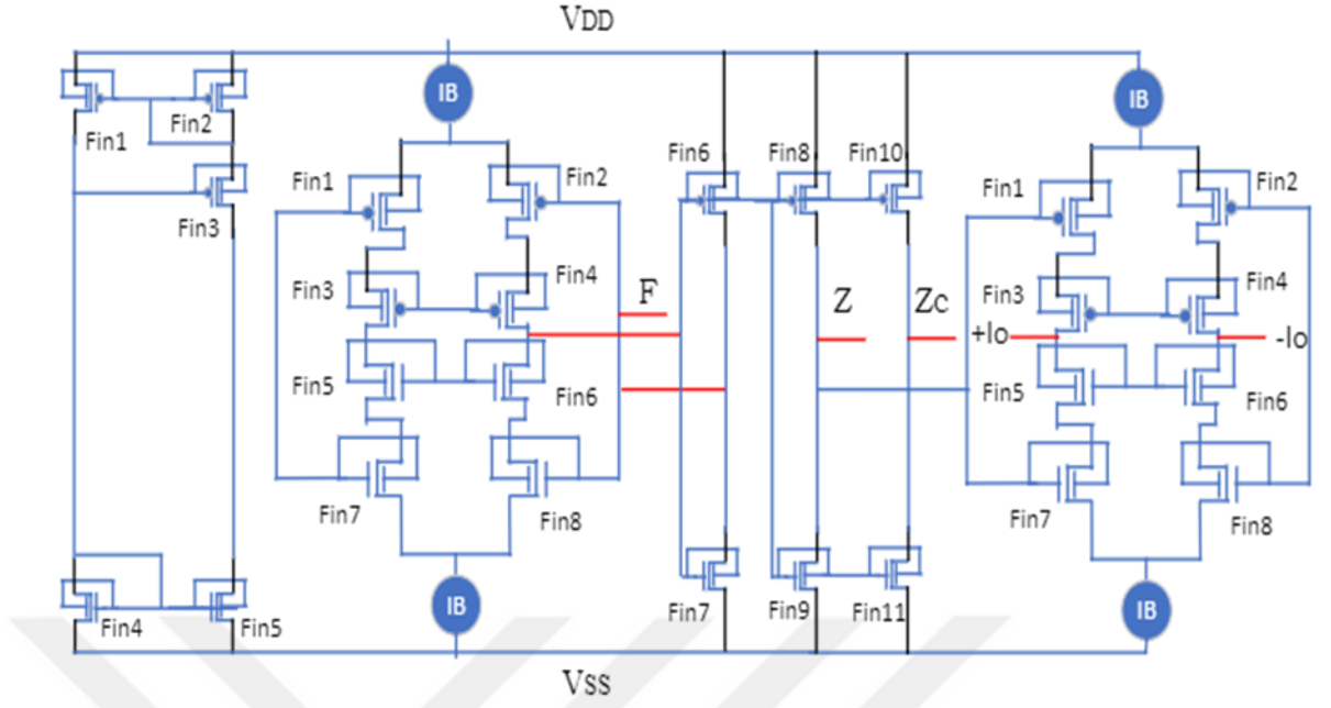
Şekil 5.34. Kullanılan ZC-CFTA'nın FinFET uygulaması
