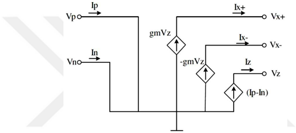
Şekil 5.21. CDTA'nın blok diyagramı
