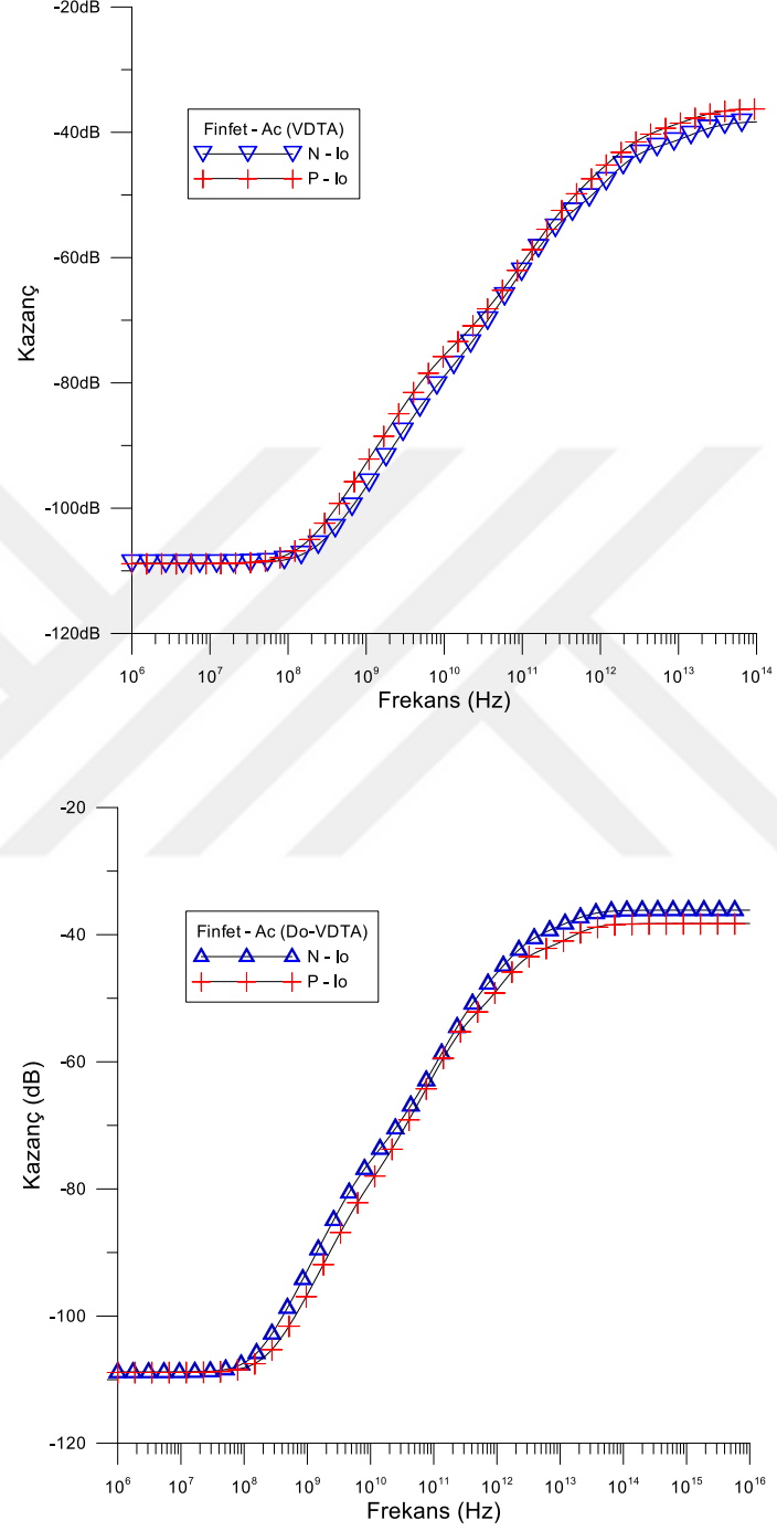
Şekil 5.9. VDTA ve DO-VDTA'nın frekans tepkileri
