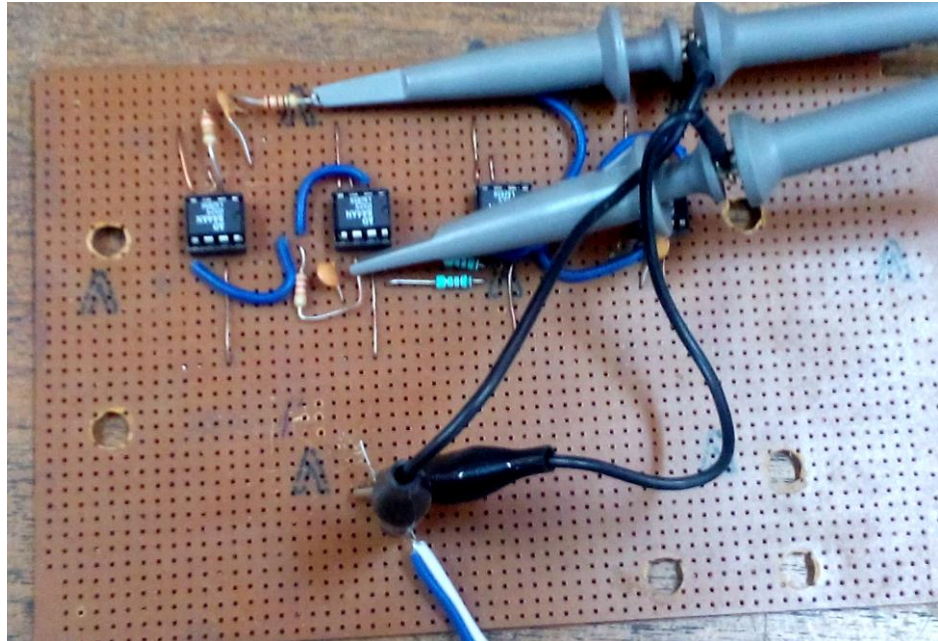
Şekil 6.47. Şekil 6.37'de gösterilen TOQSO için deneysel kurulum
