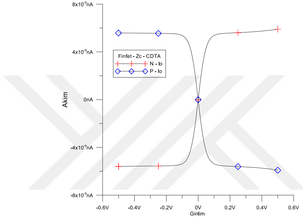
Şekil 5.25. FinFET Mu-Zc-CDTA'nın DC transfer özellikleri
