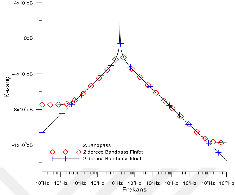
Şekil 4.26. Aktif ve pasif bant geçiren filtresi
