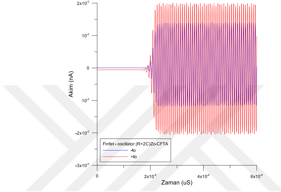
Şekil 6.41. Kuadratur osilatörün akım dalga formlarının simülasyon sonuçları
