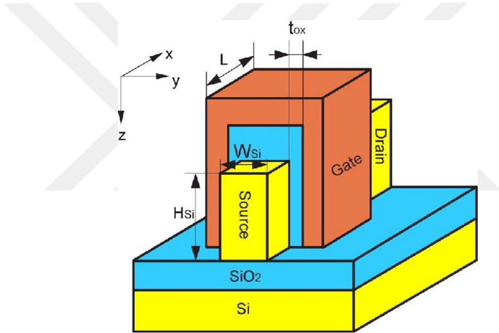
Şekil 3.12. Üçlü kapılı FinFET yapısının üç boyutlu şeması
