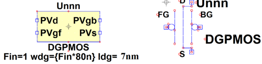
Şekil 3.17. DGPMOS sembolü
