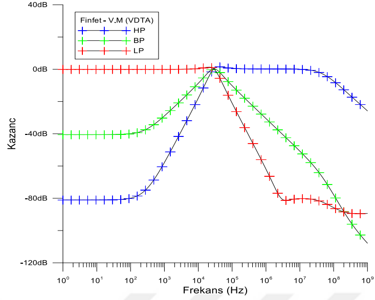
Şekil 5.13. Şekil 9'daki aktif voltaj modu çok işlevli filtre için simüle edilmiş AC transfer yanıtları
