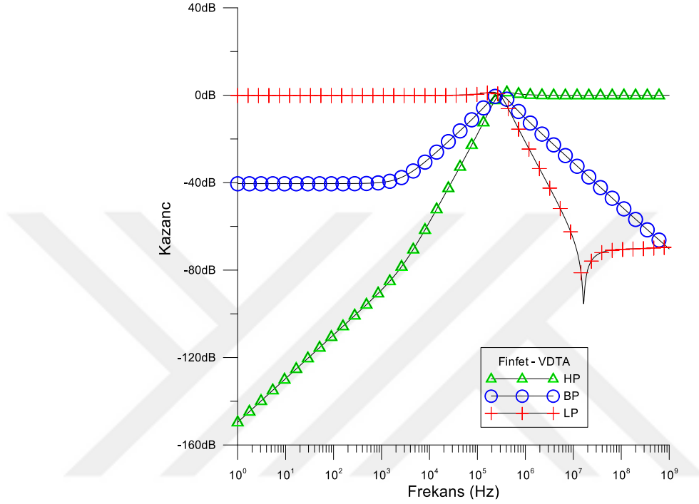
Şekil 5.11. Finfet VDTA kullanarak LP, BP, HP filtrelerinin frekans tepkileri
