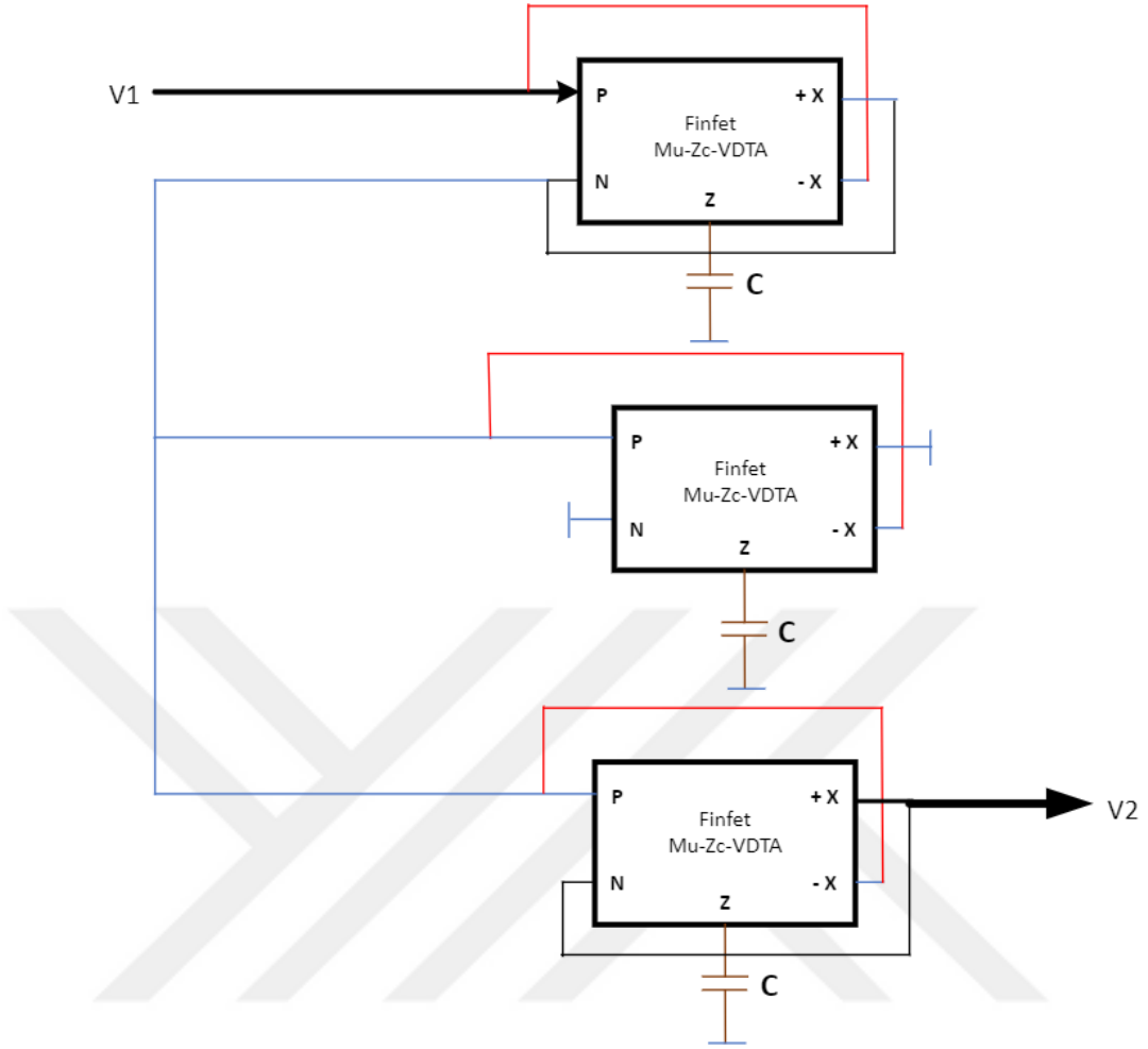
Şekil 6.11. Önerilen yapay transformatör devresi tabanlı üç Mu-Zc-VDTA
