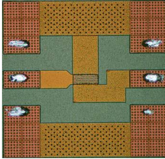
Şekil 3.13. Test çerçeveli devrenin kalıp resmi.
