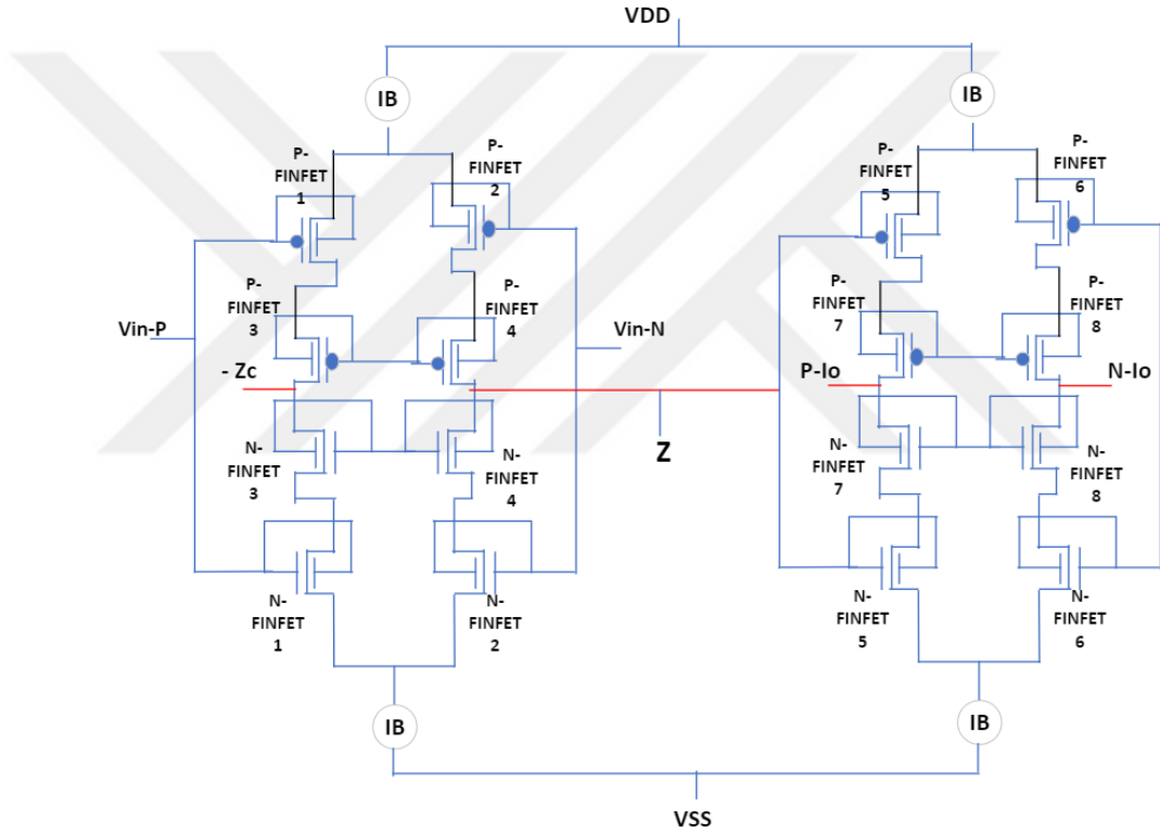
Şekil 5.4. Ek Z-kopyası ile VDTA'nın FinFET uygulaması
