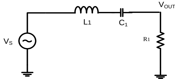
Şekil 4.24. Pasif bant geçiren RLC filtresi
