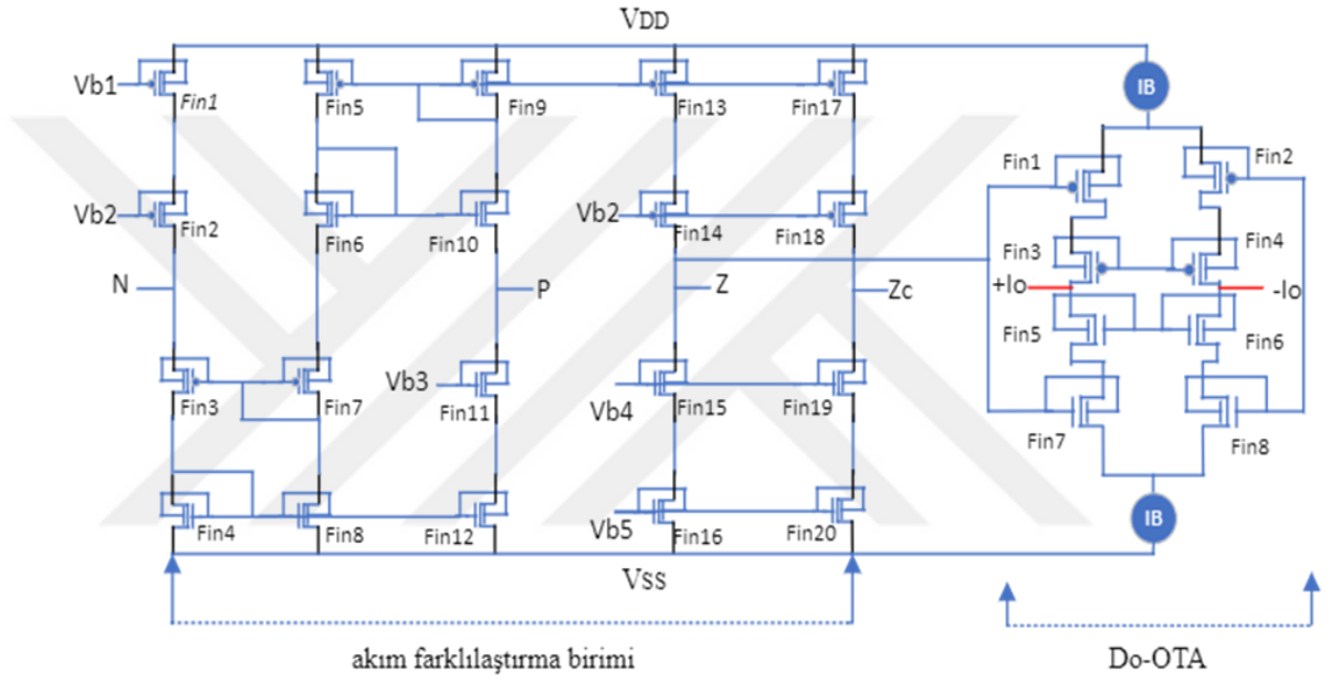
Şekil 5.24. Mu-Zc-CDTA'nın FinFET Gerçekleştirilmesi
