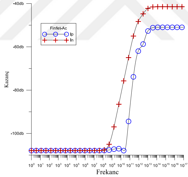
Şekil 4.8. Klasik FinFET OTA Ac akım karakteristiği
