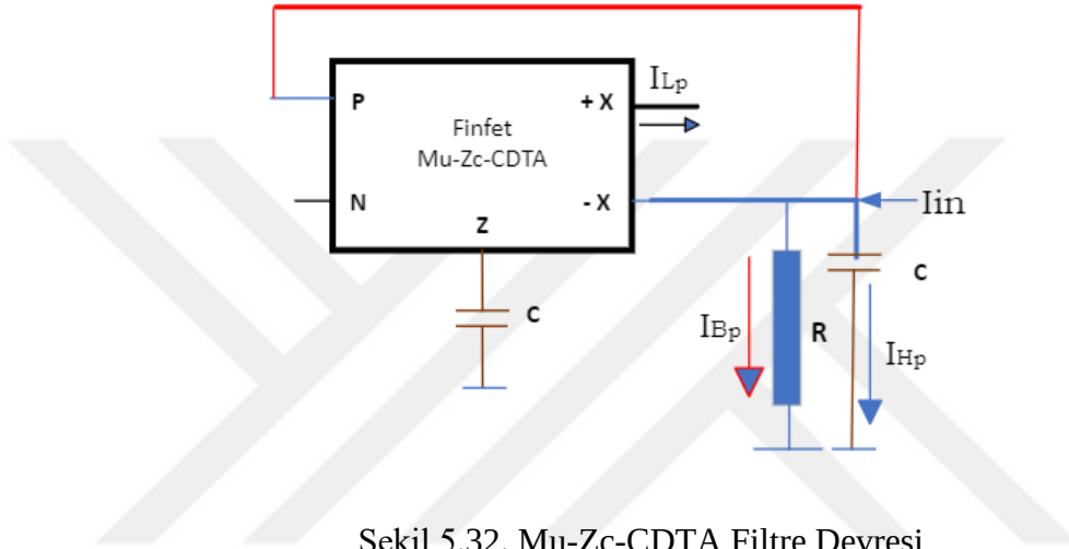
Şekil 5.32. Mu-Zc-CDTA Filtre Devresi
