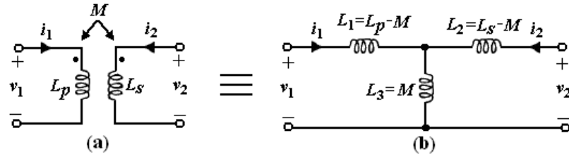
Şekil 6.20. a) Karşılıklı bağlantılı devrenin sembolü, b) eş değer devresi
