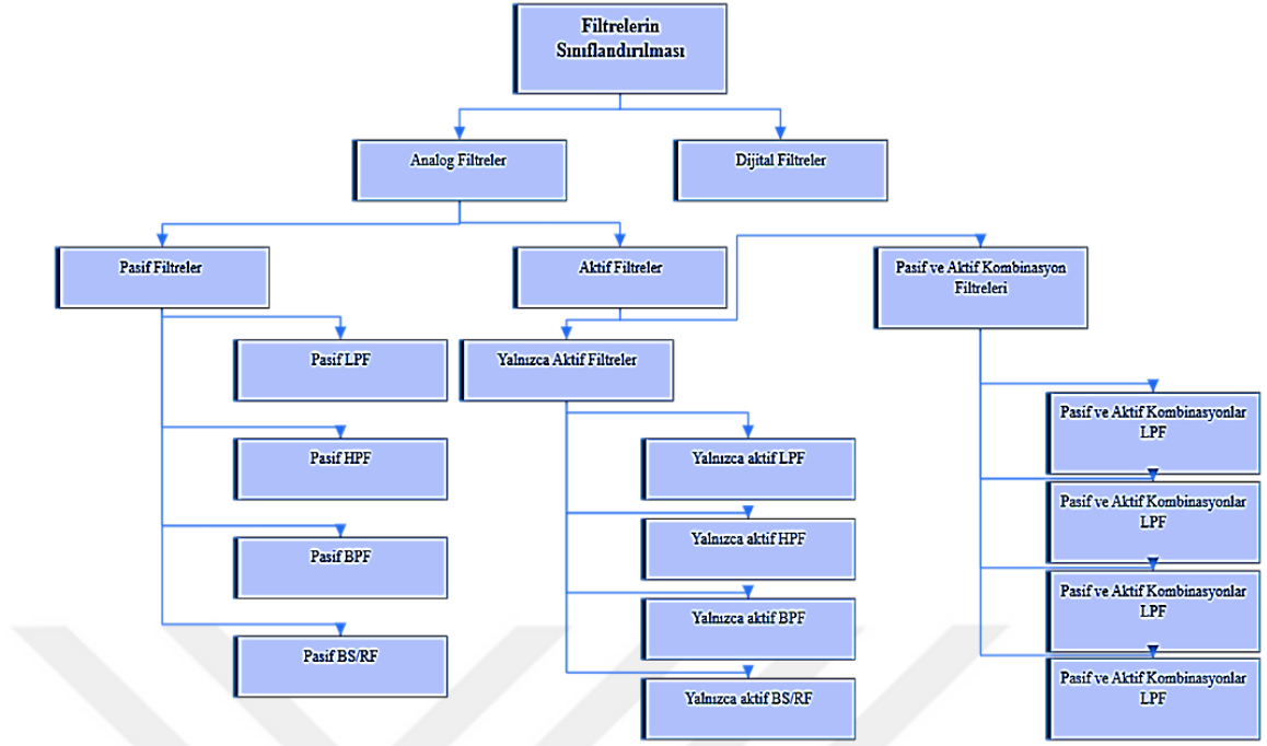
Şekil 2.1. Filtrelerin sınıflandırılması
