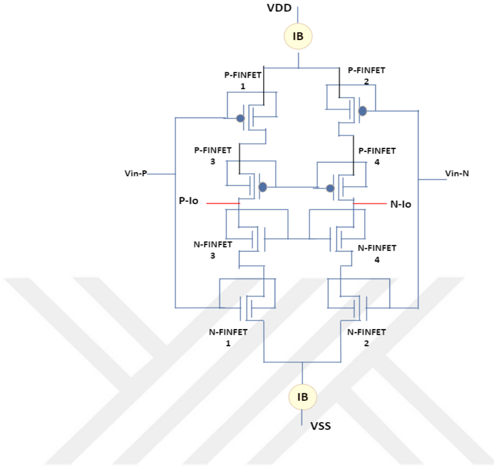
Şekil 4.11. Gelişmiş FinFET OTA yapısının şematik gösterimi
