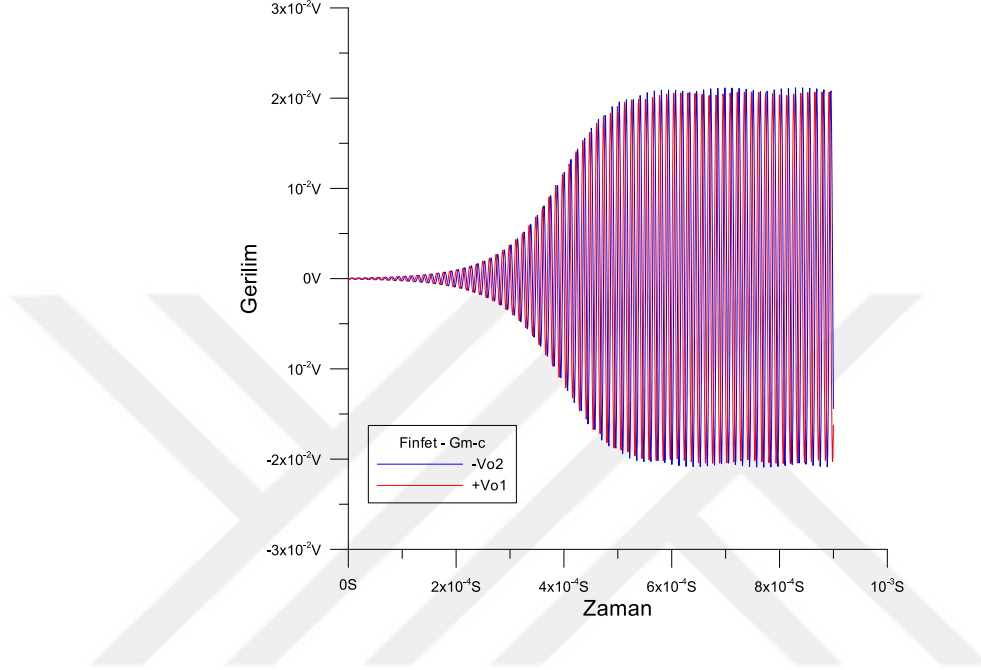
Şekil 6.27. Gm-c osilatörünün voltaj çıkışları
