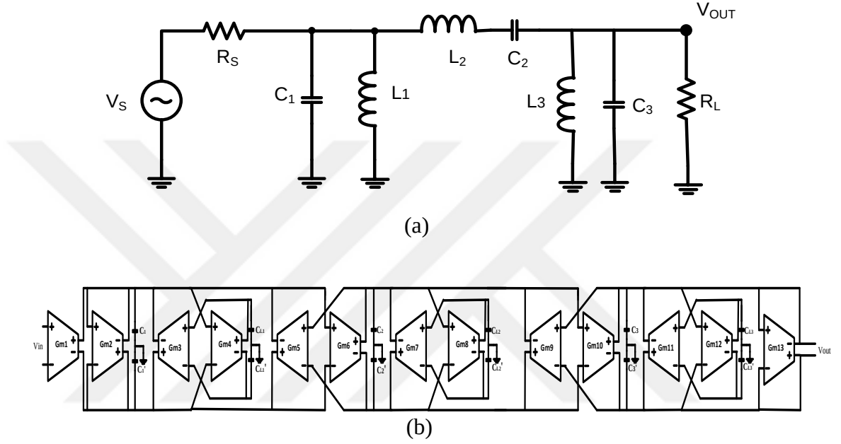
Şekil 4.31. FinFET OTA-C 6. dereceden bant geçiren Butterworth filtresi a) Pasif elemanlar ile gerçekleştirilmesi b) Aktif 6. derecede FinFET OTA-c f
