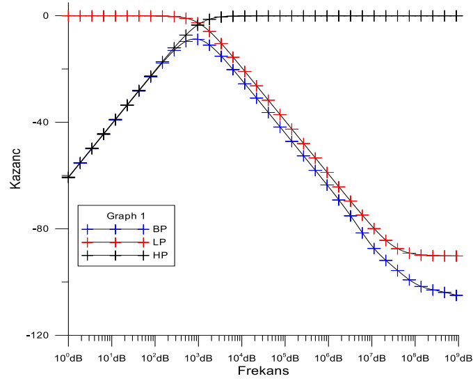
Şekil 5.33. Önerilen Mu-Zc-CDTA filtre devresinin frekans tepkisi
