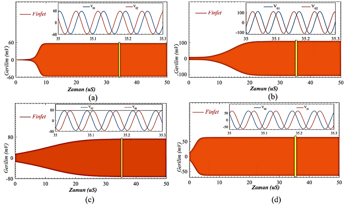
Şekil 6.29. Şekil 6.26'da önerilen TOQSO'ların simüle edilmiş geçici ve kararlı durum yanıtlarını göstermektedir.
