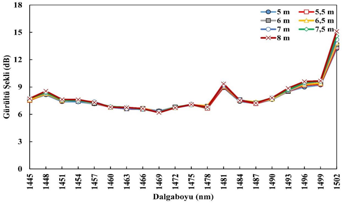
Şekil 6.62. ÜADG-TKFY I için TKF boyu-gürültü şekli değişimi
