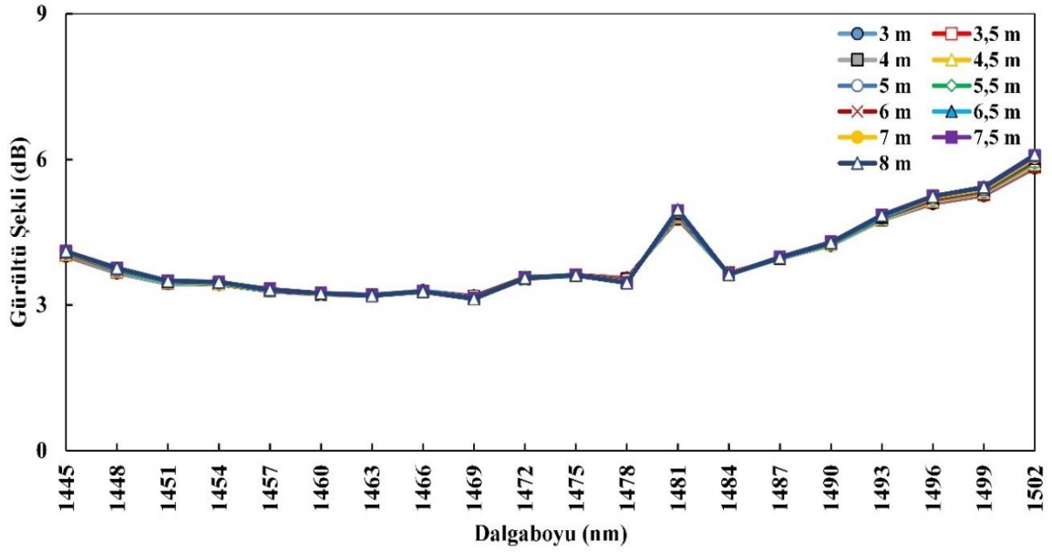
Şekil 6.45. ÜAÜG-TKFY için TKF 2 boyu-gürültü şekli değişimi
