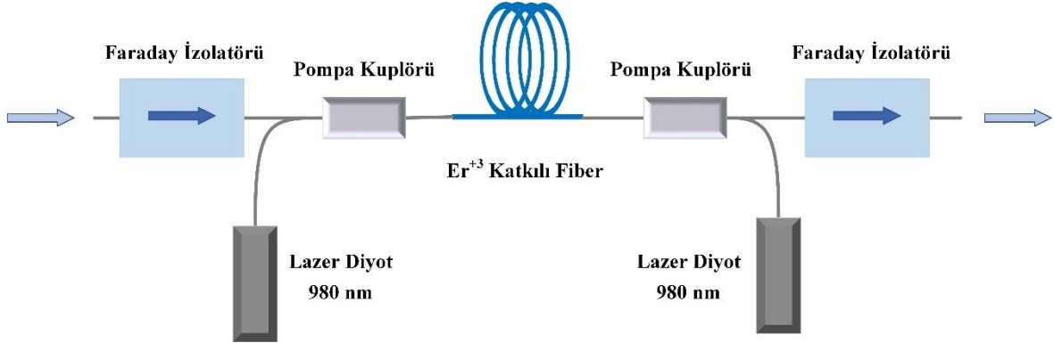
Şekil 3.4. EKFY'nin basit şematik gösterimi
