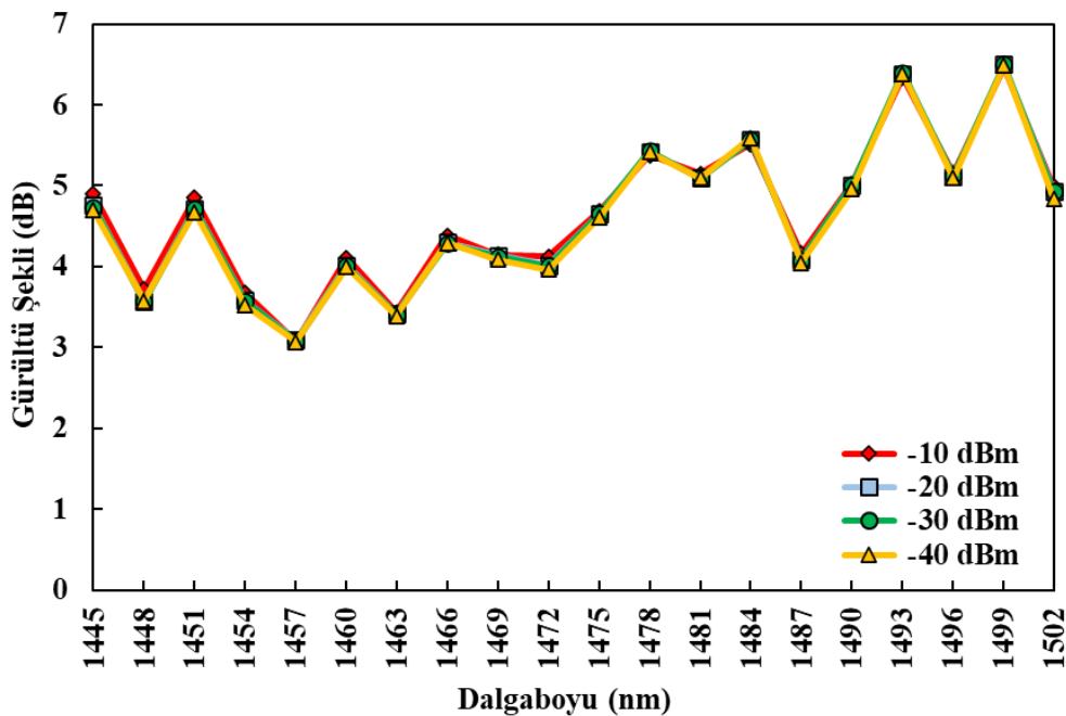
Şekil 6.15. İAÇG-TKFY için Giriş gücü-gürültü şekli değişimi
