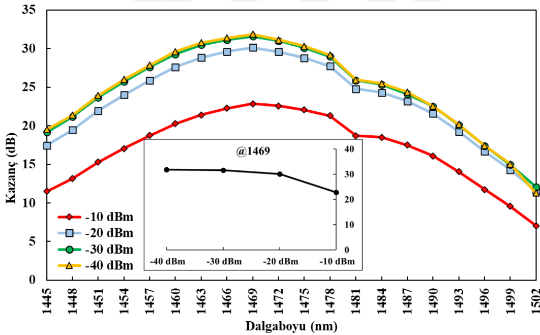
Şekil 6.57. ÜADG-TKFY I için giriş gücü-kazanç değişimi
