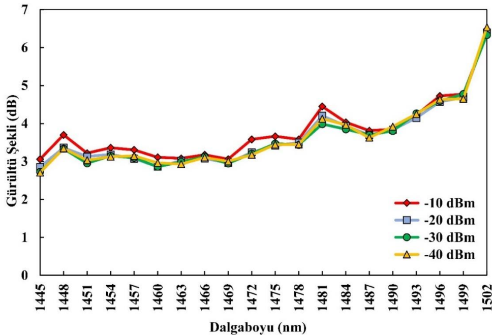
Şekil 6.7. ÇG-TKFY için giriş gücü-gürültü şekli değişimi
