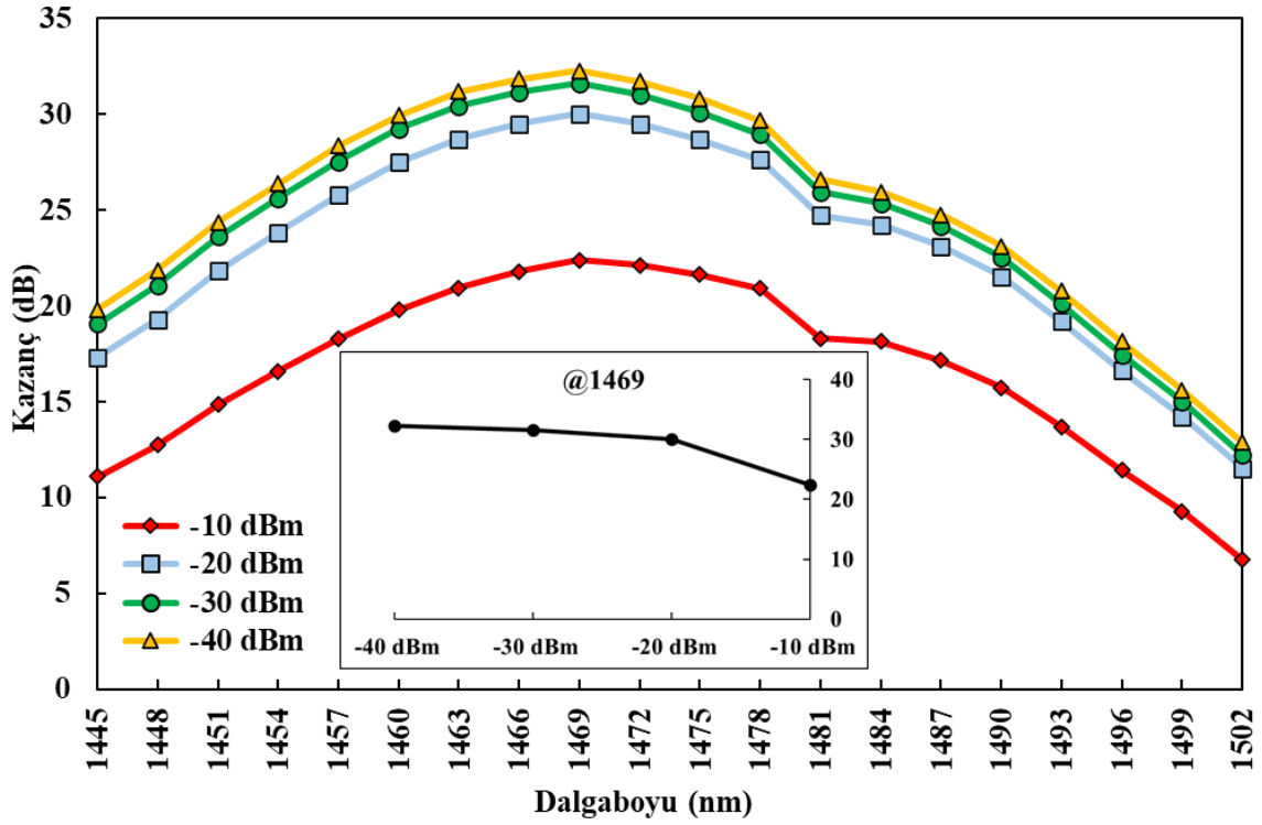
Şekil 6.65. ÜADG-TKFY II için giriş gücü-kazanç değişimi
