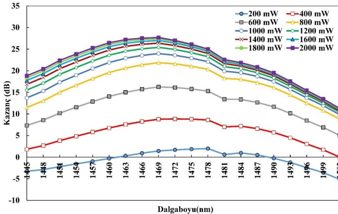
Şekil 6.42. ÜAÜG-TKFY için pompa gücü-kazanç değişimi
