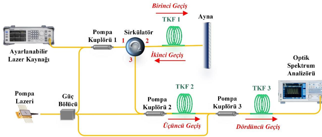
Şekil 6.72. Üç aşama dört geçiş TKFY III
