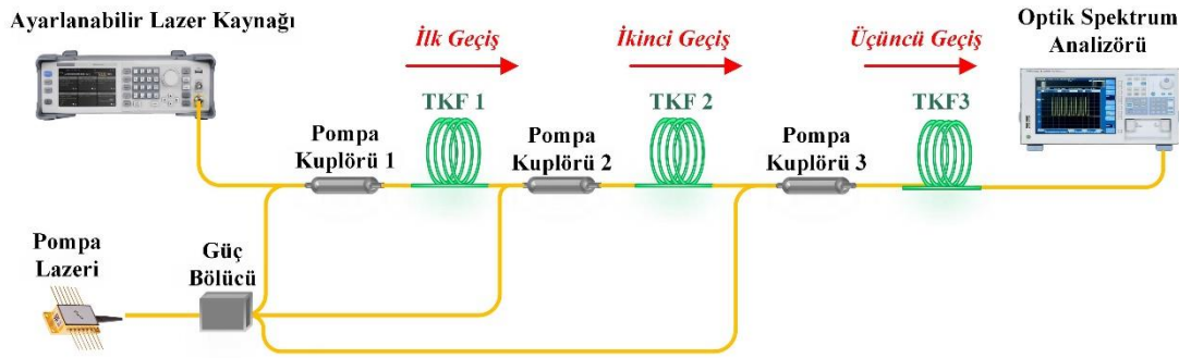
Şekil 6.39. Üç aşamalı üç geçişli TKFY
