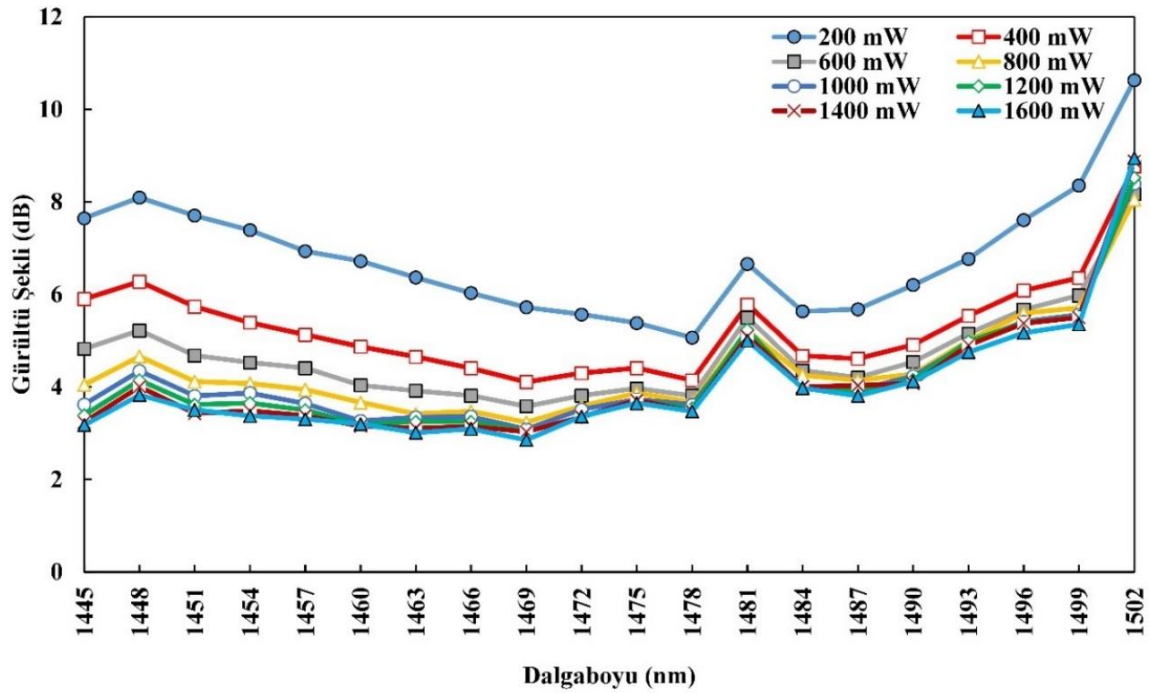
Şekil 6.52. İADG-TKFY için pompa gücü-gürültü şekli değişimi
