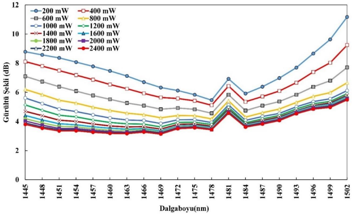
Şekil 6.84. DADG-TKFY için giriş gücü-gürültü şekli değişimi
