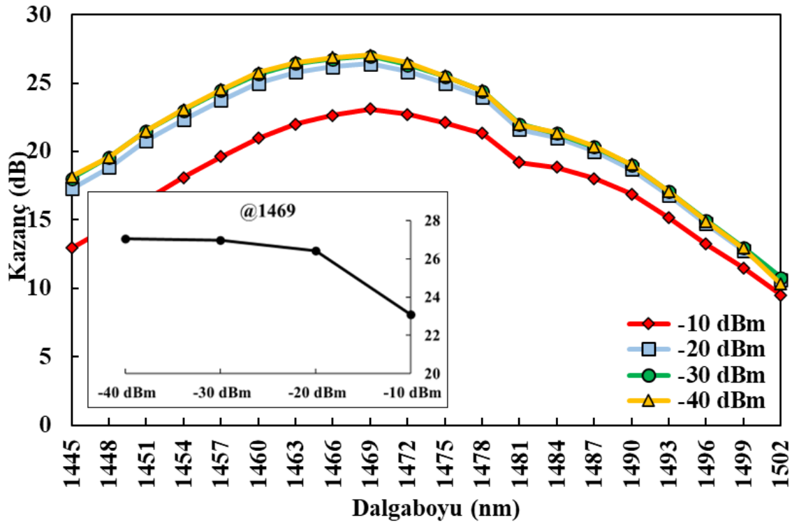
Şekil 6.24. İAÜG-TKFY I için giriş gücü-kazanç değişimi
