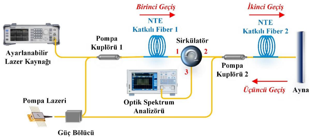
Şekil 5.4. İki aşamalı üç geçişli yükselteç konfigürasyonu I
