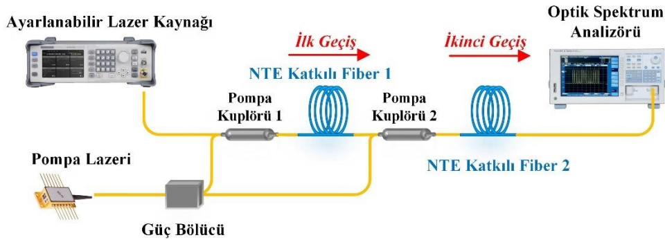
Şekil 5.3. İki aşamalı çift geçişli yükselteç tasarımı
