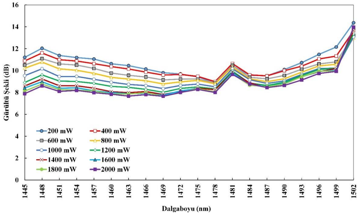
Şekil 6.76. ÜADG-TKFY III için pompa gücü-gürültü şekli değişimi
