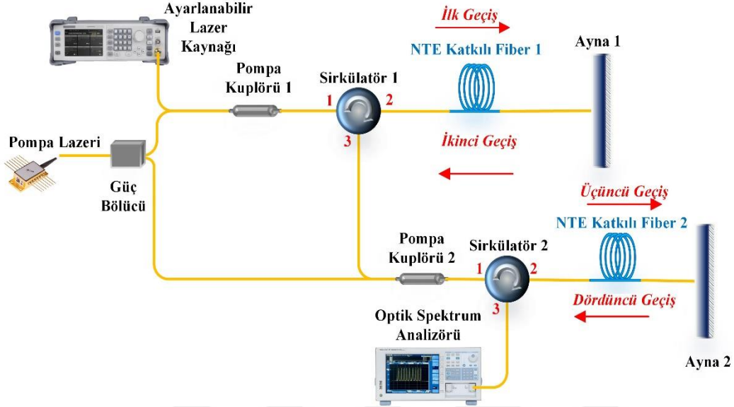
Şekil 5.7. İki aşamalı dört geçişli yükselteç konfigürasyonu
