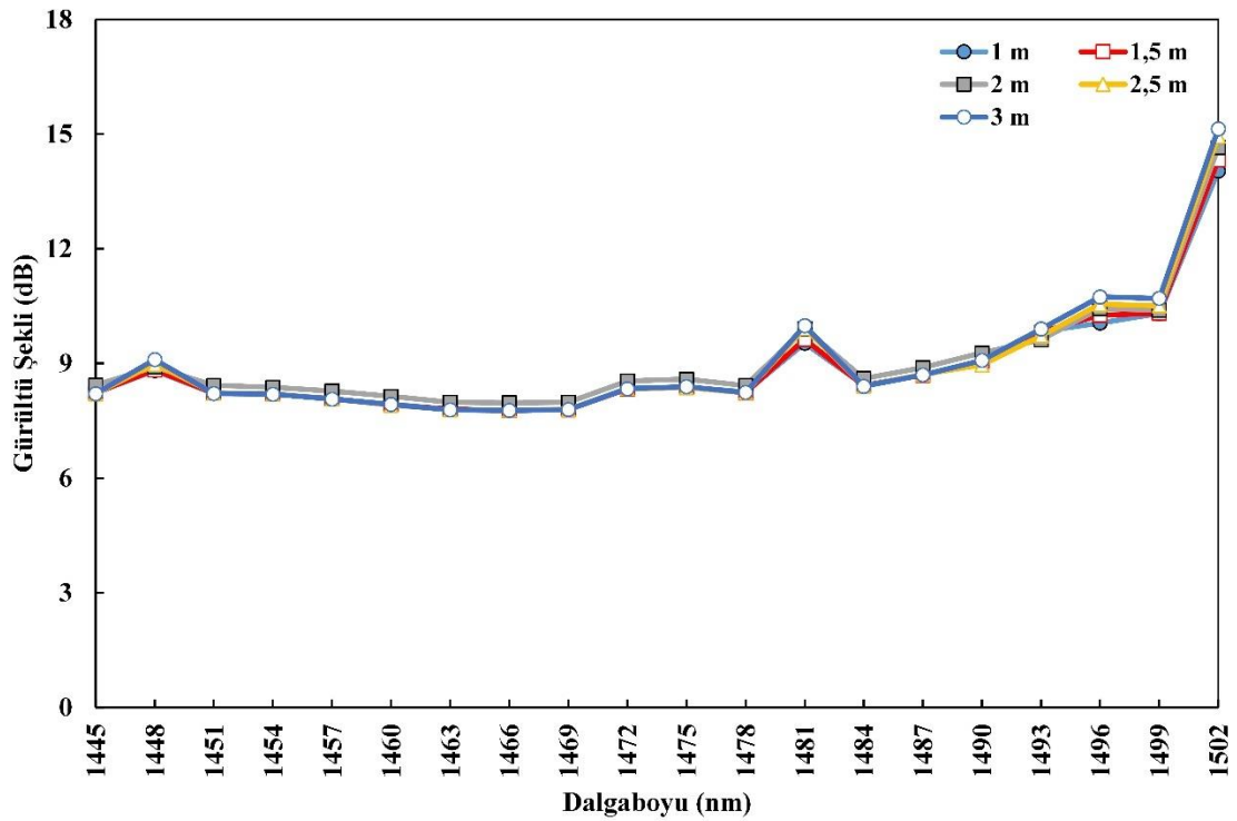
Şekil 6.70. ÜADG-TKFY II için TKF boyu-gürültü şekli değişimi
