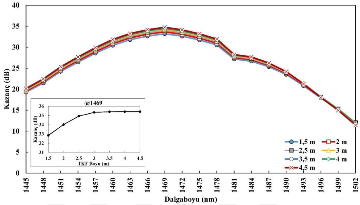
Şekil 6.36. İAÜG-TKFY II için TKF boyu-kazanç değişimi
