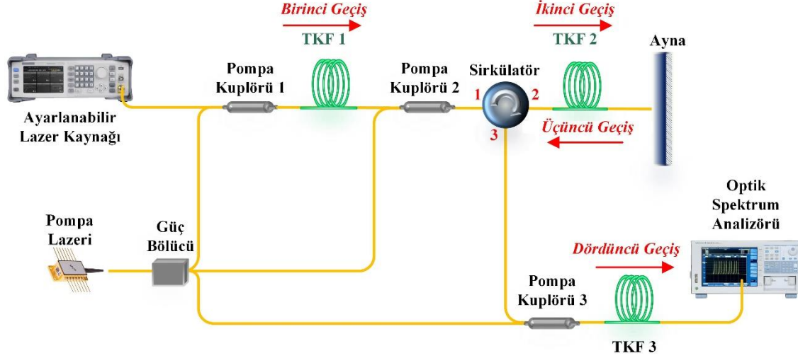
Şekil 6.64. Üç aşama dört geçişli TKFY II
