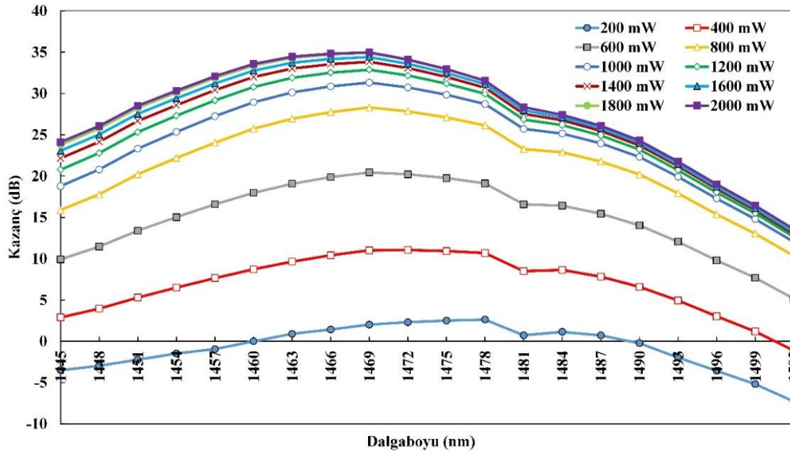
Şekil 6.75. ÜADG-TKFY III için pompa gücü-kazanç değişimi
