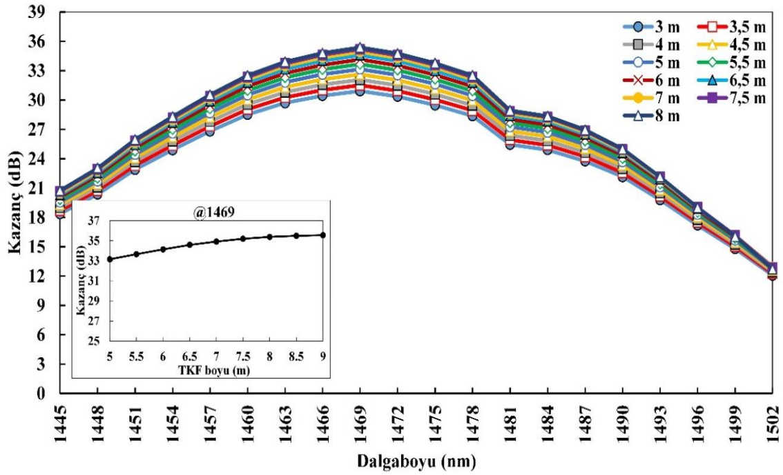
Şekil 6.44. ÜAÜG-TKFY için TKF 2 boyu-kazanç değişimi
