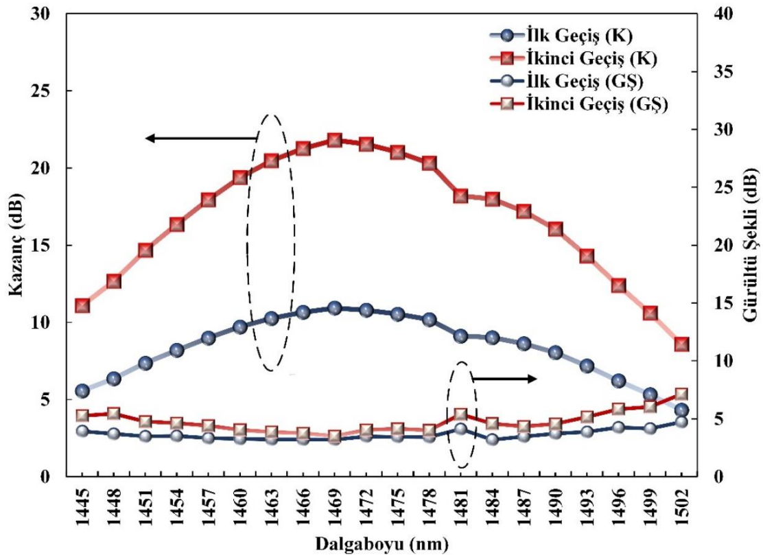
Şekil 6.12. ÇG-TKFY konfigürasyonunun her iki geçişinde elde edilen kazanç ve gürültü şekli değişimi
