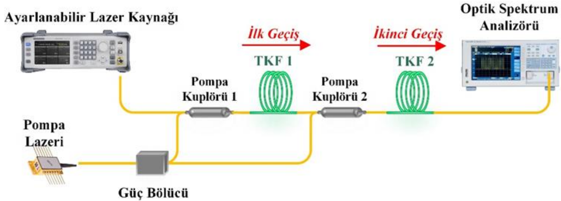
Şekil 6.13. İki Aşamalı Çift Geçişli TKFY
