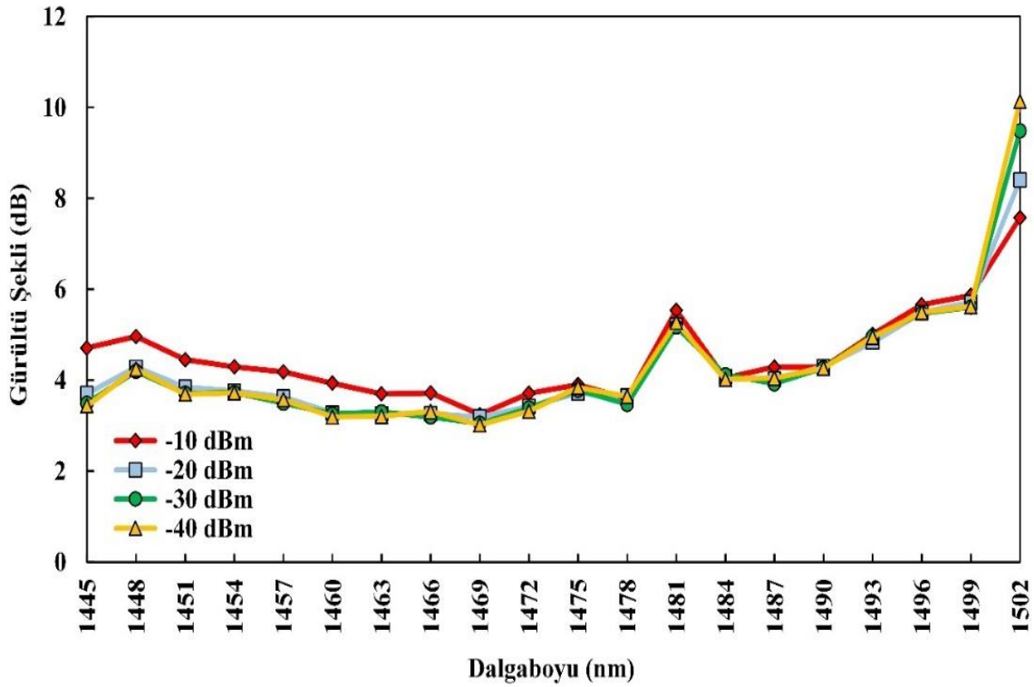
Şekil 6.50. İADG-TKFY için giriş gücü-gürültü şekli değişimi
