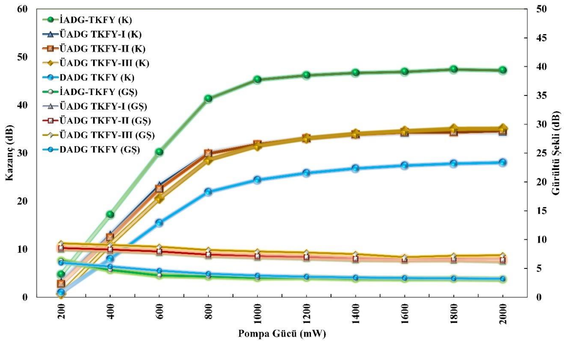
Şekil 6.88. İADG-TKFY, ÜADG-TKFY I, ÜADG-TKFY II, ÜADG-TKFY III ve DADG-TKFY tasarımlarının kazanç ve gürültü şekli karşılaştırması
