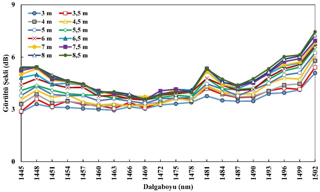
Şekil 6.11. ÇG-TKFY için TKF boyu-gürültü şekli değişimi
