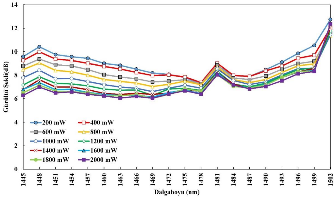
Şekil 6.60. ÜADG-TKFY I için pompa gücü-gürültü şekli değişimi
