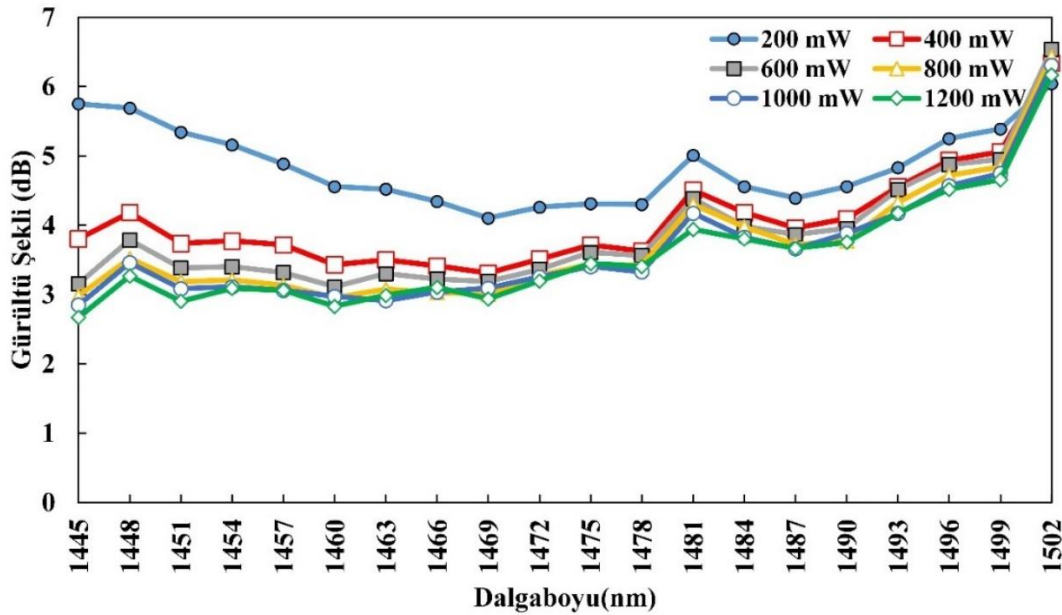
Şekil 6.9. ÇG-TKFY için pompa gücü-gürültü şekli değişimi
