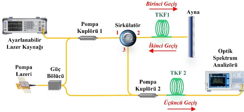
Şekil 6.31. İki aşamalı üç geçişli TKFY II
