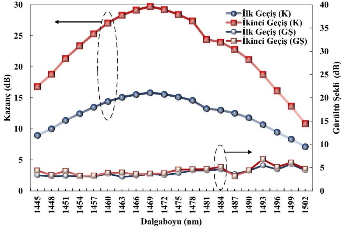
Şekil 6.21. İAÇG-TKFY konfigürasyonunun her iki geçişinde elde edilen kazanç ve gürültü şekli değişimi
