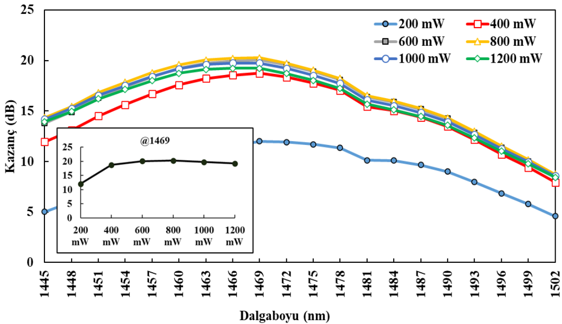
Şekil 6.8. ÇG-TKFY için pompa gücü-kazanç değişimi
