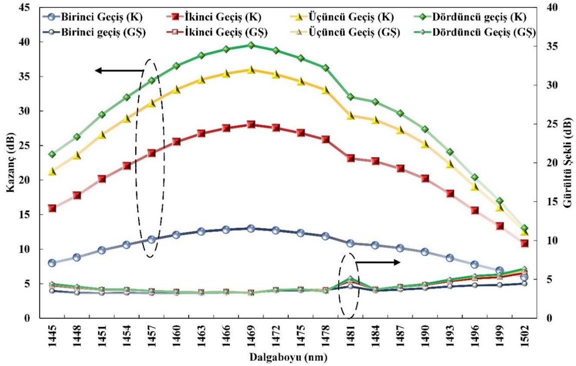
Şekil 6.87. DADG-TKFY konfigürasyonunun her iki geçişinde elde edilen kazanç ve gürültü şekli değişimi
