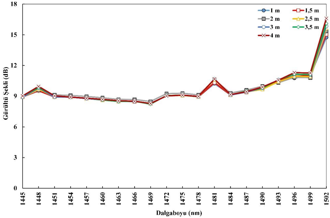
Şekil 6.78. Üç aşamalı dört geçişli TKFY III için TKF boyu-gürültü şekli değişimi
