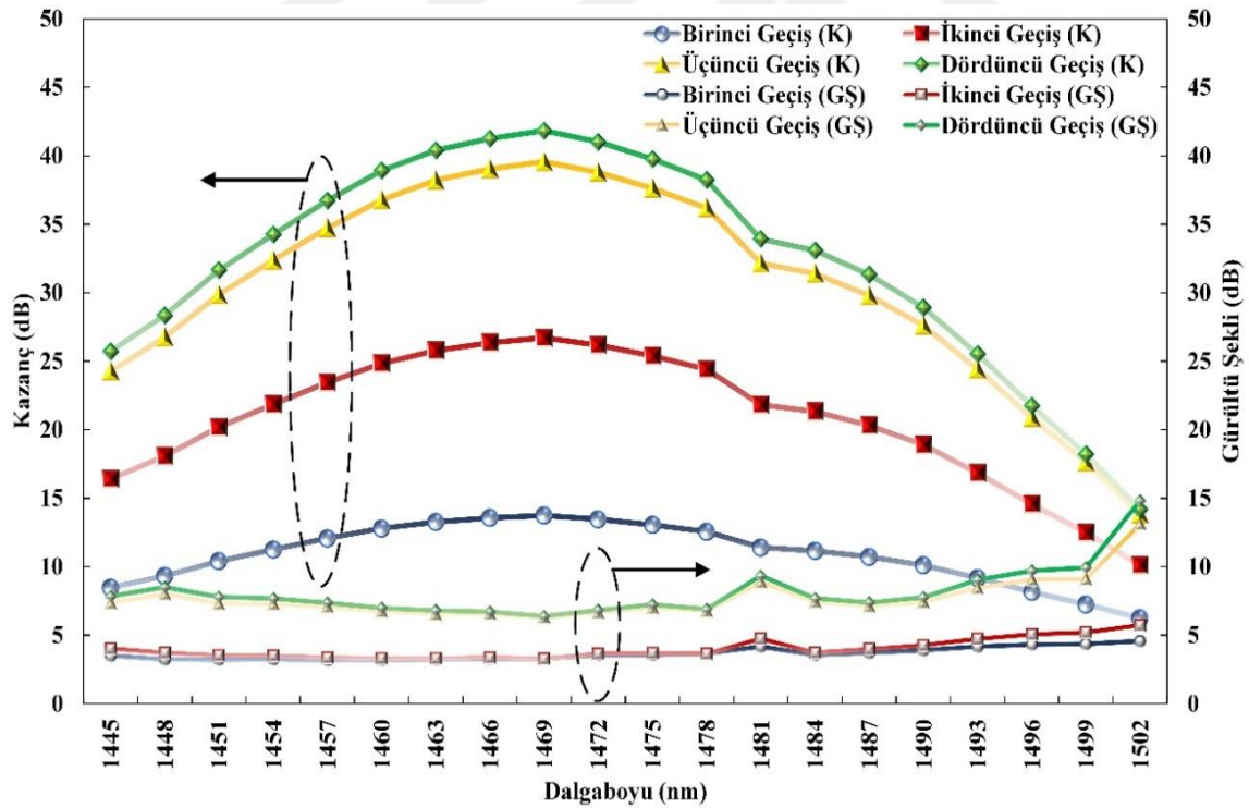
Şekil 6.71. ÜADG-TKFY III konfigürasyonunun her dört geçişinde elde edilen kazanç ve gürültü şekli değişimi
