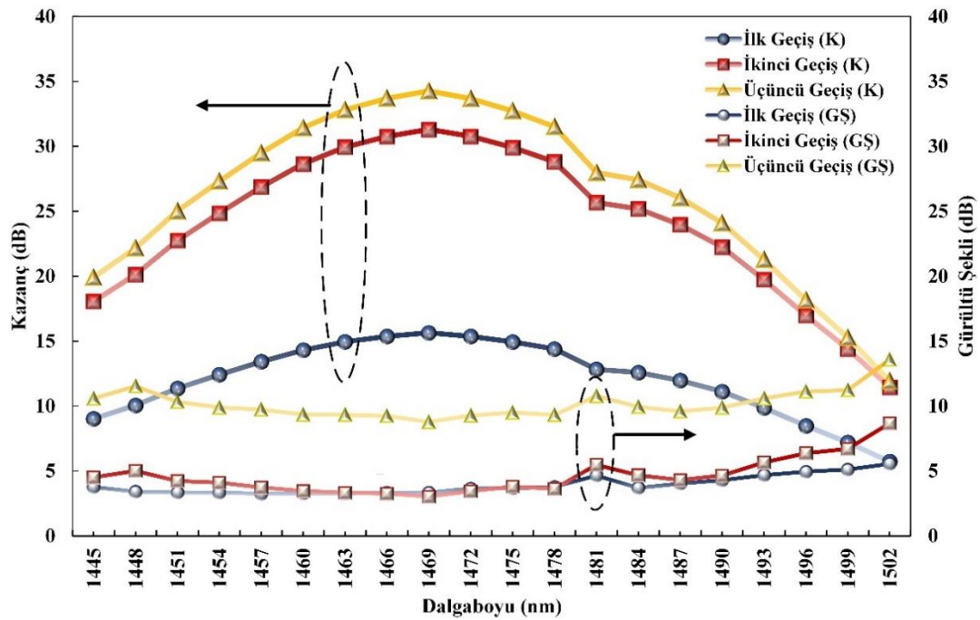
Şekil 6.38. İAÜG-TKFY II konfigürasyonunun her üç geçişinde elde edilen kazanç ve gürültü şekli değişimi
