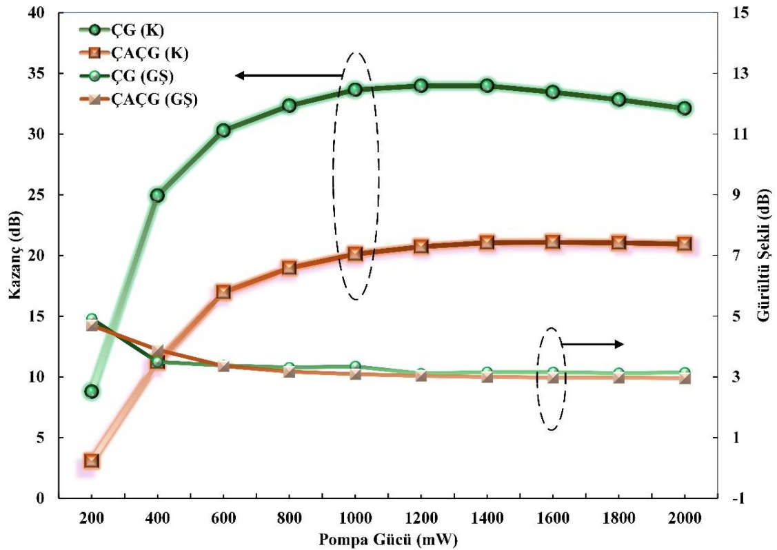
Şekil 6.22. ÇG-TKFY ve İAÇG-TKFY tasarımlarının kazanç ve gürültü şekli karşılaştırması
