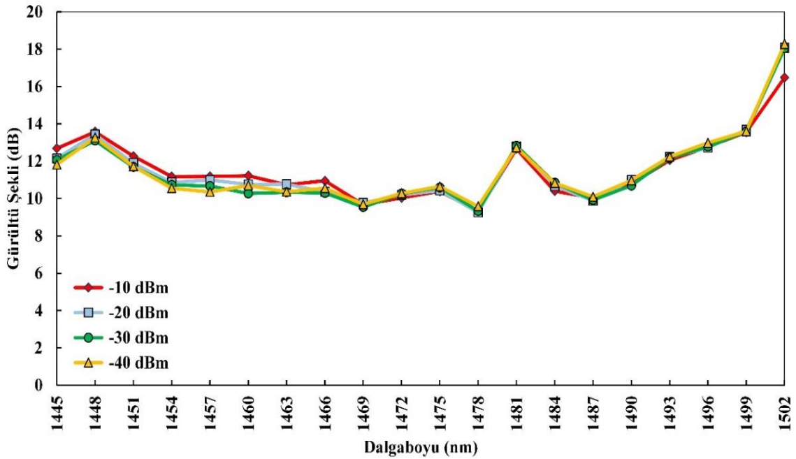
Şekil 6.66. ÜADG-TKFY II için giriş gücü-gürültü şekli değişimi
