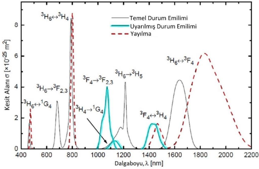
Şekil 4.2. Tulyum'un soğurma ve yayılma spektrumu
