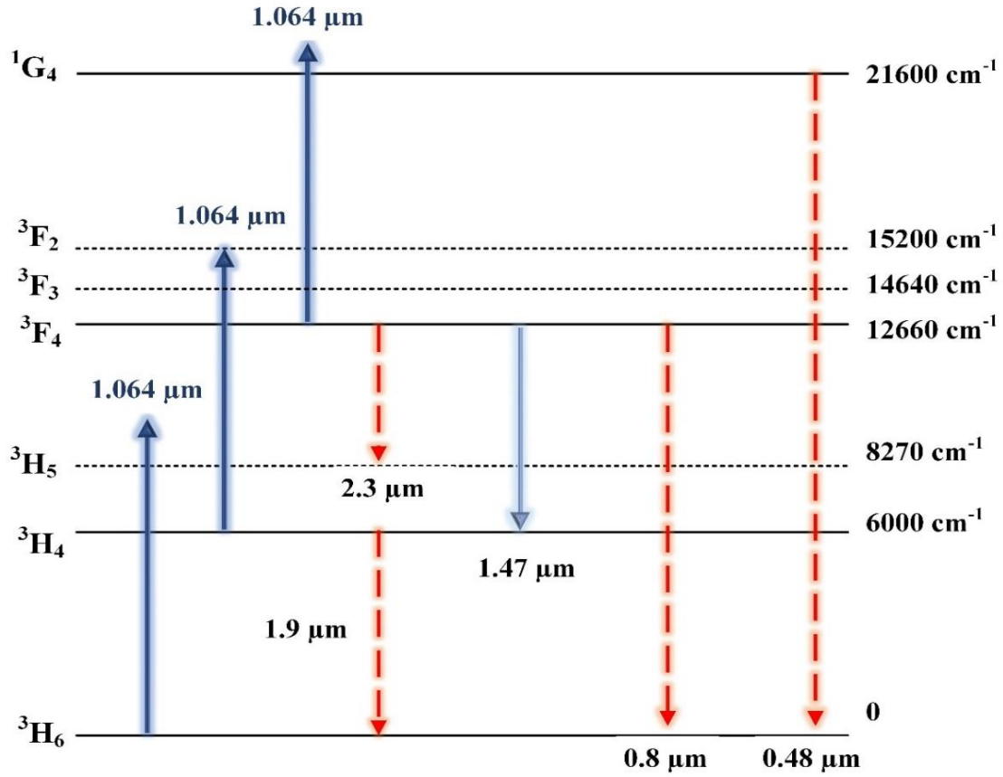
Şekil 4.4. Florit camdaki Tulyum iyonlarının enerji diyagramı
