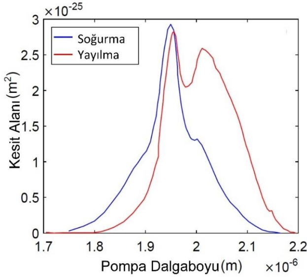
Şekil 3.6. \text{Ho}^{3+} 'un pompa soğurma ve yayılma spektrumları
