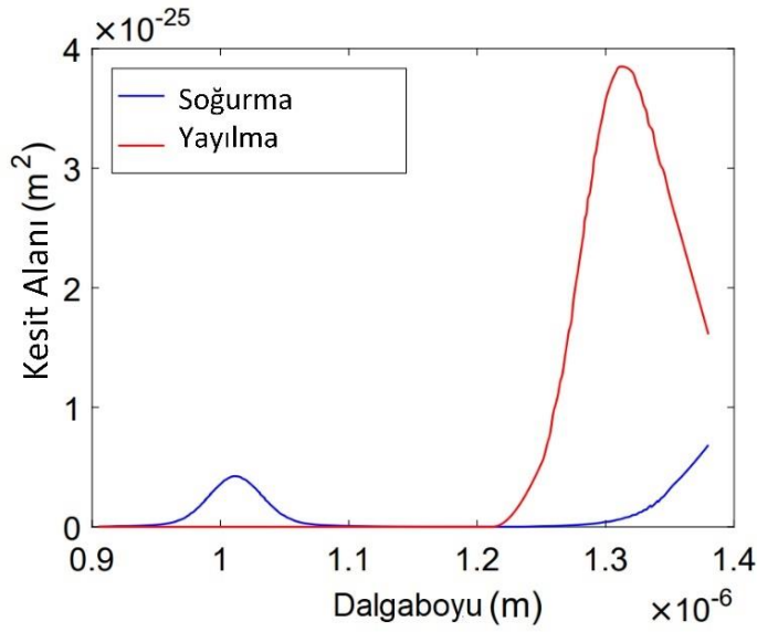
řekil 3.8. \text{Pr}^{3+} ’un soęurma ve yayılma spektrumu
