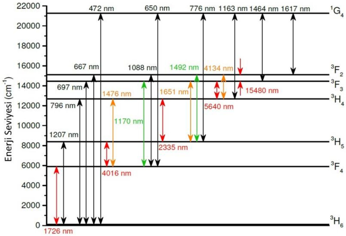
Şekil 4.1. Geçiş dalgaboylarının yer aldığı Tulyum'un enerji seviye diyagramı
