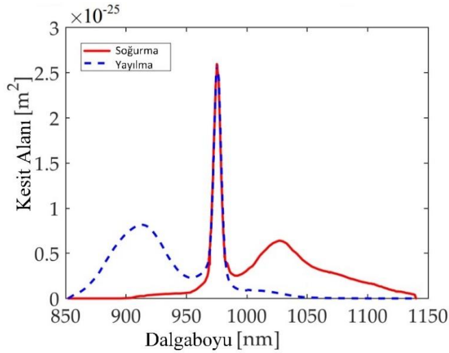
Şekil 3.7. Yb +3 'un soğurma ve yayılma spektrumu
