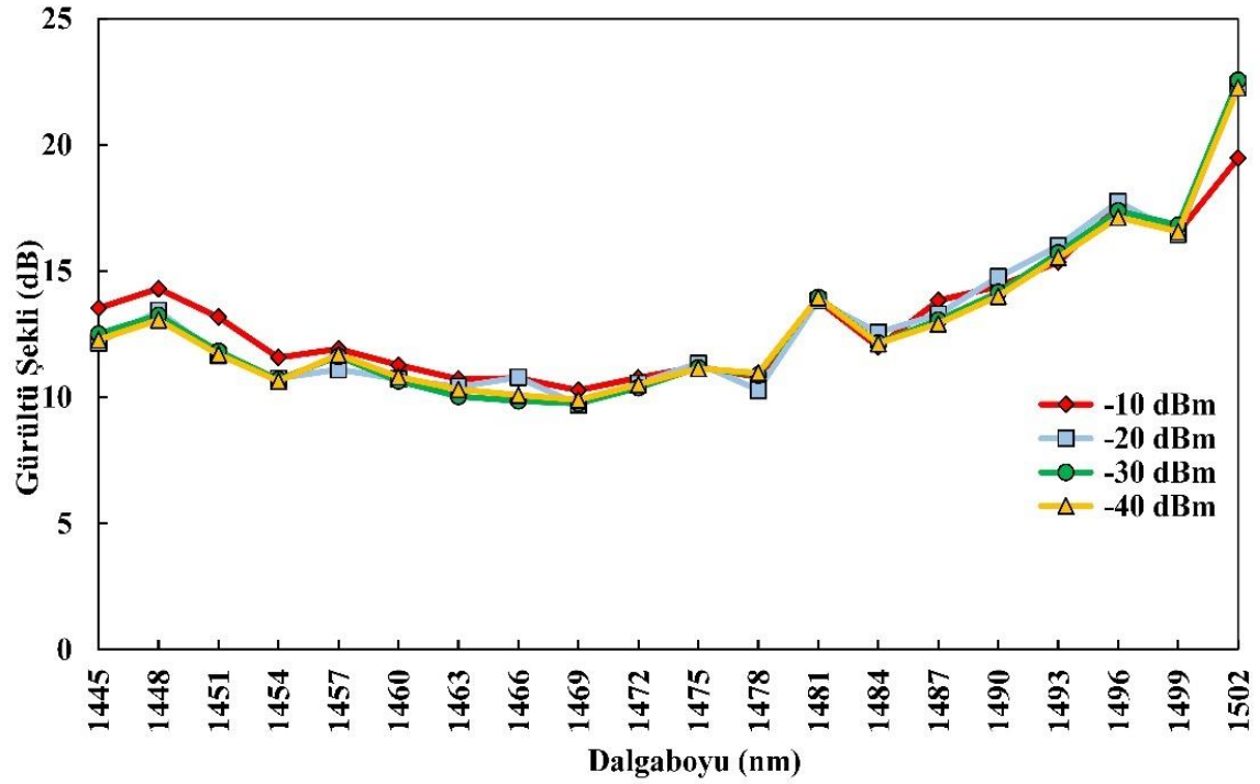
Şekil 6.33. İAÜG-TKFY II için giriş gücü-gürültü şekli değişimi
