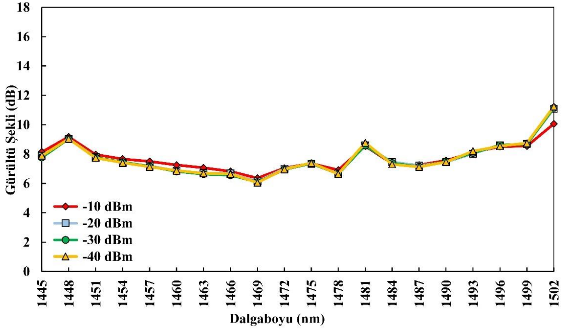
Şekil 6.58. ÜADG-TKFY I için giriş gücü-gürültü şekli değişimi
