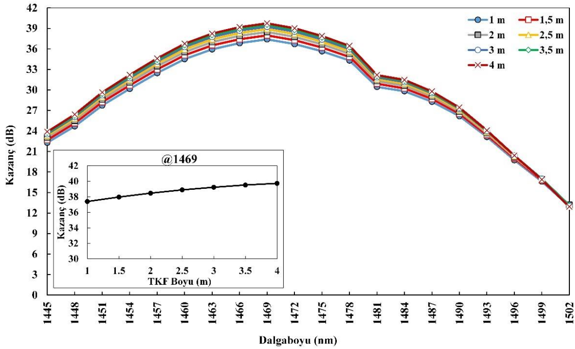
Şekil 6.85. DADG-TKFY için giriş gücü-kazanç değişimi
