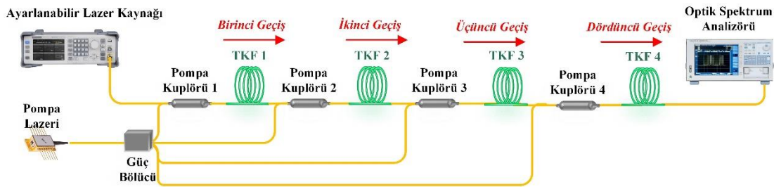
Şekil 6.80. Dört aşamalı dört geçişli TKFY
