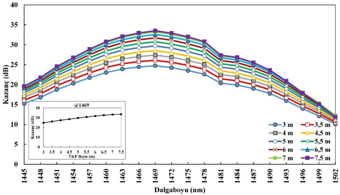
Şekil 6.28. İAÜG-TKFY I için TKF 2 boyu-kazanç değişimi
