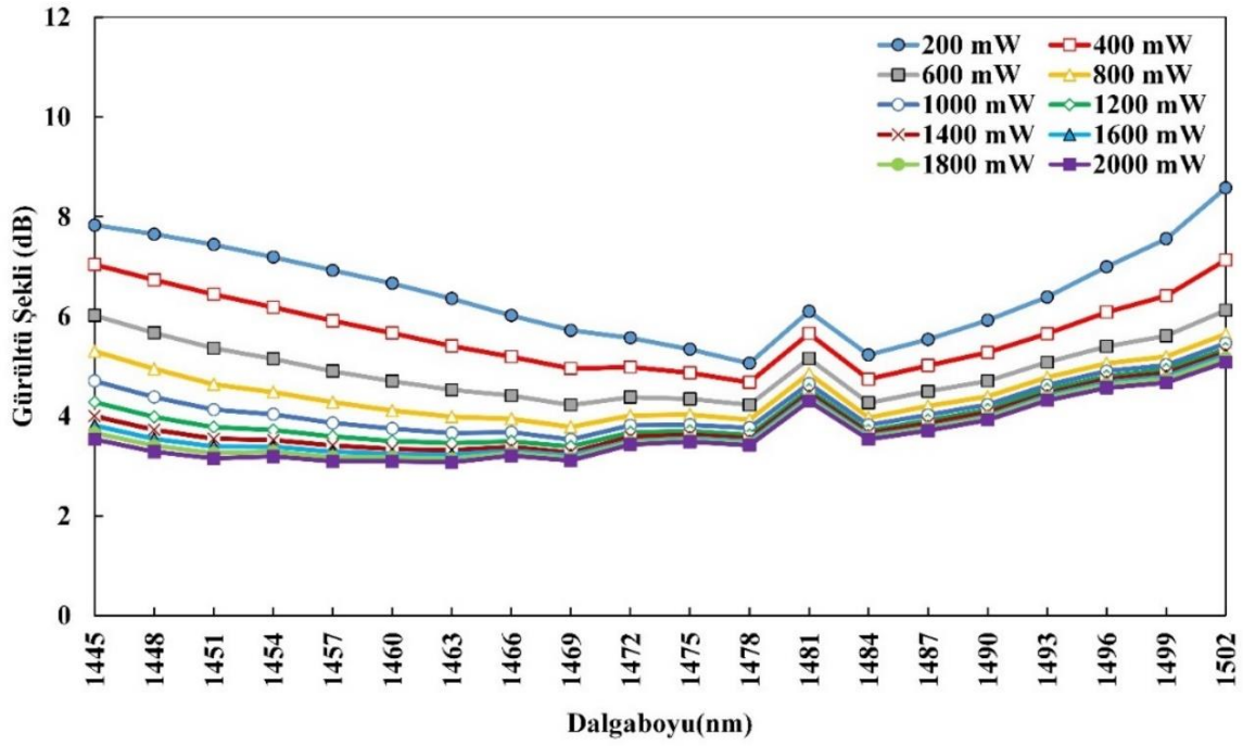
Şekil 6.43. ÜAÜG-TKFY için pompa gücü-gürültü şekli değişimi
