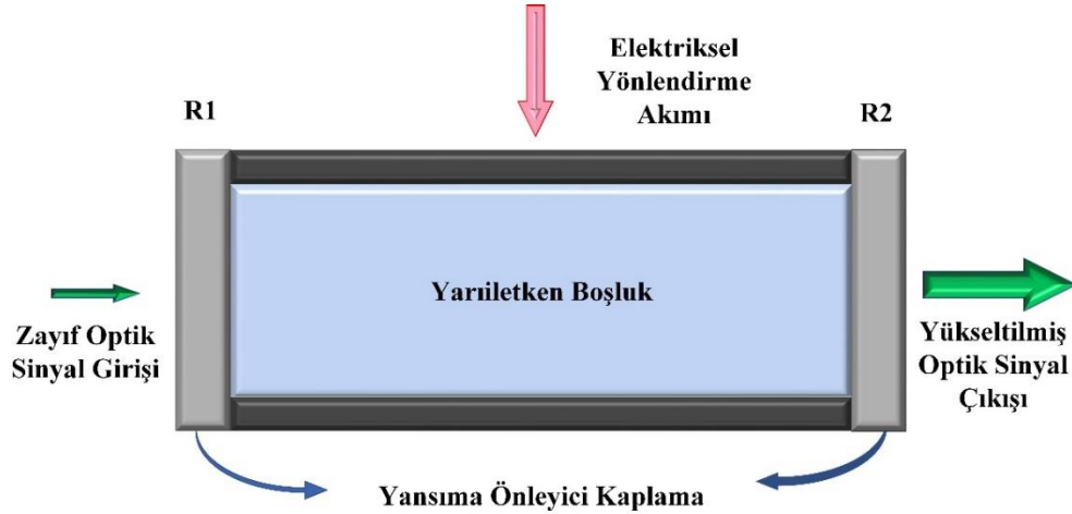
Şekil 3.2. Temel yarıiletken yükselteç şeması [84]
