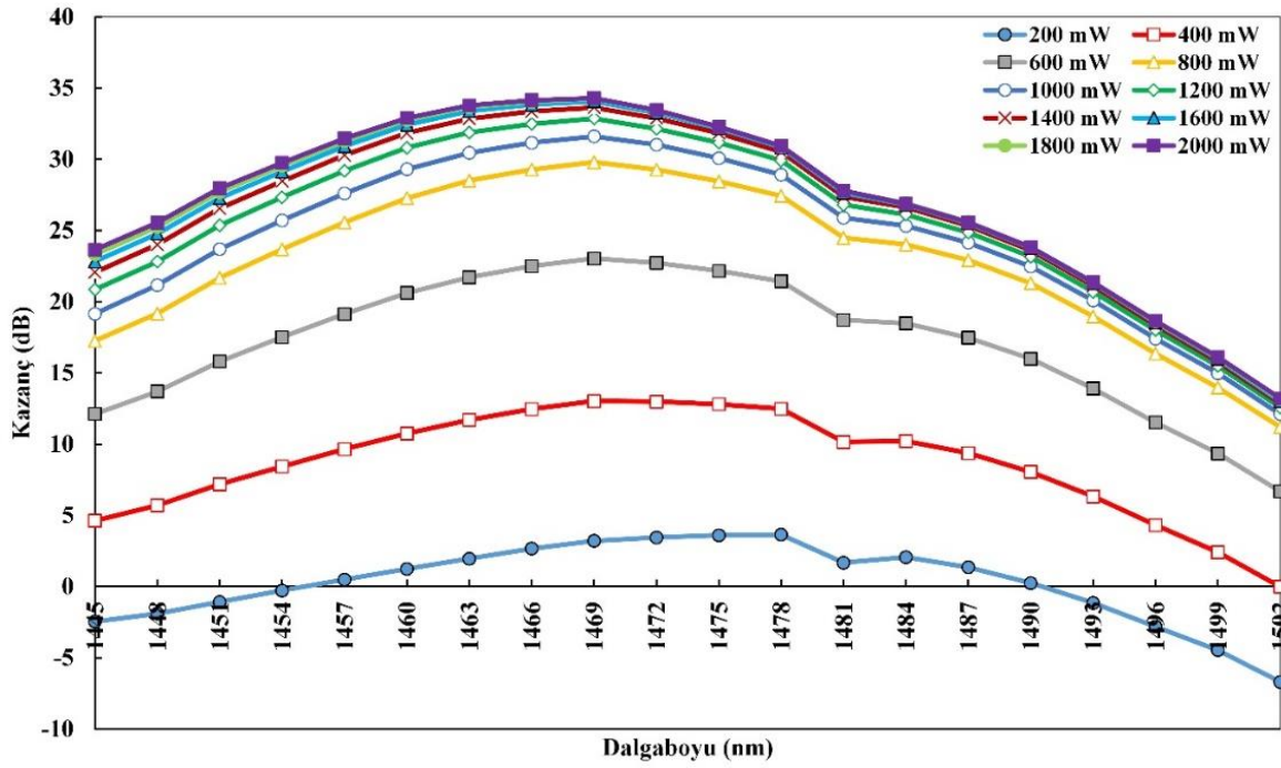
Şekil 6.59. ÜADG-TKFY I için pompa gücü-kazanç değişimi
