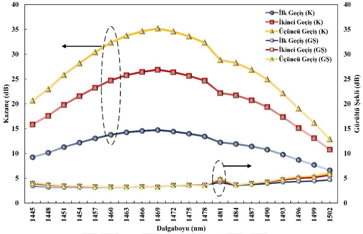
Şekil 6.46. ÜAÜG-TKFY konfigürasyonunun her iki geçişinde elde edilen kazanç ve gürültü şekli değişimi
