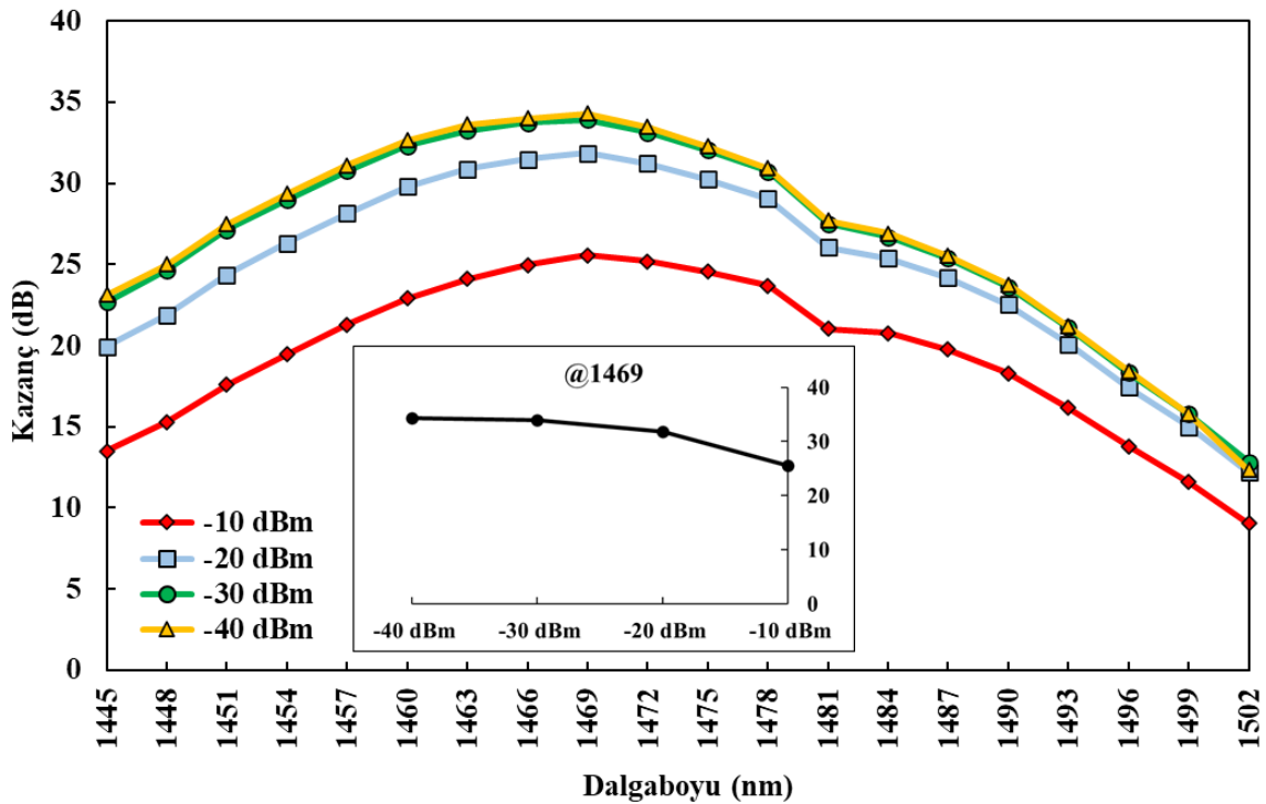
Şekil 6.49. İADG-TKFY için giriş gücü-kazanç değişimi
