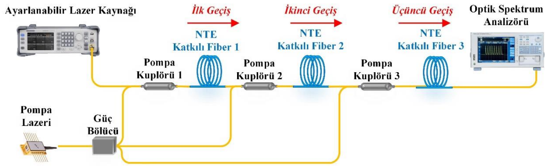
Şekil 5.6. Üç aşamalı üç geçişli yükselteç konfigürasyonu
