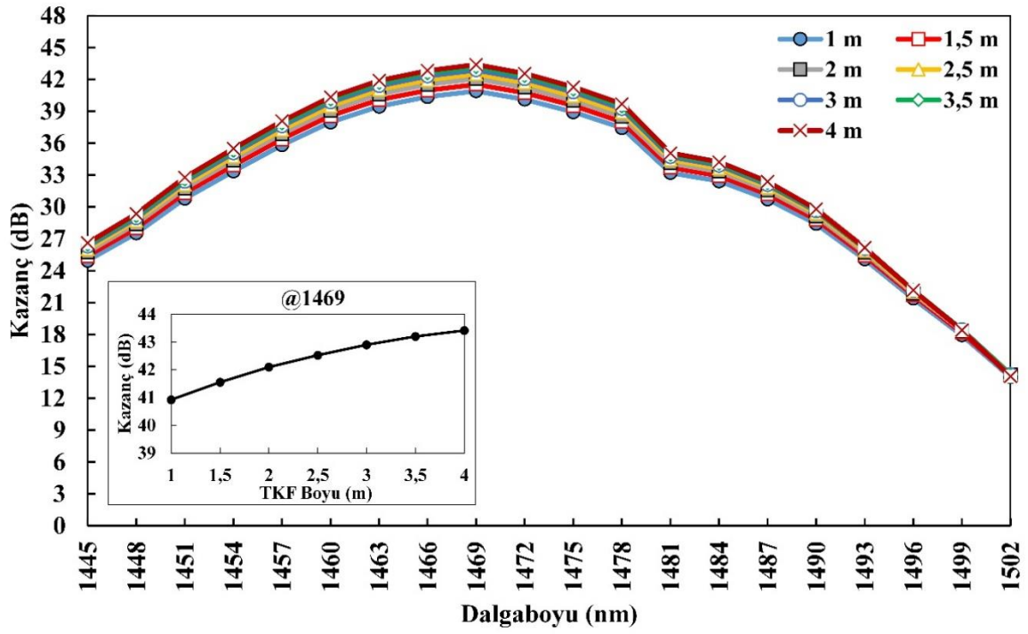
Şekil 6.77. Üç aşamalı dört geçişli TKFY III için TKF boyu-kazanç değişimi
