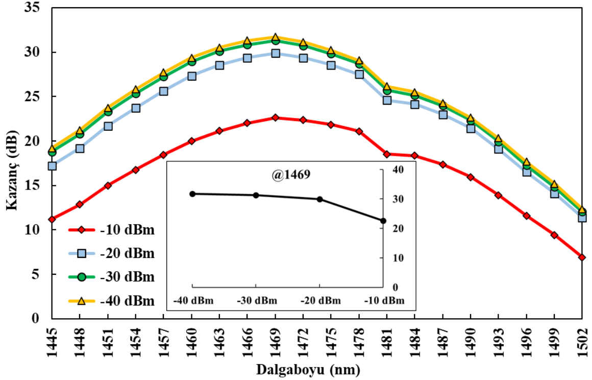
Şekil 6.73. ÜADG-TKFY III için giriş gücü-kazanç değişimi
