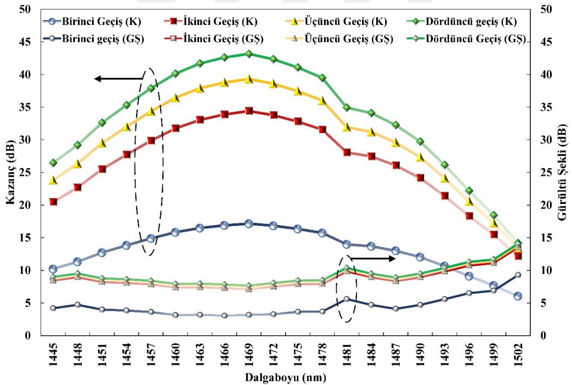
Şekil 6.79. ÜADG-TKFY III konfigürasyonunun her dört geçişinde elde edilen kazanç ve gürültü şekli değişimi
