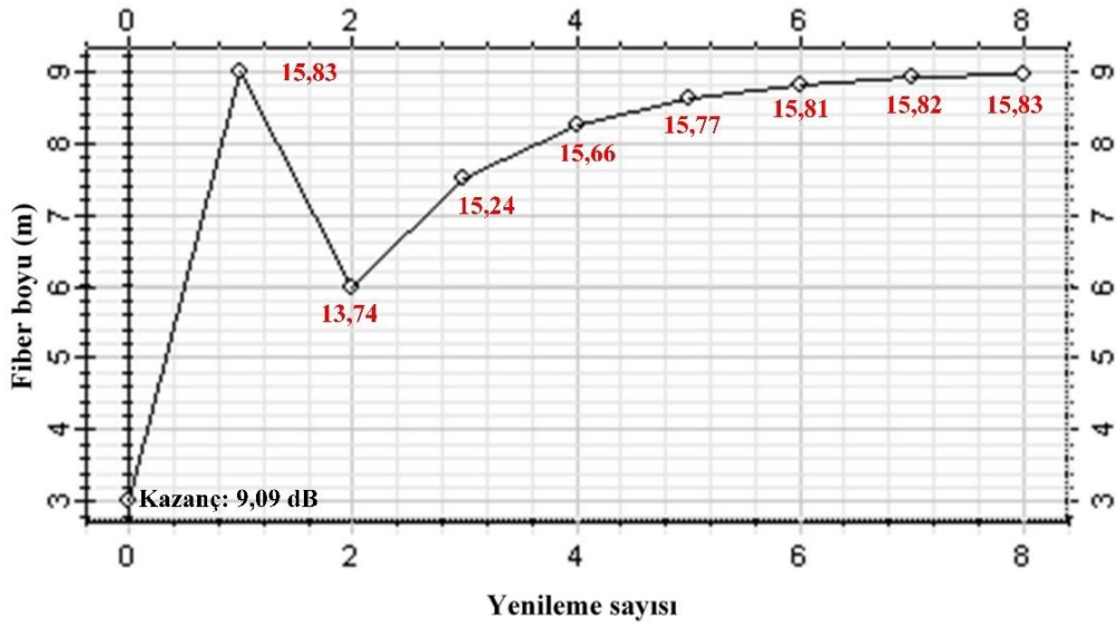
Şekil 6.18. TKF 1 boyu optimizasyonu
