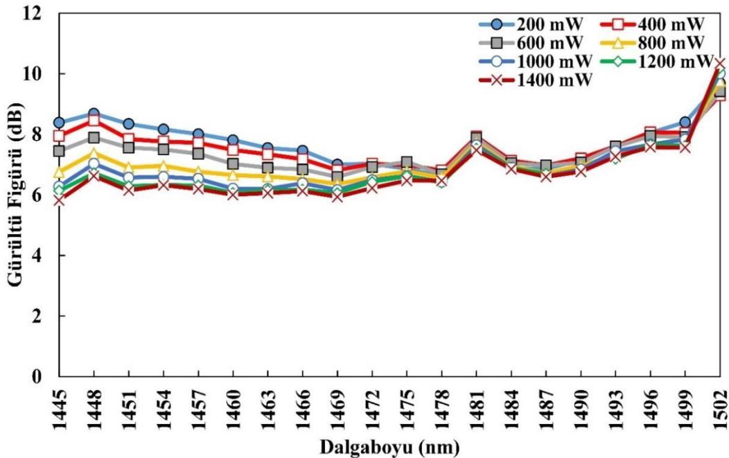
Şekil 6.27. İAÜG-TKFY I için pompa gücü- gürültü şekli değişimi
