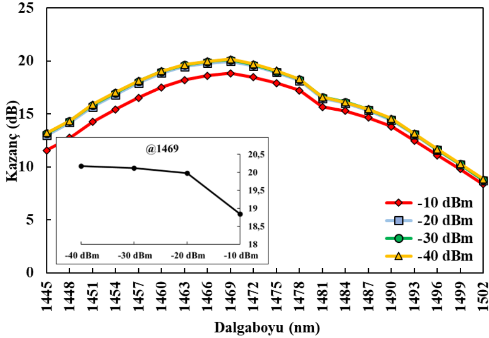
Şekil 6.14. İAÇG-TKFY için Giriş gücü-kazanç değişimi
