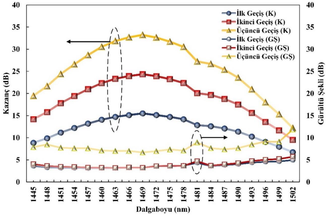
Şekil 6.30. İAÜG-TKFY I konfigürasyonunun her üç geçişinde elde edilen kazanç ve gürültü şekli değişimi
