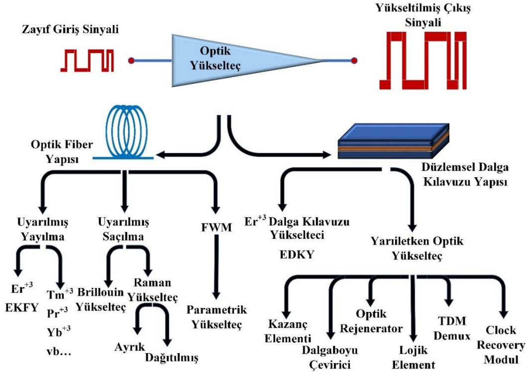
Şekil 3.1. Optik Yükselteç Türleri [82]
