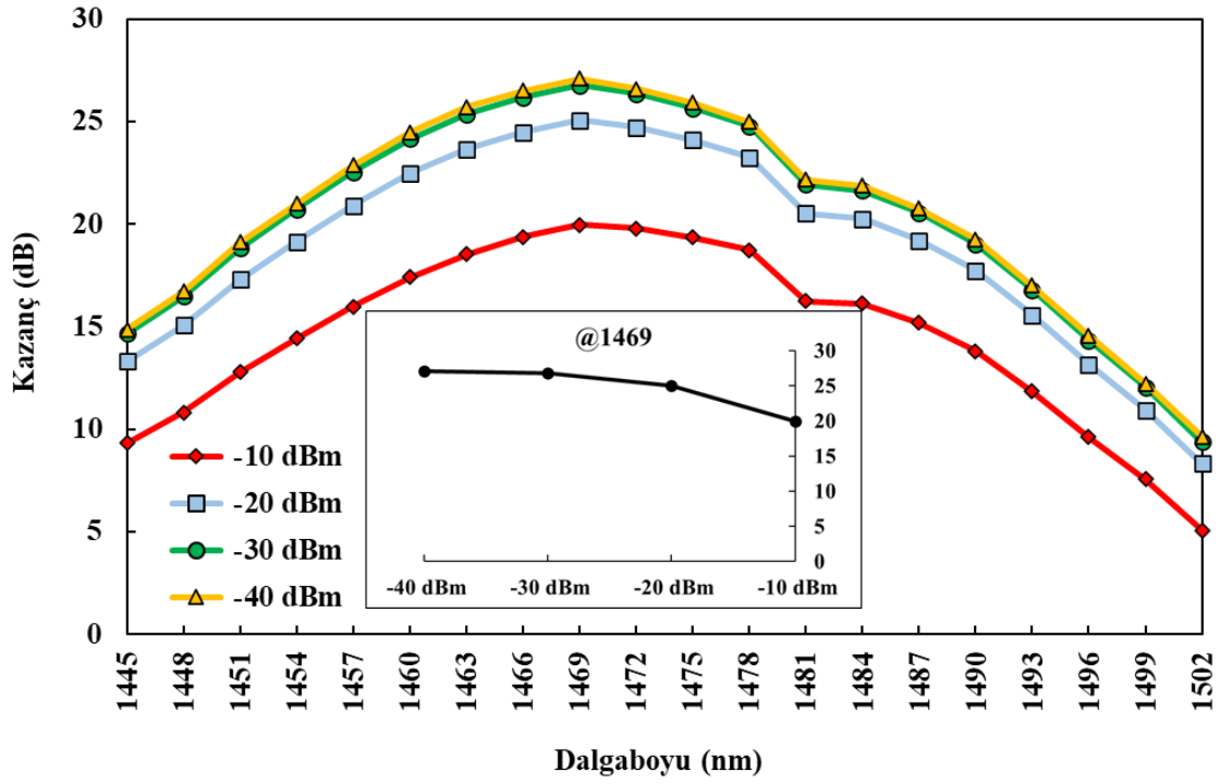
Şekil 6.81. DADG-TKFY için giriş gücü-kazanç değişimi
