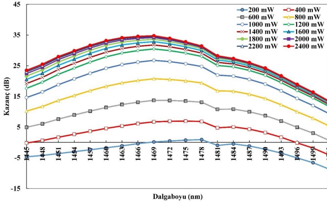
Şekil 6.83. DADG-TKFY için giriş gücü-kazanç değişimi
