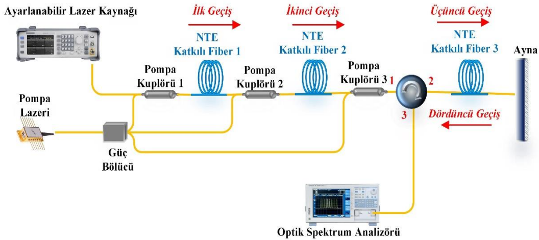
Şekil 5.8. Üç aşamalı dört geçişli yükselteç konfigürasyonu I
