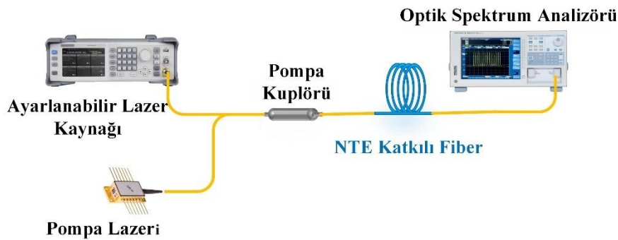
Şekil 5.1. Tek geçişli yükselteç konfigürasyonu
