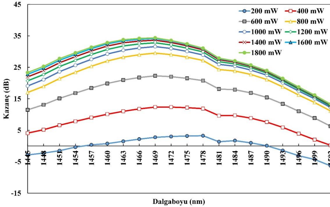
Şekil 6.67. ÜADG-TKFY II için pompa gücü-kazanç değişimi
