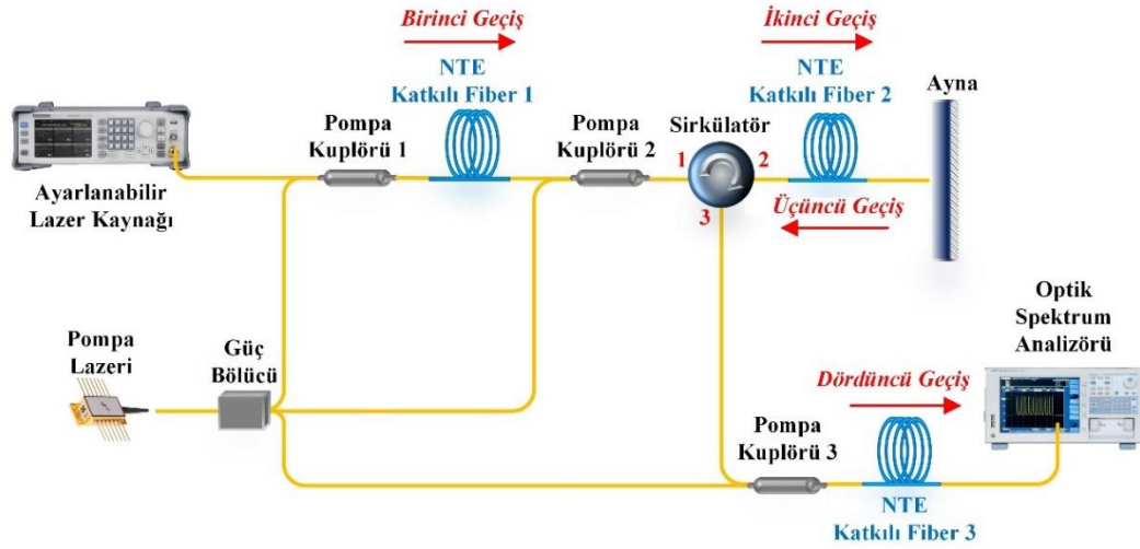
Şekil 5.9. Üç aşamalı dört geçişli yükselteç konfigürasyonu II
