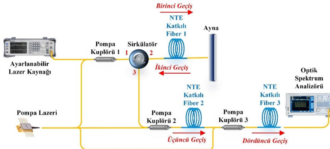
Şekil 5.10. Üç aşamalı dört geçişli yükselteç konfigürasyonu III
