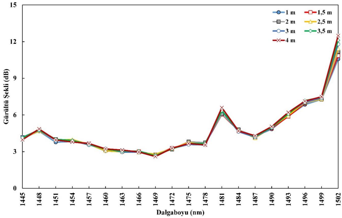
Şekil 6.54. İADG-TKFY için TKF boyu-gürültü şekli değişimi
