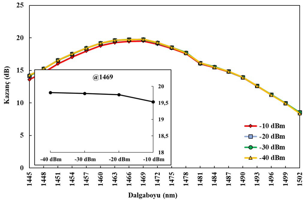
Şekil 6.6. ÇG-TKFY için giriş gücü-kazanç değişimi
