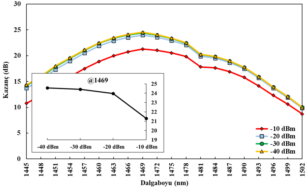
Şekil 6.40. ÜAÜG-TKFY için giriş gücü-kazanç değişimi
