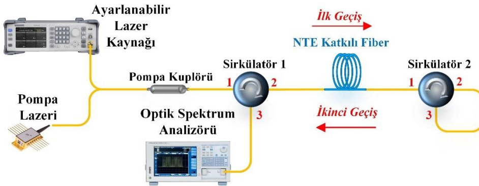
(b) Ayna ile yönlendirme yapılan konfigürasyon
