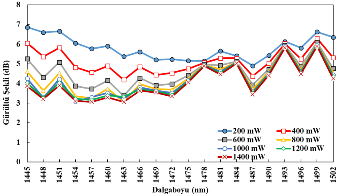
Şekil 6.17. İAÇG-TKFY için pompa gücü-gürültü şekli değişimi
