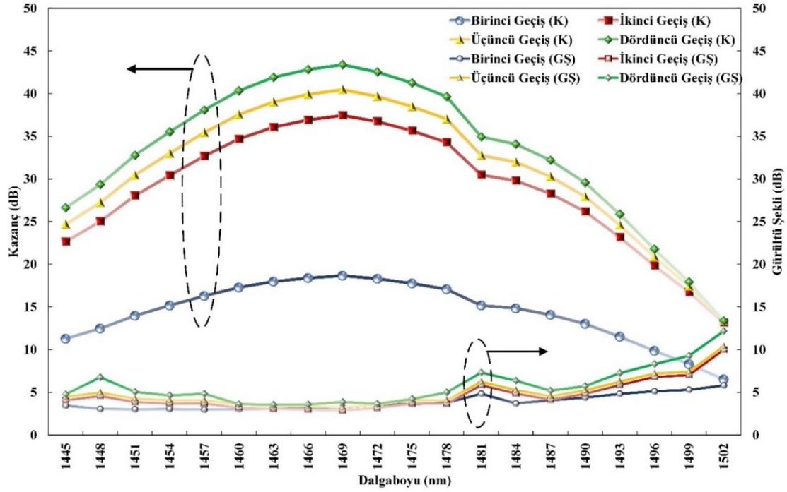
Şekil 6.55. İADG-TKFY konfigürasyonunun her dört geçişinde elde edilen kazanç ve gürültü şekli değişimi
