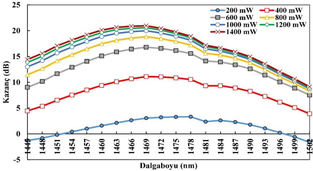
Şekil 6.16. İAÇG-TKfy için pompa gücü-kazanç değişimi
