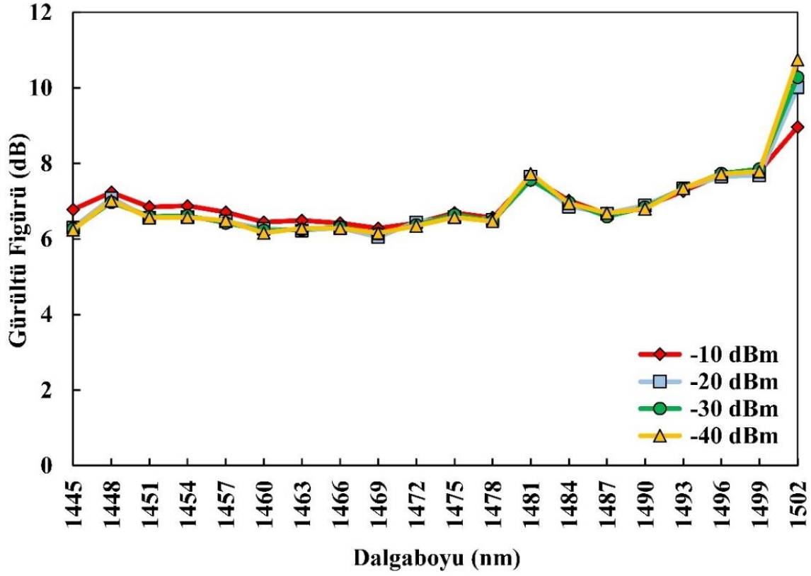
Şekil 6.25. İAÜG-TKFY I için giriş gücü-gürültü şekli değişimi
