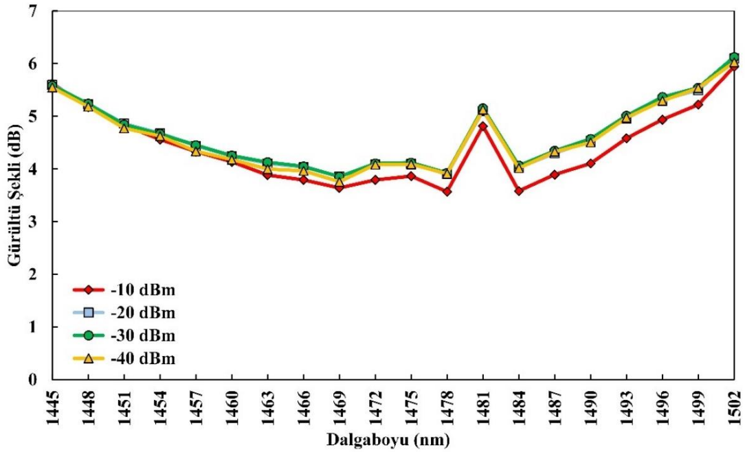
Şekil 6.82. DADG-TKFY için giriş gücü-gürültü şekli değişimi
