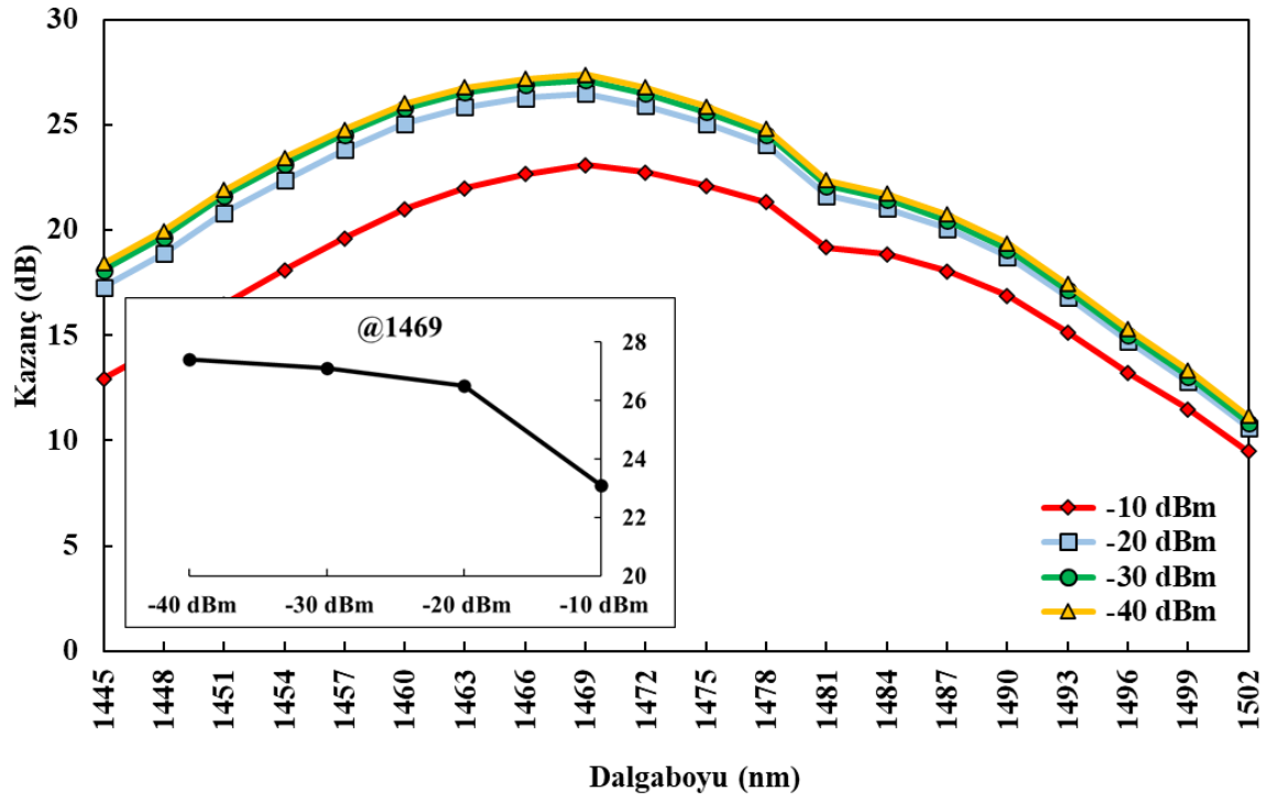
Şekil 6.32. İAÜG-TKFY II için giriş gücü-kazanç değişimi
