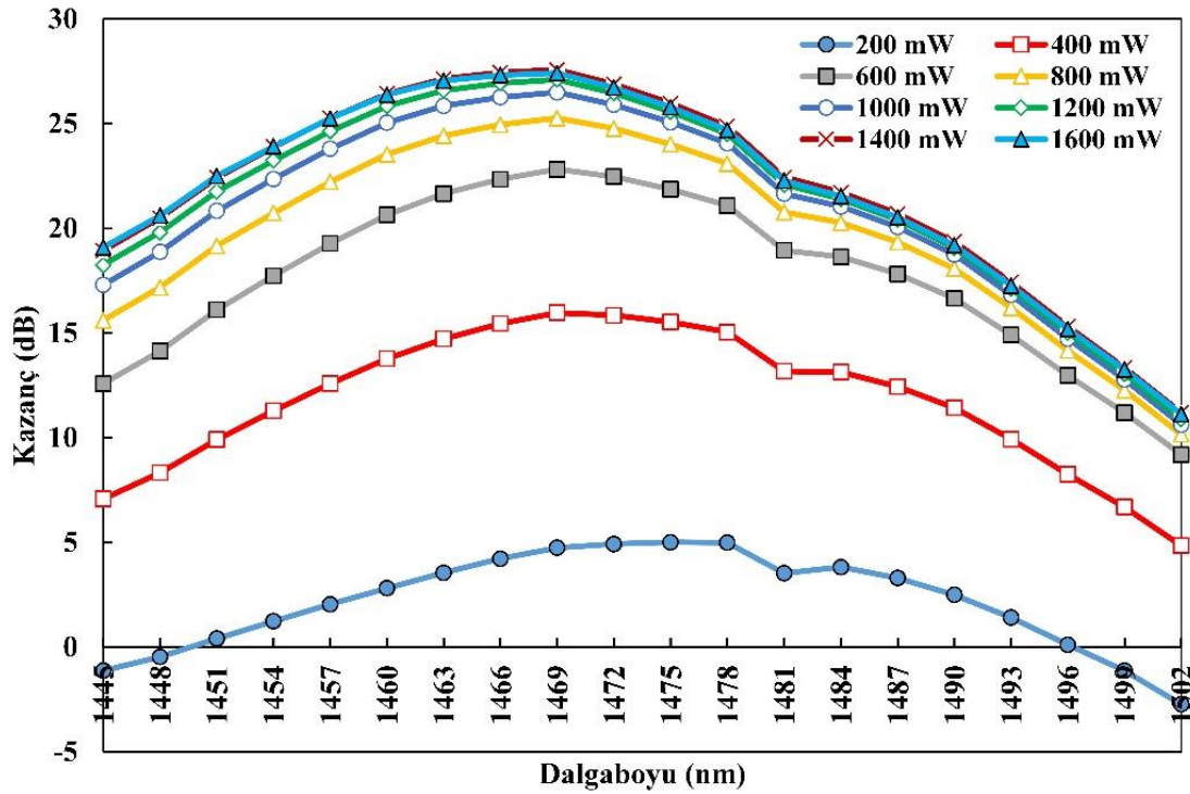
Şekil 6.34. İAÜG-TKFY II için pompa gücü-kazanç değişim grafiği
