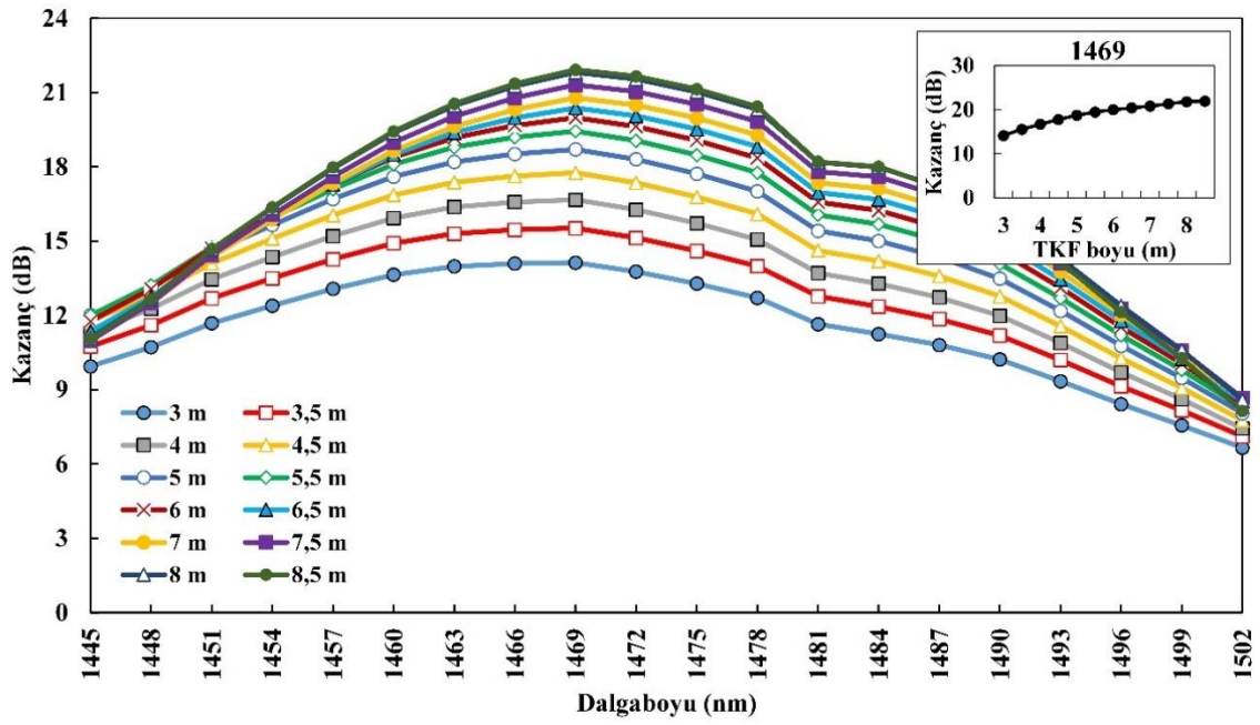
Şekil 6.10. ÇG-TKFY için TKF boyu-kazanç değişimi
