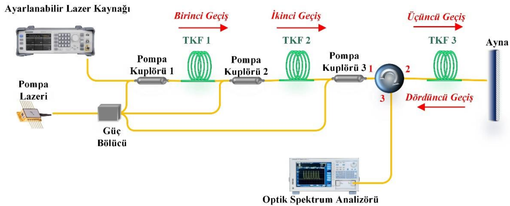
Şekil 6.56. Üç aşamalı dört geçişli TKFY I
