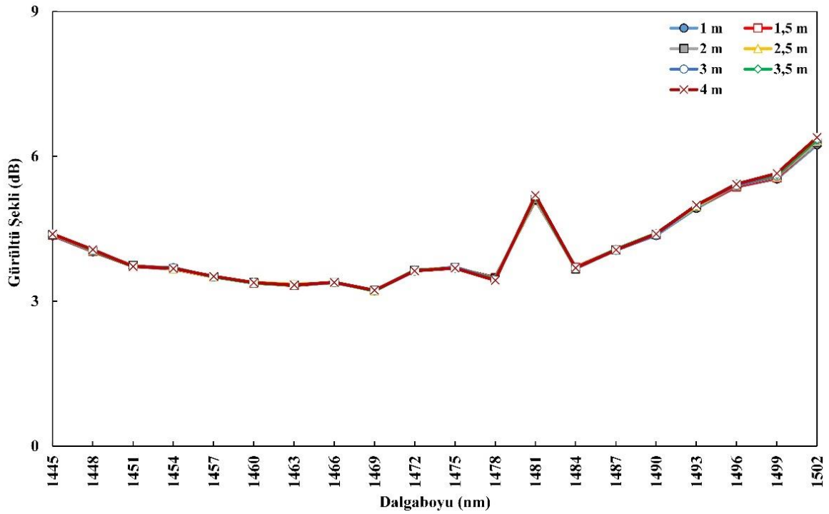
Şekil 6.86. DADG-TKFY için giriş gücü-gürültü şekli değişimi
