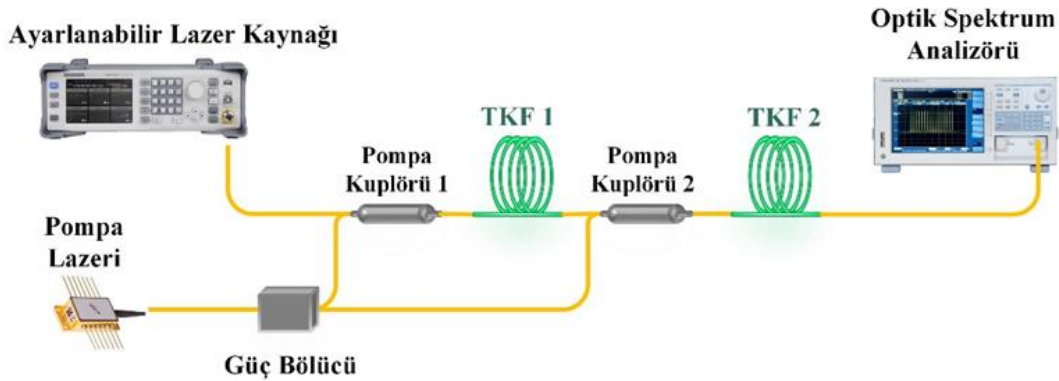
(b) İleri-İleri Yönlü Çift Geçişli TKFY (İİÇG-TKFY)
