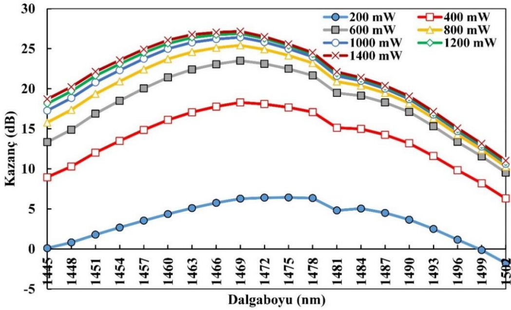
Şekil 6.26. İAÜG-TKFY I için pompa gücü-kazanç değişimi
