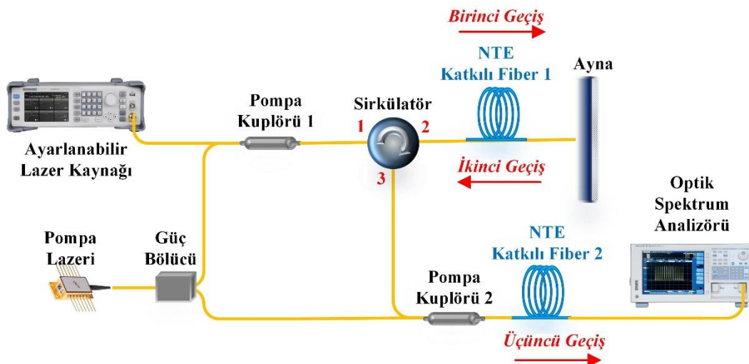
Şekil 5.5. İki aşamalı üç geçişli yükselteç konfigürasyonu II
