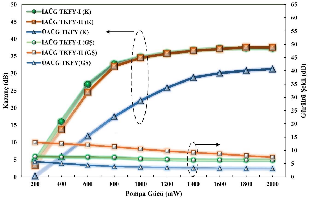
Şekil 6.47. İAÜG-TKFY I, İAÜG-TKFY II ve ÜAÜG-TKFY tasarımlarının kazanç ve gürültü şekli karşılaştırması
