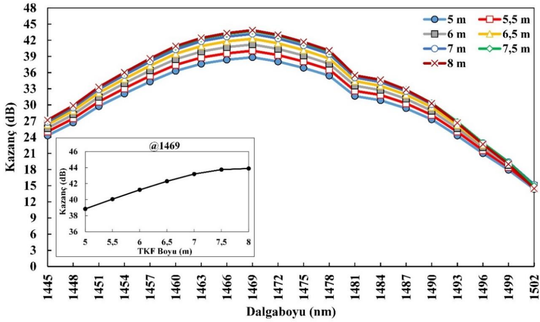
Şekil 6.61. ÜADG-TKFY I için TKF boyu-kazanç değişimi
