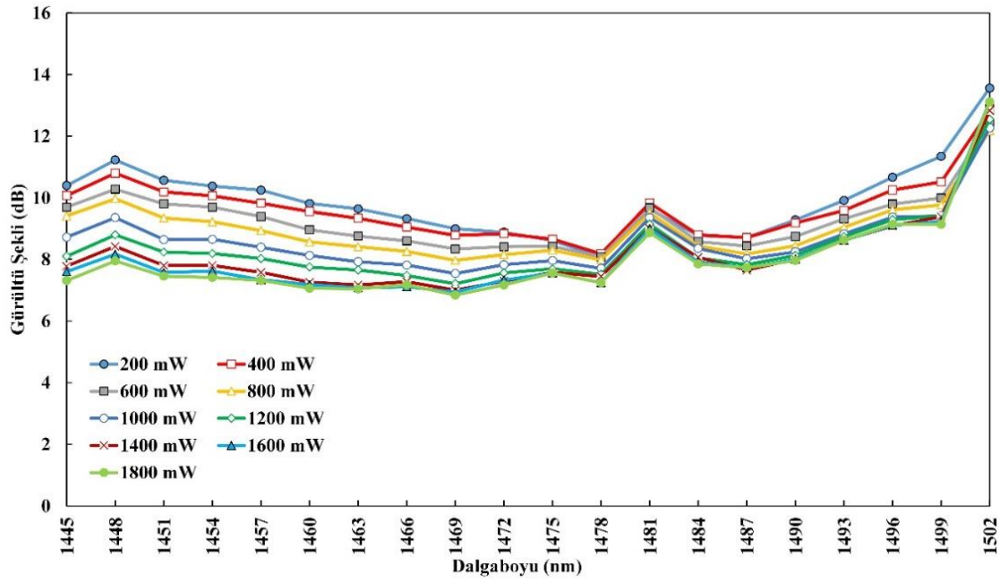
Şekil 6.68. ÜADG-TKFY II için pompa gücü-gürültü şekli değişimi
