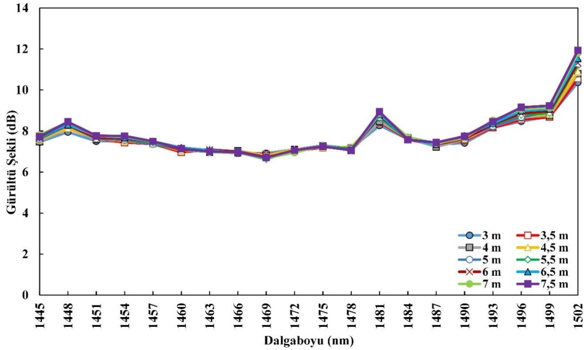
Şekil 6.29. İAÜG-TKFY I için TKF 2 boyu-gürültü şekli değişimi
