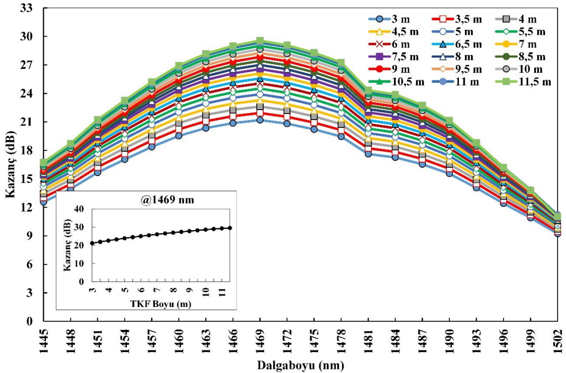
Şekil 6.19. İAÇG-TKFY için TKF 2 boyu-kazanç değişimi
