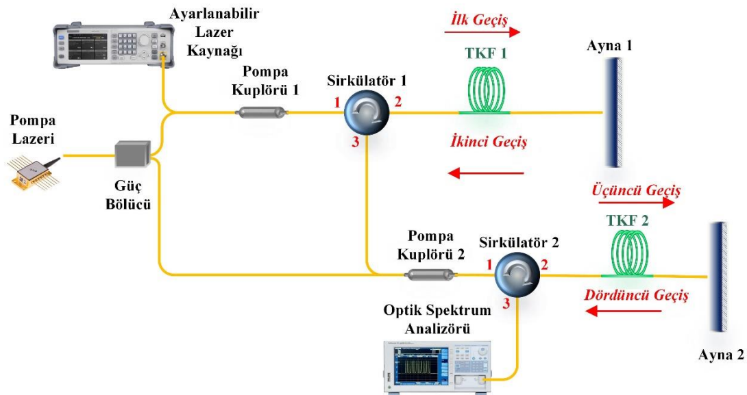
Şekil 6.48. İki aşamalı dört geçişli TKFY
