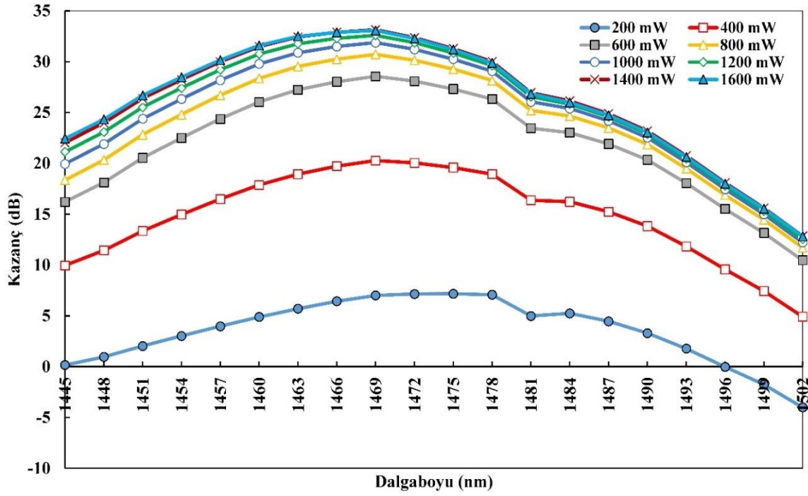
Şekil 6.51. İADG-TKFY için pompa gücü-kazanç değişimi
