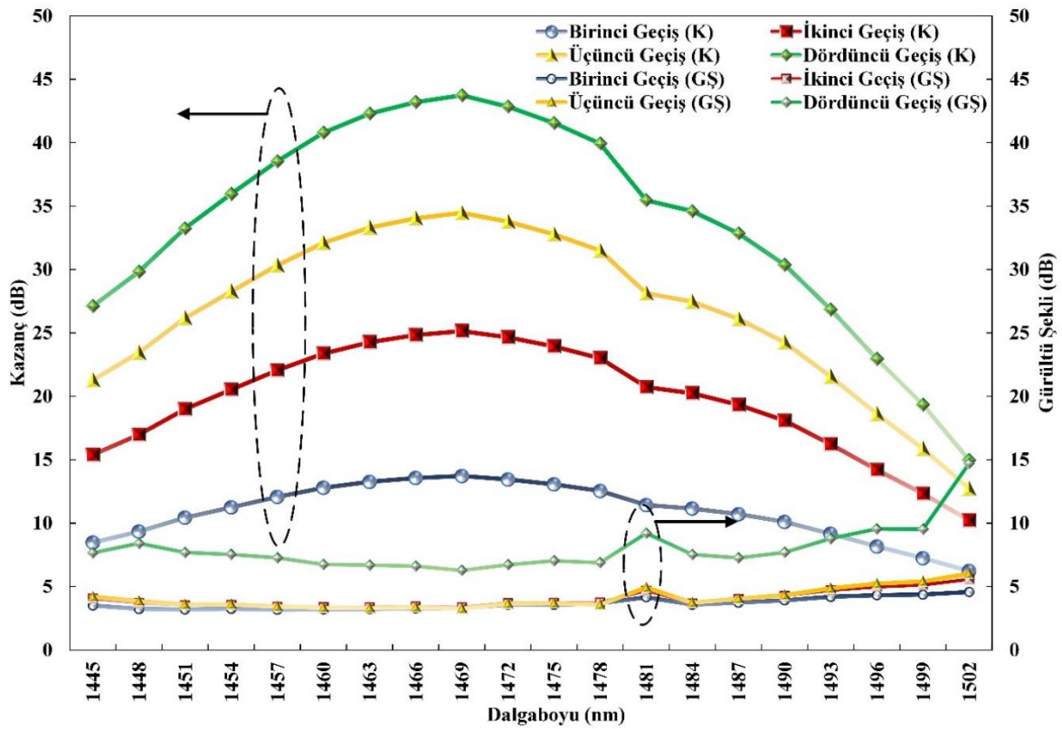
Şekil 6.63. ÜADG-TKFY I konfigürasyonunun her dört geçişinde elde edilen kazanç ve gürültü şekli değişimi
