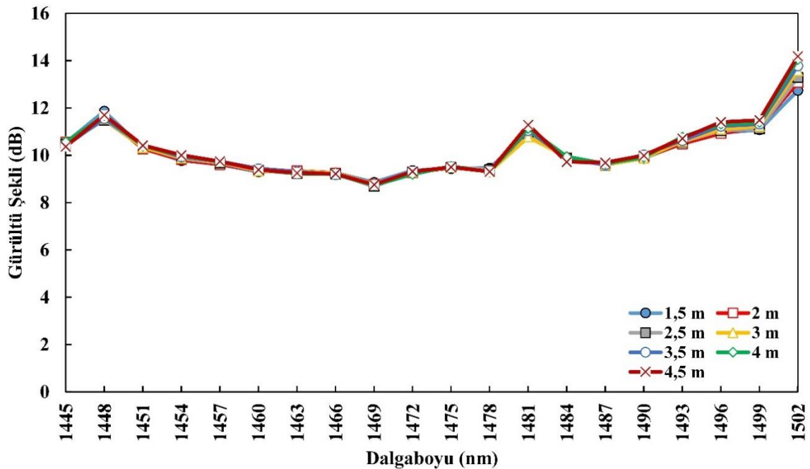
Şekil 6.37. İAÜG-TKFY II için TKF boyu-gürültü şekli değişimi
