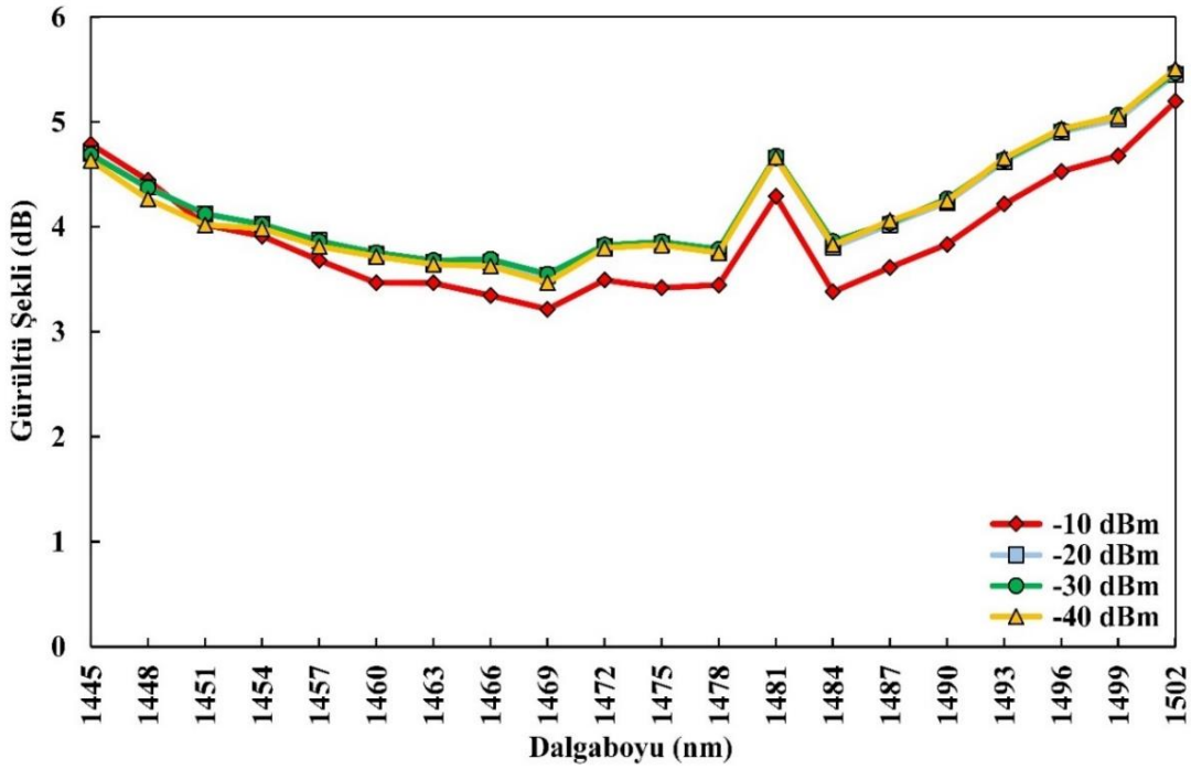
Şekil 6.41. ÜAÜG-TKFY için giriş gücü-gürültü şekli değişimi
