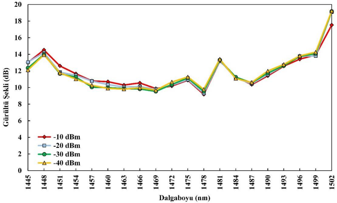
Şekil 6.74. ÜADG-TKFY III için giriş gücü-gürültü şekli değişimi
