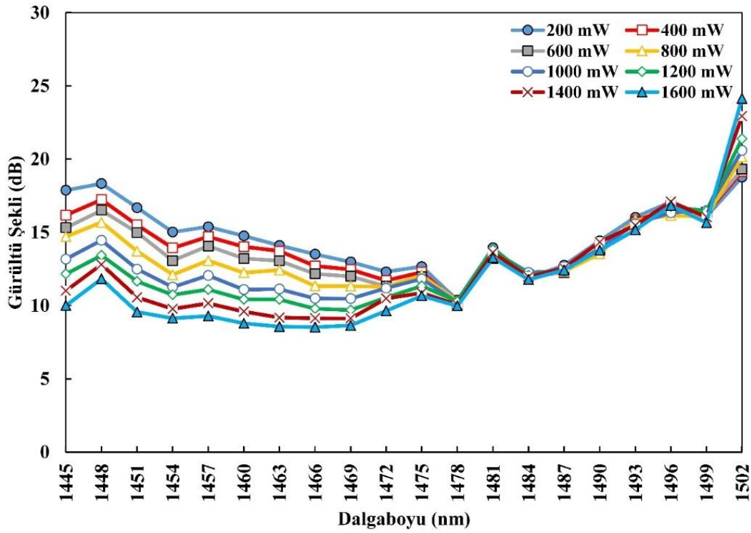
Şekil 6.35. İAÜG-TKFY II için pompa gücü- gürültü şekli değişimi
