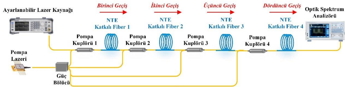
Şekil 5.11. Dört aşamalı dört geçişli yükselteç konfigürasyonu
