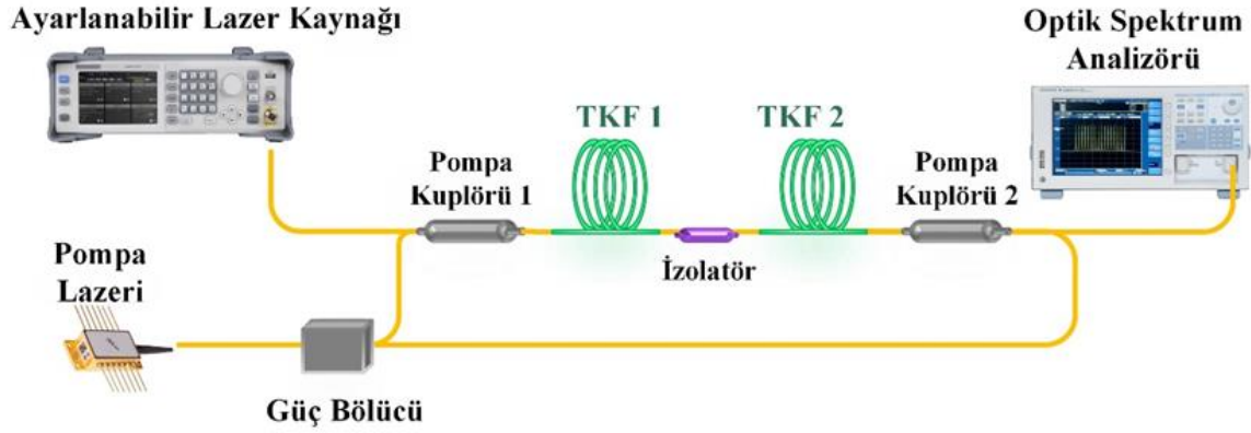
(c) İleri-Geri Yönlü Çift Geçişli TKFY (İGÇG-TKFY)
