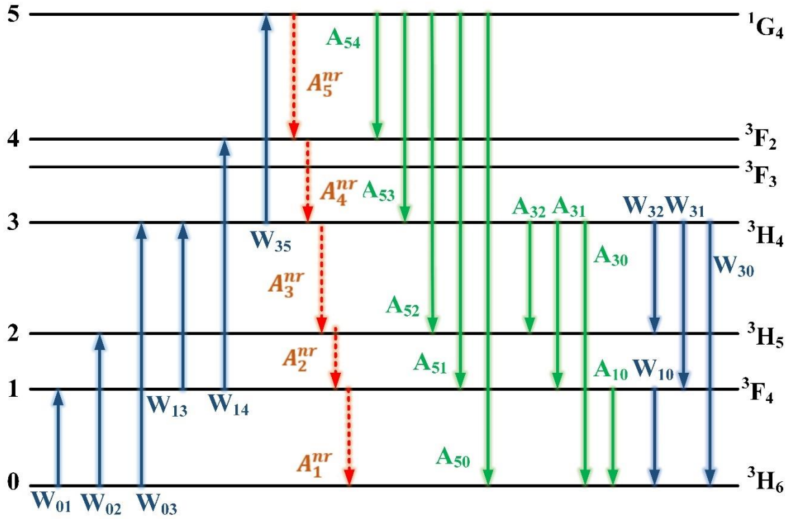
Şekil 4.6. Silika fiberdeki Tulyum iyonlarının enerji seviyeleri
