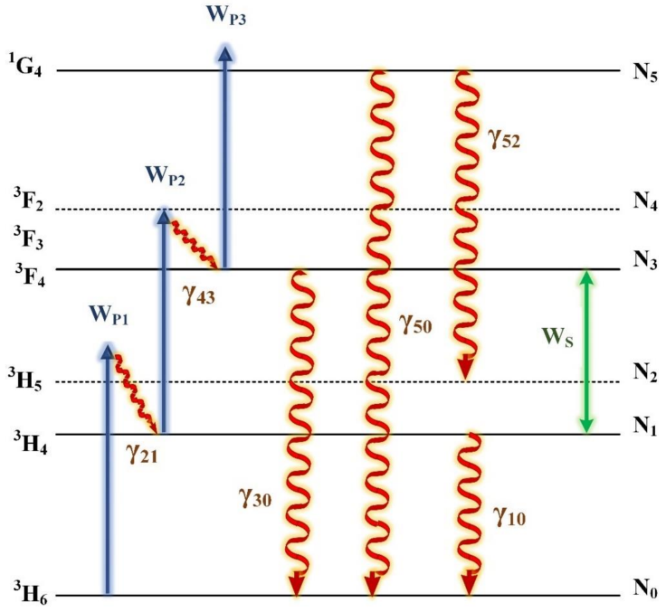
Şekil 4.5. Oran denklemleri analizi için oluşturulan model
