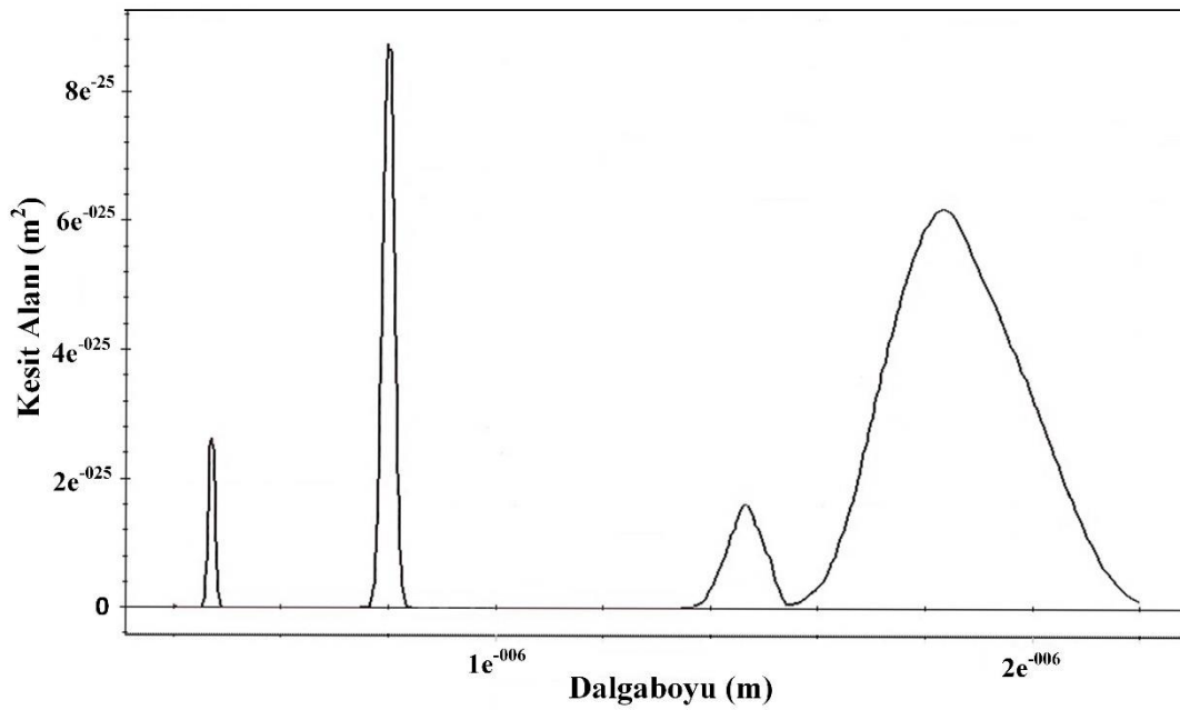
Şekil 6.1. Optisystem 21.0 Programında kullanılan Tm^{+3} yayılma spektrumu
