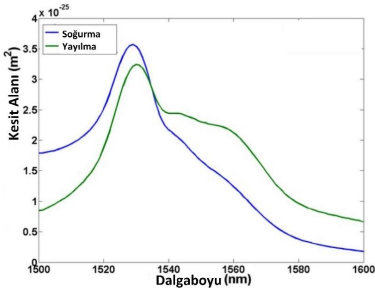
Şekil 3.5. \text{Er}^{3+} 'un soğurma ve yayılma spektrumları
