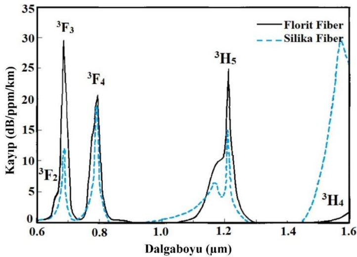
Şekil 4.3. Tulyum'un soğurma ve yayılma spektrumunun Florit (ZBLAN) ve Silika tabanlı fiber üzerinden karşılaştırması
