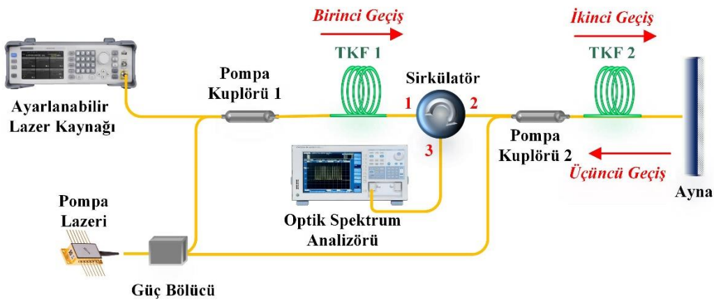
Şekil 6.23. İki aşamalı üç geçişli TKFY I
