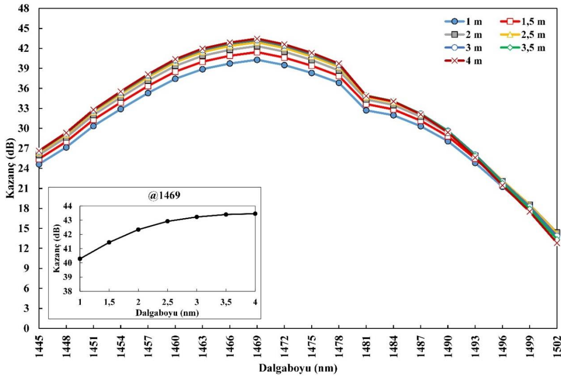
Şekil 6.53. İADG-TKFY için TKF boyu-kazanç değişimi
