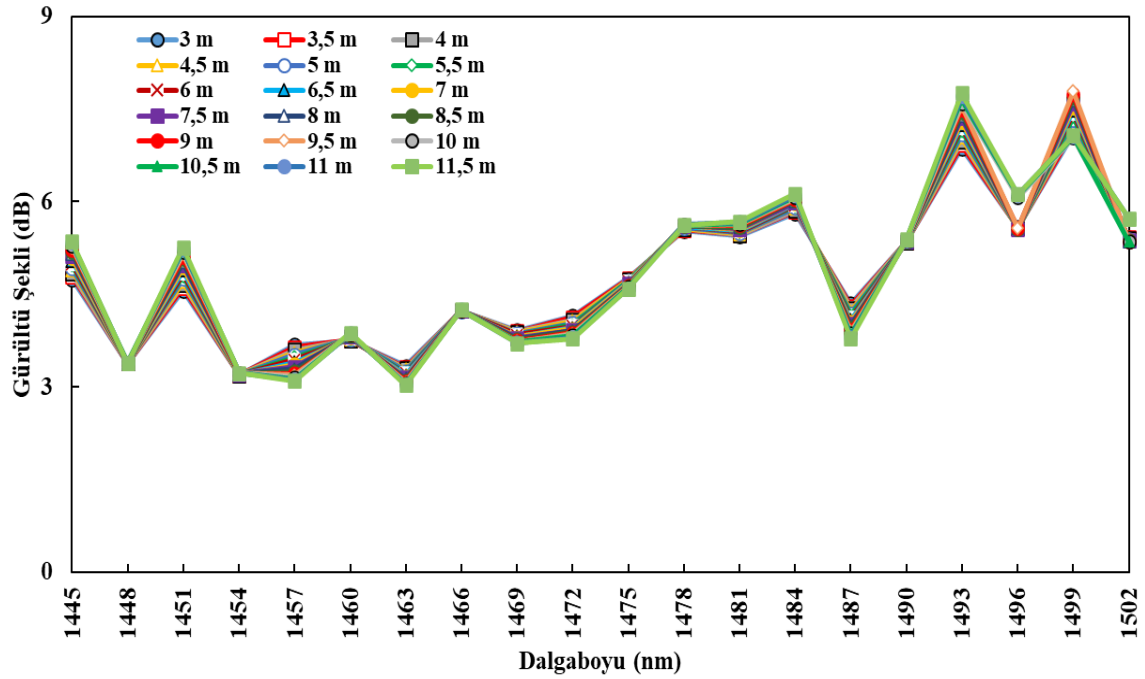
Şekil 6.20. İAÇG-TKFY için TKF 2 boyu-gürültü şekli değişimi
