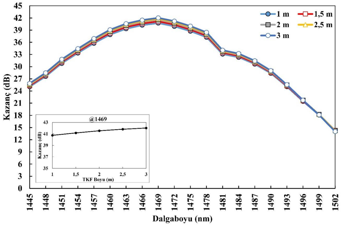
Şekil 6.69. ÜADG-TKFY II için TKF boyu-kazanç değişimi
