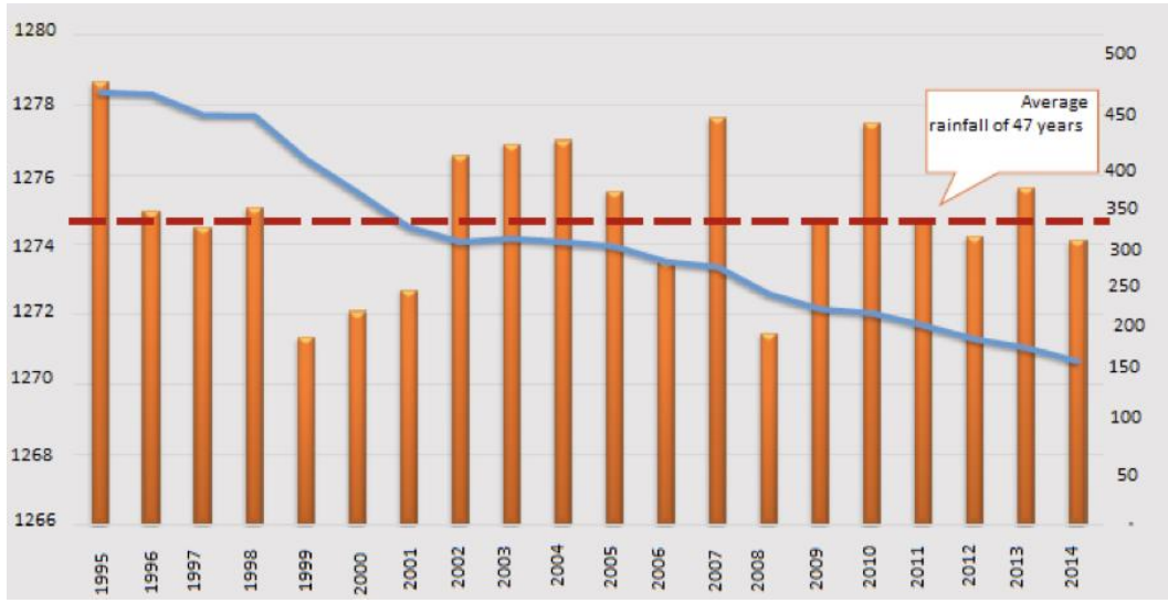
Grafik (3.1). 1995'ten 2014'e kadar Urmu Gölü'nün su seviyesindeki değişiklikler ve Urmu Gölü havzasındaki yağış oranı (ULRP)
