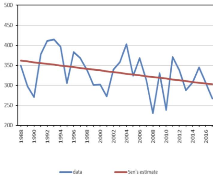
Şekil (3.4.): İran'ın ortalama yağış Oranı (mm)
