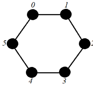
Şekil 1.4: C_6 grafi.
