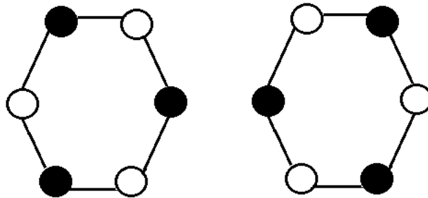
Şekil 1.5: C_6 grafinin kopma kümesi.
