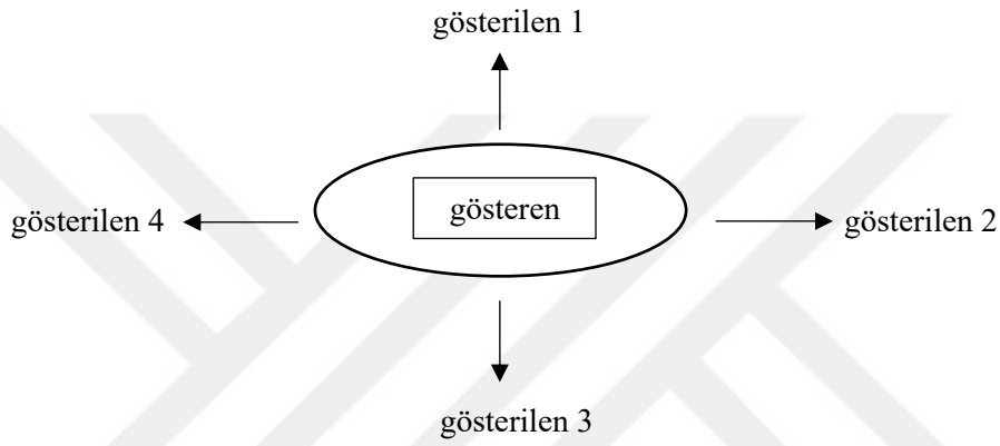
Şekil 2. 11. : Çok Anlamlılık 158
