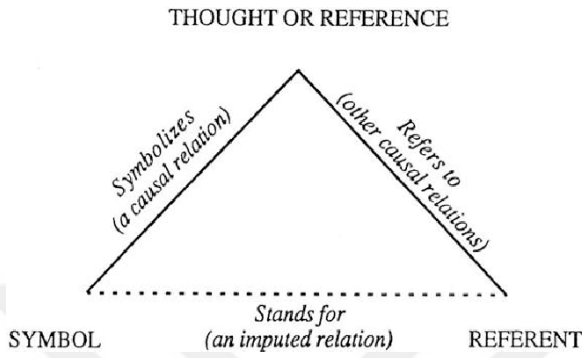
Şekil 2.2. : Ogden-Richards üçgeni
