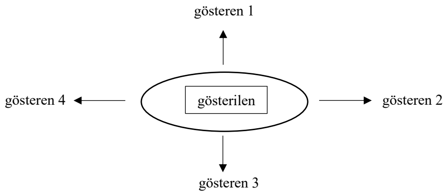
Şekil 2.8. : Eş anlamlılık 144
