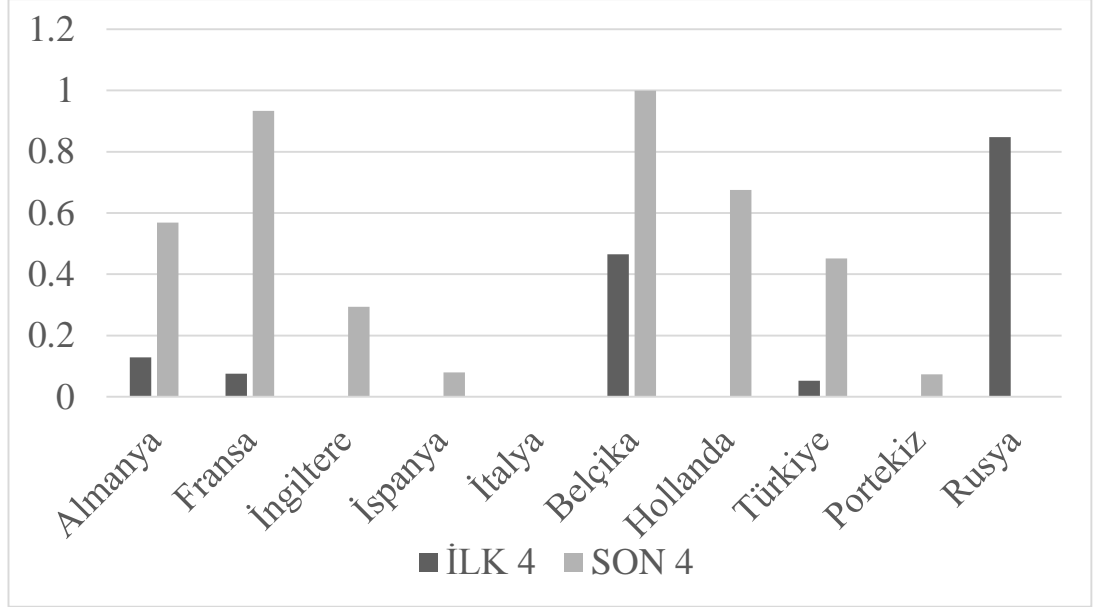
Şekil 4.3. Ülkelerin İlk 4 ve Son 4 Hafta Sıralamalarının Haftalara Göre Karşılaştırılmasına Göre Grafikleri.
