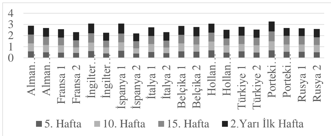
Şekil 4.1.Sezon Sonunda İlk 4 İçinde Yer Alan Takımların Belirli Haftalardaki İlk 4 İçinde Bulunma Olasılıklarına Göre Grafikleri.
