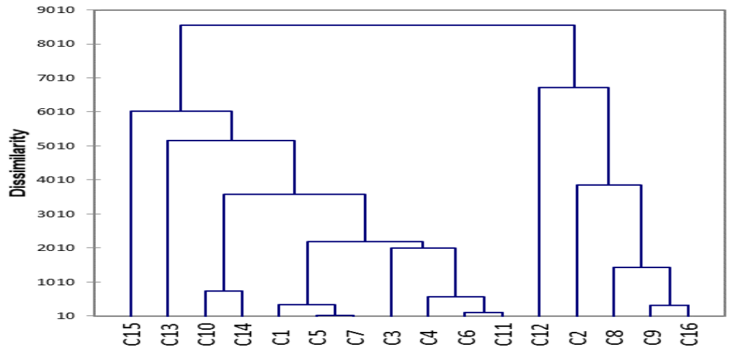
Şekil 4.1. Dendrogram
