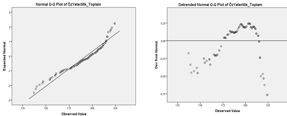
Şekil 1: Q-Q Plot ve Detrended Q-Q Plot Grafikleri
