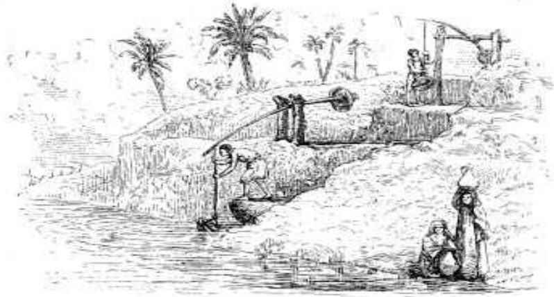
Görsel 8: Tipik bir şaduf örneği. 210
