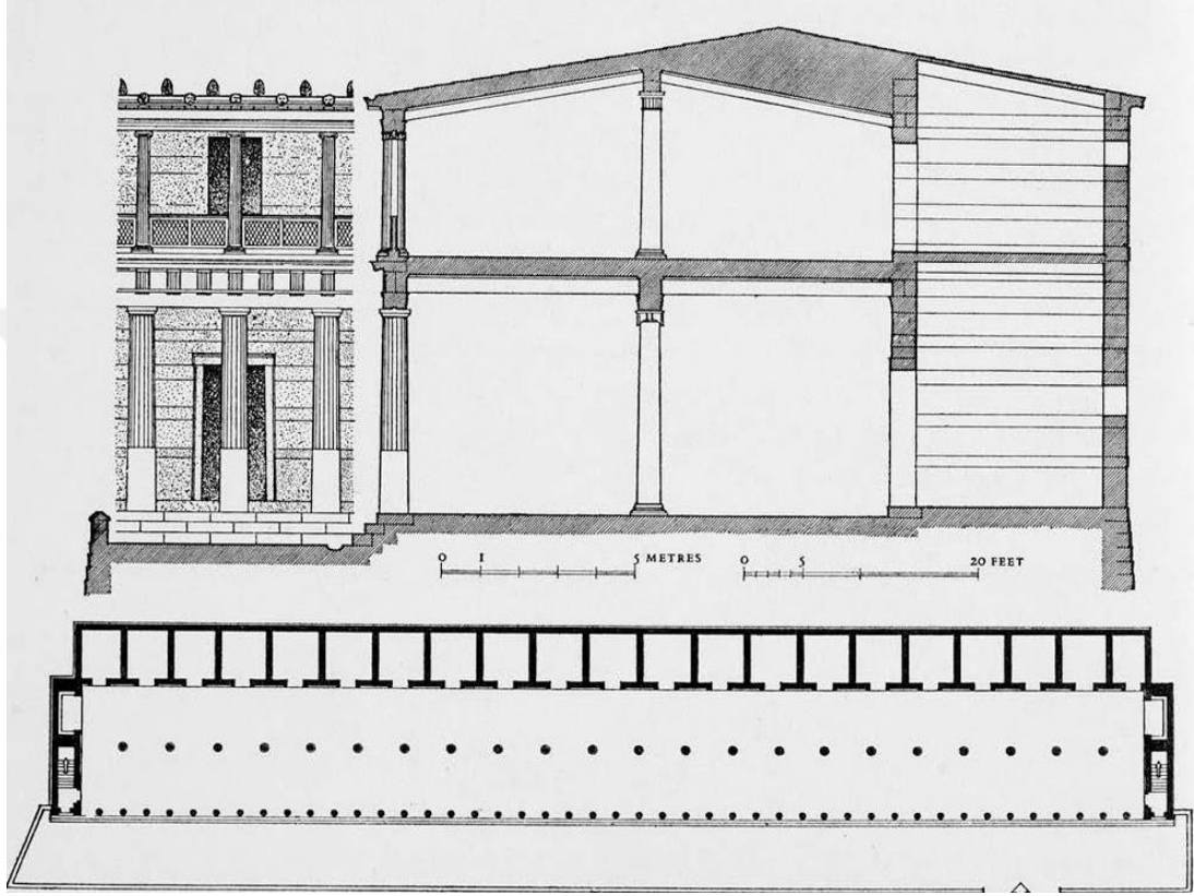
Görsel 65: Helenistik dönemde İki katlı inşa edilmeye başlanan stoalardan en önemlisi olan Attalos Stoa’sının planı. 1744
