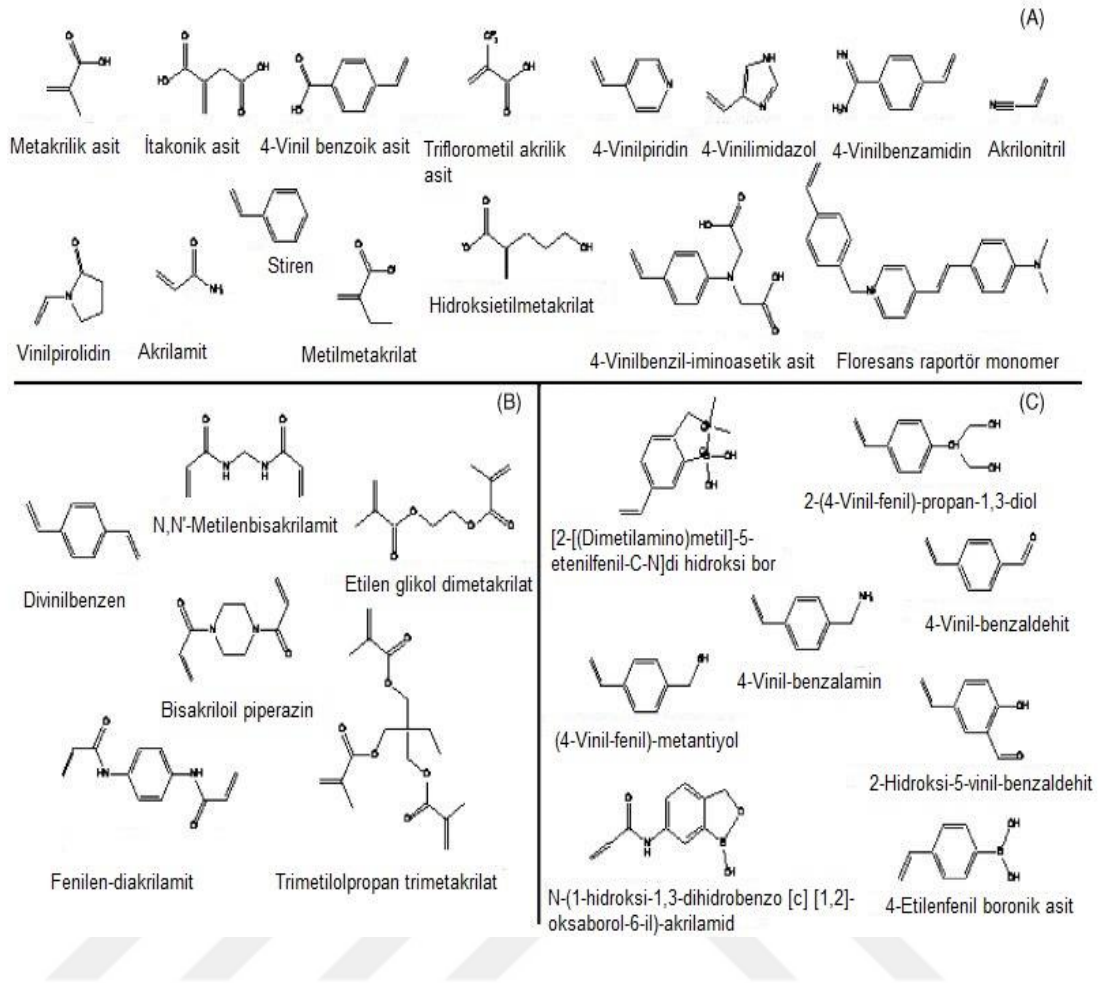
Şekil 2. 3. (A) Tek başına veya kovalent olmayan moleküler baskıda kombinasyon halinde kullanılabilen organik polimerize fonksiyonel monomerlerin örnekleri. (B) Moleküler baskılı polimerlerin sentezi için kullanılabilen çapraz bağlama monomerlerinin örnekleri. (C) Kovalent moleküler baskılamada kullanılabilen organik polimerize olabilen fonksiyonel monomerlerin örnekleri (Holthoff ve Bright, 2007).
