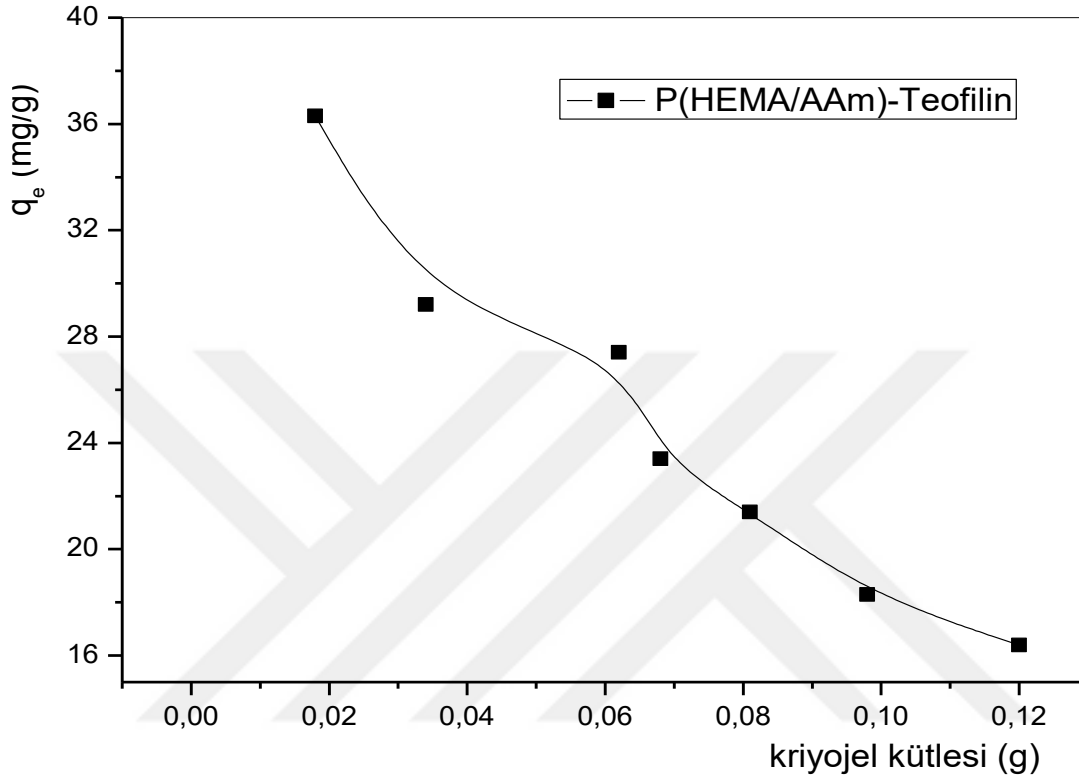
Şekil 4. 12. (PHEMA/AAm) kriyojel membran miktarının adsorpsiyon kapasitesine etkisi (25 mL 400 ppm teofilin, fosfat tamponu, pH=7, 25°C, 3 saat).
