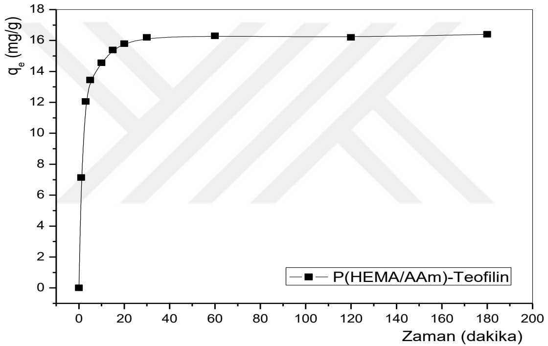
Şekil 4.18. Etkileşim süresinin adsorpsiyon kapasitesine etkisi (25 mL 400 ppm teofilin, 0,12 gram kriyojel, fosfat tamponu, pH=7, 25°C).
