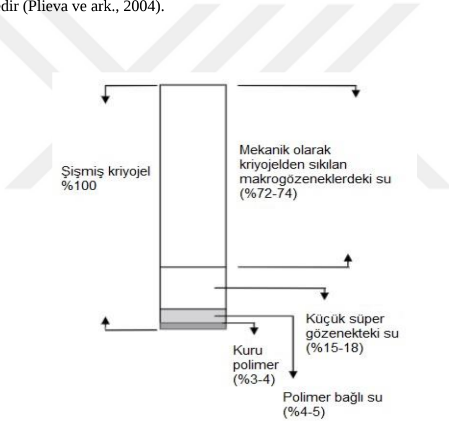
Şekil 2.7. (-12°C)' de hazırlanan süper makrogözenekli monolitik kriyojelin bileşimi (Adrados ve ark., 2001).
