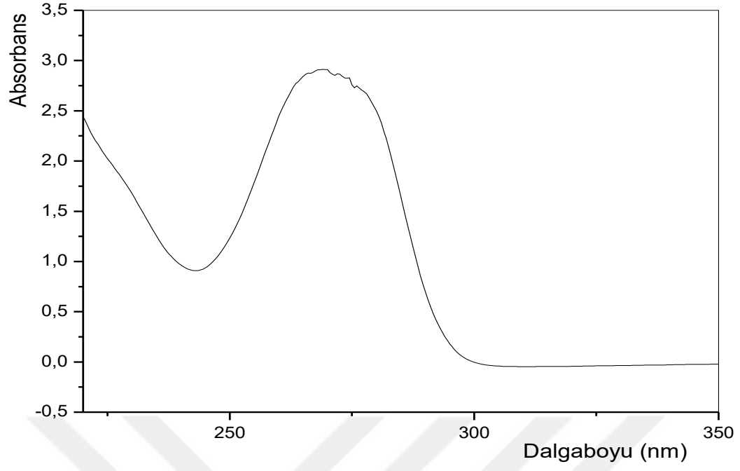
Şekil 3. 2. Teofilin çözeltisi için UV-Vis spektroskopisi (50 ppm, saf suda, \lambda_{\text{max}} = 271 \text{ nm} ).
