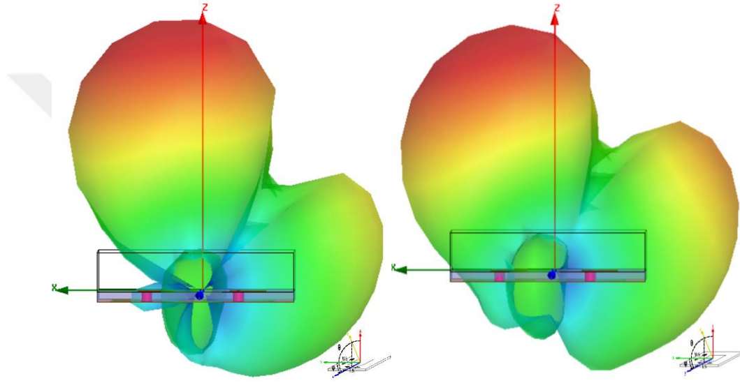
Şekil 4-9 \phi=0^\circ Ekseni 3 Boyutlu Hüzme Yönlendirme
