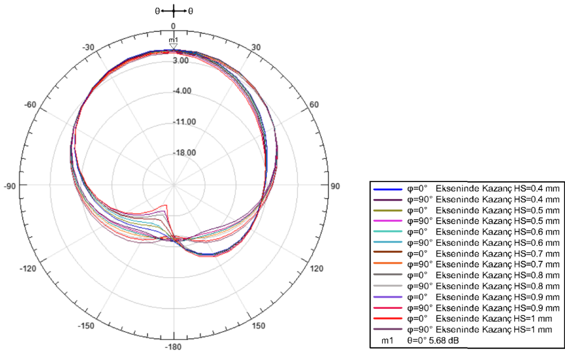
Şekil 3-13 \phi=0^\circ & \phi=90^\circ Eksenlerinde Alttaş Yüksekliği Kazanç Analizi (Polar Grafik)
