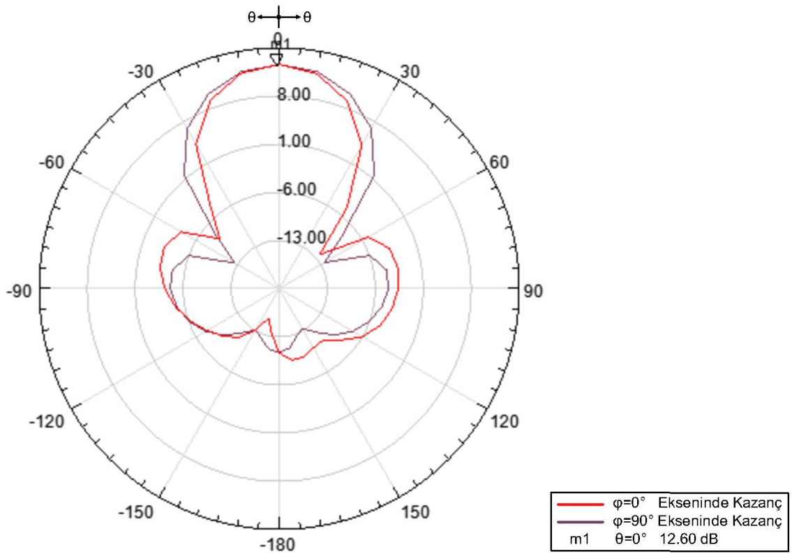
Şekil 4-7 \phi=0^\circ & \phi=90^\circ Eksenleri Kazanç (Polar Grafik)
