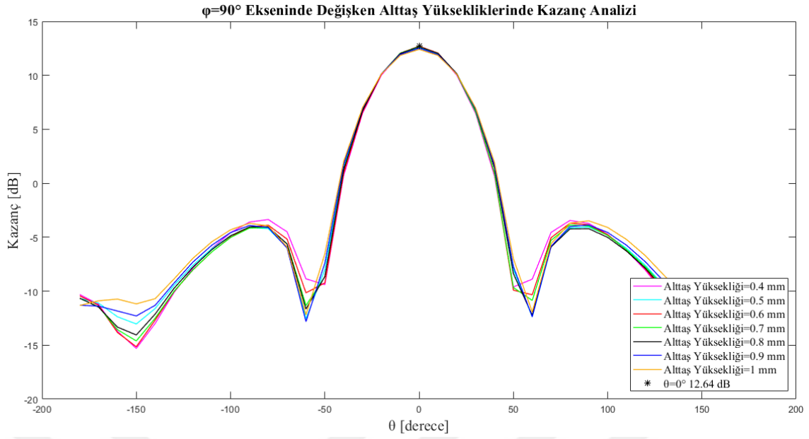
Şekil 4-13 \varphi=0^\circ ve \varphi=90^\circ Eksenlerinde Değişken Altaş Yüksekliklerinde Kazanç Analizi
