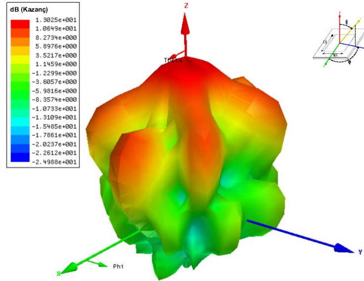
Şekil 4-21 3 Boyutlu Kazanç Grafiği
