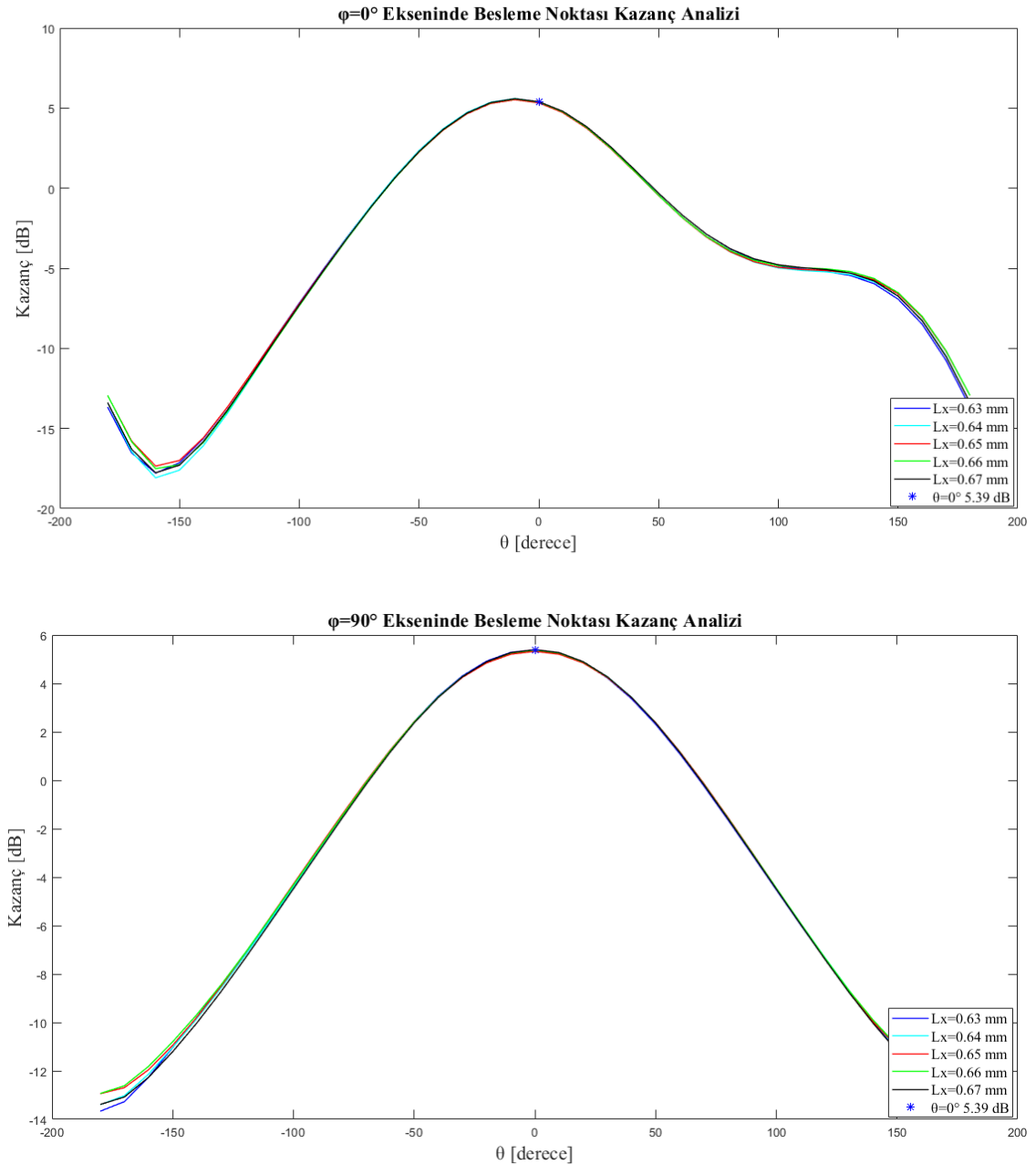
řekil 3-9 \varphi=0^\circ & \varphi=90^\circ Eksenlerinde Besleme Noktası Kazan Analizleri
