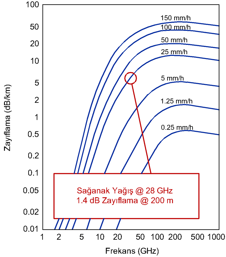
Şekil 1-1 Frekans – Zayıflama [14]
