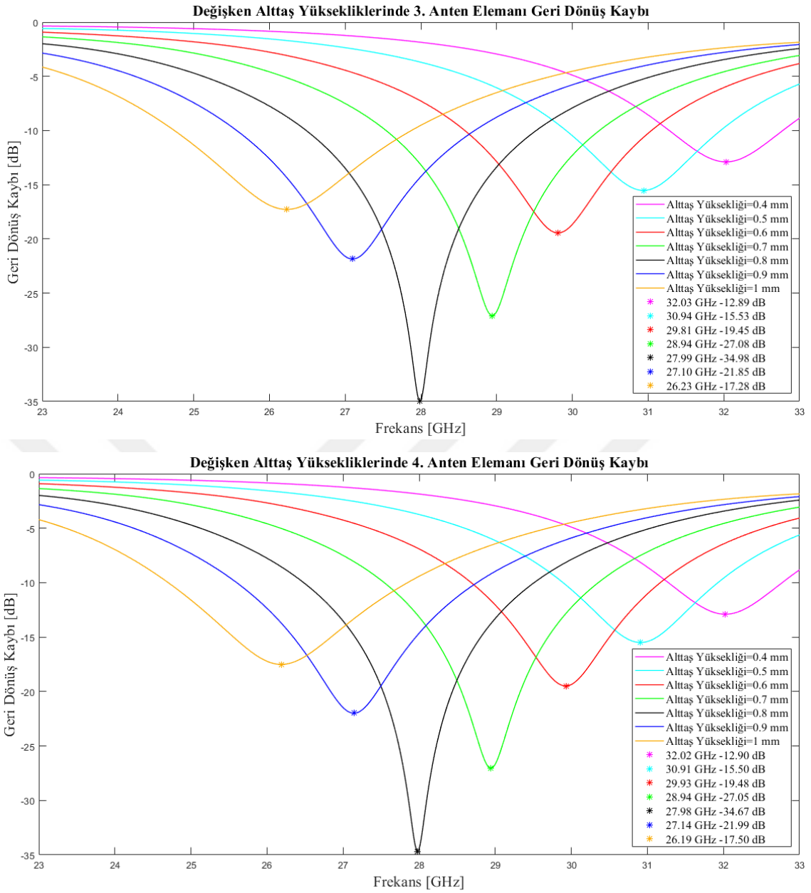
Şekil 4-11 Değişken Altaş Yüksekliklerinde Anten Elemanları Geri Dönüş Kaybı Değerleri
