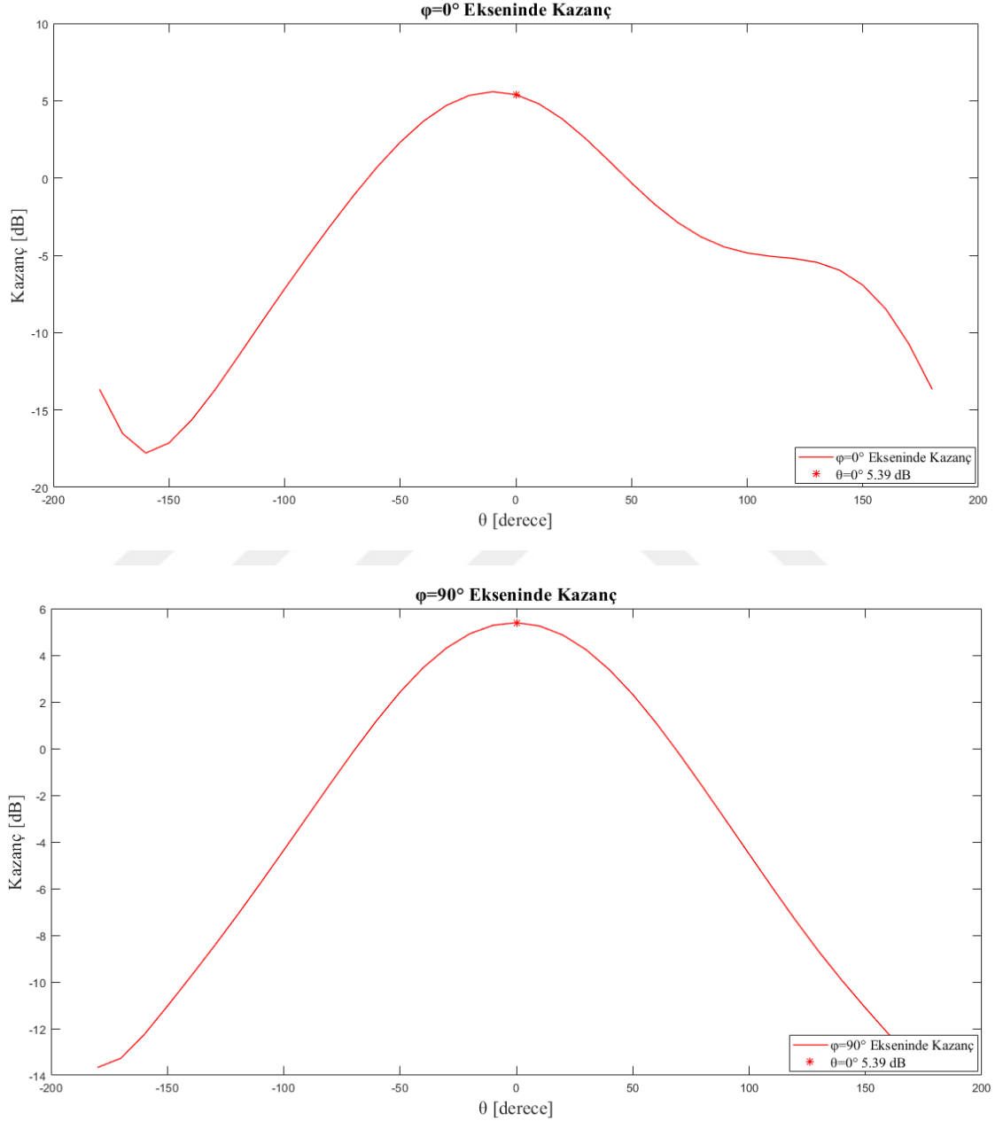
Şekil 3-5 \phi=0^\circ & \phi=90^\circ Eksenlerinde Kazanç Grafikleri
