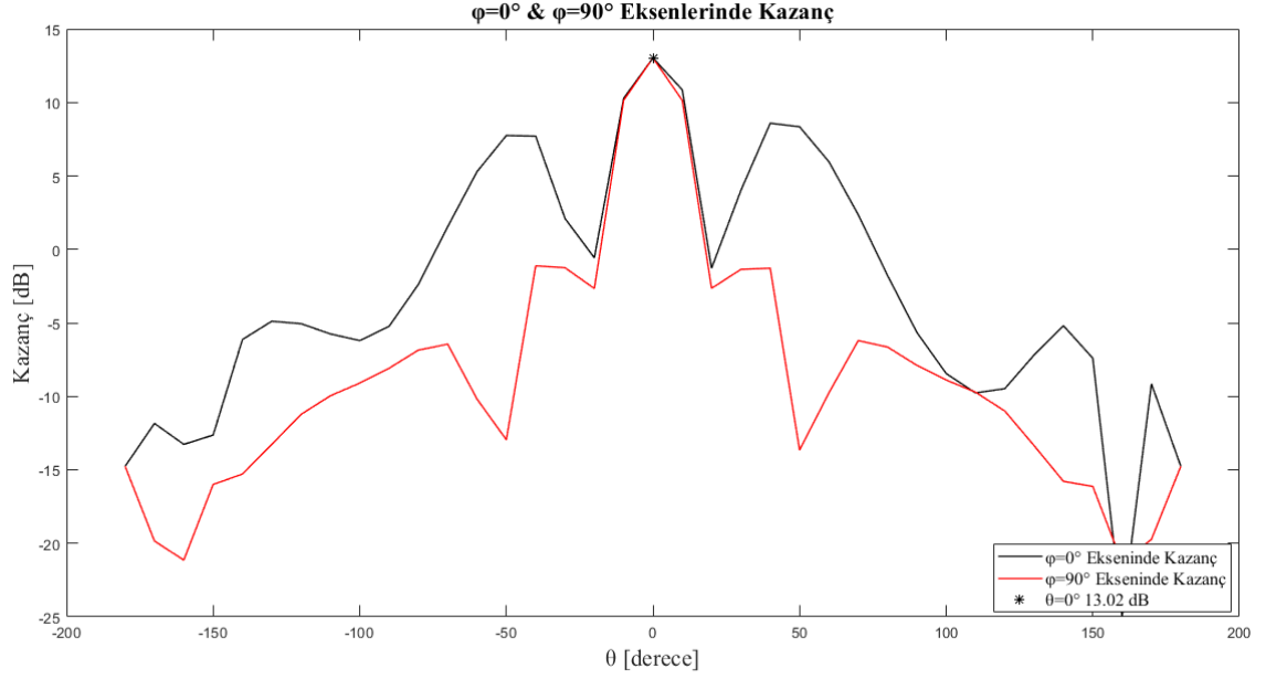
Şekil 4-19 \phi=0^\circ & \phi=90^\circ Eksenlerinde Kazanç
