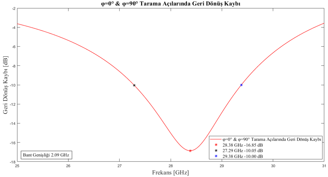
Şekil 3-14 \phi=0^\circ & \phi=90^\circ Tarama Açılarında Geri Dönüş Kaybı
