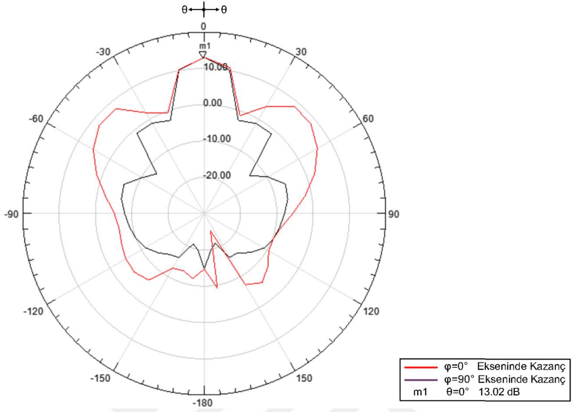
Şekil 4-20 \phi=0^\circ ve \phi=90^\circ Eksenlerinde Kazanç (Polar Grafik)
