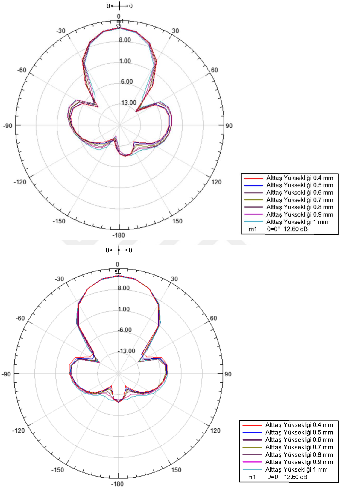
Şekil 4-14 \phi=0^\circ ve \phi=90^\circ Eksenlerinde Değişken Altaş Yüksekliklerinde Kazanç Analizi (Polar Grafik)
