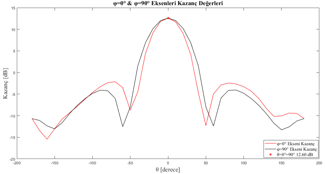
Şekil 4-6 \phi=0^\circ & \phi=90^\circ Eksenleri Kazanç Değerleri
