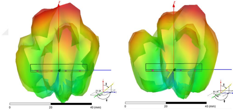
Şekil 4-22 X Ekseninde 3 Boyutlu Hüzmeye Yönlendirme
