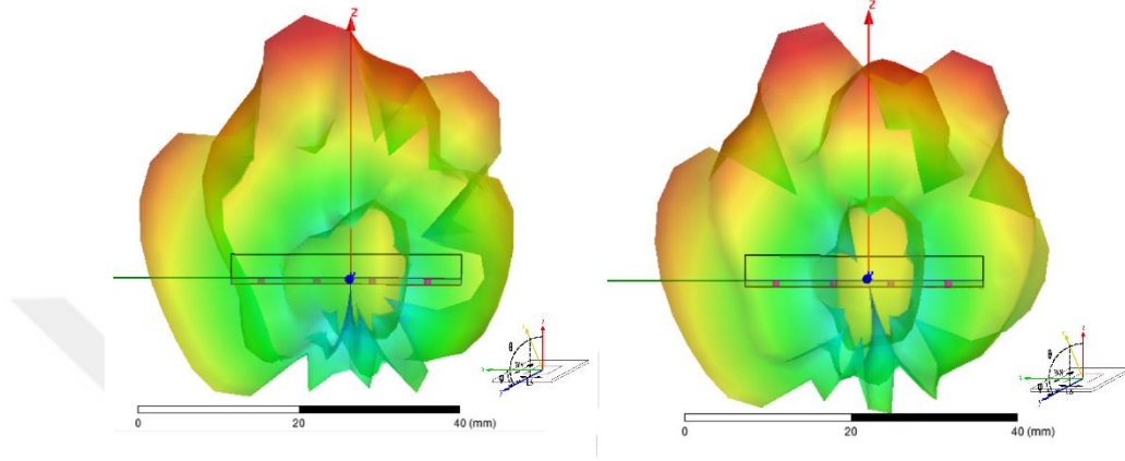
Şekil 4-22 X Ekseninde 3 Boyutlu Hüzmeye Yönlendirme
