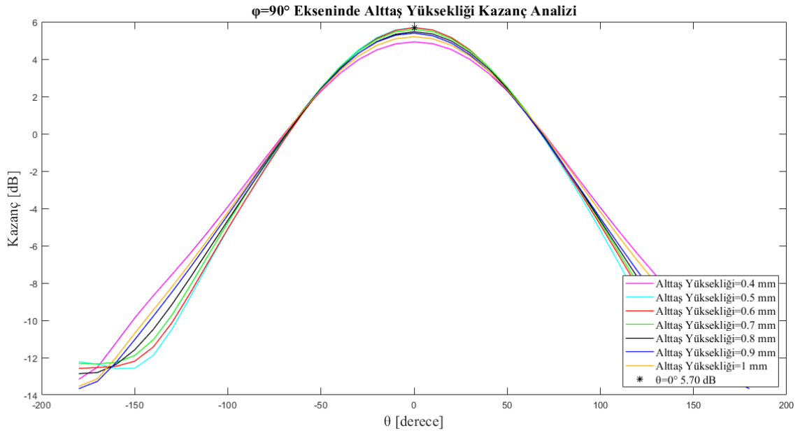
Şekil 3-12 \phi=0^\circ & \phi=90^\circ Eksenlerinde Alttaş Yüksekliği Kazanç Analizi
