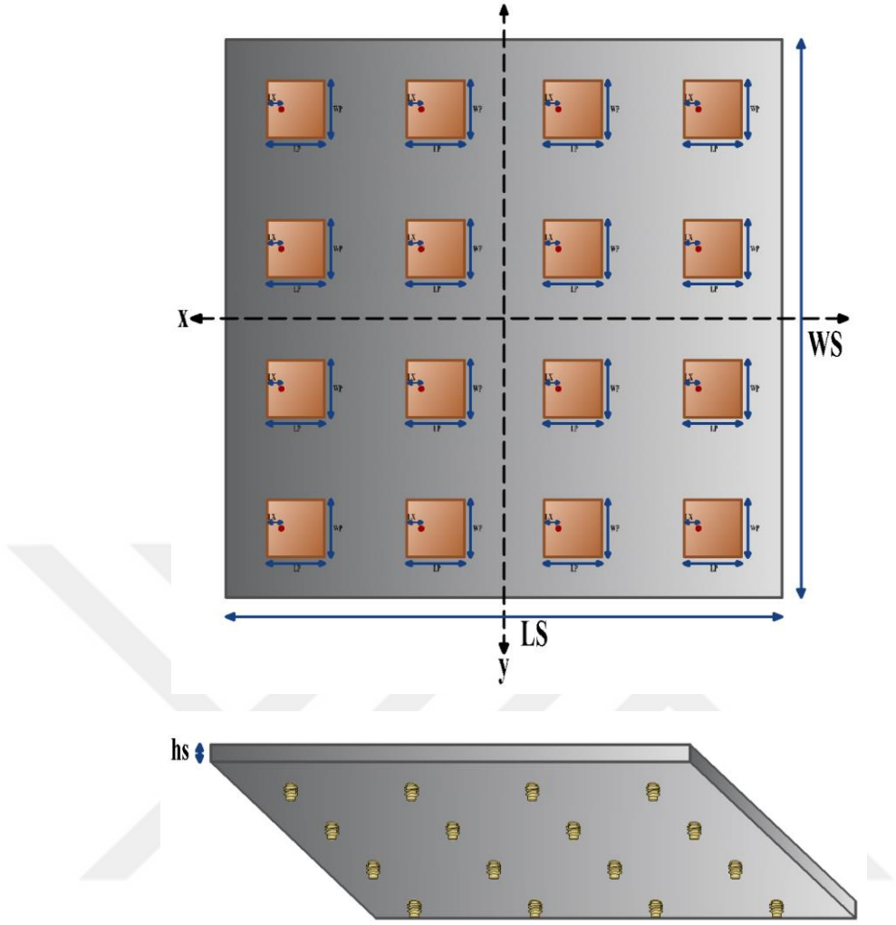
Şekil 4-15 4x4 Düzlemsel Dizi Anten Görseli
