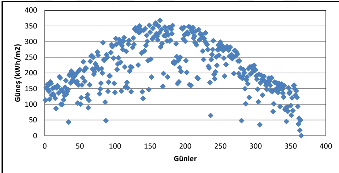
Şekil 6.9. Kandağhar şehrine ait gün- güneş ışıınımlı grafiğı
