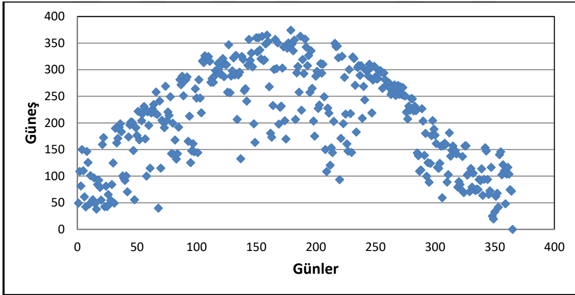
Şekil 6.4. Herat şehrine ait gün- güneş ışıını mı grafiği
