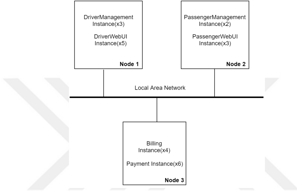
Şekil 5.2. Aynı servis örneklerinin bir grupta toplandığı örnek bir dağıtım alternatifi
