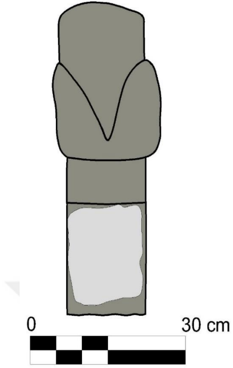
Çizim 26. Başucu Taşı (Kat. No: 15).
