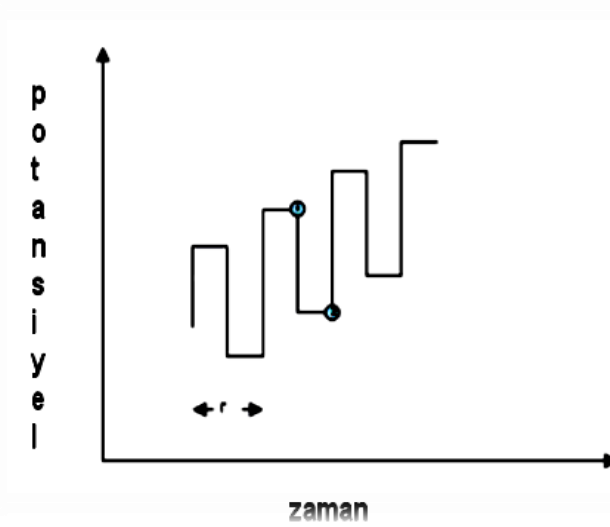
Şekil 2.5. Kare dalga voltametrisi için uyarma sinyali
