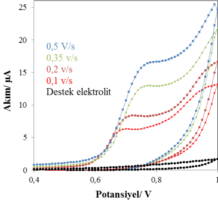
Şekil 4.3. 1,01 \times 10^{-4} mol.L -1 CAR'ın, MeOH-BR ortamında (1:5) ZnO NP-KPE'de farklı tarama hızlarında alınan dönüşümlü voltamogramları
