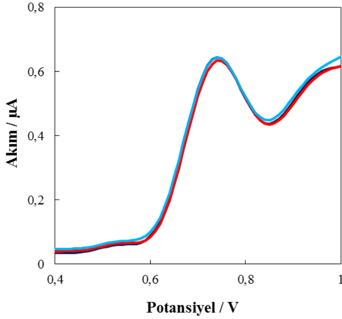
Şekil 4.15. KDAAdSV yöntemi ile aynı gün, aynı çözeltide yapılan ölçümlere ait voltamogramlar ( E_{bir} : 0,3 V, t_{bir} : 15 s, C_{CAR} : 1,01 \times 10^{-4} \text{ mol L}^{-1} , pH 8,0)
