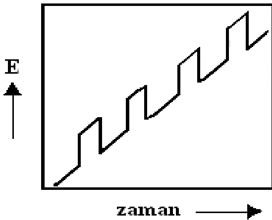
Şekil 2.4. Diferansiyel puls voltametrisi için uyarma sinyali
