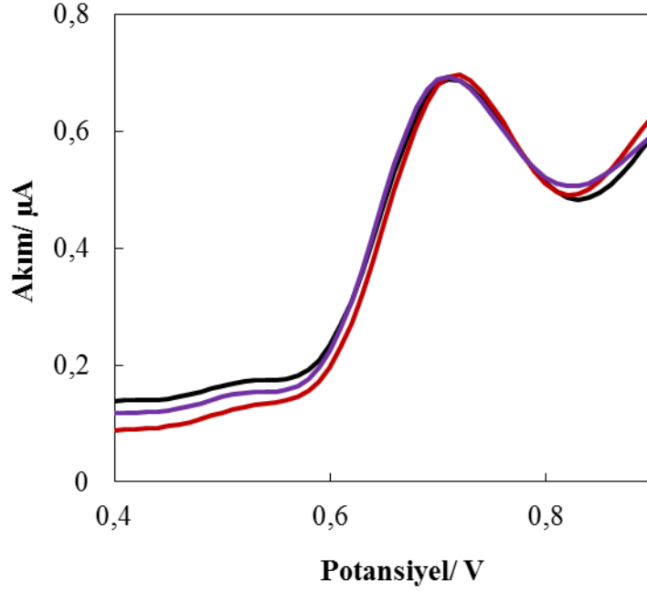
Şekil 4.16. KDAAdSV yöntemi ile farklı gün, farklı çözeltide yapılan ölçümlere ait voltamogramlar ( E_{bir} : 0,3 V, t_{bir} : 15 s, C_{CAR} : 1,01 \times 10^{-4} \text{ mol L}^{-1} , pH 8,0)
