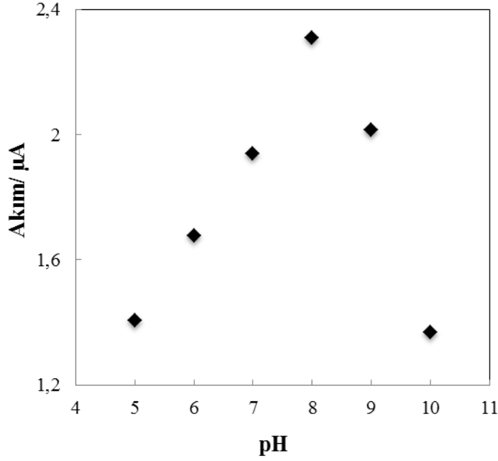
Şekil 4.6. 1,01 \times 10^{-4} \text{ molL}^{-1} CAR'ın ZnO NP-KPE'ta KDV yöntemi ile elde edilen pik akımlarının pH ile değişim grafiği
