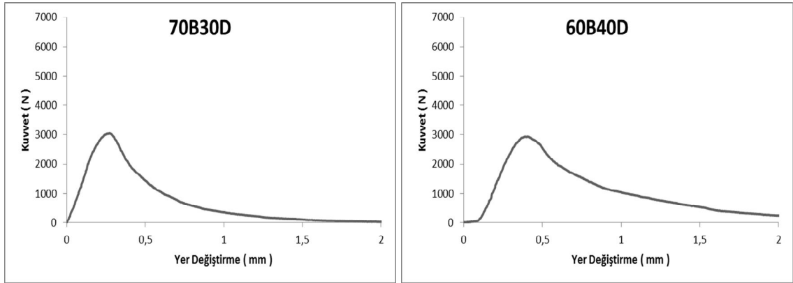
Şekil 4.23 Eş basınç-sıcaklık değerleri için Kuvvet yerdeğiştirme grafikleri
