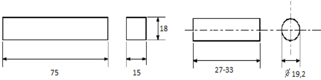
Şekil 3.39 Ham numune geometrileri
