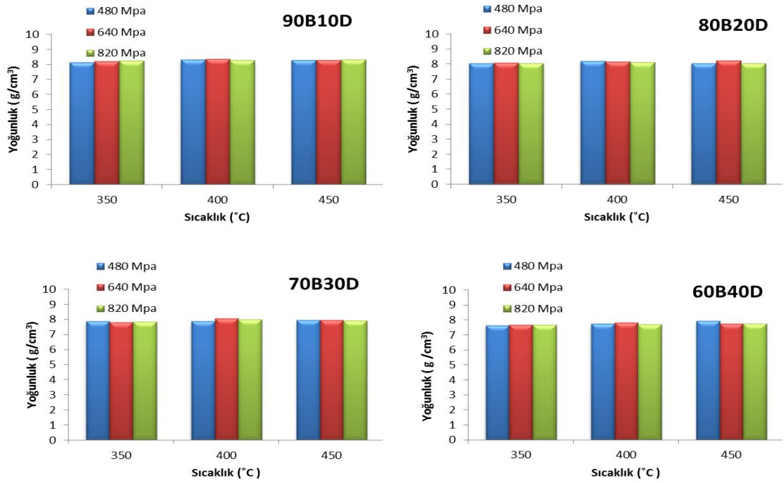
Şekil 4.1 Silindirik numunelerin yoğunluk değerleri
