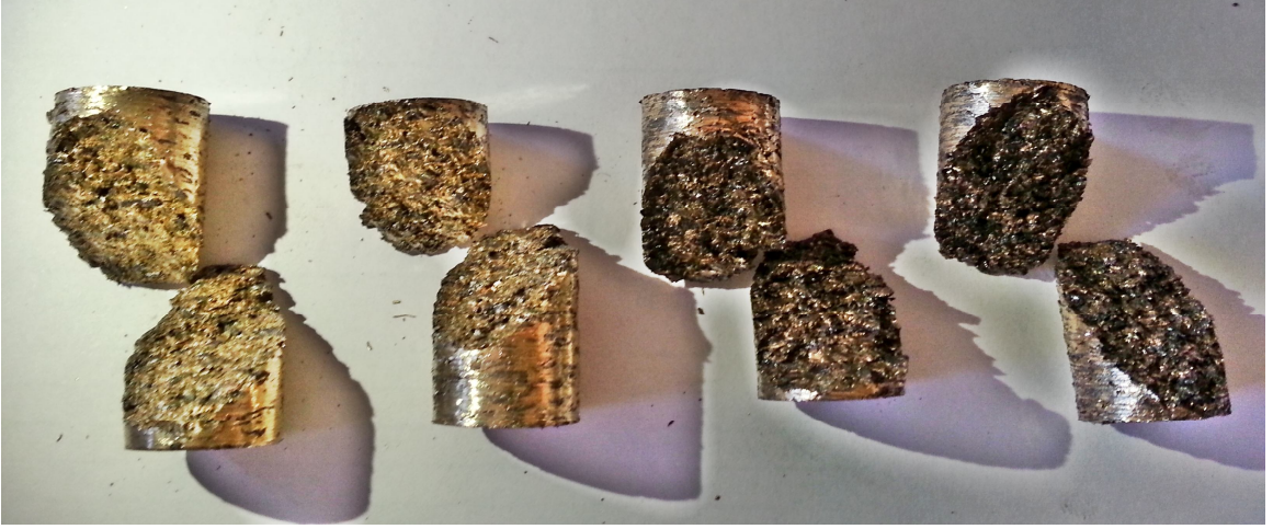
Şekil 4.10 820MPa ve 400°C de üretilen numuneler (%90-80-70-60 CuSn10) kırılma şekilleri
