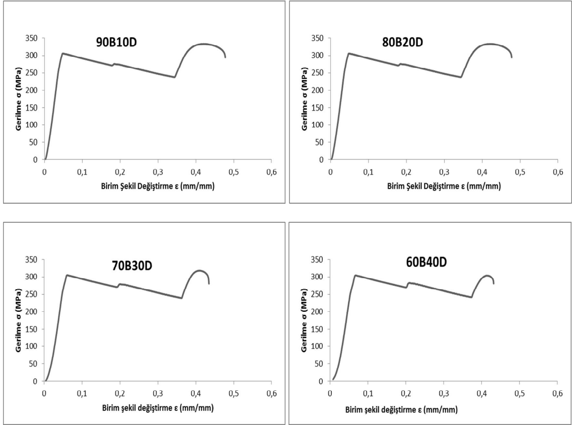
Şekil 4.12 Eş basınç-sıcaklık değerleri için gerçek gerilme-gerçek şekil değiştirme grafikleri
