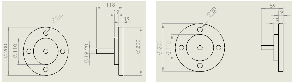
Şekil 3.20 Silindirik erkek zımbalar teknik resim
