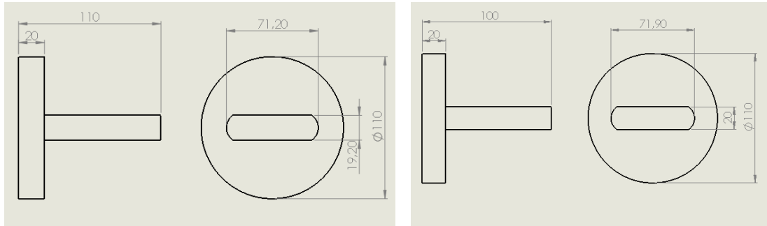
Şekil 3.22 Prizmatik erkek zımbalar teknik resim
