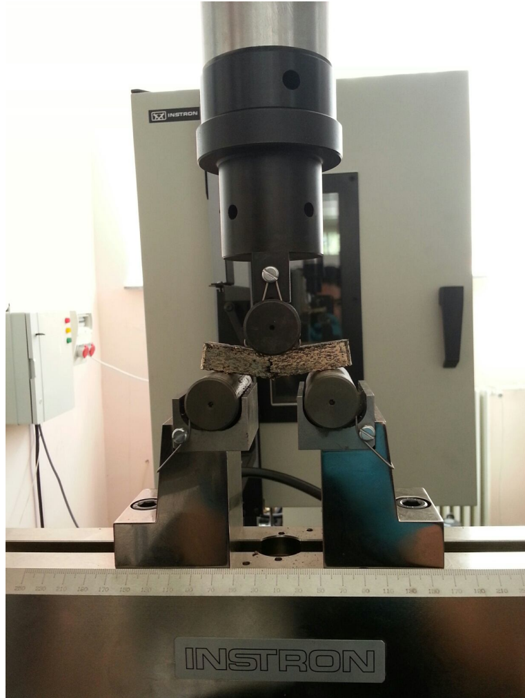
Şekil 3.55 Üç noktadan Eğme testi
