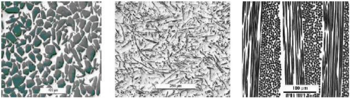
Şekil 3.2 Takviye fazına göre mikro yapılar (Eker A.)
