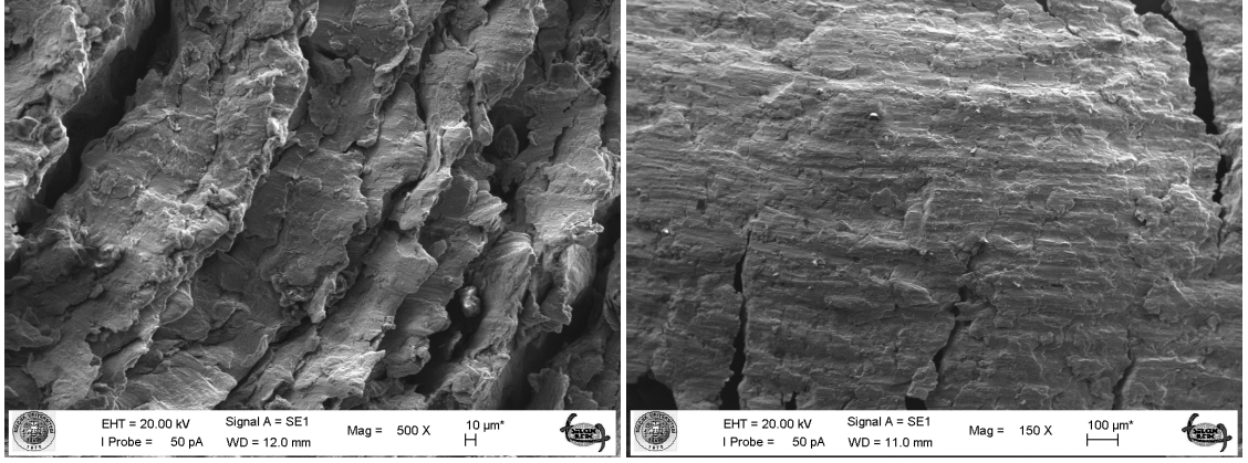
Şekil 3.13. 40 dakika ultrasonik temizlik sonrasında talaşların taramalı elektron mikroskobu görüntüsü a) CuSn10(10µm) b) CuSn10(100µm) c) GGG-40(10µm) d) GGG-40(100µm)
