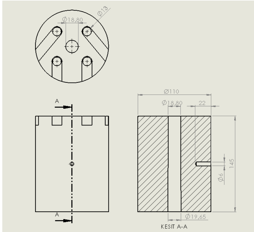
Şekil 3.19 Dişi silindirik kalıp teknik resim
