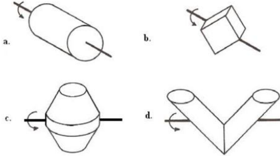
Şekil 3.23 Karıştırıcı tipleri (German, 1989)
