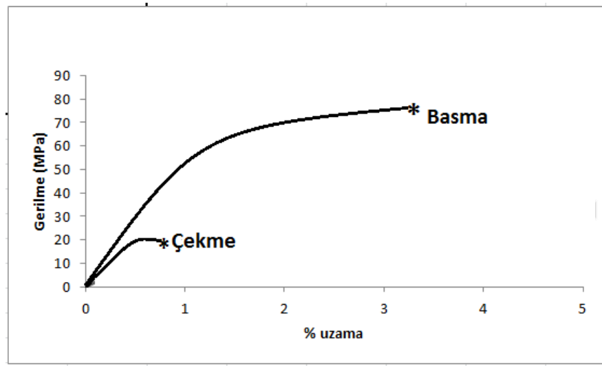
Şekil 3.52 Gri dökme demirin basma ve çekme deneyleri ile elde edilen mühendislik -gerilme ve uzama diyagramları
