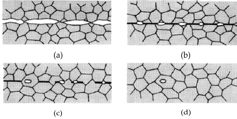
Şekil 3.4 Difüzyon bağı oluşumu (Madeleine Durand-Charre, 2003)
