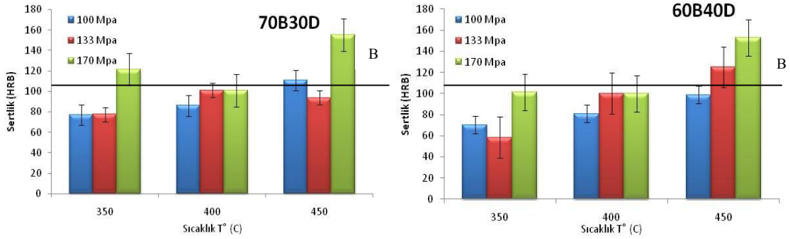
Şekil 4.6 Prizmatik numunelerde Brinell sertlik değerleri
