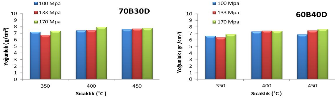
Şekil 4.2 Prizmatik numunelerin yoğunluk değerleri
