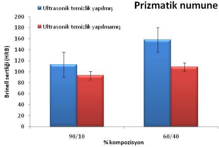
Şekil 3.16 Ultrasonik temizliğin Brinell sertliğine etkisi
