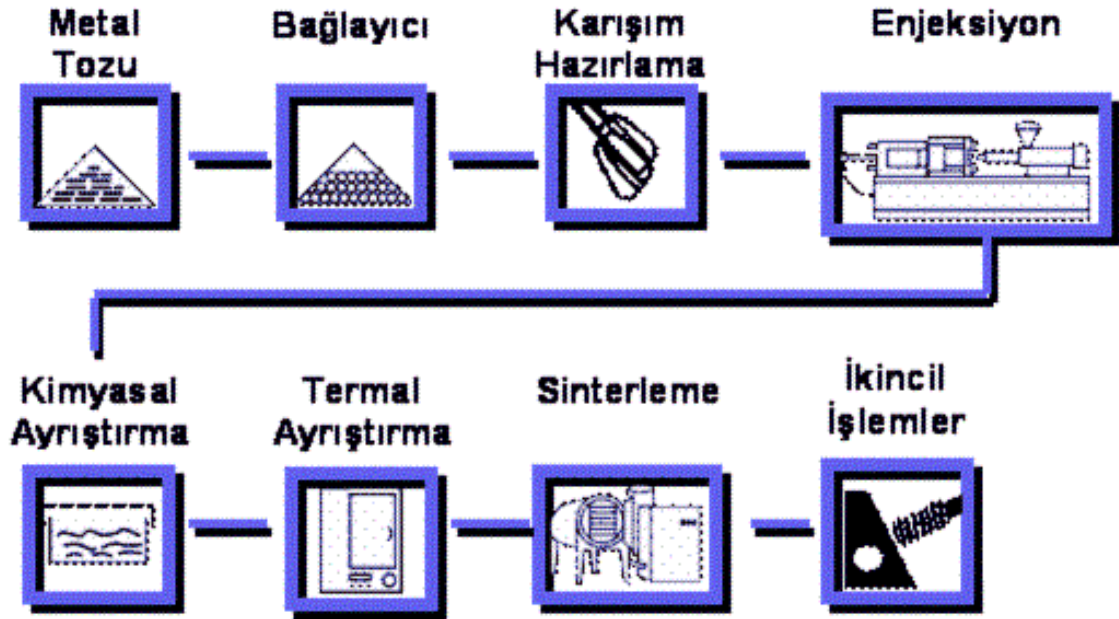
Şekil 3.7 Toz metalürjisi aşamaları (www.cneteknoloji.net)
