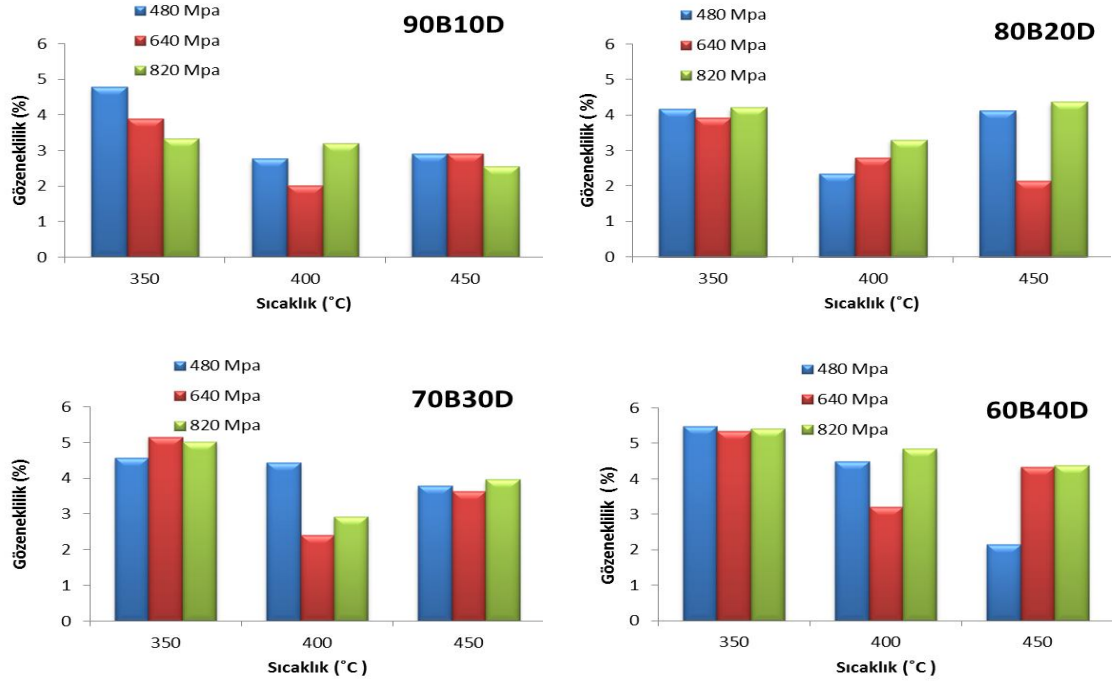
Şekil 4.3 Silindirik numunelerin gözeneklilik testi sonuçları
