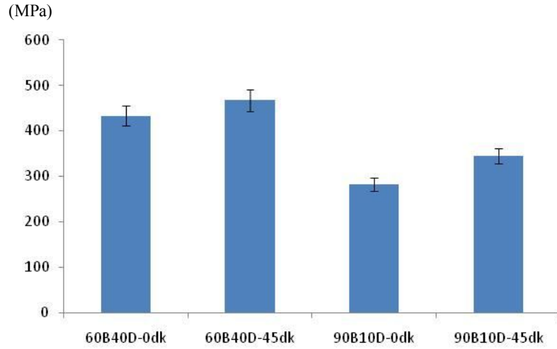
Şekil 3.16 Ultrasonik temizliğin Brinell sertliğine etkisi
