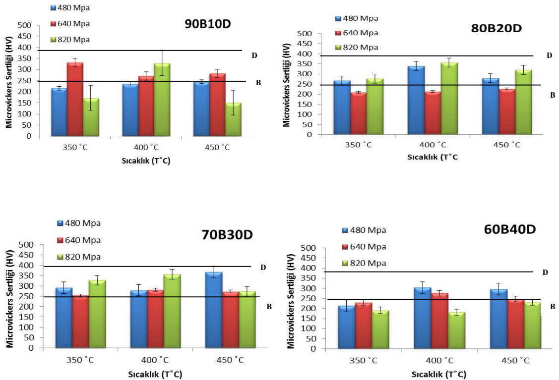
Şekil 4.7 Silindirik numunelerde mikro vikers sertlik değerleri
