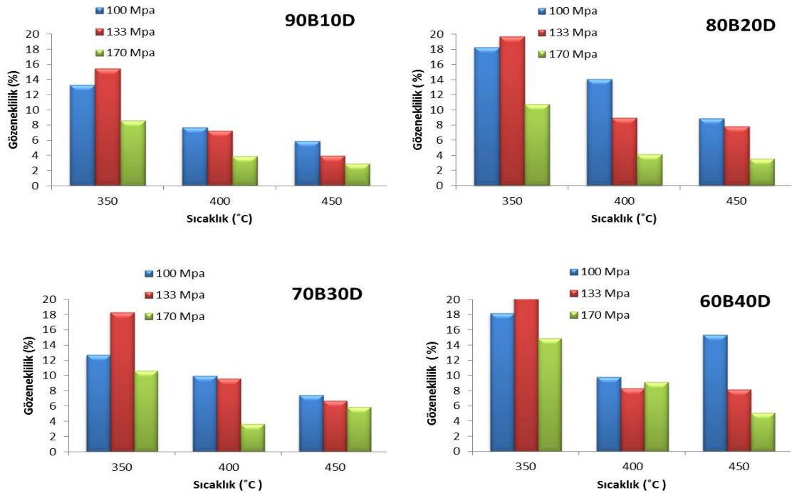
Şekil 4.4 Prizmatik numunelerin gözeneklilik testi sonuçları
