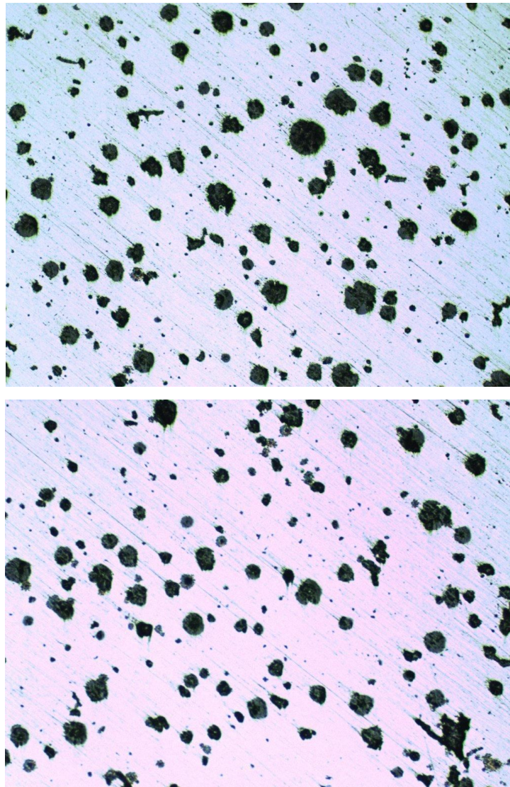
Şekil 3.9. GGG 40 mikro yapı görüntüsü (100X)
