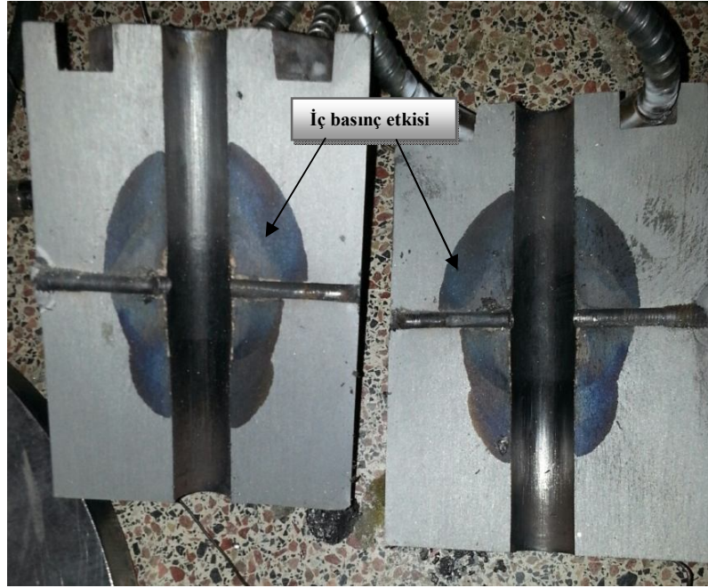
Şekil 3.33 İç basınç etkisi altında kırılan sıcak pres kalıbı
