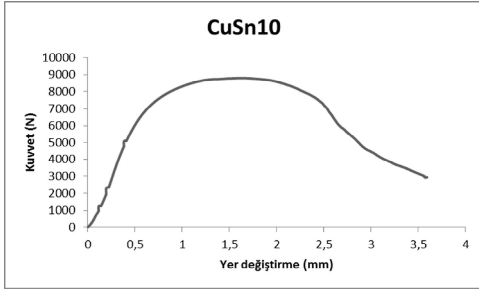
Şekil 4.22 Saf CuSn10 eğilme grafięi
