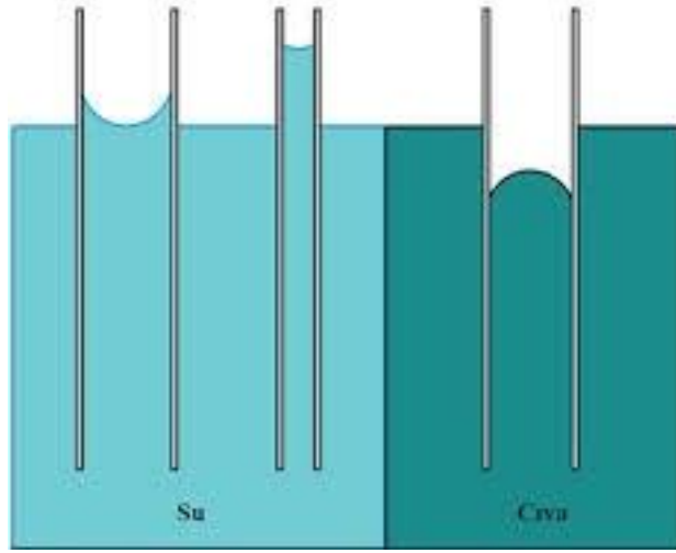
Şekil 3.5 Kapilar etki (Çengel Y., 2008)
