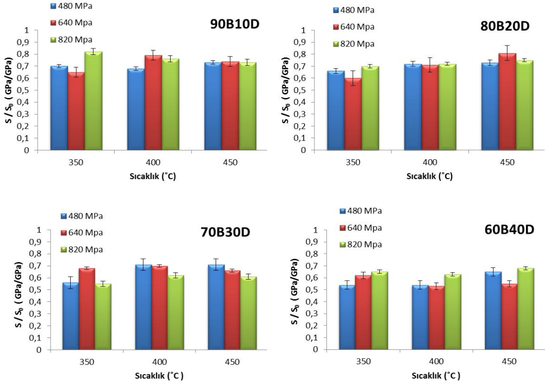
Şekil 4.16 Bağlı Sekant Modülü
