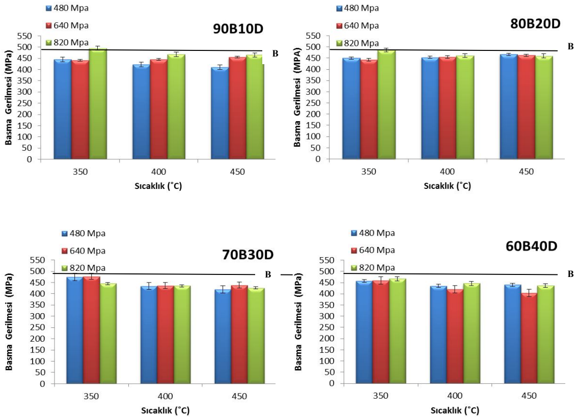
Şekil 4.13 Basma gerilmesi sonuçları
