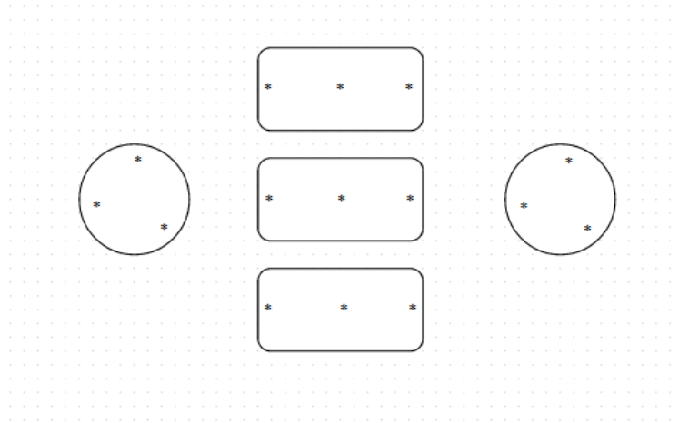
Şekil 3.45 Silindirik numune sertlik şeması
