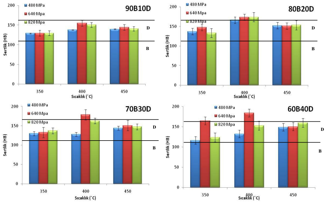
Şekil 4.5 Silindirik numunelerde Brinell sertlik değerleri
