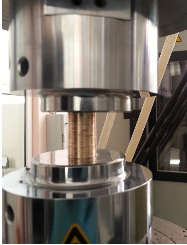
Şekil 3.54 Basma testi
