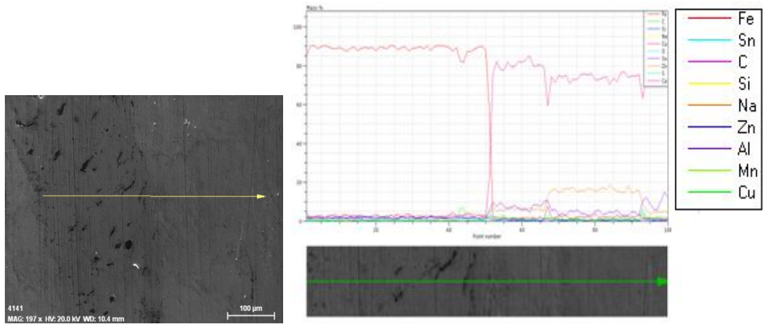
Şekil 3.14 Prizmatik numunenin EDX görüntüleri
