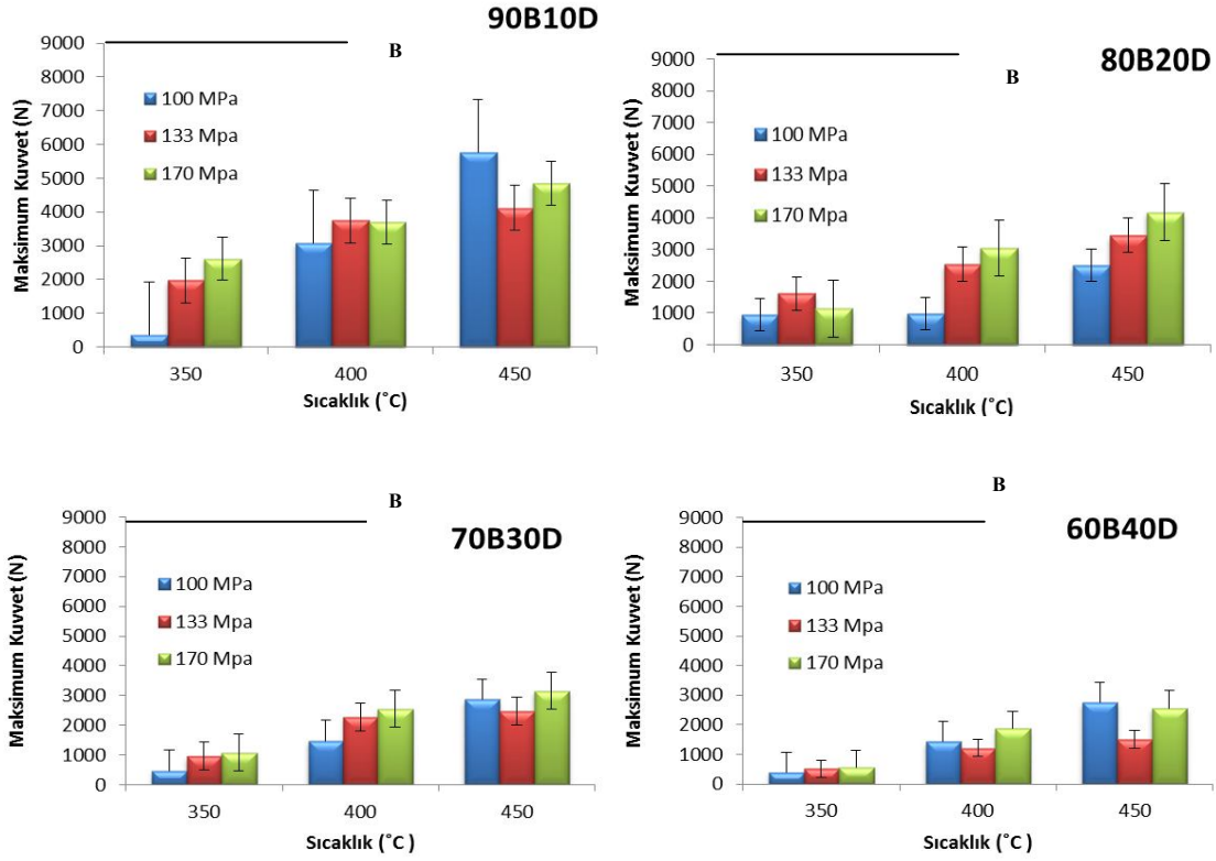
Şekil 4.24 Eğme deneyi sonuçları
