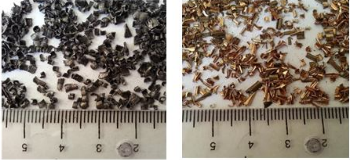
Şekil 3.32 GGG 40 ve CuSn10 talaşları
