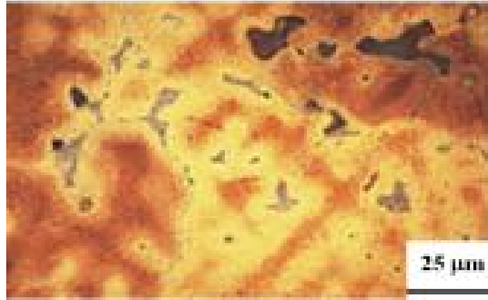
Şekil 3.10 CuSn10 mikro yapı (100X) ( www.mesmetal.com )
