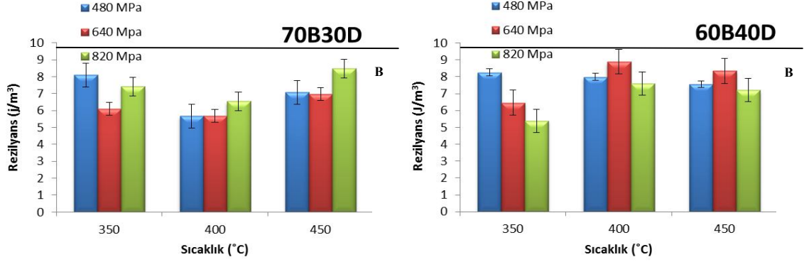
Şekil 4.14 Rezilyans modülü sonuçları
