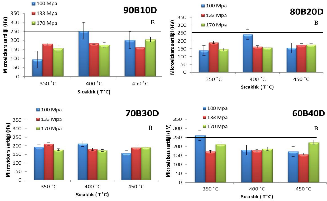
Şekil 4.8 Prizmatik numunelerde mikro vikers sertlik değerleri
