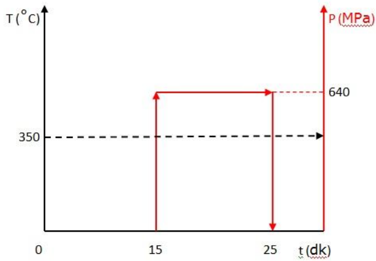
Şekil 3.36 Üretim grafiği
