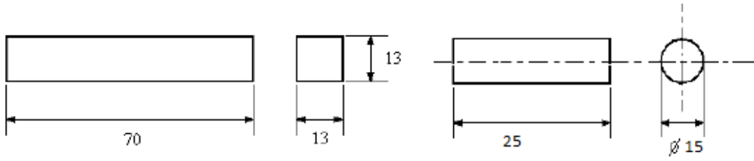
Şekil 3.39 Ham numune geometrileri
