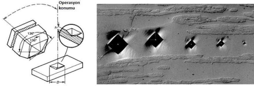
Şekil 3.49 Mikro Vickers piramit ve ucun numune üzerindeki görüntüsü (temsili)
