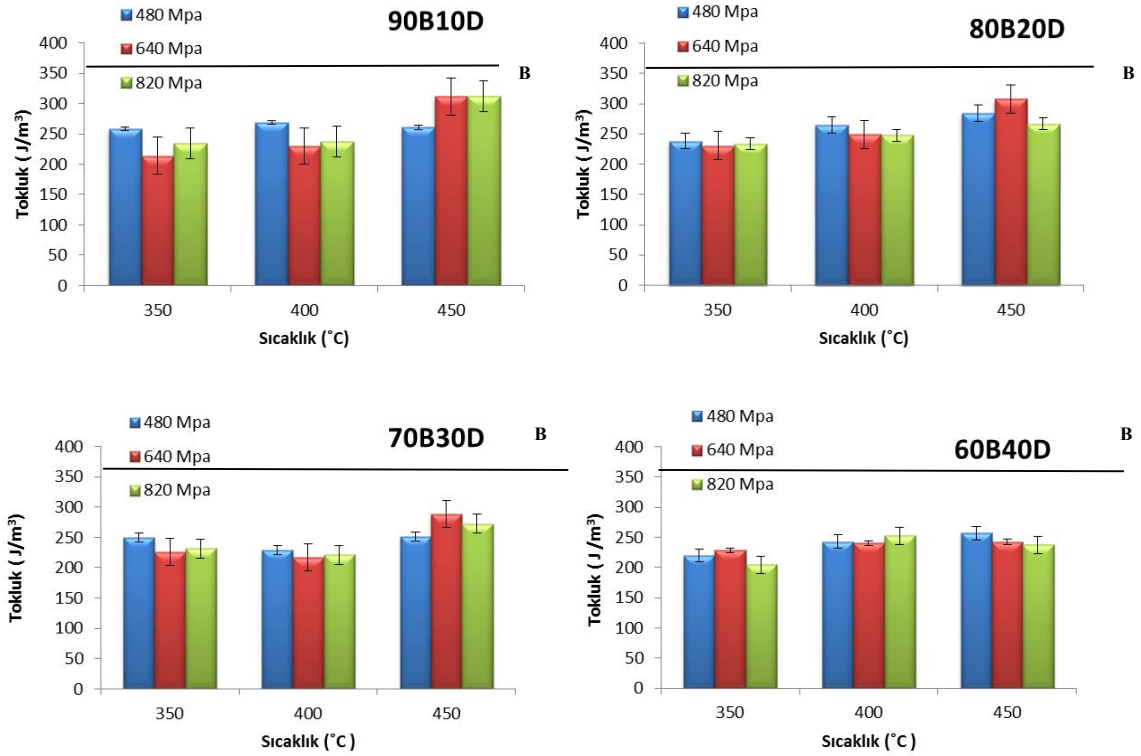
Şekil 4.15 Tokluk sonuçları
