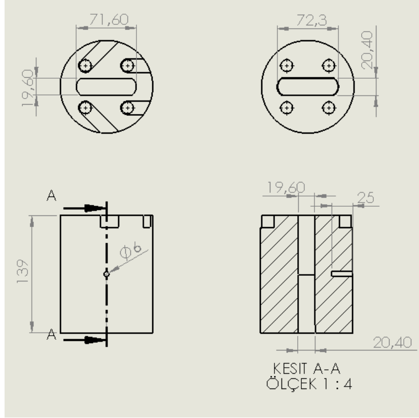
Şekil 3.21 Prizmatik dişi kalıp teknik resim
