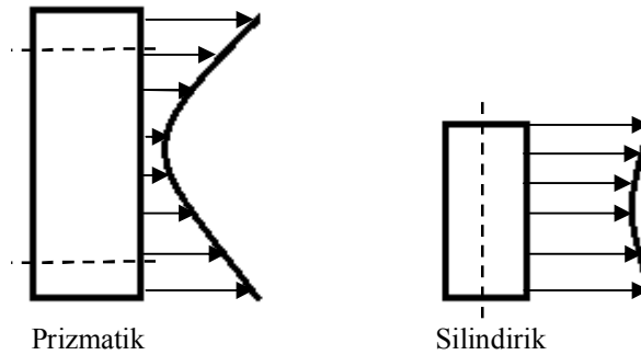
Şekil 4.18 Silindirik numune ve prizmatik numunenin sertlik profili
