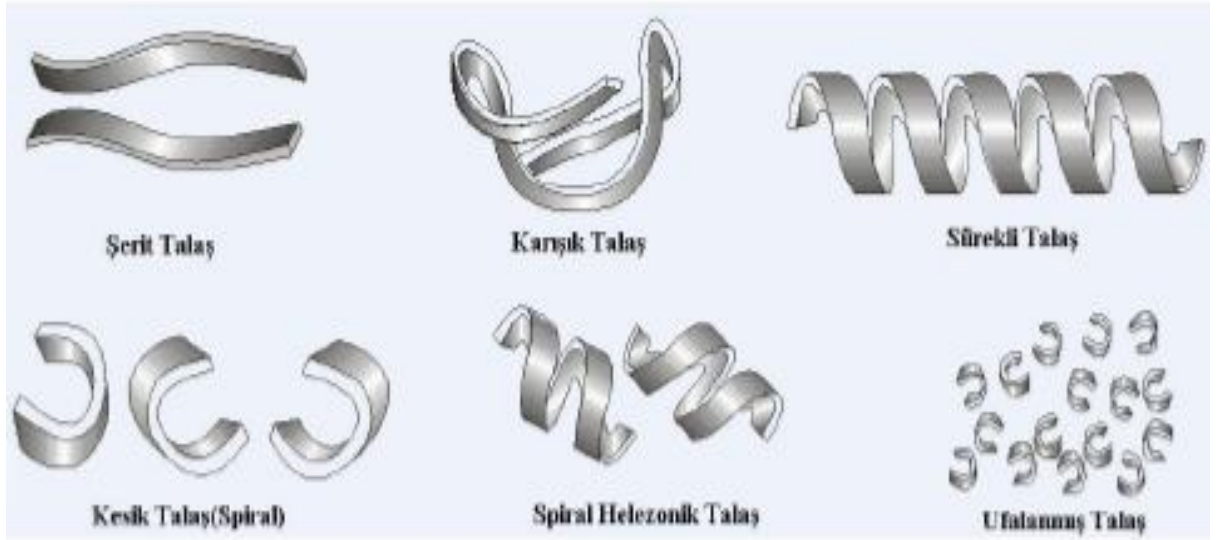
Şekil 3.8 Talaş şekilleri (Şahin, 2001)
