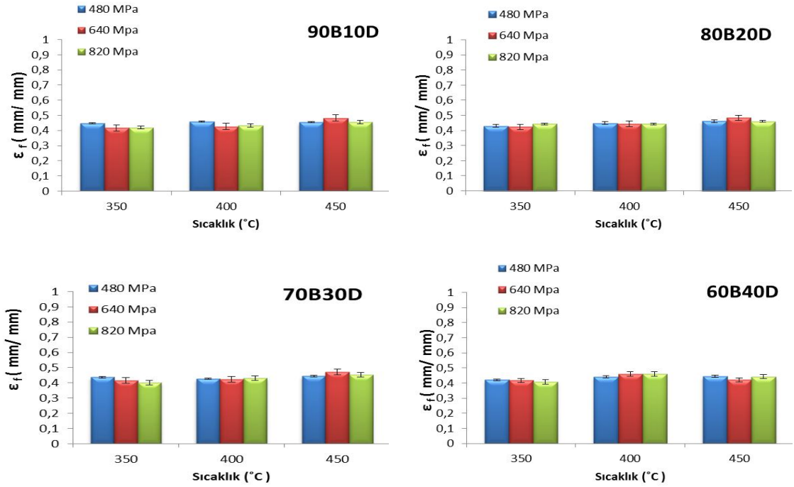
Şekil 4.17 Kırılma anındaki kısalma ( \epsilon_f ) grafikleri
