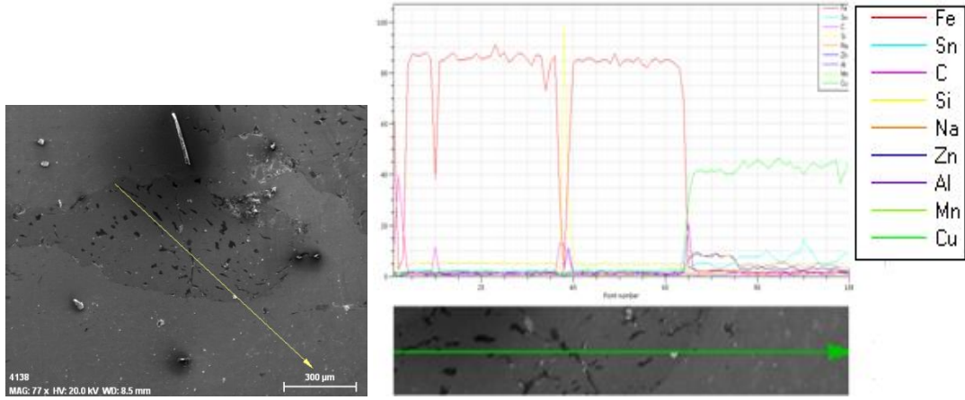
Şekil 3.14 Prizmatik numunenin EDX görüntüleri
