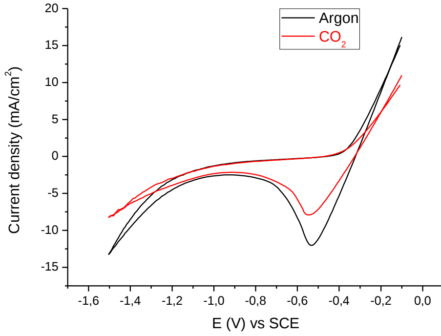
Ek 38. Pb çalışma elektrodu üzerinde argon atmosferindeki formik asit (—) ve formik asit içindeki doymuş \text{CO}_2 (—) çözeltisinin (-0.1, -1.5) V aralığında alınan dönüşümlü voltamogramı (%90 \text{HCOOH} , %10 \text{H}_2\text{O} , destek elektrolit: 0.2 M \text{KCOOH} , referans elektrot: SCE) (v: 100 mV/s)
