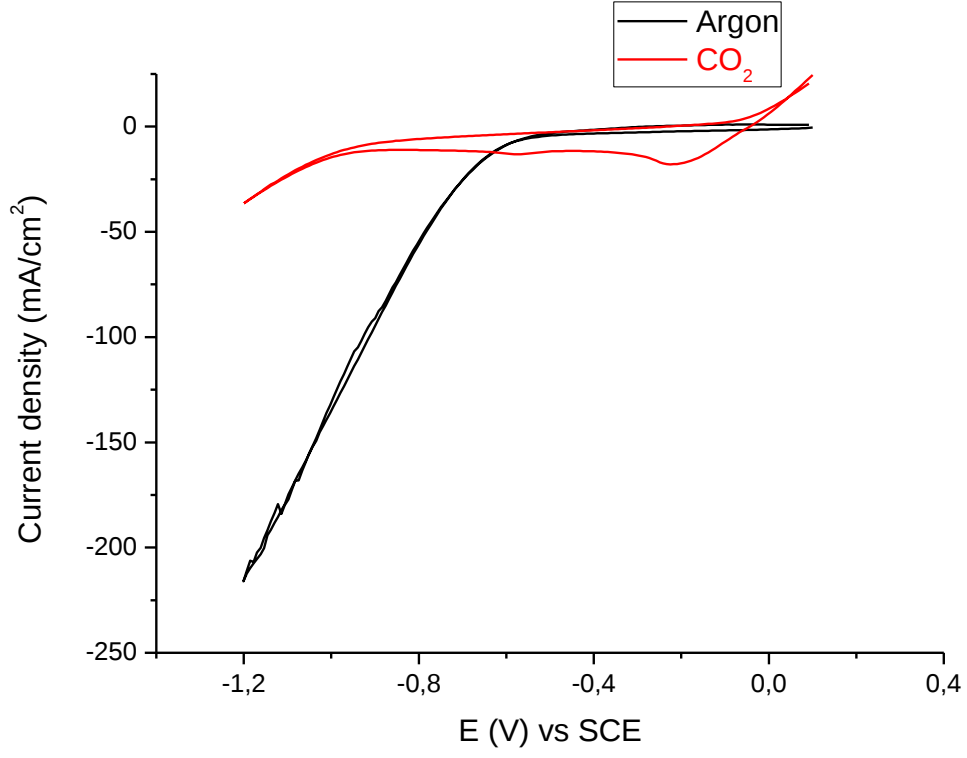
Ek 33. Cu çalışma elektrodu üzerinde argon atmosferindeki formik asit (—) ve formik asit içindeki doymuş \text{CO}_2 (—) çözeltisinin (0.1, -1.2) V aralığında alınan dönüşümlü voltamogramı (%90 \text{HCOOH} , %10 \text{H}_2\text{O} , destek elektrolit: 0.2 M \text{KCOOH} , referans elektrot: SCE) (v: 100 mV/s)
