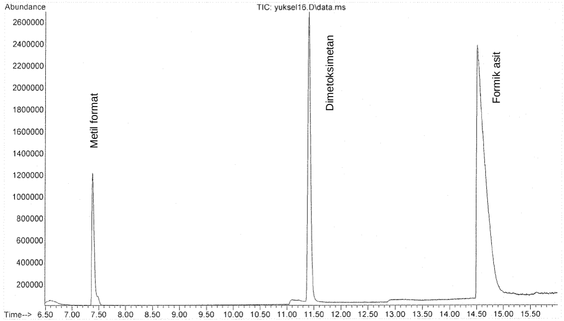
Şekil 6.45. Pb Elektrot – Metanol deneyinde yaklaşık 34,000 C yük saydıktan sonra alınan örneğin GCMS kromatogramı (Metanol kolondan ayırdıktan sonra alınan kromatogram).
