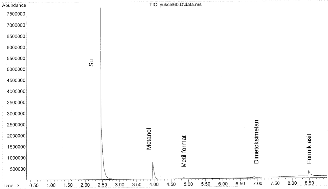
EK 25. Mo Kaplı Grafit Çubuk Elektrot – Metanol deneyinde yaklaşık 53,000 C yük saydıktan sonra alınan örneğin GCMS kromatogramı (Su piki dahil).
