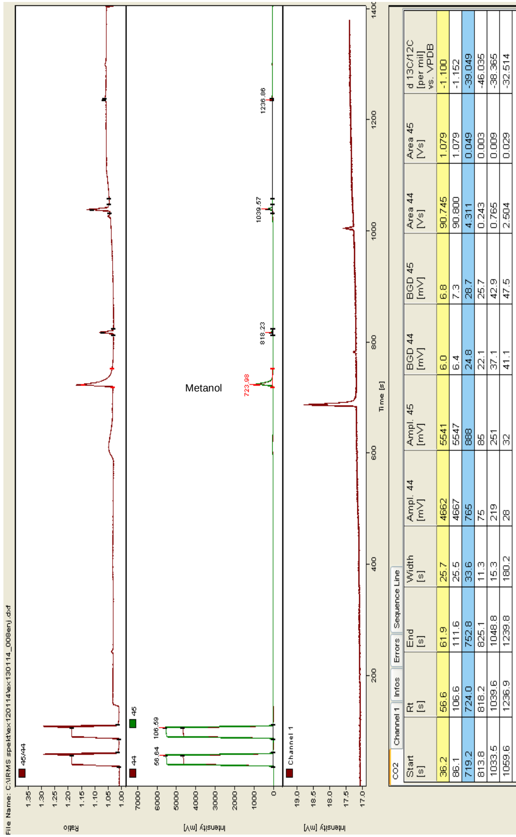
Şekil 6.31. Mo Kaplı Bakır Elektrot – Metanol deneyinde yaklaşık 25,000 C yük saydıktan sonra alınan örnekğin IRMS spektrumu.
