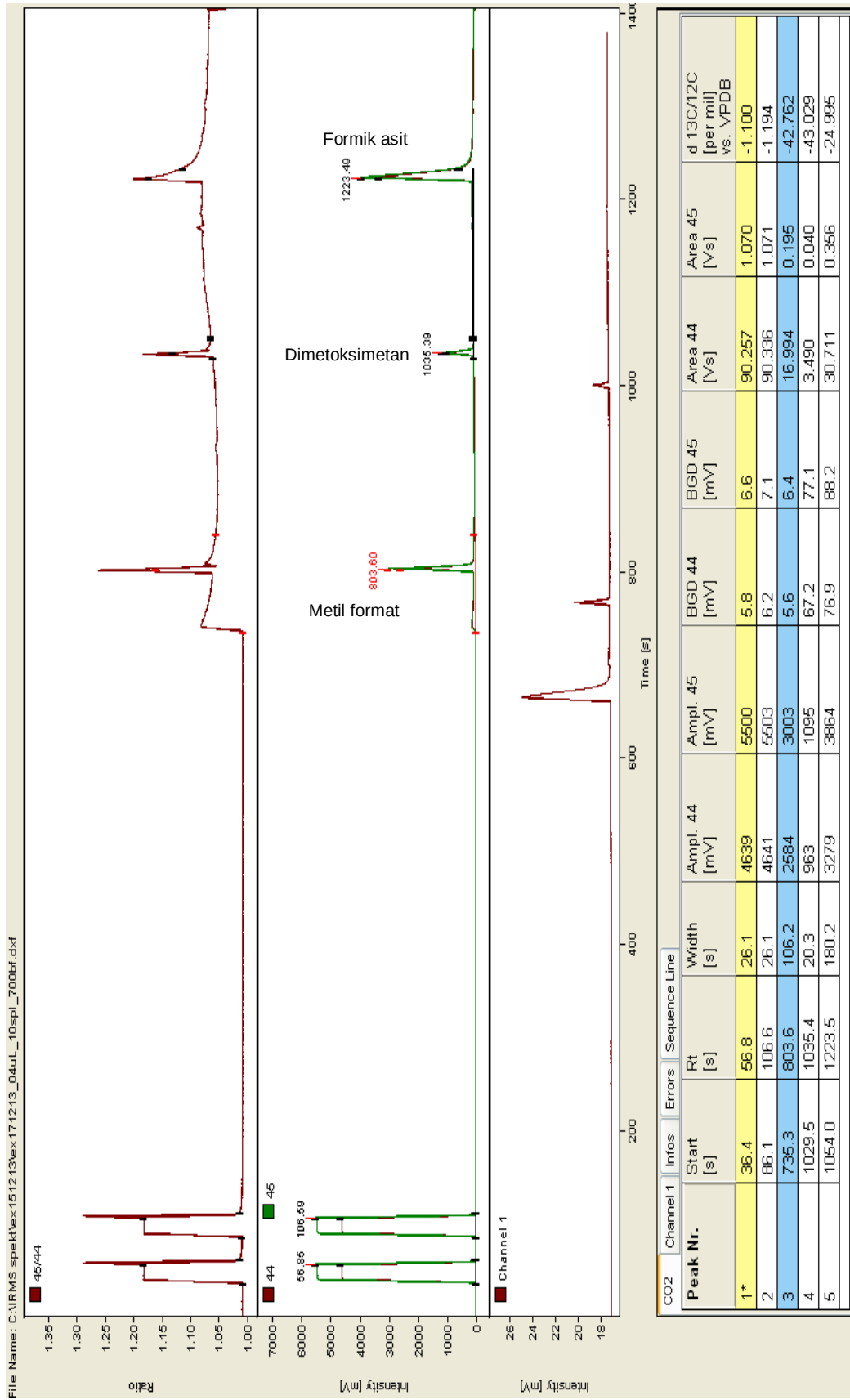
Şekil 6.23. Mo Kaplı Grafit Çubuk Elektrot – Metanol deneyinde yaklaşık 53,000 C yük saydıktan sonra alınan örnekğin IRMS spektrumu (Metanol kolondan ayrıldıktan sonra alınan spektrum).
