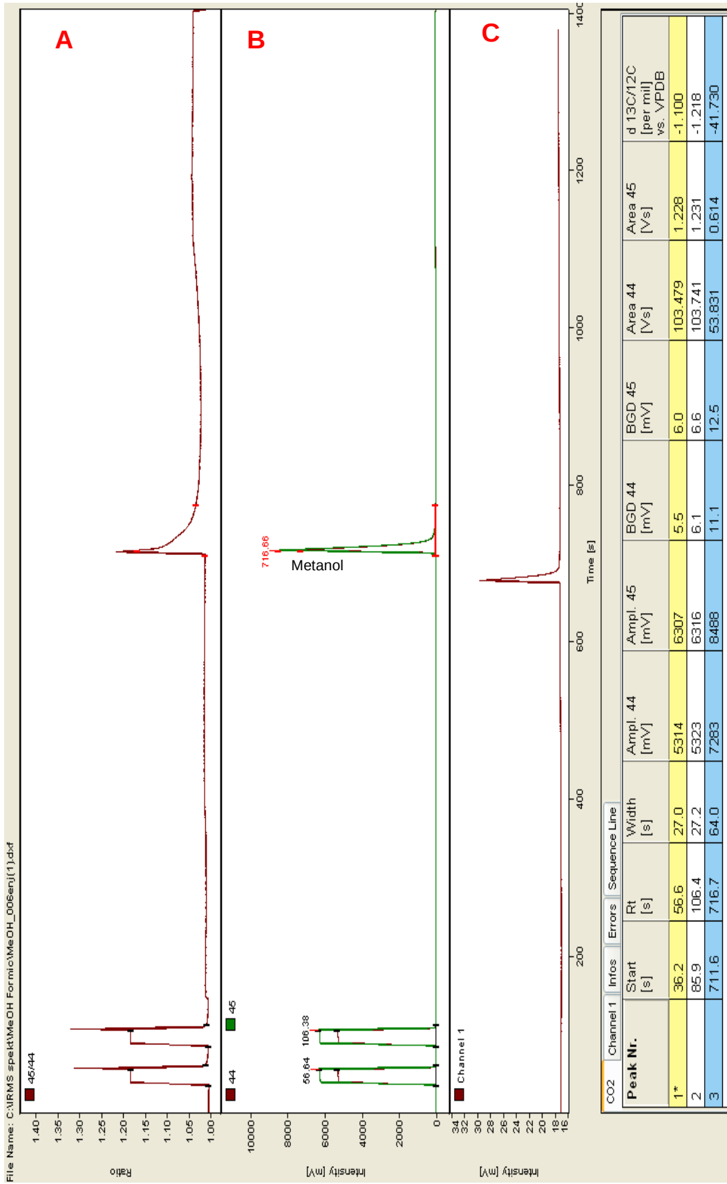
Ek 2. \delta^{13}\text{C} değeri - 41.730 olan metanole ait IRMS spektrumu ( A : IRMS 45/44 oran spektrumu, B : IRMS 44 ve 45 kütleleri için pik şiddetlerini gösteren spektrum, C : FID (Flame ionization dedector) spektrumu)
