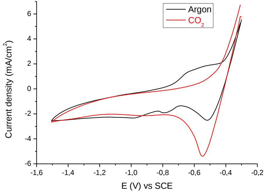
Ek 28. Pb çalışma elektrodu üzerinde argon atmosferindeki metanol (—) ve metanol içindeki doymuş CO 2 (—) çözeltisinin (-0.3, -1.5) V aralığında alınan dönüşümlü voltamogramı (%90 CH 3 OH, %10 H 2 O, destek elektrolit: 0.1 M NaClO 4 , referans elektrot: SCE) (v: 100 mV/s)
