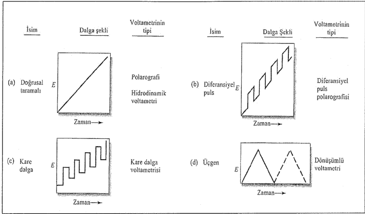
Şekil 4.1. Voltametrizde kullanılan potansiyel uyarma sinyalleri [47]
