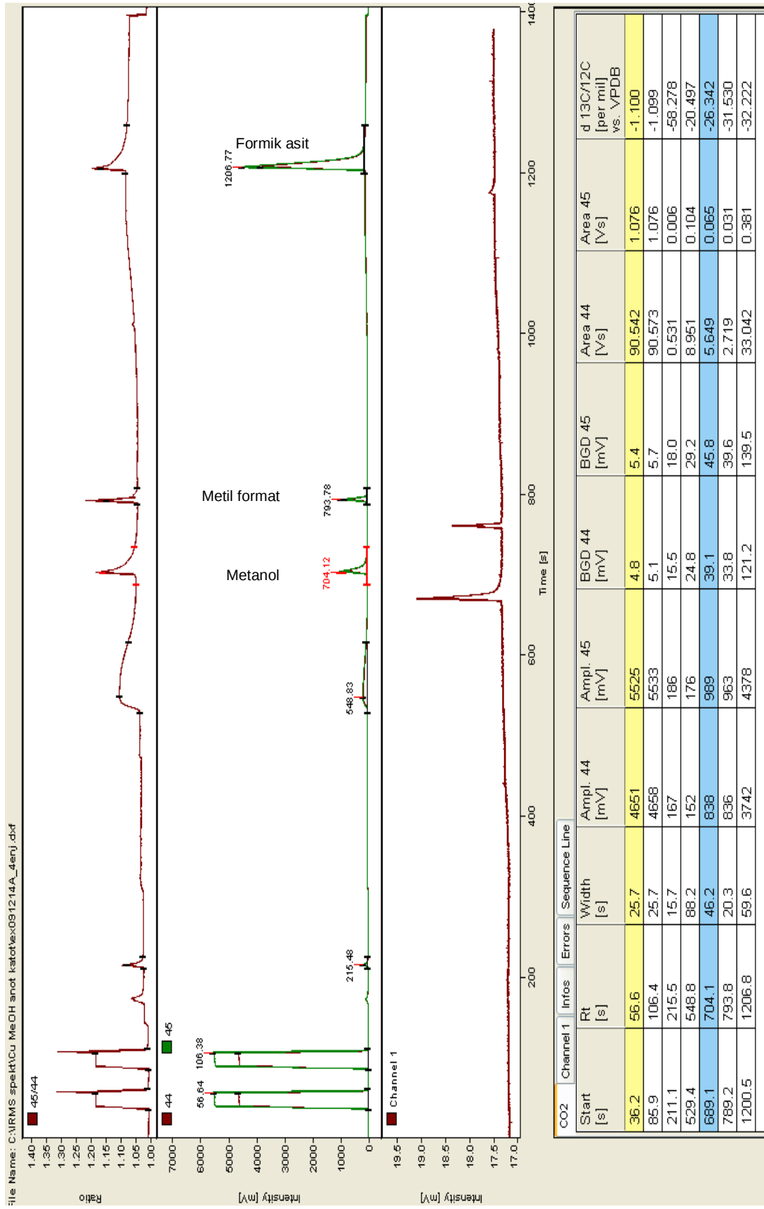
Ek 18. Cu Elektrot – Metanol deneyinde yaklaşık 104,000 C yük saydıktan sonra anolit çözeltiden alınan örneğin IRMS spektrumu
