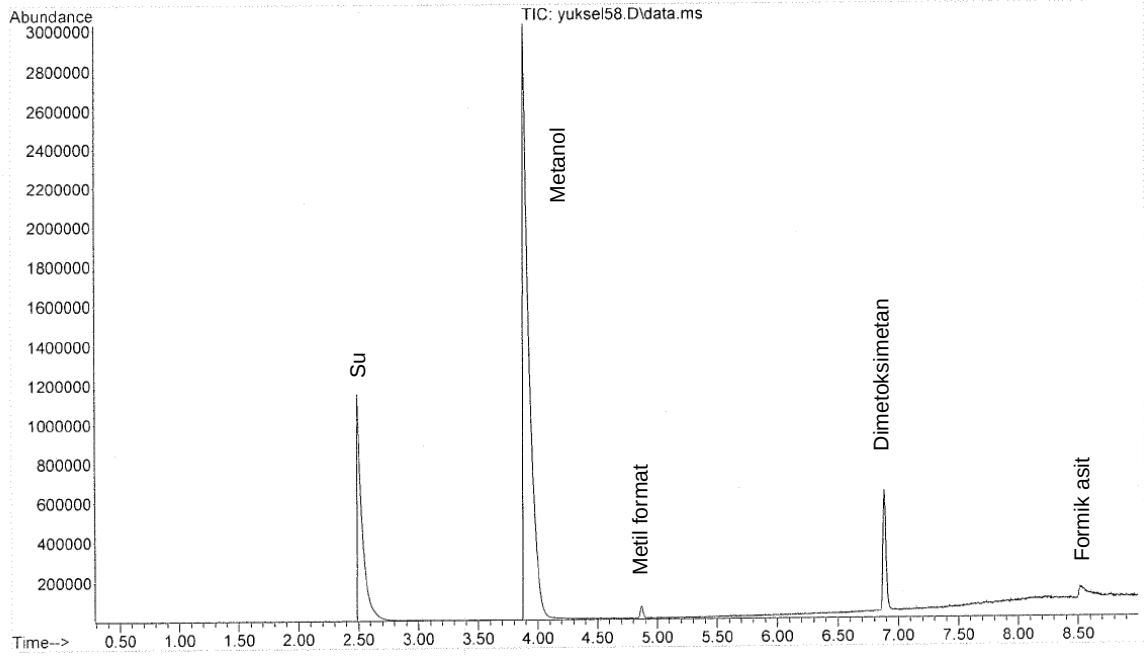
EK 24. Mo Kaplı Grafit Çubuk Elektrot – Metanol deneyinde yaklaşık 13,000 C yük saydıktan sonra alınan örneğin GCMS kromatogramı (Su piki dahil).
