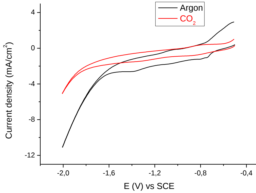
Ek 29. Pb çalışma elektrodu üzerinde argon atmosferindeki metanol (—) ve metanol içindeki doymuş CO 2 (—) çözeltisinin (-0.5, -2.0) V aralığında alınan dönüşümlü voltamogramı (%90 CH 3 OH, %10 H 2 O, destek elektrolit: 0.1 M NaClO 4 , referans elektrot: SCE) (v: 100 mV/s)
