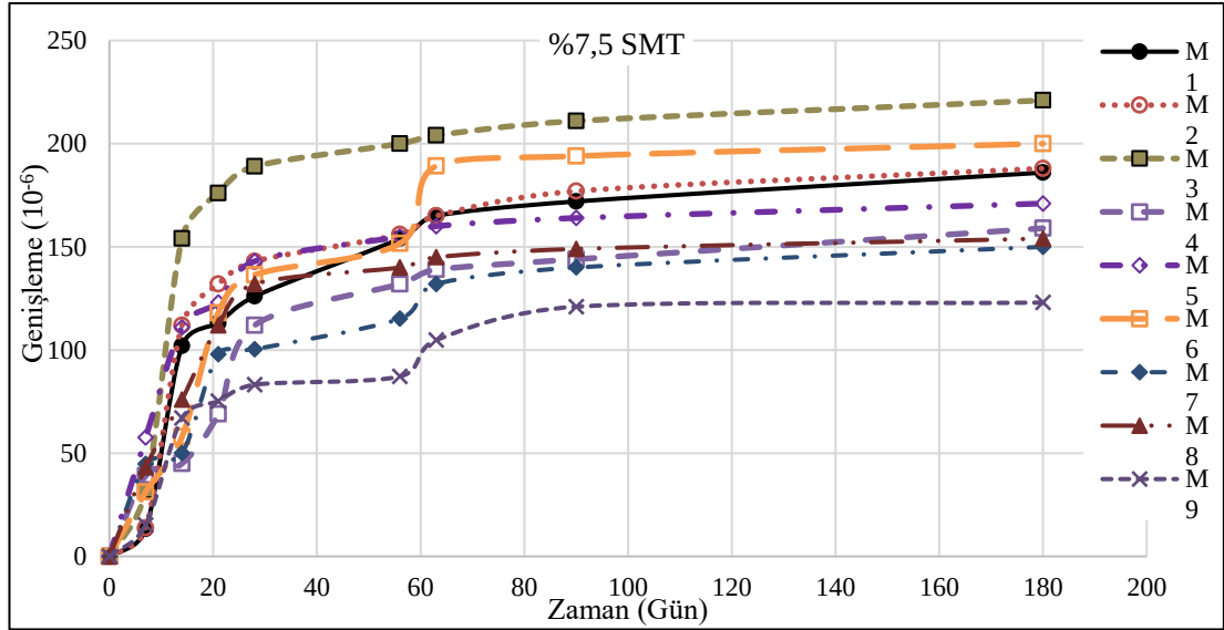
Şekil 4.37 %7,5 SMT kompozitlerin sülfat ( \text{MgSO}_4 ) direnci
