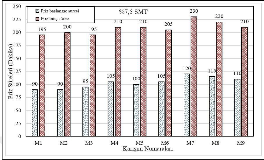
Şekil 4.1 %7,5 SMT kompozitlerin ilk ve son priz süreleri
