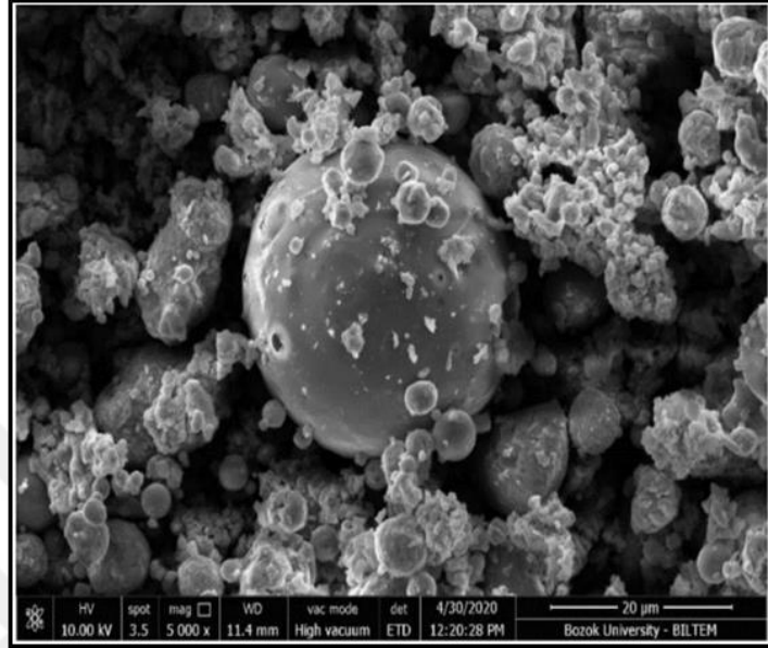
Şekil 2.3 C sınıfı uçucu kül (x5000) SEM görüntüsü (Kaya, 2016)
