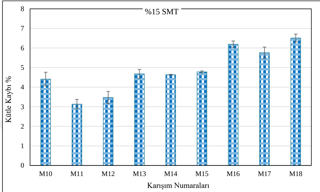
Şekil 4.32 180 gün boyunca HCl'ye maruz kalan %15 SMT kompozitlerin kütle kaybı %'si
