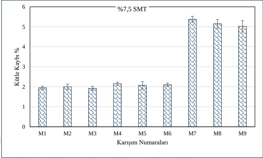
Şekil 4.39 180 gün boyunca NaCl'ye maruz kalan %7,5 SMT kompozitlerin ağırlık kaybı %'si
