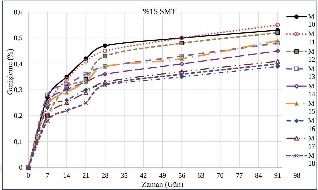
Şekil 4.46 %15 SMT kompozitlerin alkali-silika reaksiyon direnci
