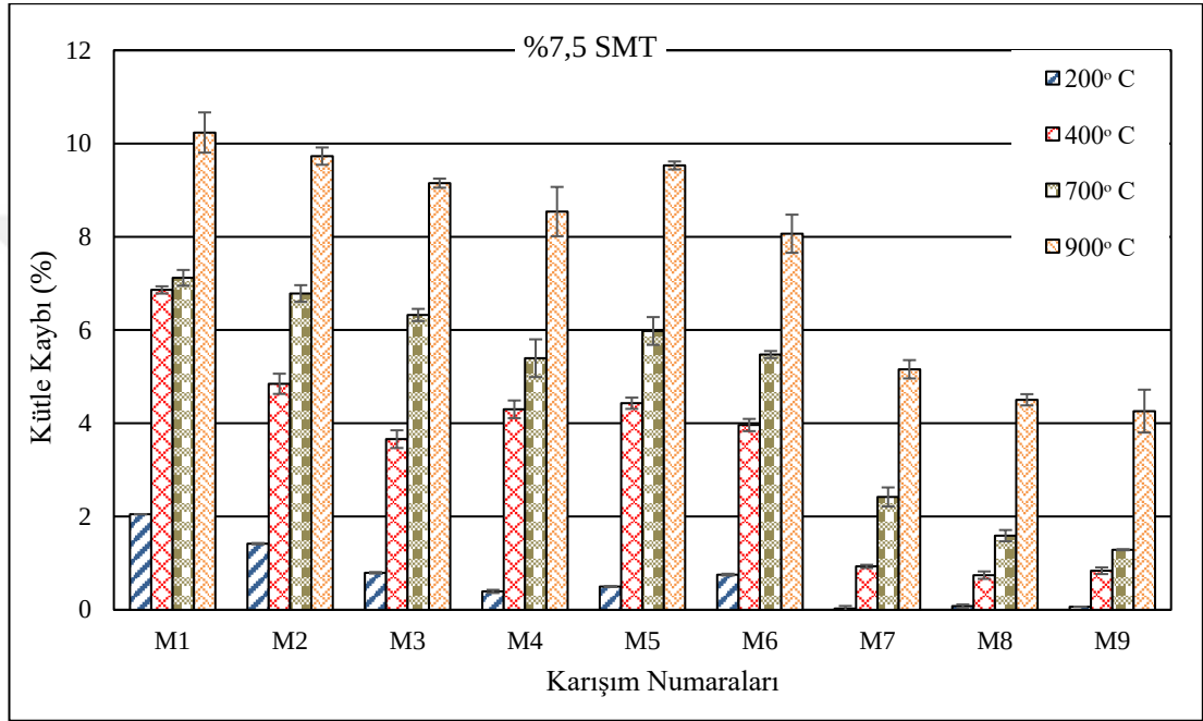
Şekil 4.15 Yüksek sıcaklığa maruz kalan %7,5 SMT kompozitlerin ağırlık kaybı %'si
