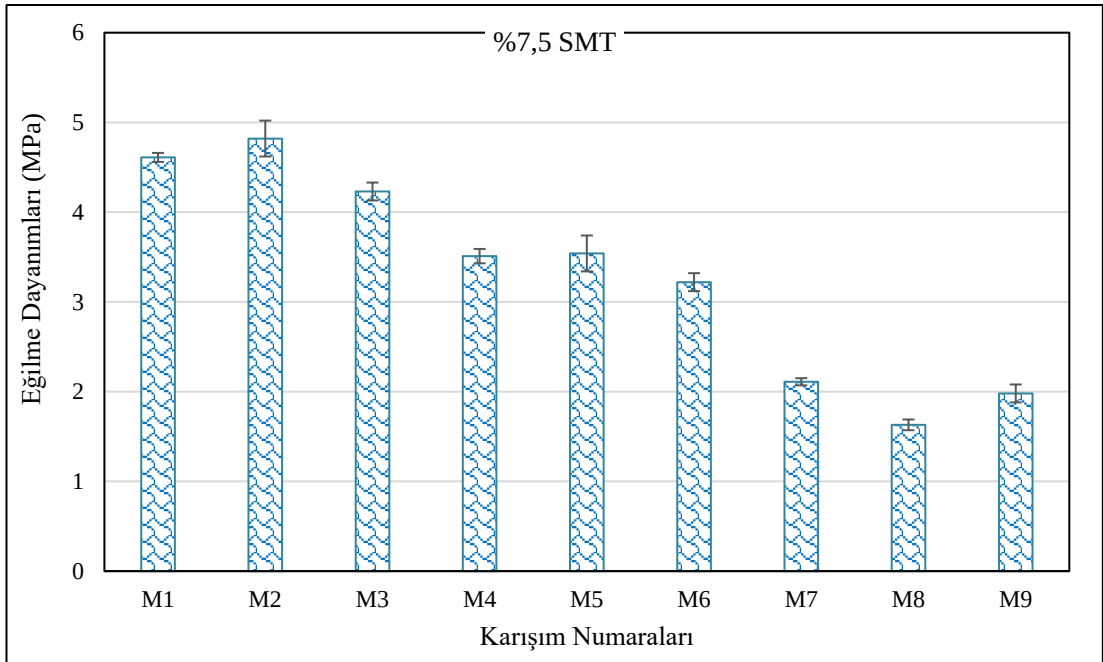
Şekil 4.35 180 gün boyunca HCl'ye maruz kalan %7,5 SMT kompozitlerin eğilme dayanımı
