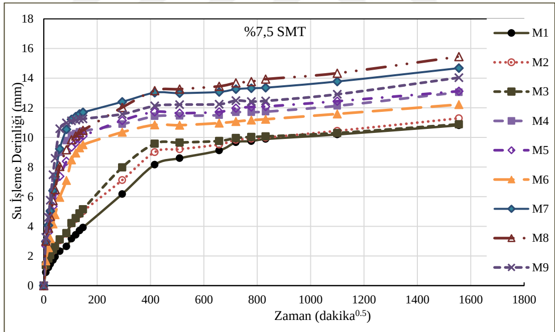
Şekil 4.29 %7,5 SMT kompozitlerin kapilerite özelliği
