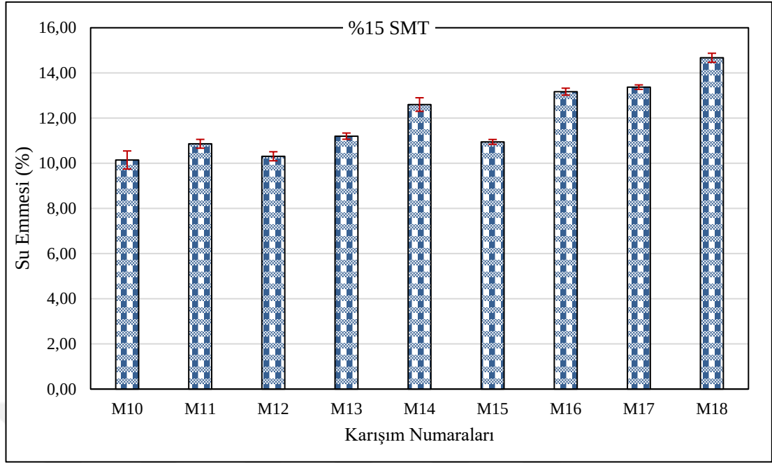
Şekil 4.10 %15 SMT kompozitlerin su emmesi
