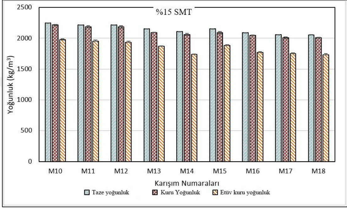
Şekil 4.6 %15 SMT kompozitlerin taze, sertleşmiş ve etüv kuru yoğunlukları
