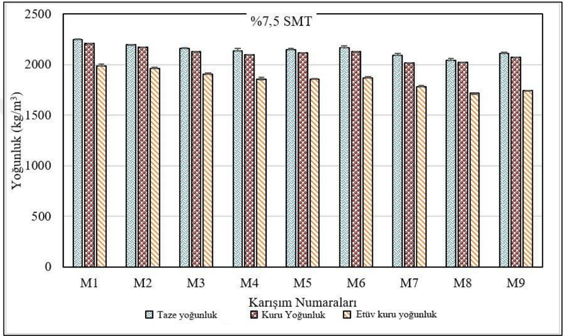
Şekil 4.5 %7,5 SMT kompozitlerin taze, sertleşmiş ve etüv kuru yoğunlukları
