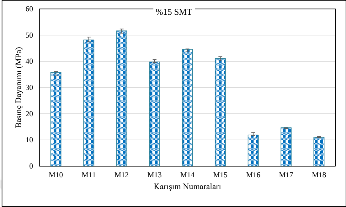
Şekil 4.34 180 gün boyunca HCl'ye maruz kalan %15 SMT kompozitlerin basınç dayanımı
