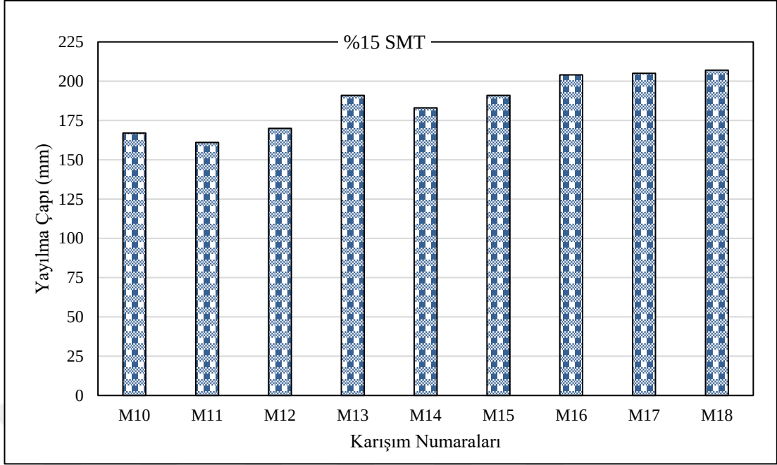
Şekil 4.4 %15 SMT kompozitlerin yayılma çapı
