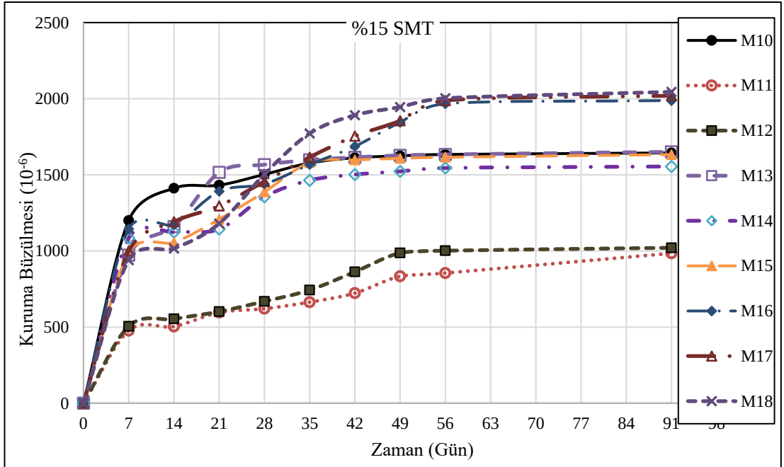
Şekil 4.28 %15 SMT kompozitlerin kuruma büzölmesi
