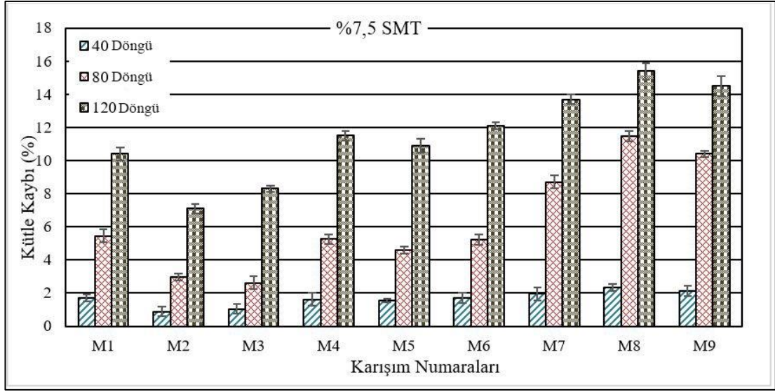
Şekil 4.21 Donma-çözölmeye maruz kalan %7,5 SMT kompozitlerin ağırlık kaybı %'si
