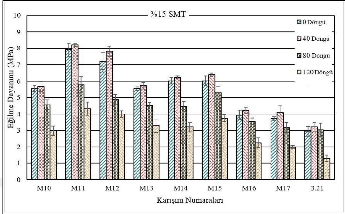
Şekil 4.26 Donma-çözölmeye maruz kalan %15 SMT kompozitlerin eğilme dayanımı
