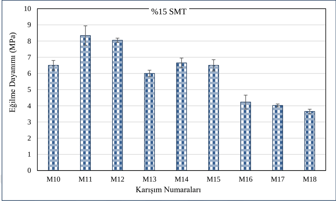
Şekil 4.44 180 gün boyunca NaCl'ye maruz kalan %15 SMT kompozitlerin eğilme dayanımı
