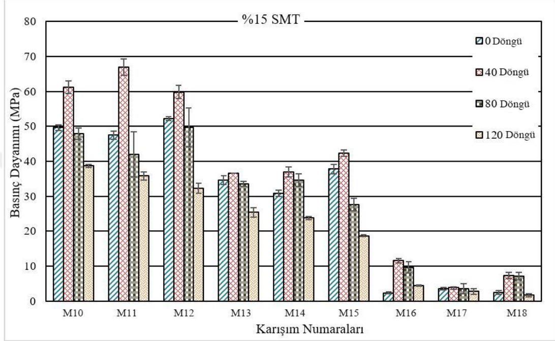
Şekil 4.24 Donma-çözölmeye maruz kalan %15 SMT kompozitlerin basınç dayanımı
