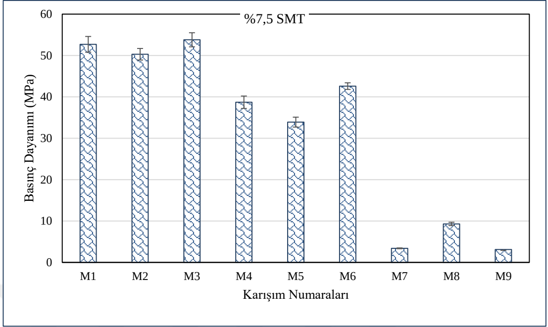
Şekil 4.41 180 gün boyunca NaCl'ye maruz kalan %7,5 SMT kompozitlerin basınç dayanımı
