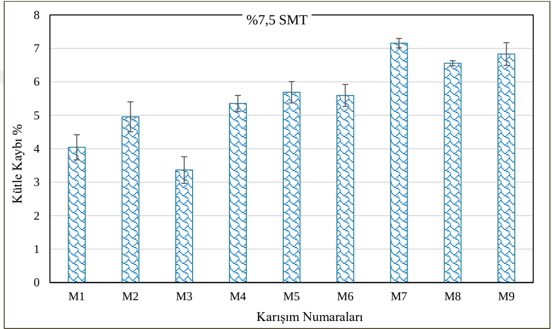
Şekil 4.31 180 gün boyunca HCl'ye maruz kalan %7,5 SMT kompozitlerin kütle kaybı %'si
