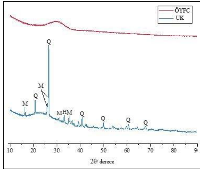
Şekil 3.1 YFC ve UK'nin XRD modeli (Q:Quartz, M:Mullite; H:Hematit)
