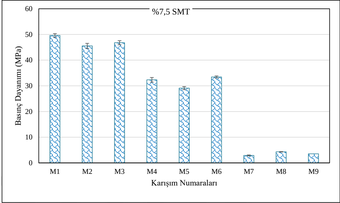
Şekil 4.33 180 gün boyunca HCl'ye maruz kalan %7,5 SMT kompozitlerin basınç dayanımı
