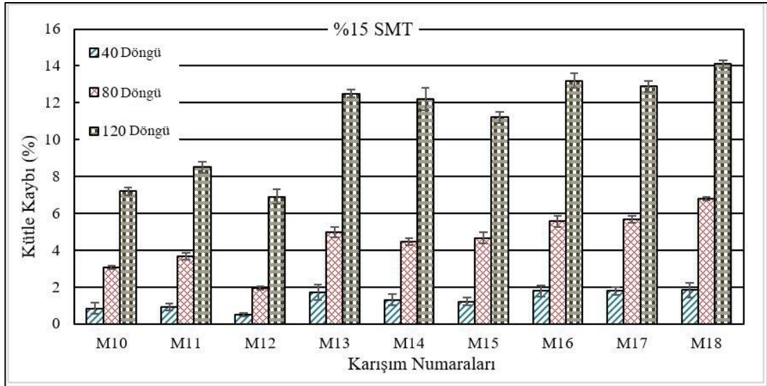
Şekil 4.22 Donma-çözölmeye maruz kalan %15 SMT kompozitlerin ağırlık kaybı %'si
