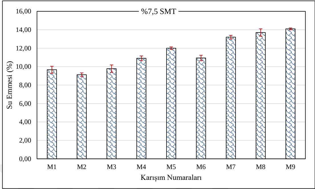
Şekil 4.9 %7,5 SMT kompozitlerin su emmesi
