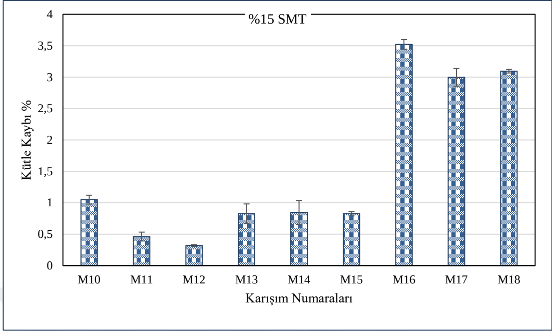
Şekil 4.40 180 gün boyunca NaCl'ye maruz kalan %15 SMT kompozitlerin ağırlık kaybı %'si
