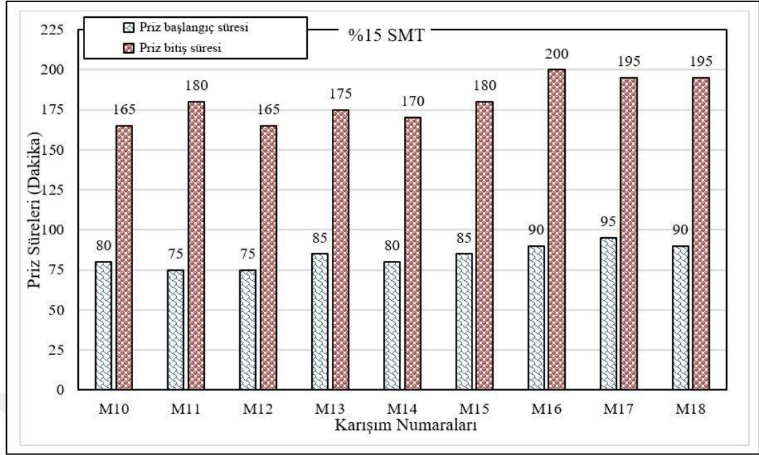
Şekil 4.2 %15 SMT kompozitlerin ilk ve son priz süreleri
