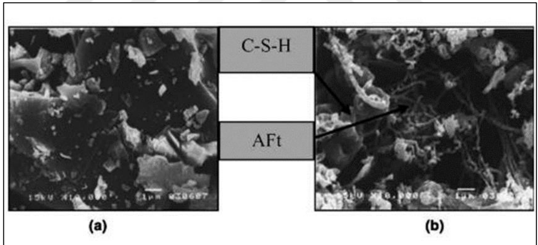
Şekil 2.9 Mikroskop altı görüntüsü. (a) Portland çimentosu ve (b) çamur tozu (Chatveera vd., 2006)
