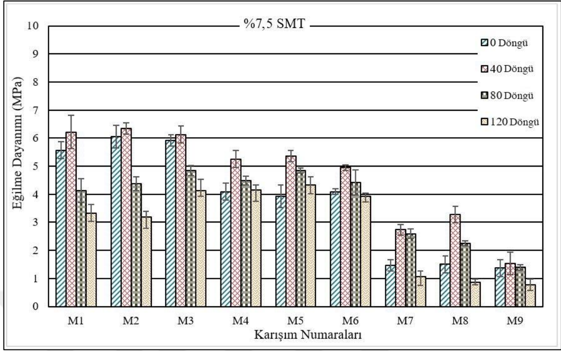
Şekil 4.25 Donma-çözölmeye maruz kalan %7,5 SMT kompozitlerin eğilme dayanımı
