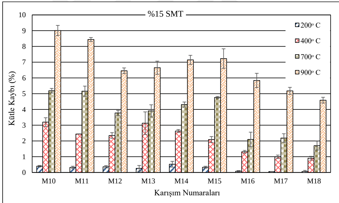
Şekil 4.16 Yüksek sıcaklığa maruz kalan %15 SMT kompozitlerin ağırlık kaybı %'si
