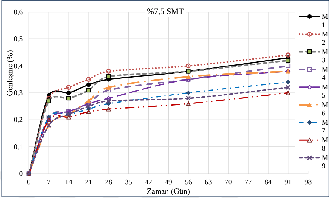
Şekil 4.45 %7,5 SMT kompozitlerin alkali-silika reaksiyon direnci
