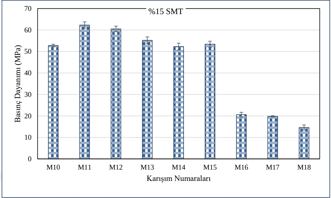
Şekil 4.42 180 gün boyunca NaCl'ye maruz kalan %15 SMT kompozitlerin basınç dayanımı
