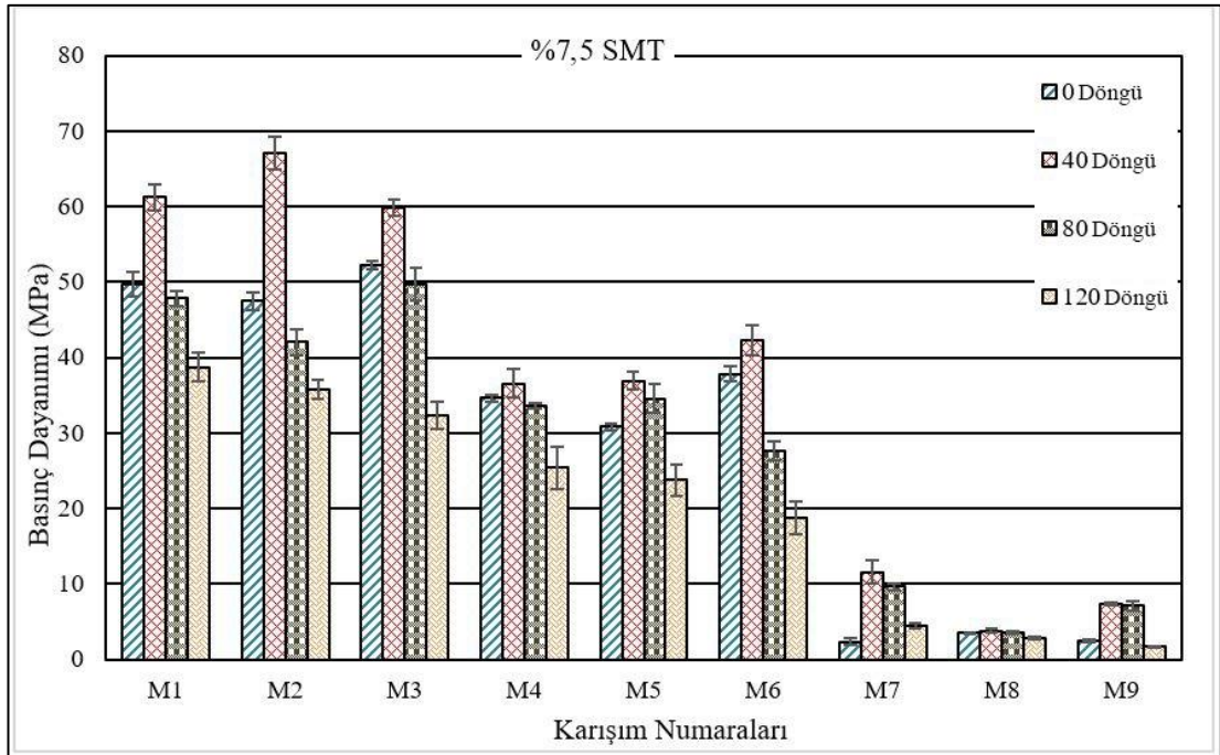
Şekil 4.23 Donma-çözülmeye maruz kalan %7,5 SMT kompozitlerin basınç dayanımı
