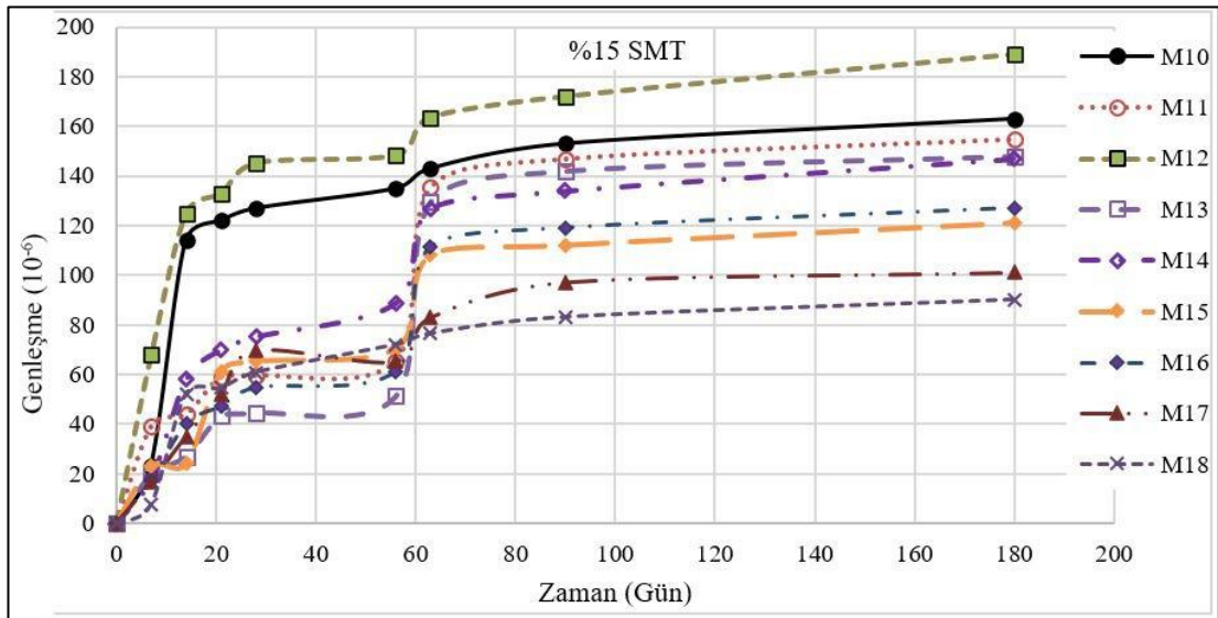
Şekil 4.38 %15 SMT kompozitlerin sülfat ( \text{MgSO}_4 ) direnci
