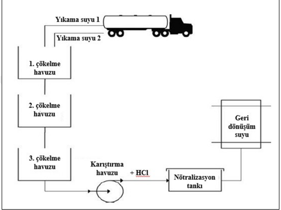
Şekil 2.7 Hazır beton tesisinde yıkama suyunun geri kazanımı işlemi (Tsimas ve Zervaki, 2011)
