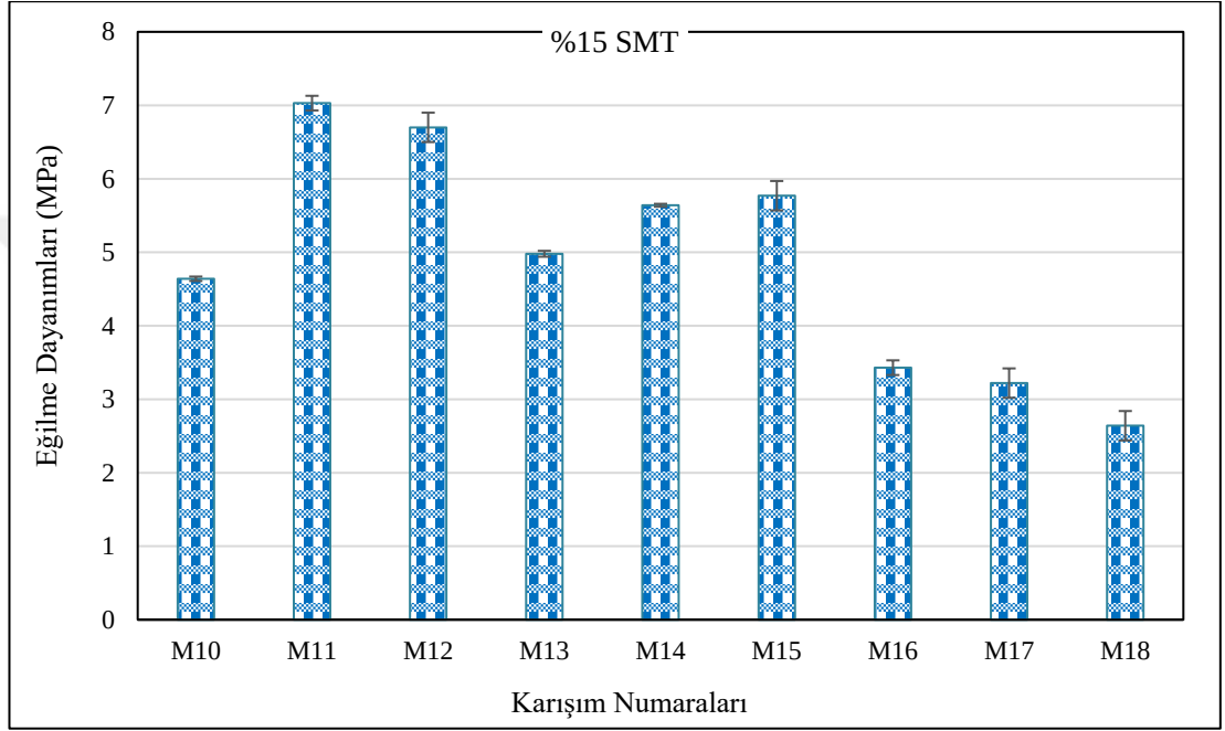
Şekil 4.36 180 gün boyunca HCl'ye maruz kalan %15 SMT kompozitlerin eğilme dayanımı
