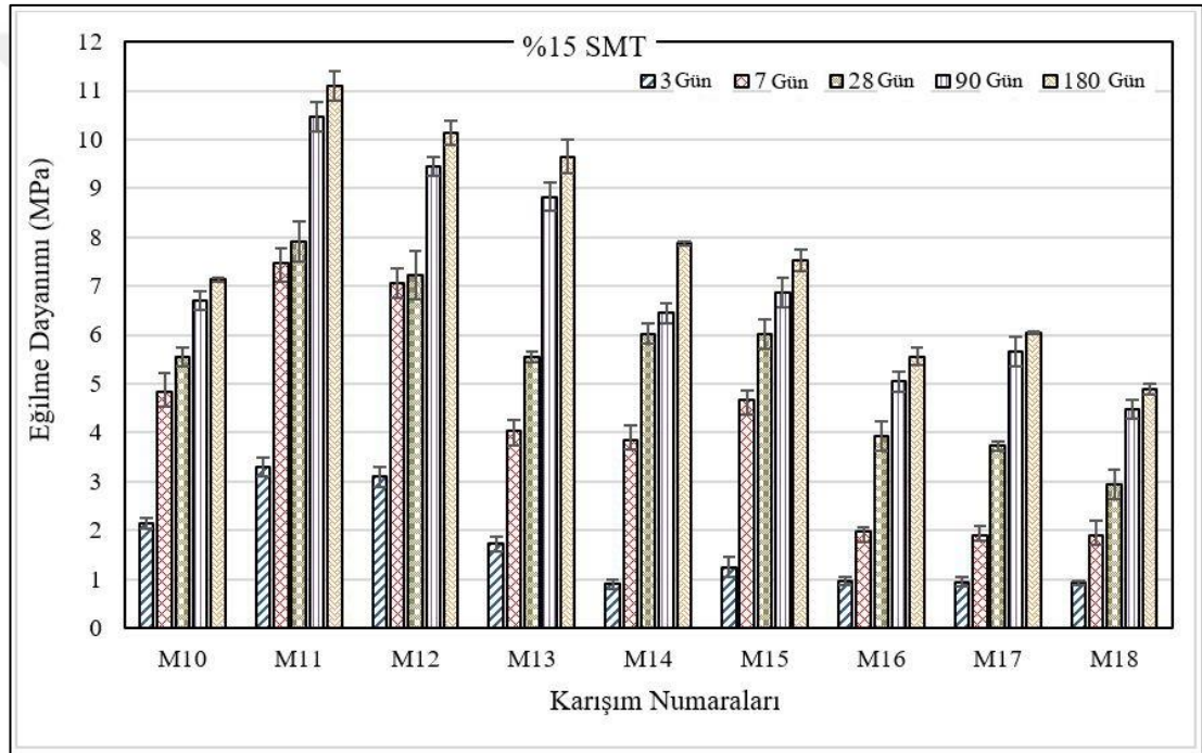
Şekil 4.14 %15 SMT kompozitlerin eğilme dayanımı ve standart sapması
