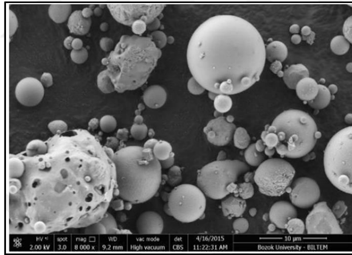
Şekil 2.5 Soma C sınıfı uçucu külünün SEM görüntüsü (x8000), (Kaya, 2016)
