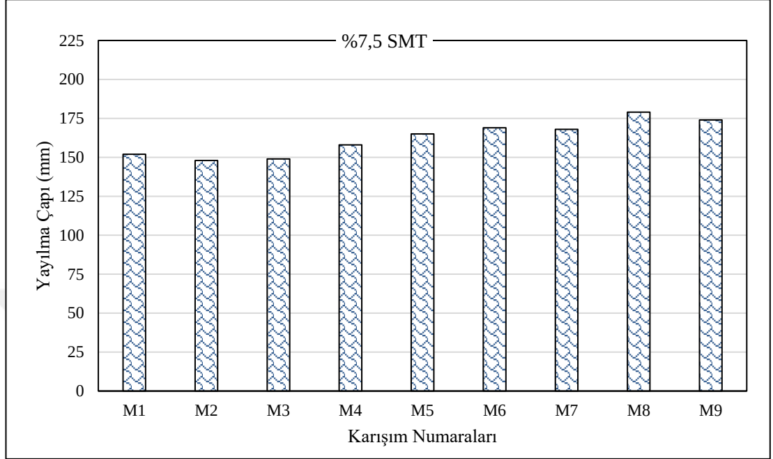
Şekil 4.3 %7,5 SMT kompozitlerin yayılma çapı
