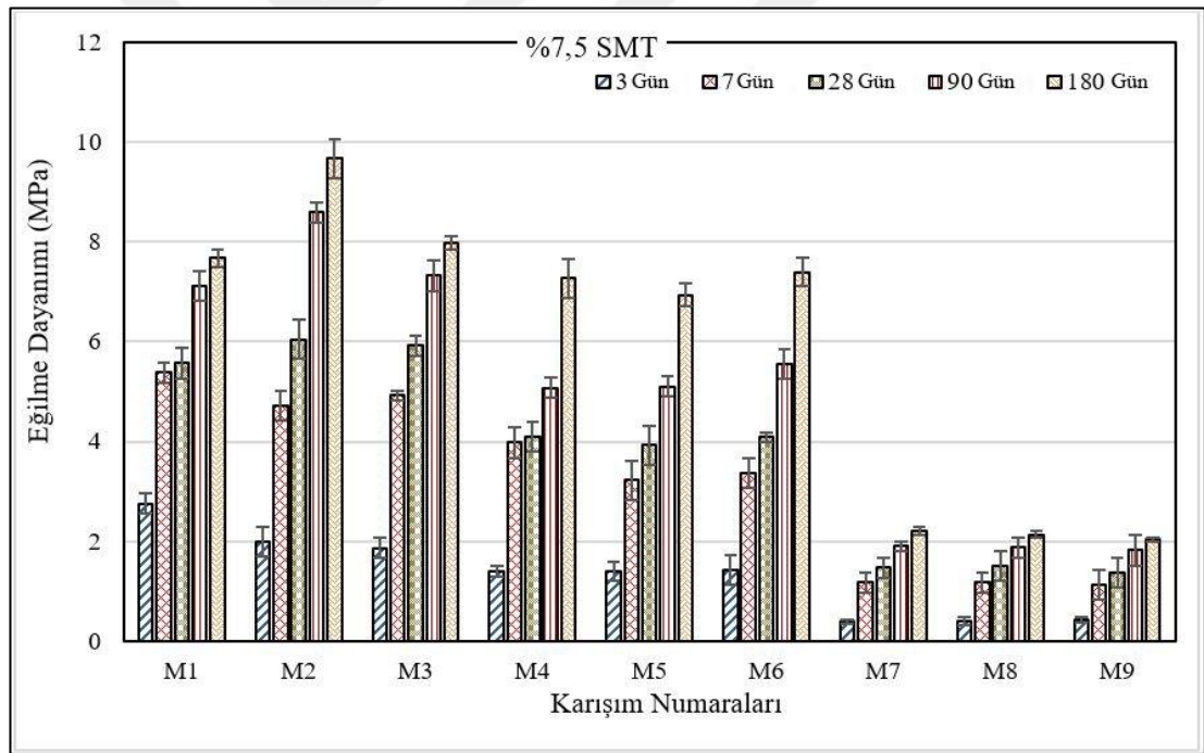
Şekil 4.13 %7,5 SMT kompozitlerin eğilme dayanımı ve standart sapması
