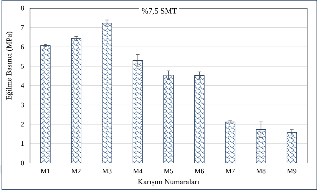
Şekil 4.43 180 gün boyunca NaCl'ye maruz kalan %7,5 SMT kompozitlerin eğilme dayanımı
