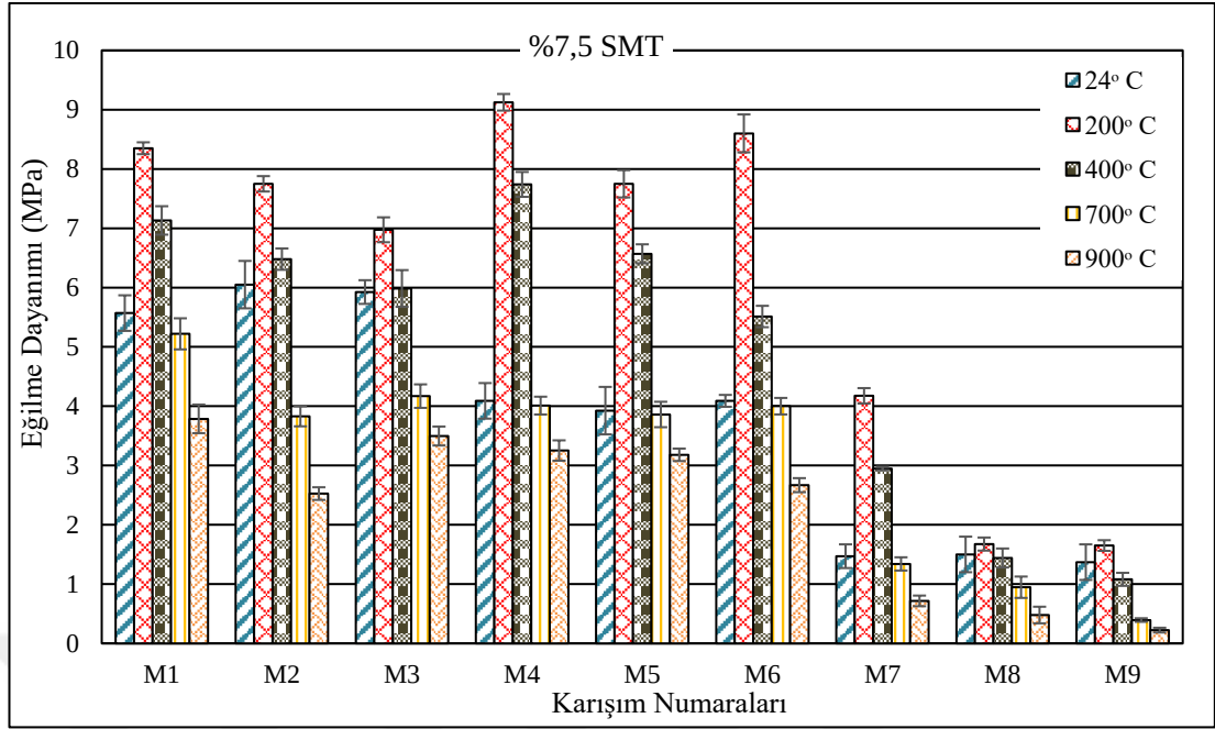
Şekil 4.19 Yüksek sıcaklığa maruz kalan %7,5 SMT kompozitlerin eğilme dayanımı
