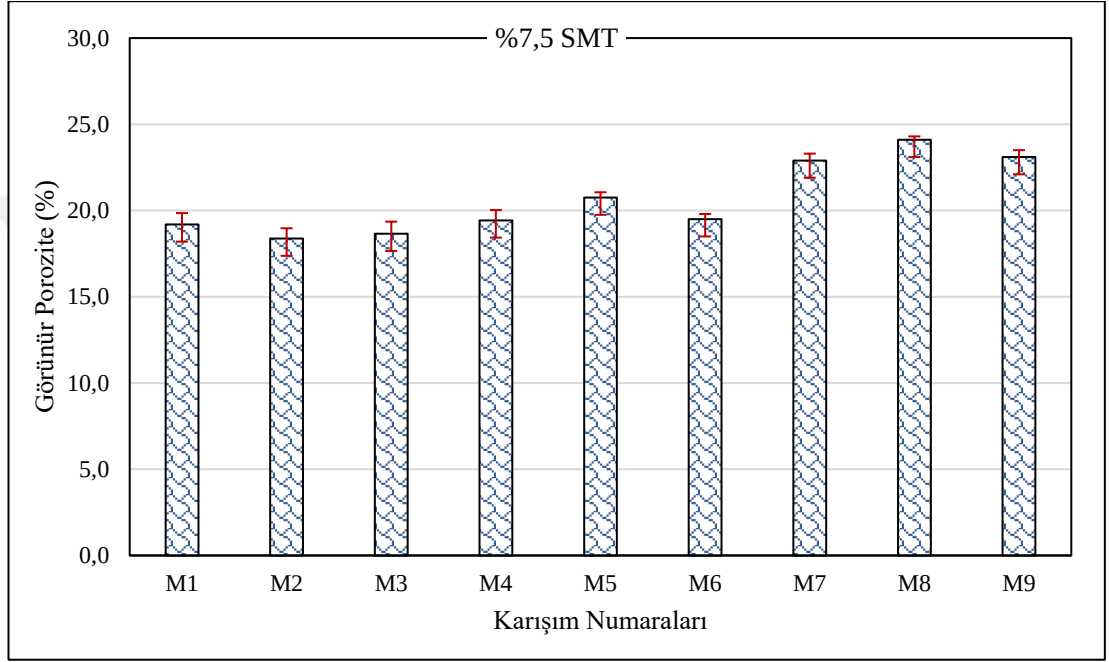
Şekil 4.7 %7,5 SMT kompozitlerin görünür poroziteleri
