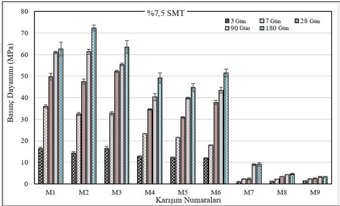
Şekil 4.11 %7,5 SMT kompozitlerin basınç dayanımı
