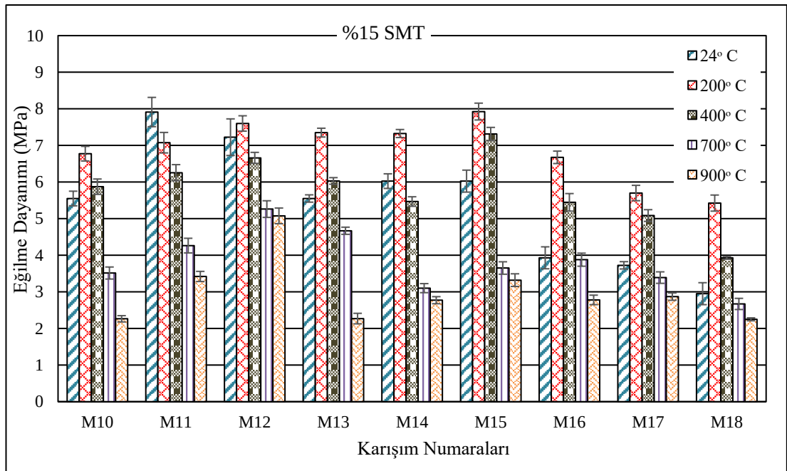
Şekil 4.20 Yüksek sıcaklığa maruz kalan %15 SMT kompozitlerin eğilme dayanımı
