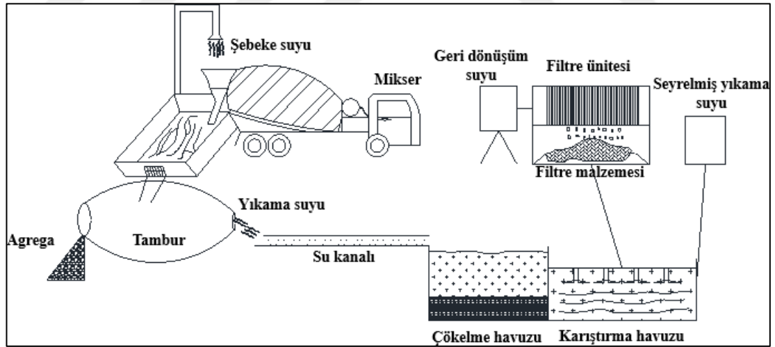
Şekil 2.6 Türkiye’de bir hazır beton tesisinde geri dönüşüm sistemi
