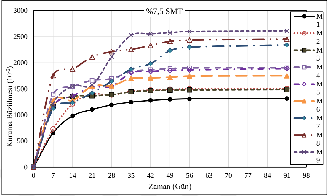
Şekil 4.27 %7,5 SMT kompozitlerin kuruma büzülmesi
