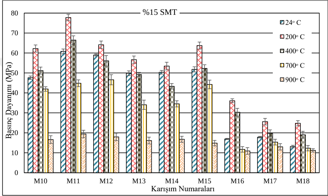
Şekil 4.18 Yüksek sıcaklığa maruz kalan %15 SMT kompozitlerin basınç dayanımı
