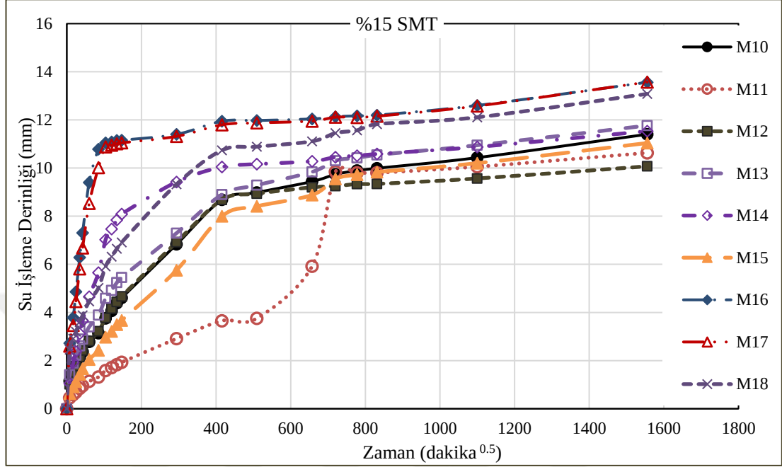
Şekil 4.30 %15 SMT kompozitlerin kapilerite özelliği
