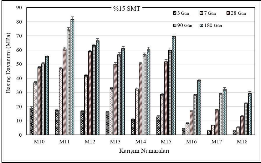
Şekil 4.12 %15 SMT kompozitlerin basınç dayanımı ve standart sapması
