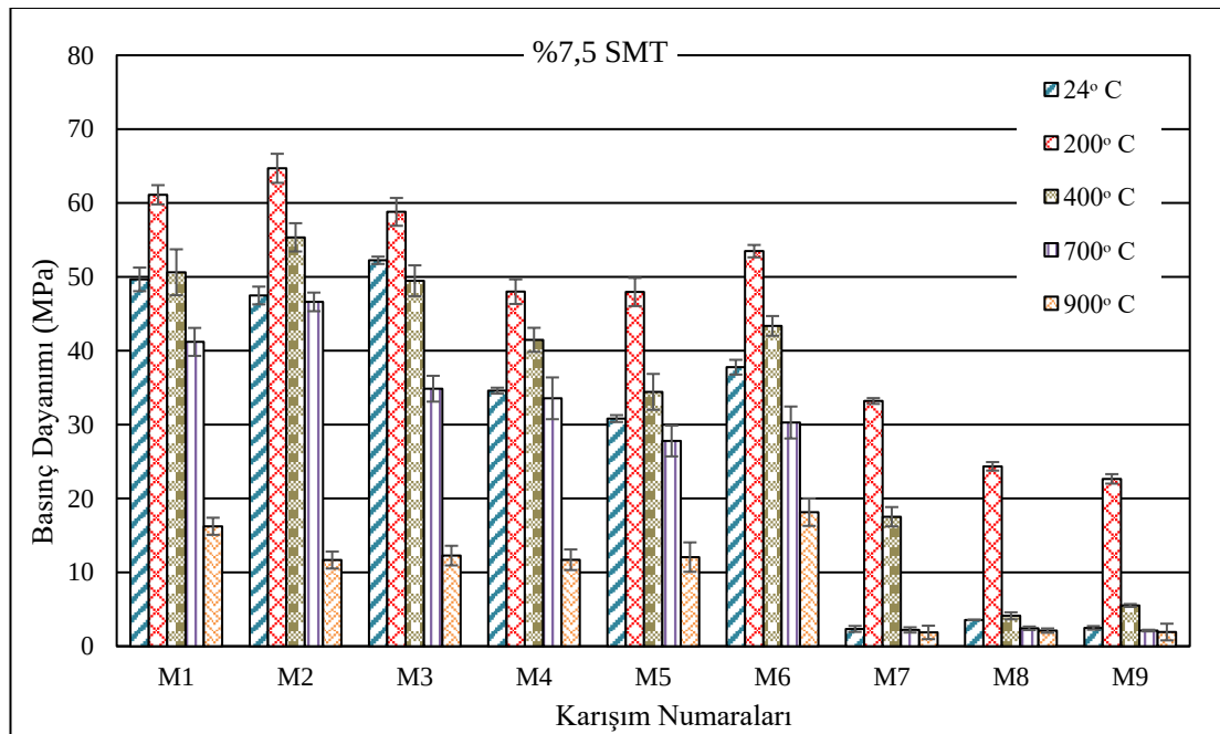
Şekil 4.17 Yüksek sıcaklığa maruz kalan %7,5 SMT kompozitlerin basınç dayanımı
