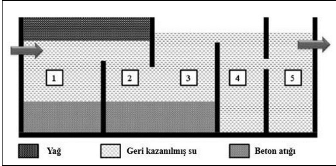
Şekil 2.8 Çökeltme havuzu yapısı (Vieira ve de Figueiredo, 2016)
