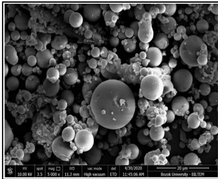
Şekil 2.4 F sınıfı uçucu kül (x5000) SEM görüntüsü (Kaya, 2016)
