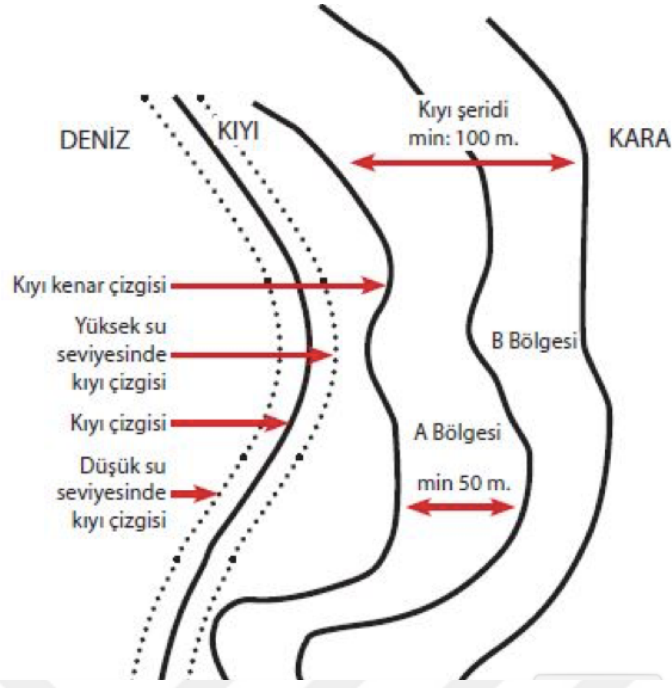
Şekil 2.10. Kıyı özellikleri (Kutlu, 2021).
