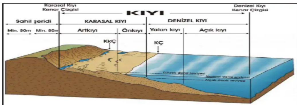
Şekil 2.9. Kıyı bandı (Turoğlu, 2010).
