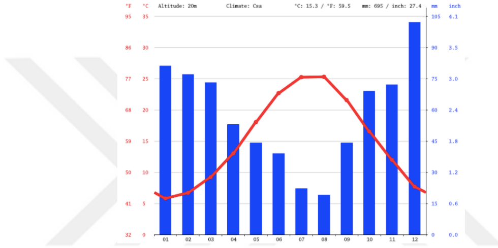
Şekil 4.5. Bandırma İlçesi yıllık yağış ve sıcaklık verileri (Anonim 10, 2021).
