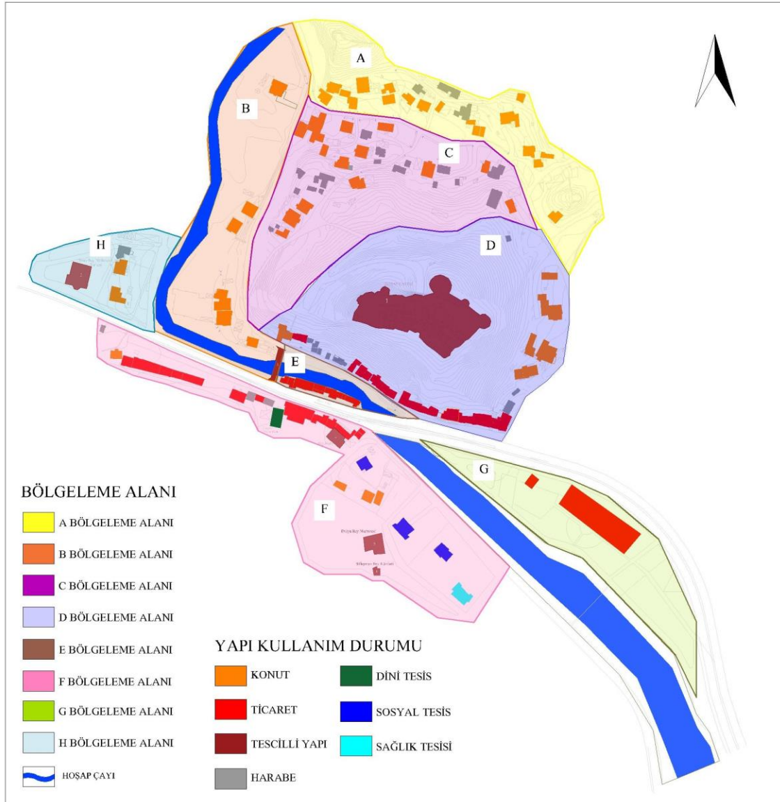
Şekil 5.1. Hoşap Kalesi ve çevresi bölgeleme alanı paftası.
