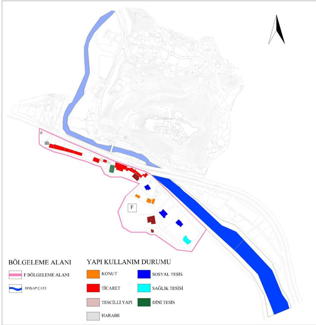
Şekil 5.29. Yapı kullanım durumu paftası.
