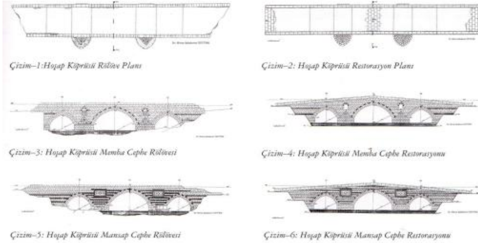
Şekil 4.6. Hoşap Evliya Bey Köprüsü plan ve görünüşler (Öztürk, 2009a).
