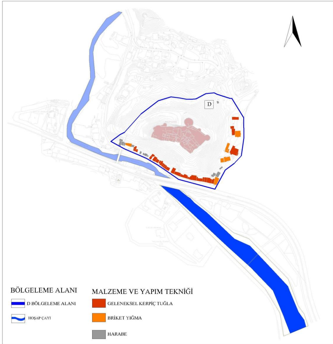
Şekil 5.20. Malzeme ve yapım tekniği paftası.
